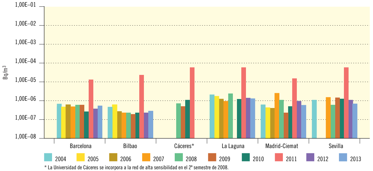
Figura 3.5b. Red de alta sensibilidad. Partículas de polvo en el aire. Muestreador alto flujo
