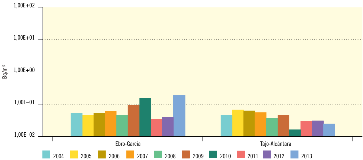
Figura 3.62a. Red de alta sensibilidad. Agua superficial
