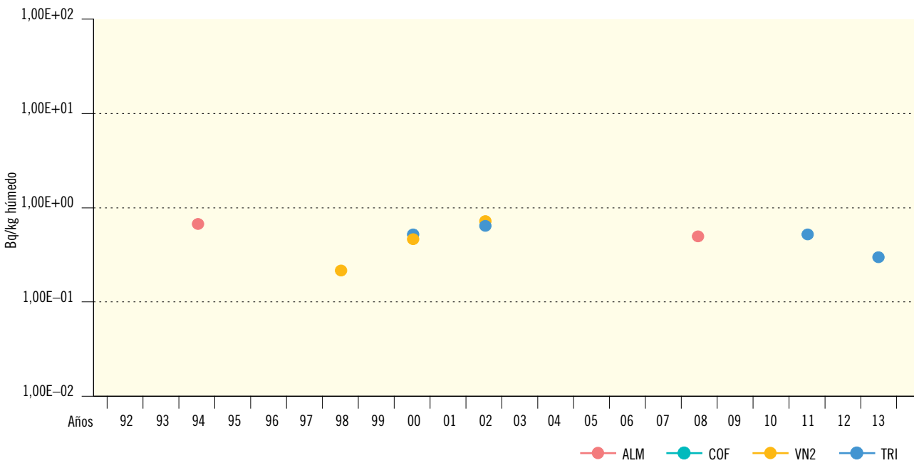
Figura 2.31b. Miel. Concentración de actividad de Cs-137 (Bq/kg húmedo)
