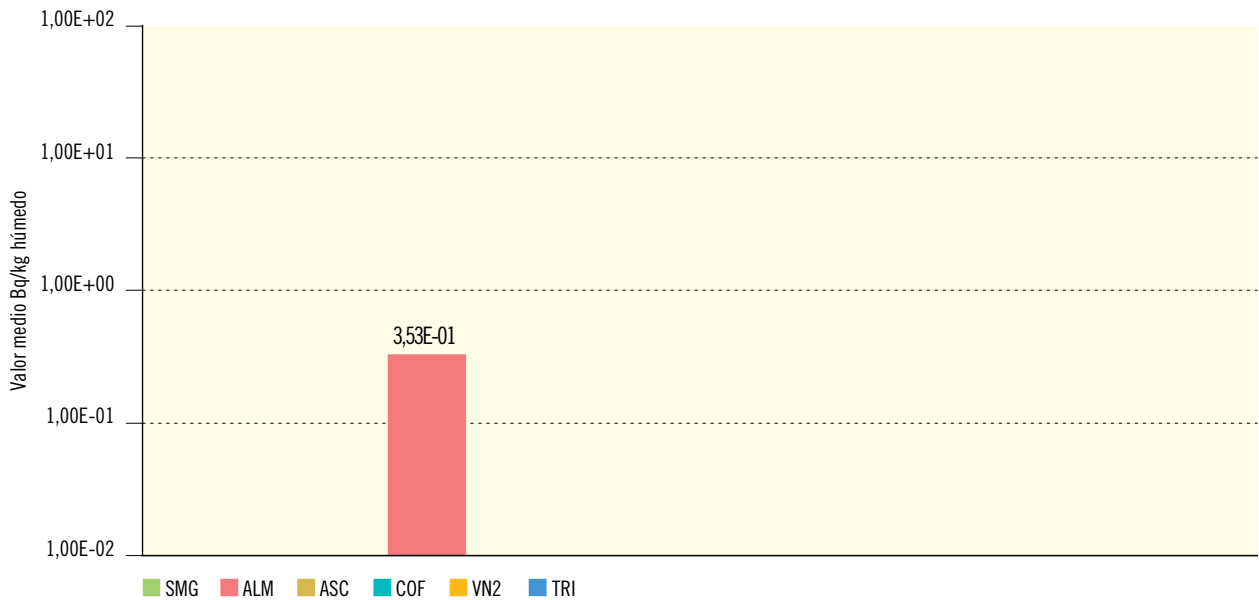
Figura 2.33b. Peces y mariscos. Evolución de la concentración de actividad de Cs-134
