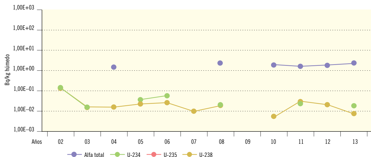
Figura 2.46. Juzbado. Carne y aves. Valores de concentración de actividad (Bq/kg húmedo)
