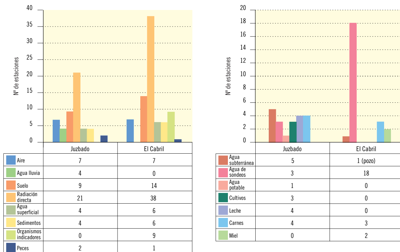
Figura 2.34. Número de estaciones de muestreo en los PVRA de las instalaciones del ciclo de combustible
