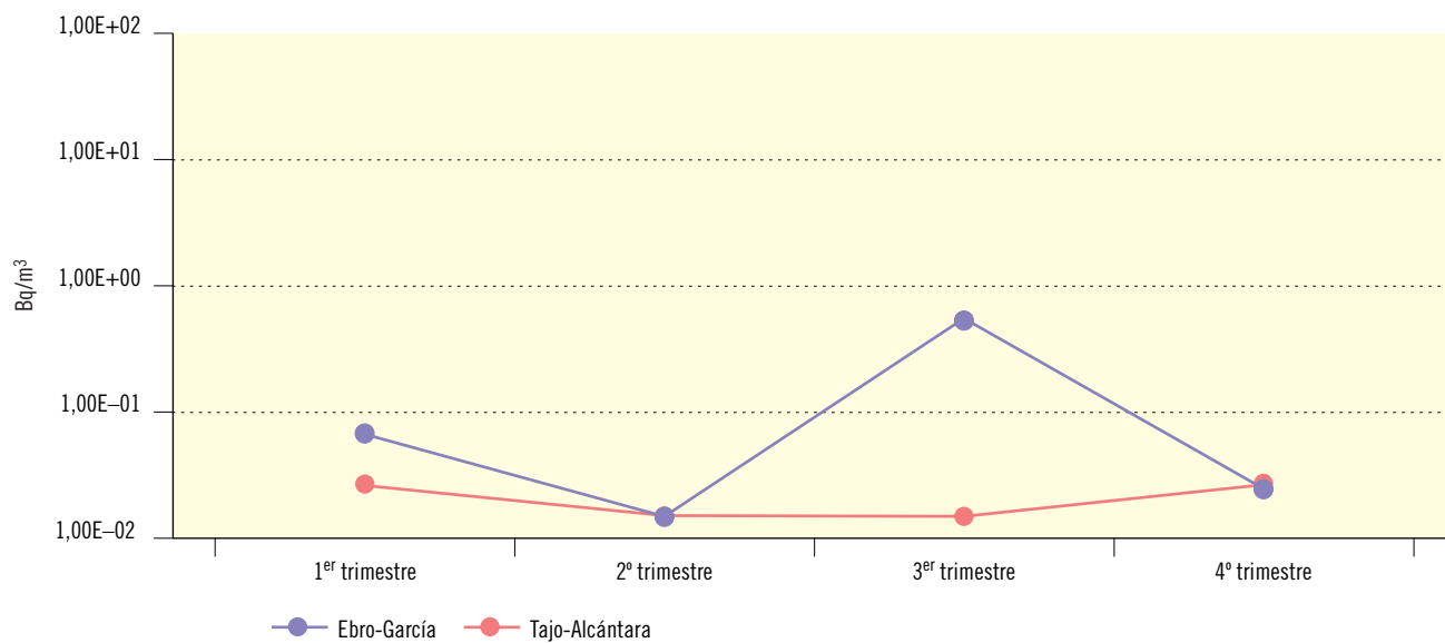
Figura 3.62b. Red de alta sensibilidad. Agua superficial. Concentración de actividad Cs-137 (Bq/m 3 )
