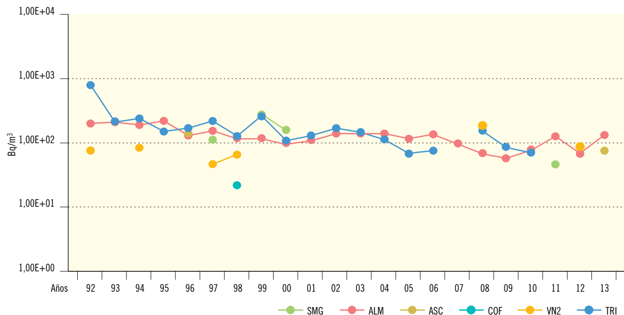
Figura 2.28b. Leche. Concentración de actividad de Cs-137 (Bq/m³)
