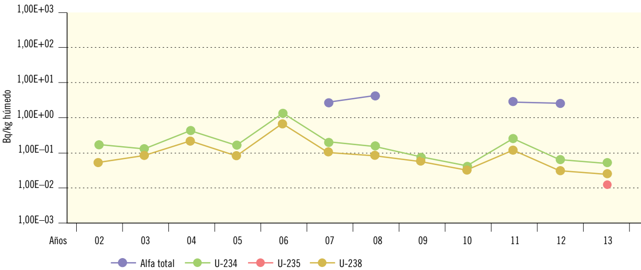
Figura 2.50. Juzbado. Peces. Valores de concentración de actividad (Bq/kg húmedo)
