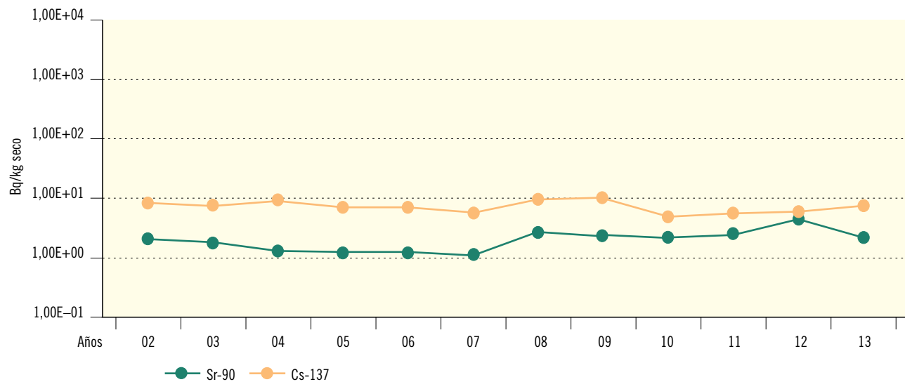
Figura 2.40. El Cabril. Suelo. Valores de concentración de actividad (Bq/kg seco)
