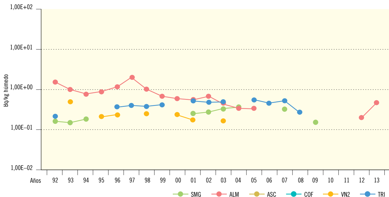
Figura 2.32b. Peces y mariscos. Concentración de actividad de Cs-137 (Bq/kg húmedo)
