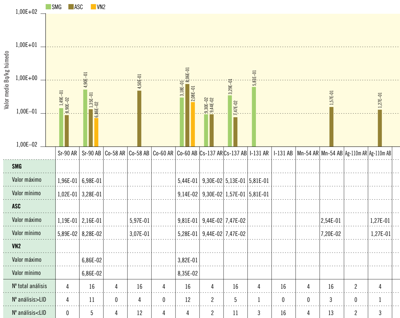
Figura 2.22b. Plantas acuáticas. Concentración de actividad (Bq/kg húmedo)
