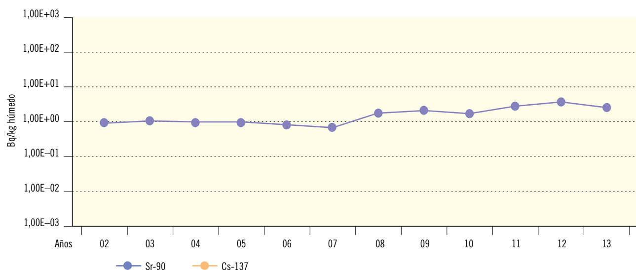
Figura 2.47. El Cabril. Carne y aves. Valores de concentración de actividad (Bq/kg húmedo)
