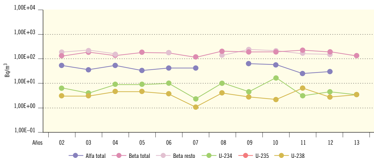
Figura 2.43. Juzbado. Agua potable. Valores de concentración de actividad (Bq/m 3 )
