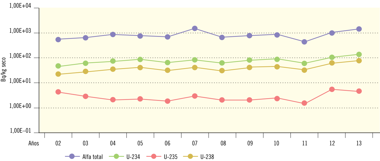
Figura 2.44. Juzbado. Sedimentos de fondo. Valores de concentración de actividad (Bq/kg seco)
