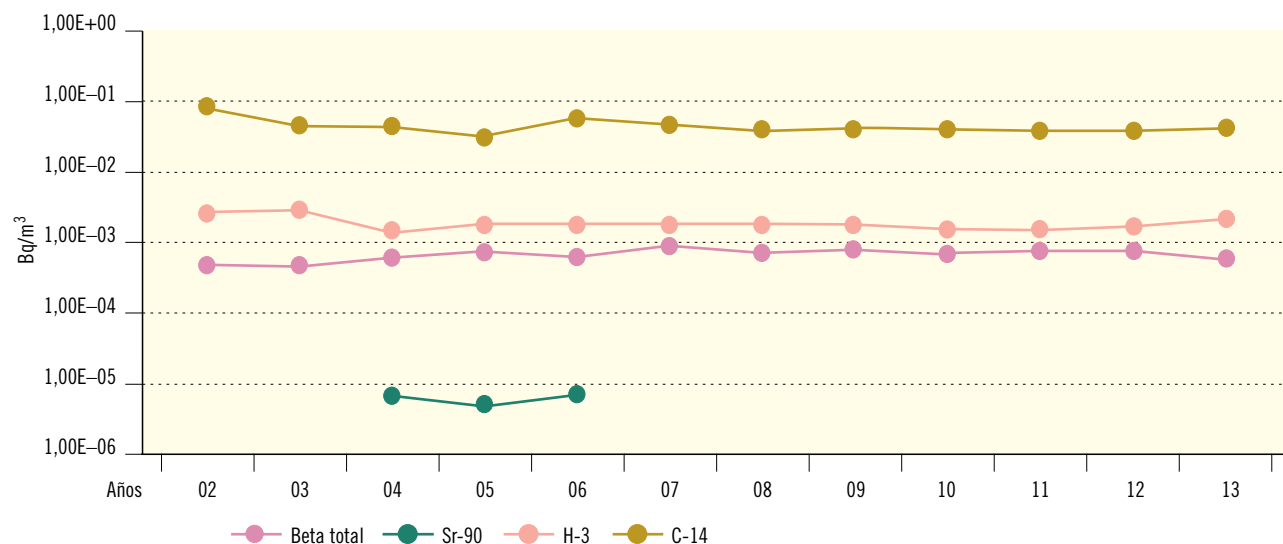
Figura 2.36. El Cabril. Partículas de polvo en el aire. Valores de concentración de actividad (Bq/m 3 )
