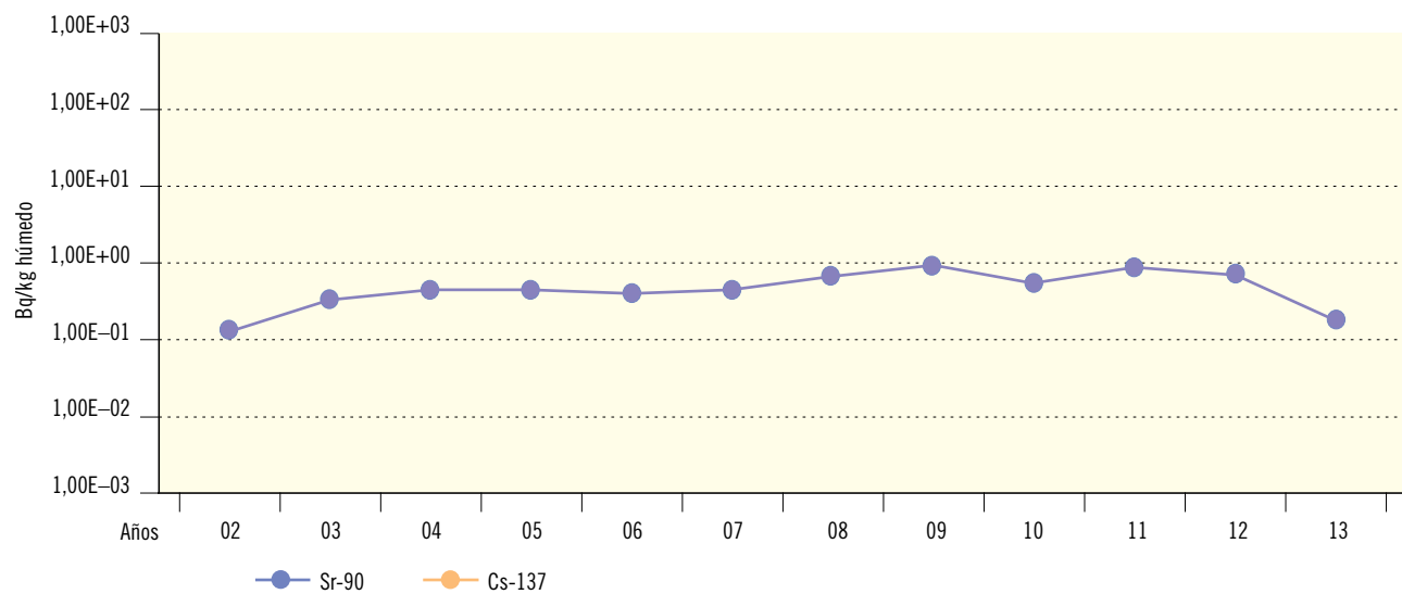
Figura 2.51. El Cabril. Peces. Valores de concentración de actividad (Bq/kg húmedo)
