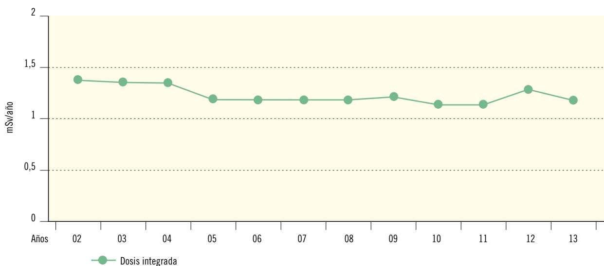
Figura 2.37. Juzbado. Radiación directa. Dosis integrada (DTL) (mSv/año)
