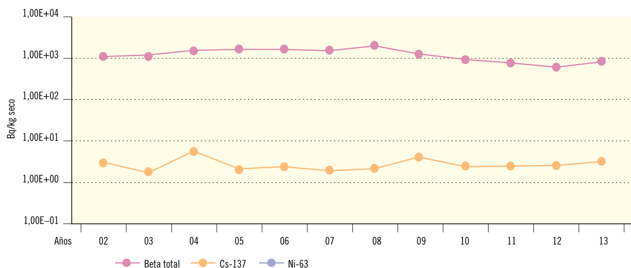
Figura 2.45. El Cabril. Sedimentos de fondo. Valores de concentración de actividad (Bq/kg seco)
