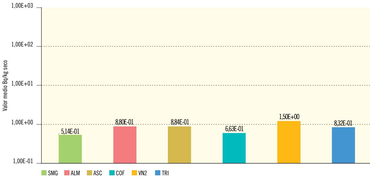
Figura 2.18b. Sedimentos de fondo. Concentración de actividad de Sr-90 (Bq/kg seco)
