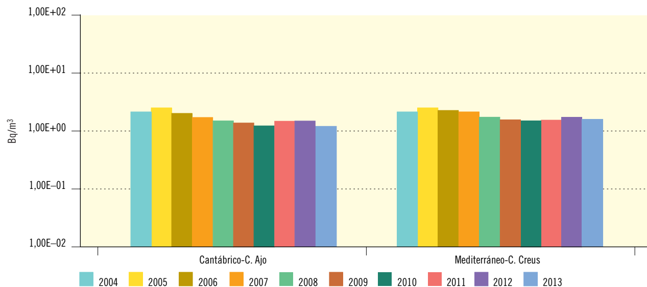
Figura 3.68a. Red de alta sensibilidad. Agua de mar
