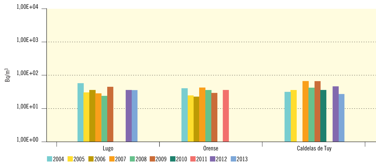
Figura 3.26. Río Miño Evolución temporal del índice de actividad alfa total
