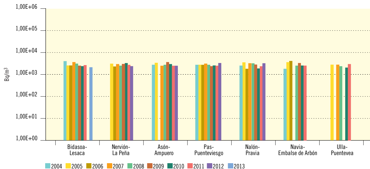
Figura 3.25. Cuencas del norte de España
