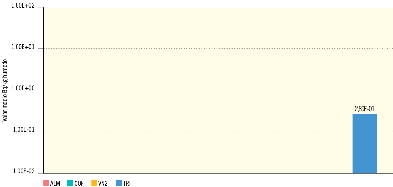
Figura 2.31b. Miel. Concentración de actividad de Cs-137 (Bq/kg húmedo)
