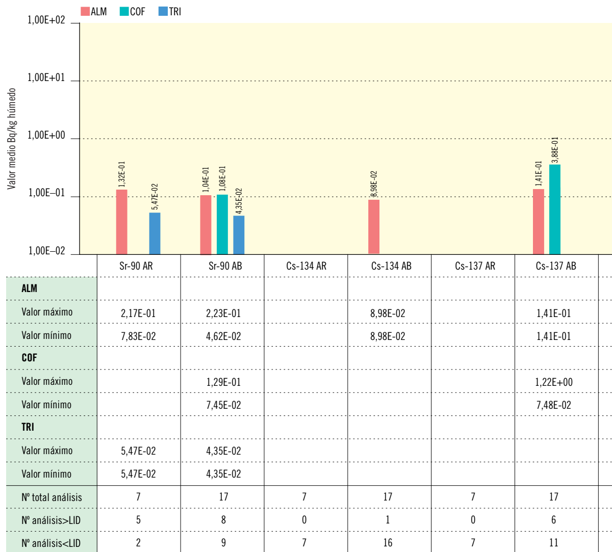
Figura 2.23b. Plantas de orilla. Concentración de actividad (Bq/kg húmedo)
