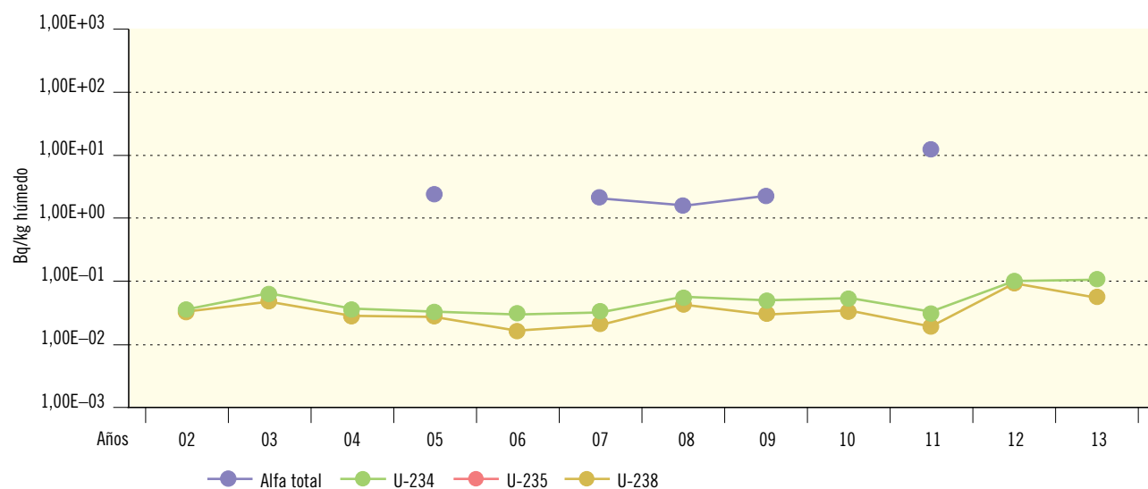
Figura 2.48. Juzbado. Vegetales de hoja no ancha. Valores de concentración de actividad (Bq/kg húmedo)
