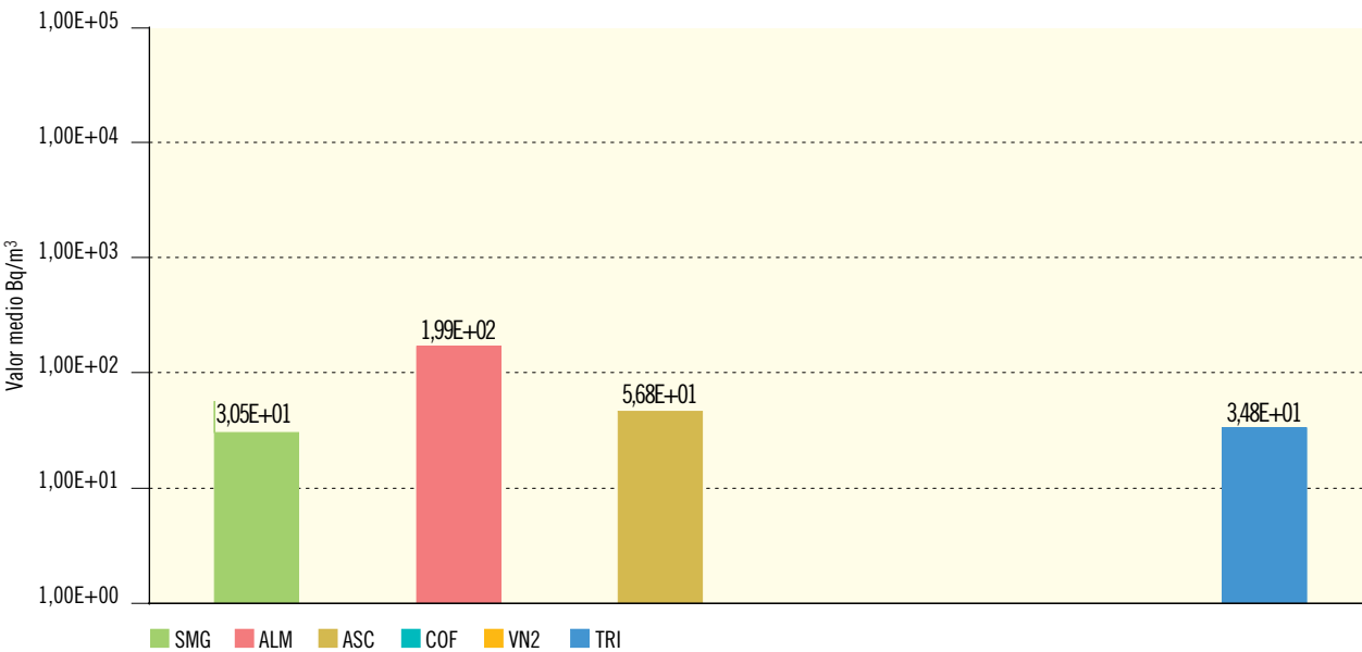
Figura 2.16b. Agua potable. Concentración del índice de actividad beta resto (Bq/m³)
