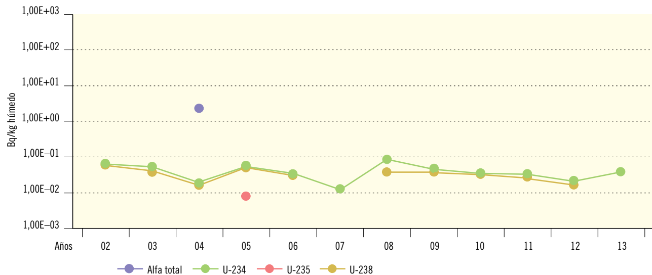
Figura 2.49. Juzbado. Vegetales de hoja ancha. Valores de concentración de actividad (Bq/kg húmedo)
