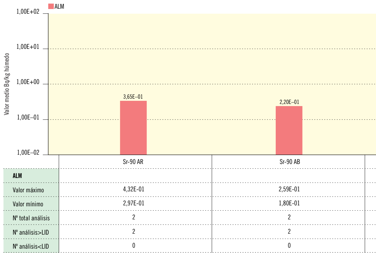
Figura 2.24b. Plantas terrestres. Concentración de actividad (Bq/kg húmedo) Valores de la campaña de 2013
