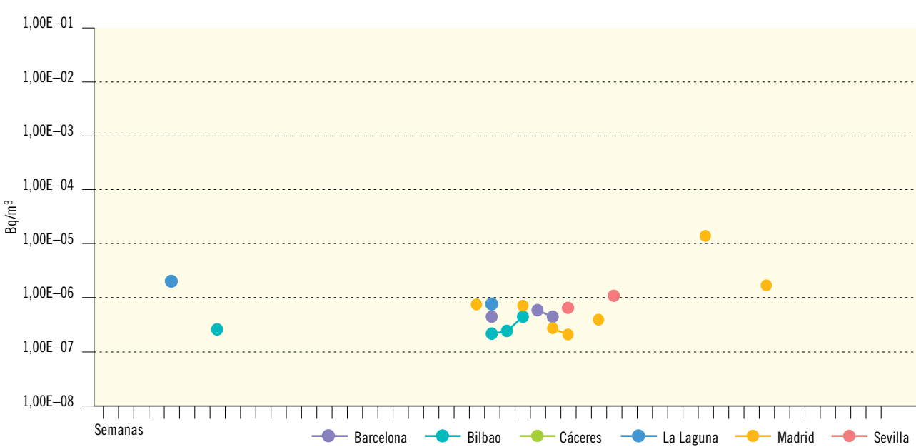
Figura 3.5b. Red de alta sensibilidad. Partículas de polvo en el aire. Muestreador alto flujo
