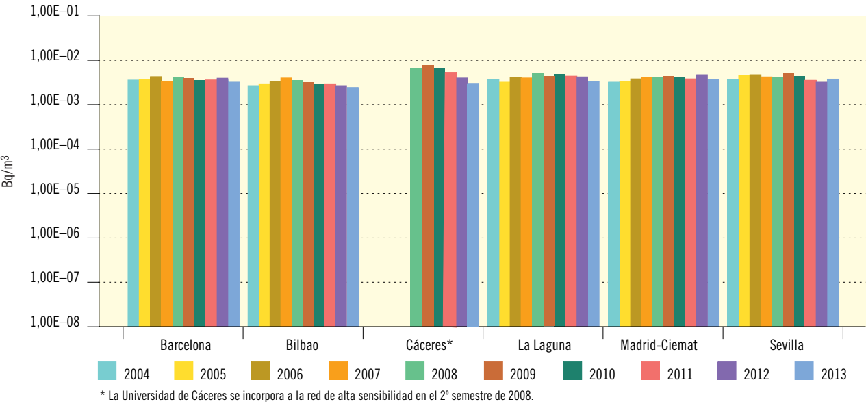
Figura 3.6b. Red de alta sensibilidad. Partículas de polvo en el aire. Muestreador alto flujo
