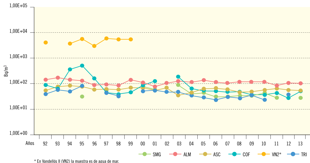
Figura 2.13b. Agua superficial. Concentración del índice de actividad beta resto (Bq/m³)
