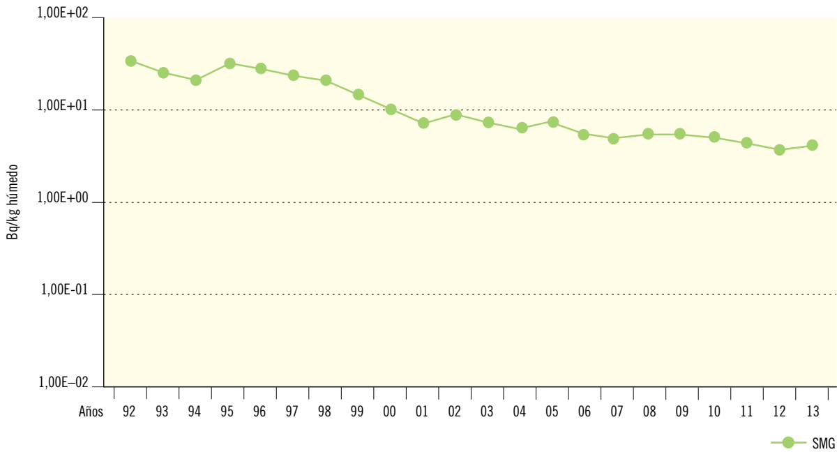
Figura 2.26b. Fauna terrestre. Concentración de actividad (Bq/kg húmedo)
