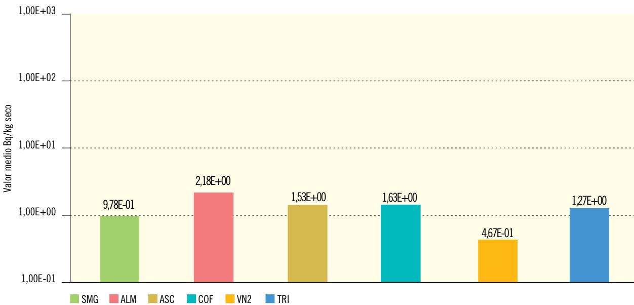
Figura 2.20b. Sedimentos de fondo. Concentración de actividad de Co-60 (Bq/kg seco)
