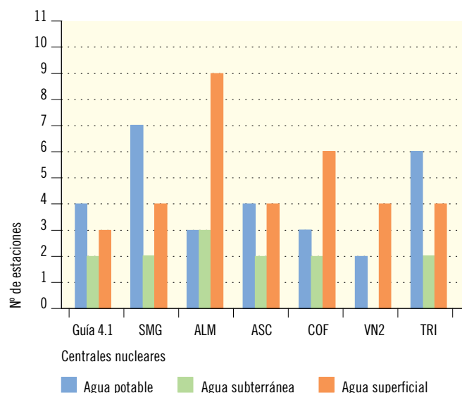
Figura 2.5. Número de estaciones de muestreo en los PVRA de las centrales nucleares. Año 2013
