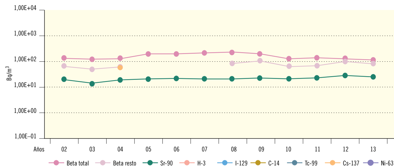
Figura 2.42. El Cabril. Agua superficial. Valores de concentración de actividad (Bq/m 3 )
