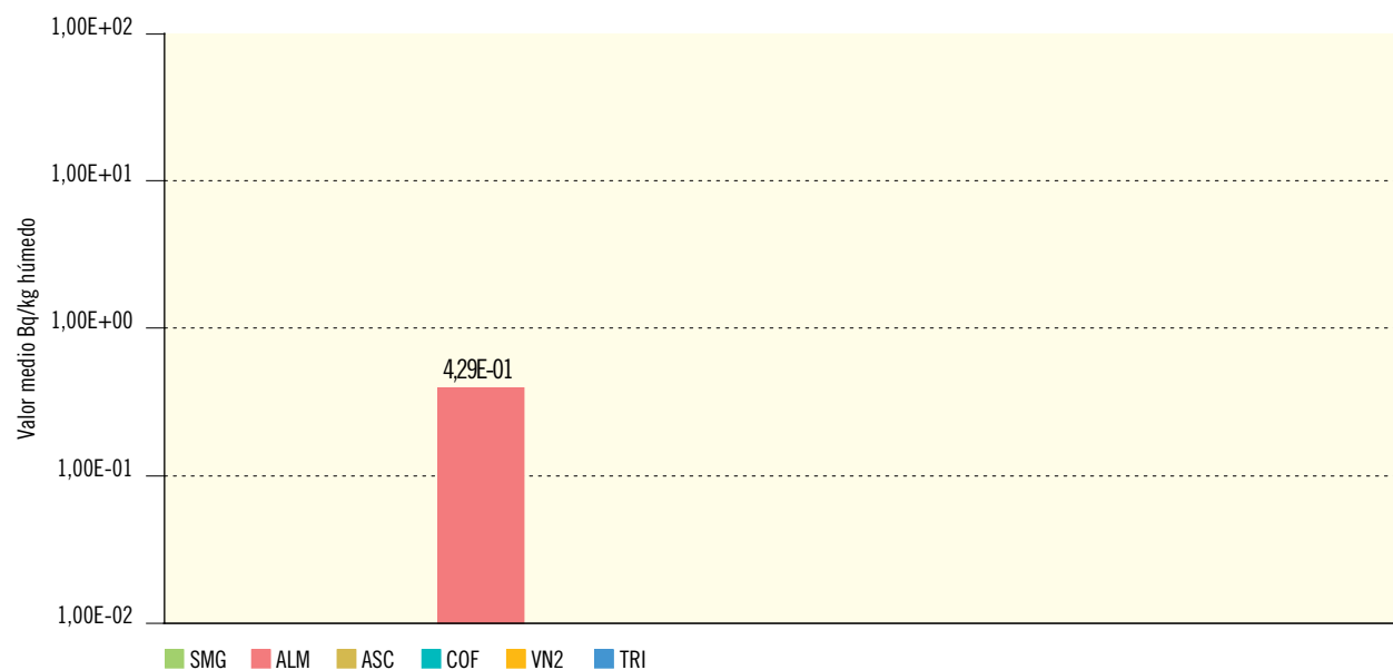
Figura 2.32b. Peces y mariscos. Concentración de actividad de Cs-137 (Bq/kg húmedo)
