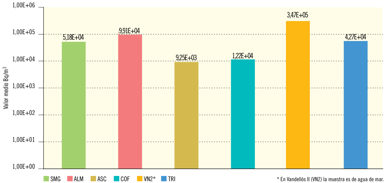
Figura 2.14b. Agua superficial. Concentración de actividad de H-3 (Bq/m³) Valores de la campaña de 2013
