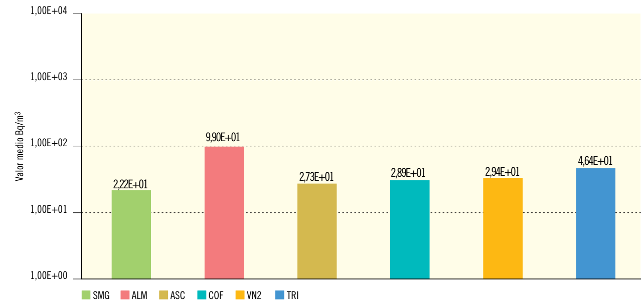
Figura 2.27b. Leche. Concentración de actividad de Sr-90 (Bq/m³)
