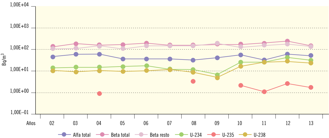
Figura 2.41. Juzbado. Agua superficial. Valores de concentración de actividad (Bq/m³) Evolución temporal valores medios
