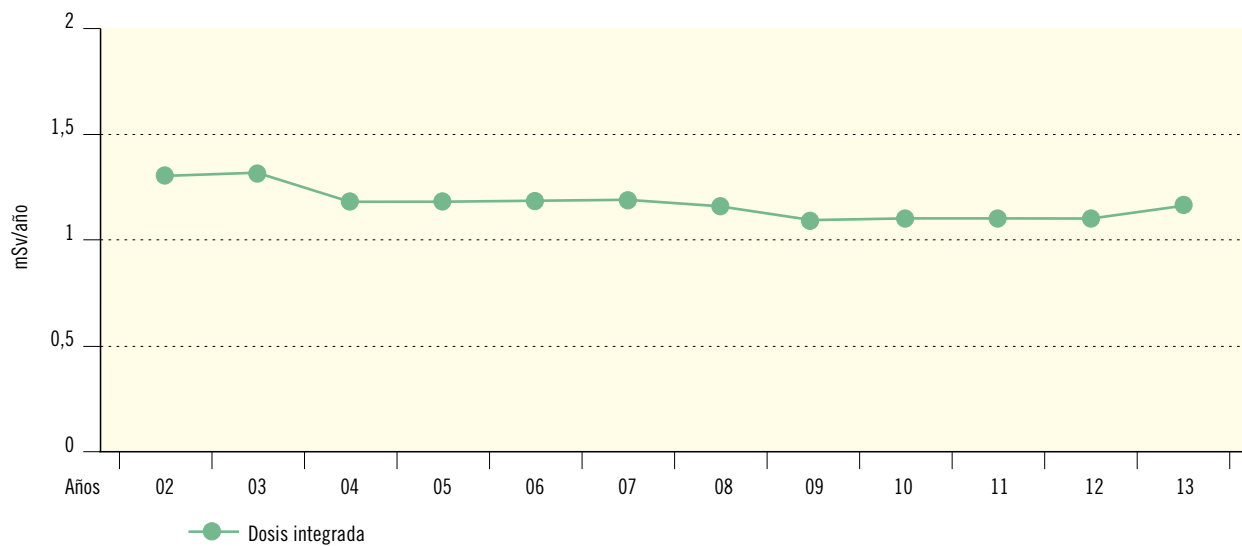
Figura 2.38. El Cabril. Radiación directa. Dosis integrada (DTL) (mSv/año)
