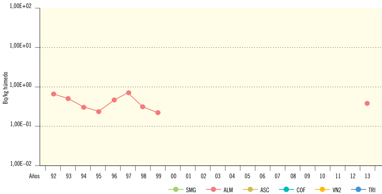
Figura 2.33b. Peces y mariscos. Evolución de la concentración de actividad de Cs-134
