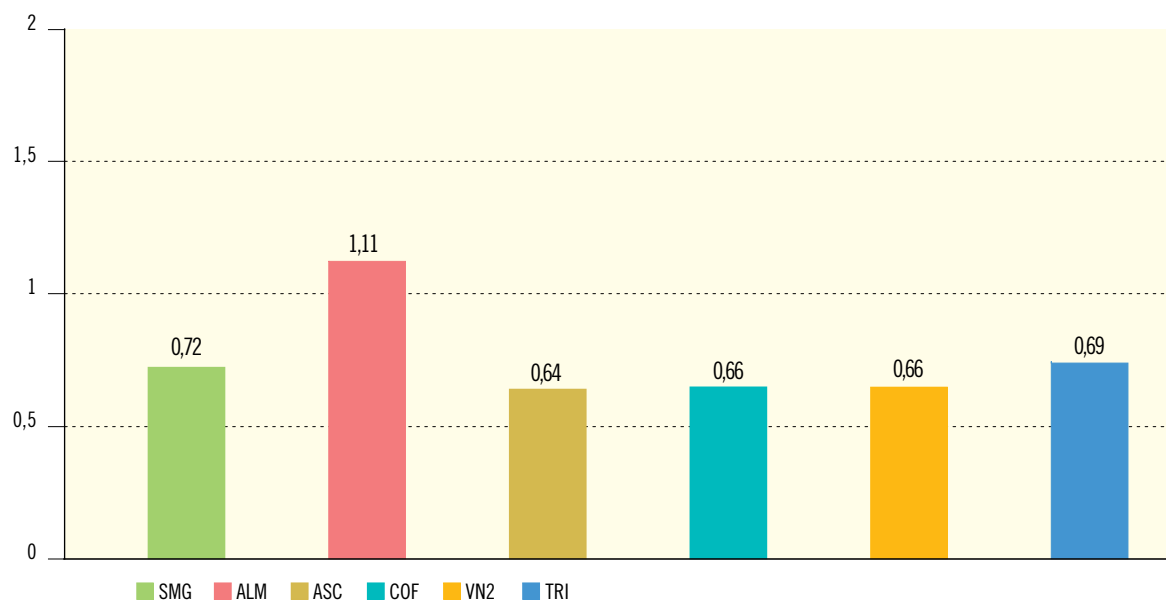
Figura 2.9b. Radiación directa. Dosis integrada (DTL) (mSv/año)
