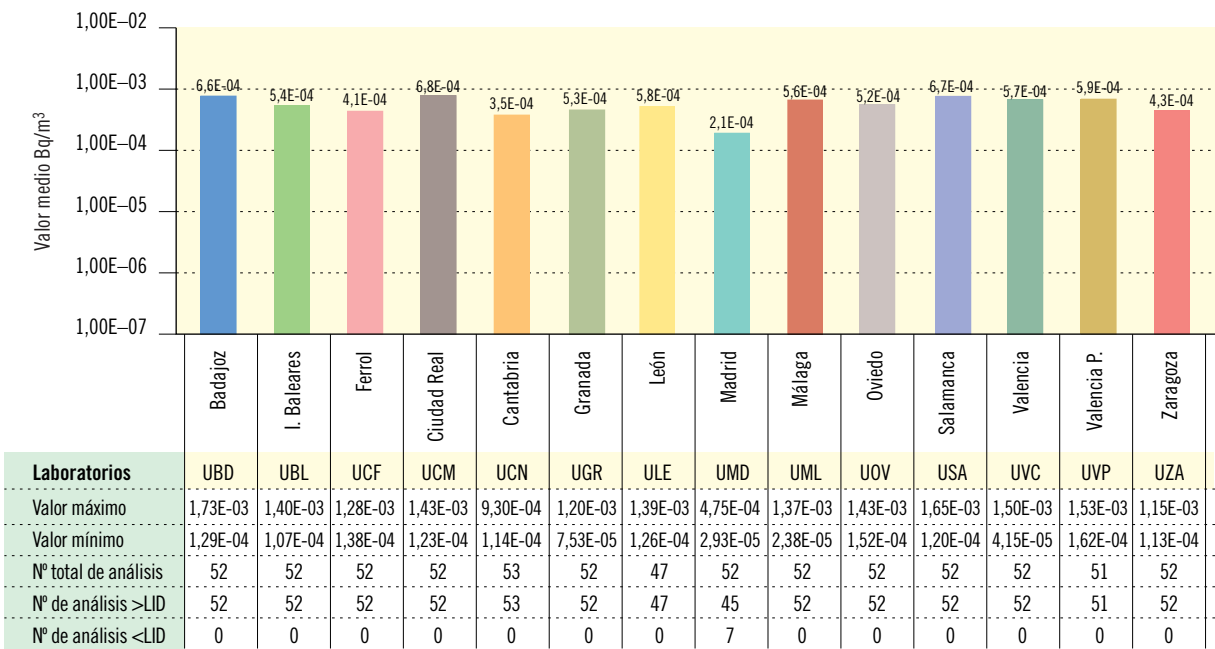
Figura 3.3b. Partículas de polvo en el aire. Concentración del índice de actividad beta total (Bq/m³) Valores de la campaña de 2013
