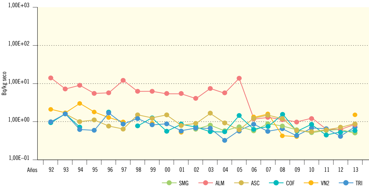
Figura 2.18b. Sedimentos de fondo. Concentración de actividad de Sr-90 (Bq/kg seco)
