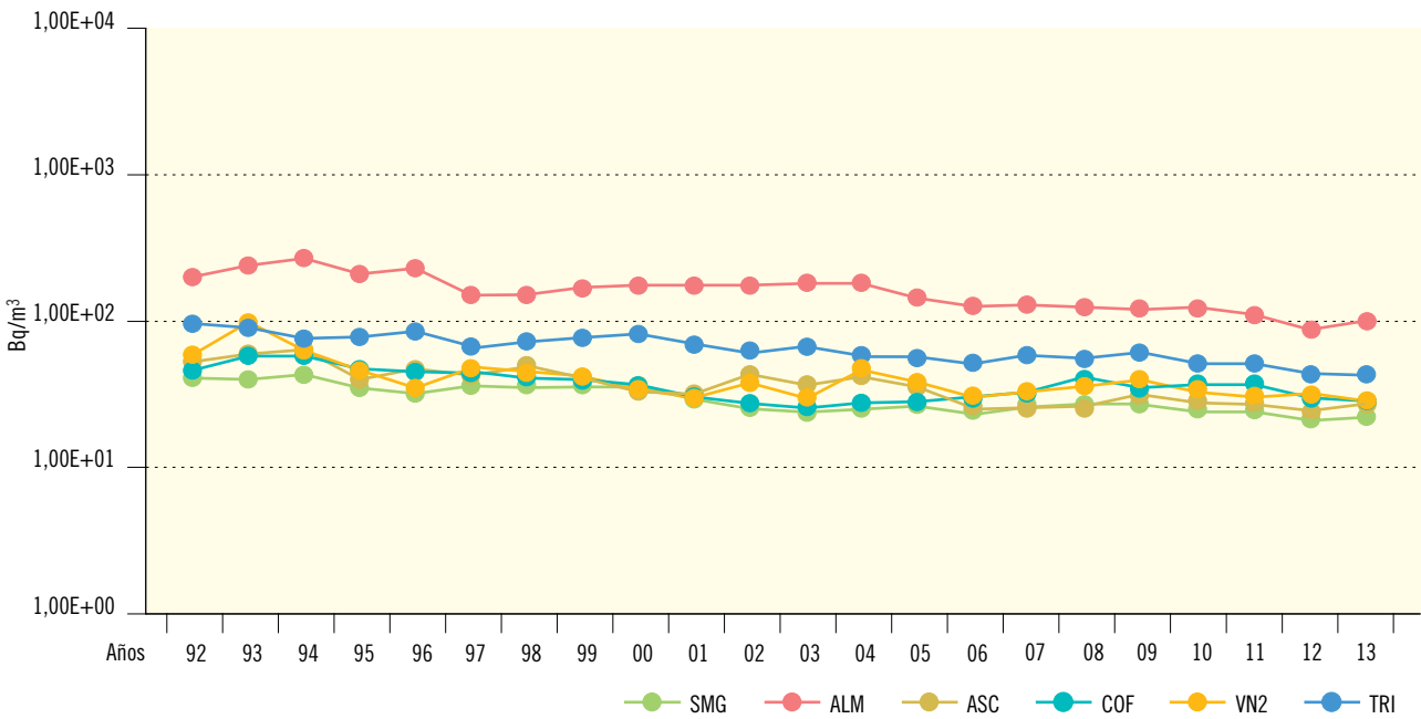
Figura 2.27b. Leche. Concentración de actividad de Sr-90 (Bq/m³)
