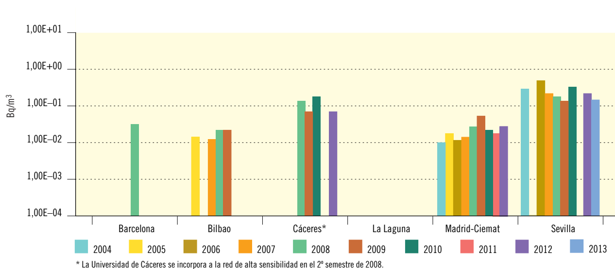
Figura 3.15b. Red de alta sensibilidad. Agua potable. Concentración de actividad de Cs-137 (Bq/m³)
