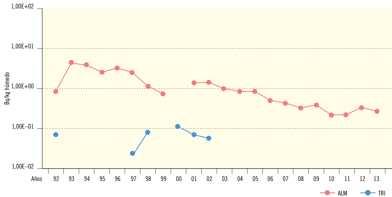
Figura 2.24b. Plantas terrestres. Concentración de actividad (Bq/kg húmedo) Valores de la campaña de 2013
