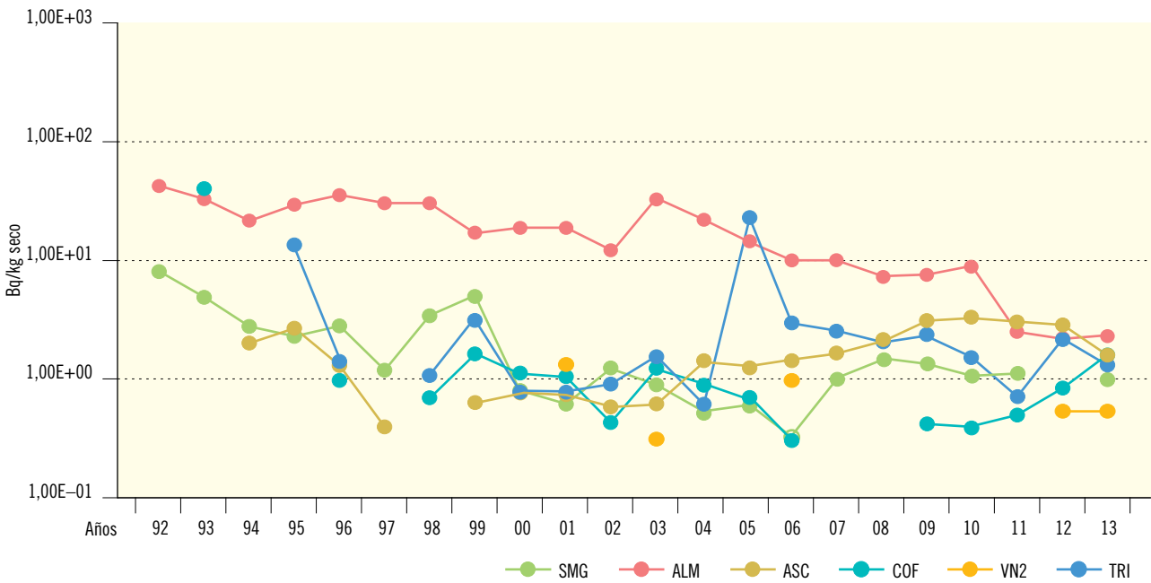
Figura 2.20b. Sedimentos de fondo. Concentración de actividad de Co-60 (Bq/kg seco)
