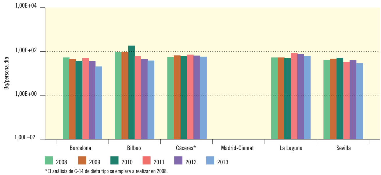
Figura 3.20b. Red de alta sensibilidad. Dieta tipo. Concentración de actividad de C-14 (Bq/persona.día)
