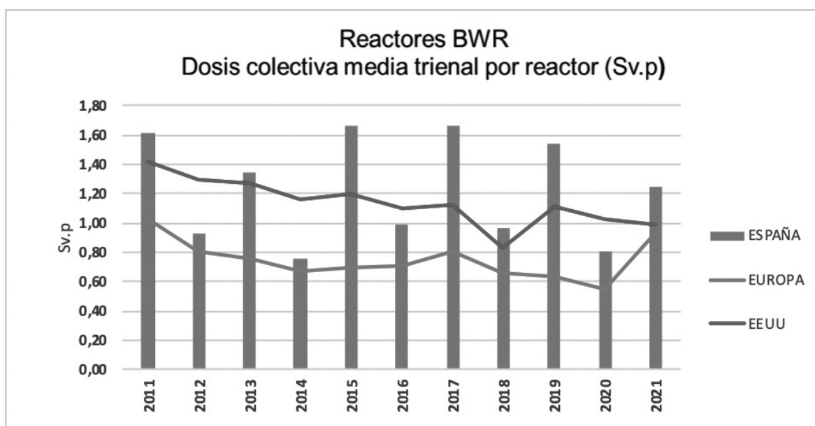
Figura 15.A.2. Dosis colectiva trienal media (Sv-persona) para reactores de tipo BWR. Comparación internacional.
