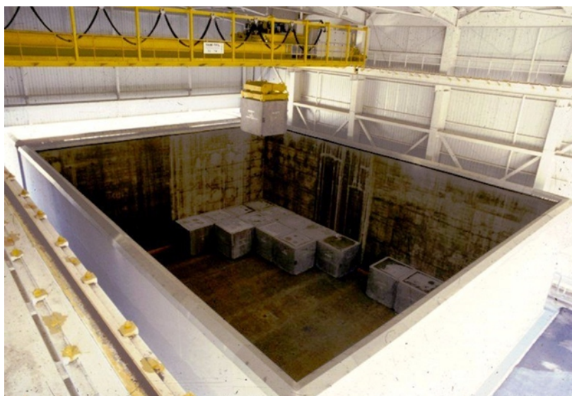
Imagen de carga de contenedor en celda de RBMA del centro de almacenamiento de El Cabril.
