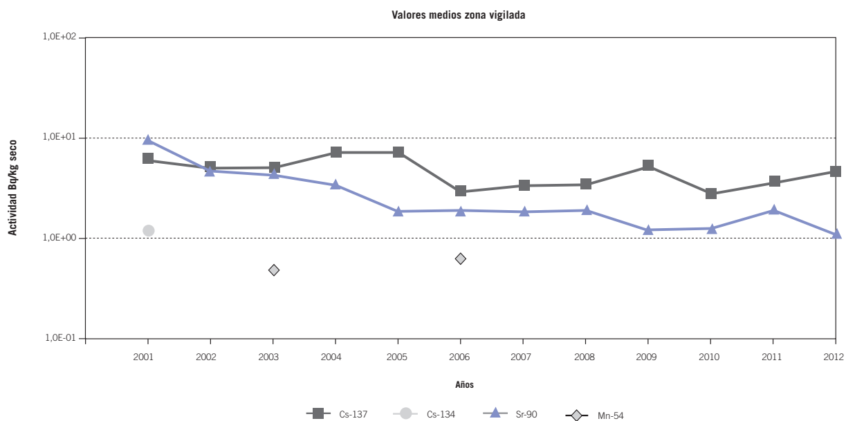
Figura 4.4.1.3. Evolución temporal de la actividad radiológica en suelo en la instalación Vandellós I
