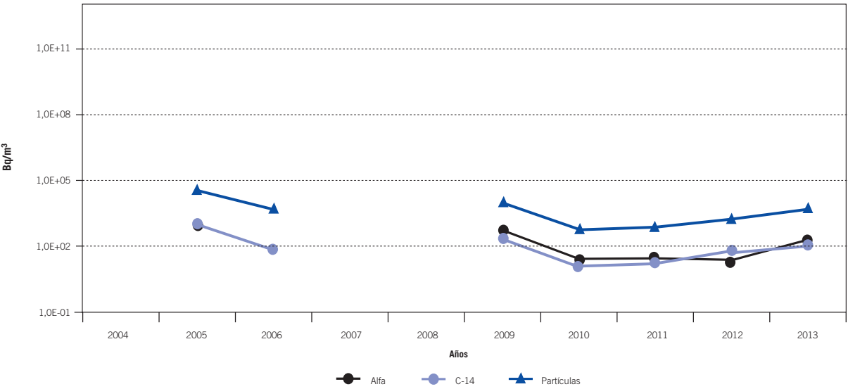
Figura 4.4.1.2. Evolución temporal de la actividad radiológica en aire en la instalación Vandellós I
