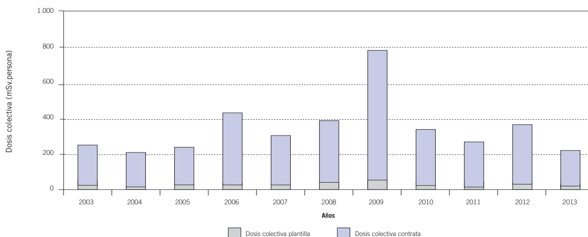
Figura 4.2.6.6.1. Distribución de dosis colectiva para la central nuclear de Trillo
