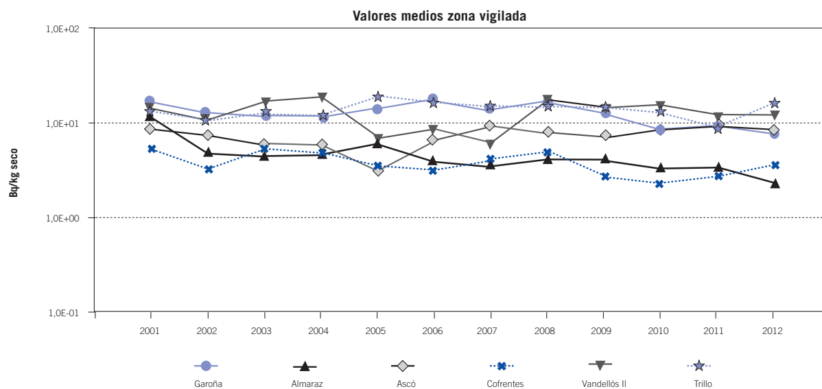
Figura 5.2.2.1.4. Muestras de suelo. Evolución temporal de Cs-137
