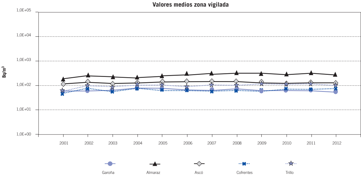
Figura 5.2.2.1.5. Muestras de agua potable. Evolución temporal de actividad beta total
