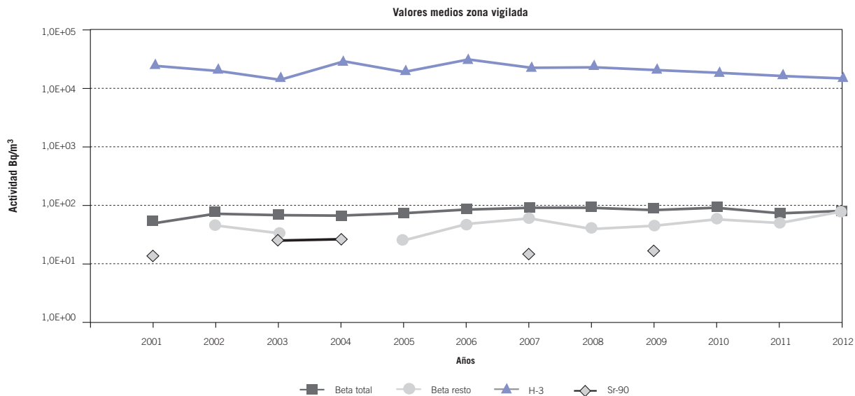
Figura 4.4.2.5. Resultados históricos de la vigilancia radiológica ambiental en agua potable en la central nuclear José Cabrera. Año 2012
