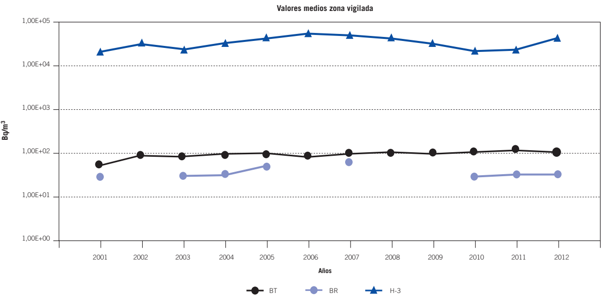
Figura 4.2.6.6.7. Muestras de agua potable. Evolución temporal de actividad beta total, beta resto y tritio. Central nuclear de Trillo
