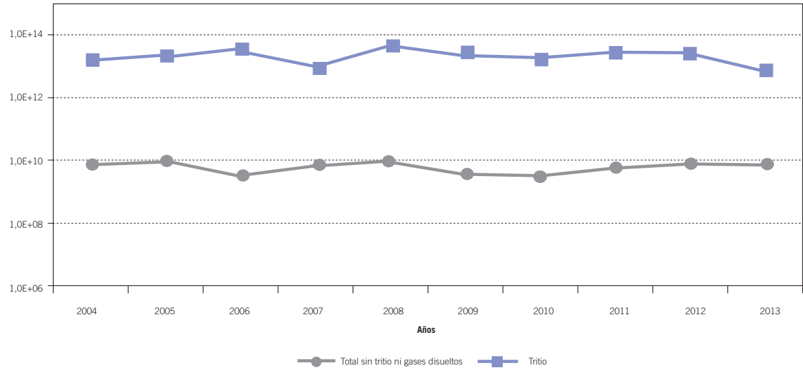
Figura 4.2.6.3.4. Central nuclear Ascó II. Actividad de efluentes radiactivos líquidos (Bq)
