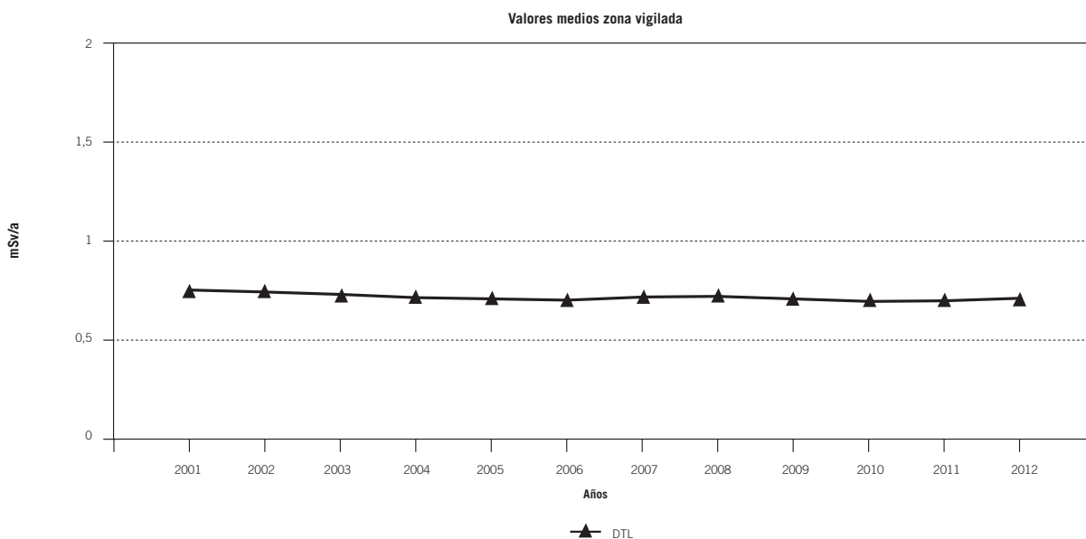
Figura 4.2.6.6.9. Radiación directa. Dosis integrada. Valores de los DTL. Central nuclear de Trillo
