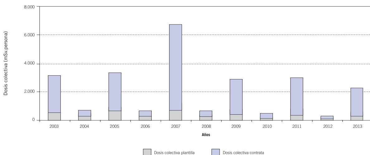
Figura 4.2.6.4.1. Distribución de dosis colectiva para la central nuclear de Cofrentes
