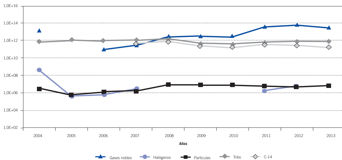
Figura 4.2.6.3.3. Central nuclear Ascó I. Actividad de efluentes radiactivos gaseosos (Bq)
