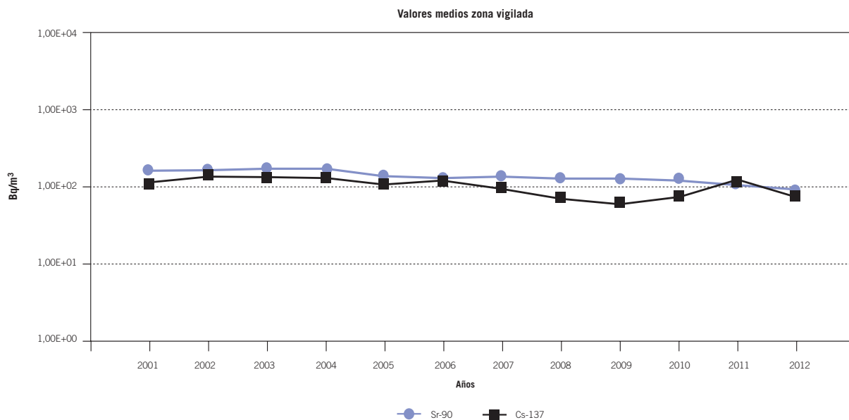
Figura 4.2.6.2.8. Muestras de leche. Evolución temporal de Sr-90 y CS-137. Central nuclear de Almaraz
