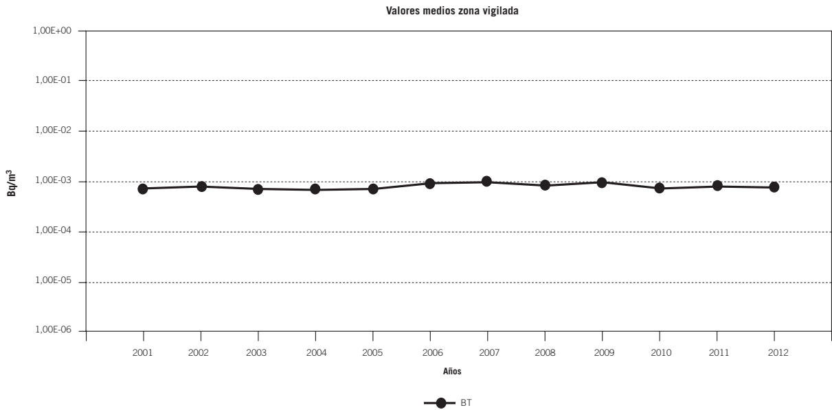
Figura 4.2.6.2.5. Aire. Evolución temporal del índice de actividad beta total. Central nuclear de Almaraz
