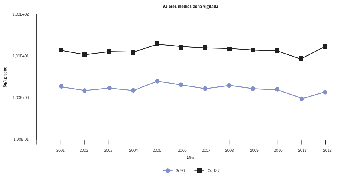
Figura 4.2.6.6.6. Muestras de suelo. Evolución temporal de Sr-90 y CS-137. Central nuclear de Trillo
