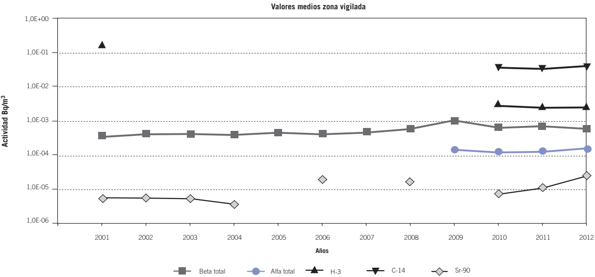
Figura 4.4.2.3. Resultados históricos de la vigilancia radiológica ambiental en aire en la central nuclear José Cabrera. Año 2012
