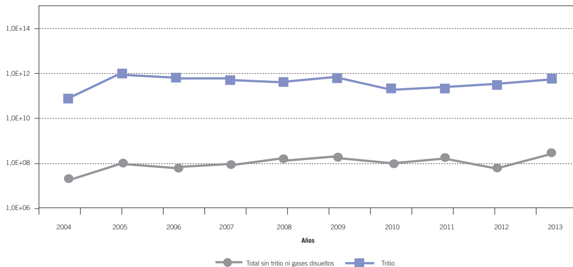
Figura 4.2.6.4.2. Central nuclear de Cofrentes. Actividad de efluentes radiactivos líquidos (Bq)
