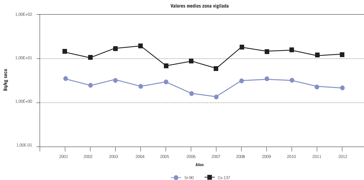
Figura 4.2.6.5.6. Muestras de suelo. Evolución temporal de Sr-90 y CS-137. Central nuclear Vandellós II
