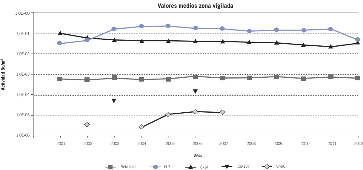
Figura 4.4.1.2. Evolución temporal de la actividad radiológica en aire en la instalación Vandellós I
