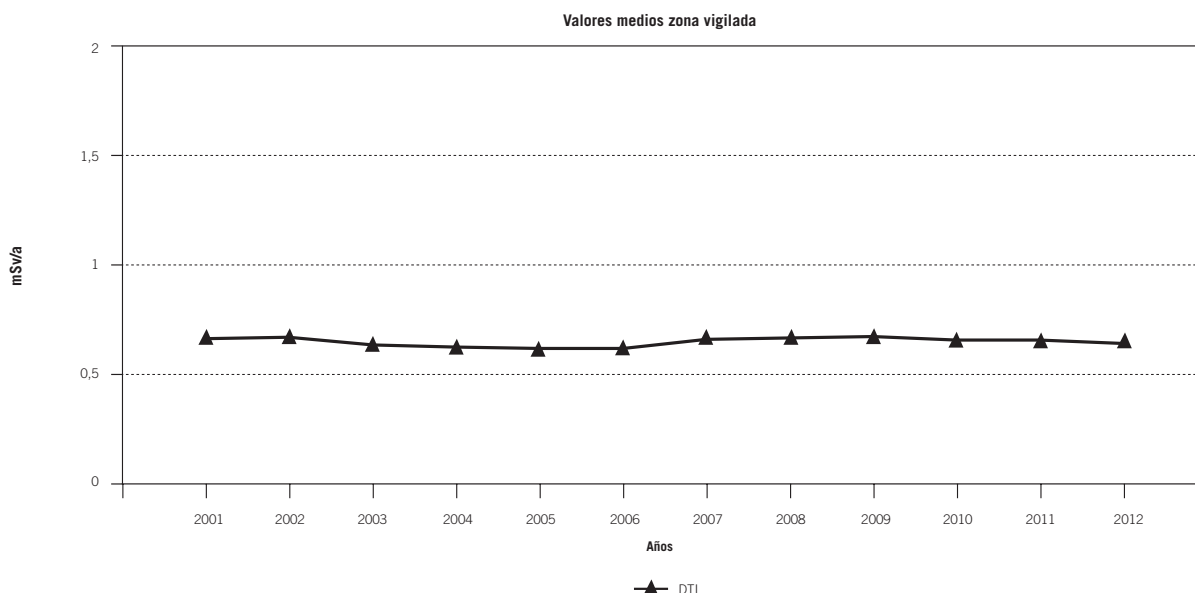
Figura 4.2.6.5.8. Radiación directa. Dosis integrada. Valores de los DTL. Central nuclear Vandellós II
