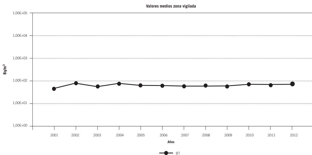
Figura 4.2.6.4.7. Muestras de agua potable. Evolución temporal de actividad beta total. Central nuclear de Cofrentes
