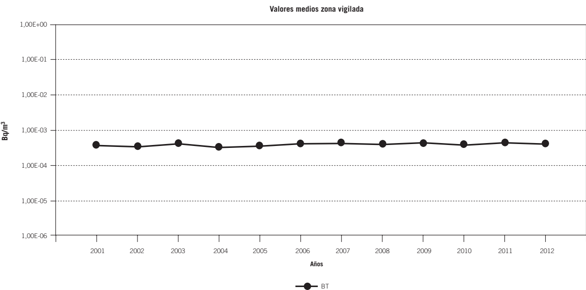
Figura 4.2.6.1.5. Aire. Evolución temporal del índice de actividad beta total. Central nuclear de Santa María de Garoña
