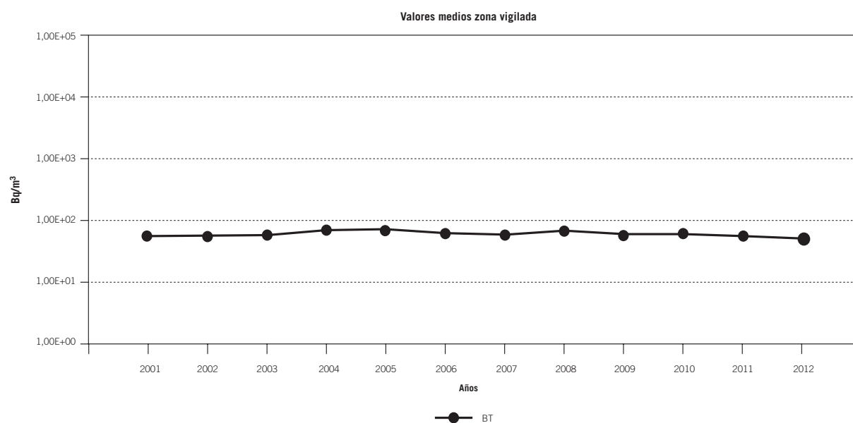
Figura 4.2.6.1.7. Muestras de agua potable. Evolución temporal de actividad beta total. Central nuclear de Santa María de Garoña
