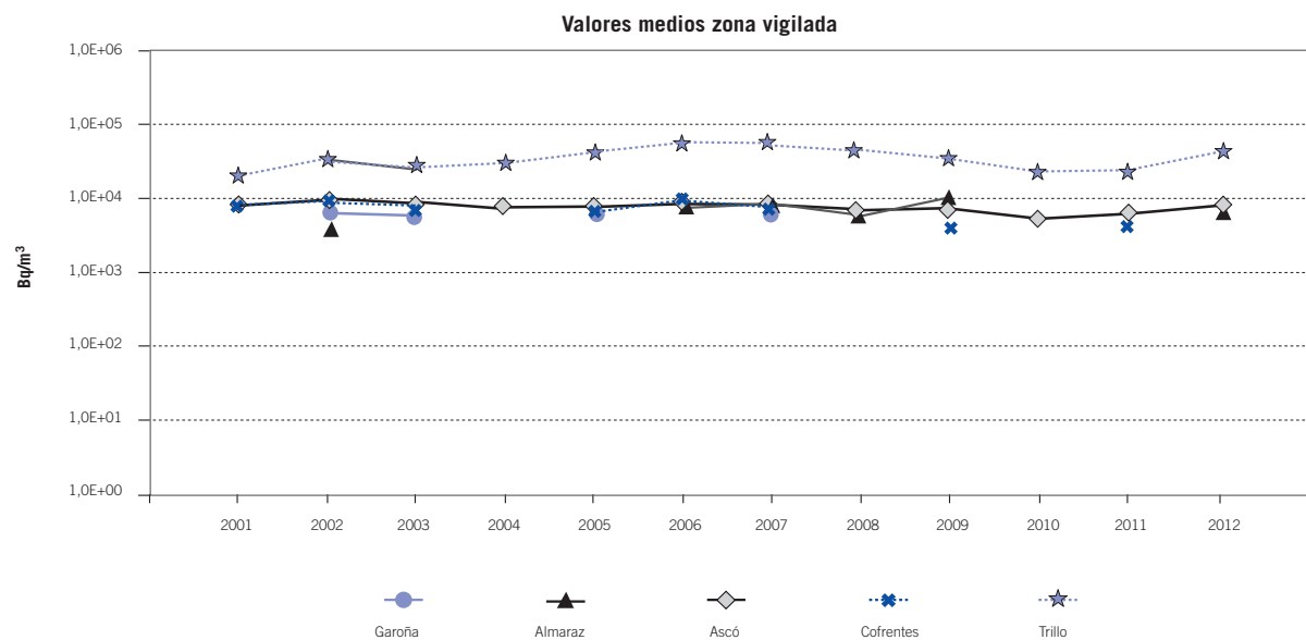
Figura 5.2.2.1.8. Muestras de agua potable. Evolución temporal de tritio
