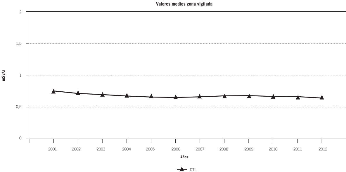
Figura 4.2.6.4.9. Radiación directa. Dosis integrada. Valores de los DTL. Central nuclear de Cofrentes
