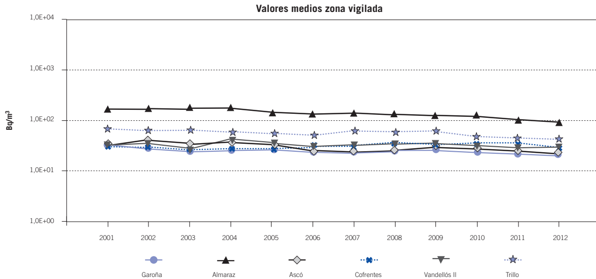
Figura 5.2.2.1.9. Muestras de leche. Evolución temporal del Sr-90
