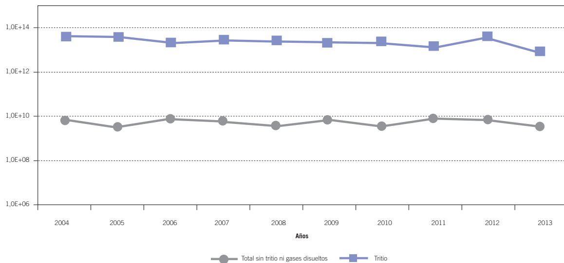
Figura 4.2.6.3.2. Central nuclear Ascó I. Actividad de efluentes radiactivos líquidos (Bq)
