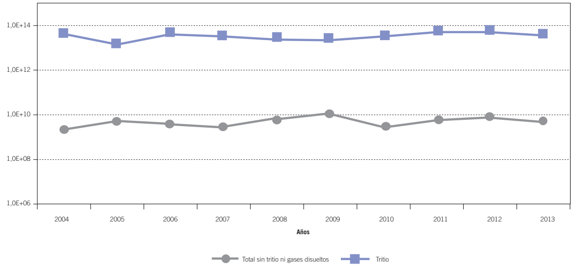
Figura 4.2.6.2.2. Central nuclear de Almaraz. Actividad de efluentes radiactivos líquidos (Bq)
