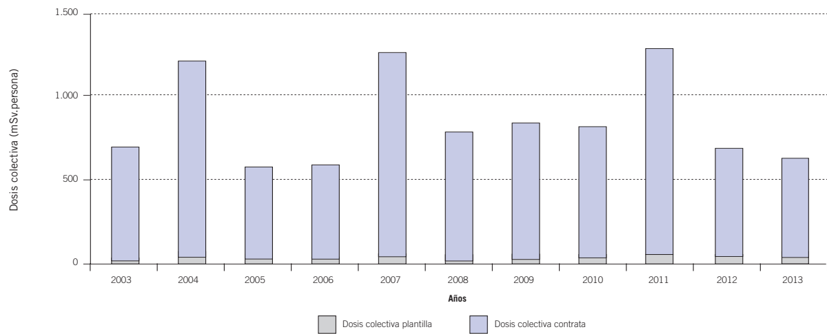
Figura 4.2.6.3.1. Distribución de dosis colectiva para la central nuclear de Ascó
