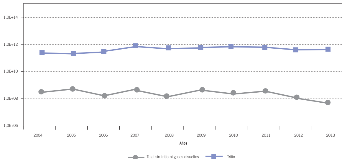
Figura 4.2.6.1.2. Central nuclear de Santa María de Garoña. Actividad de efluentes radiactivos líquidos (Bq)
