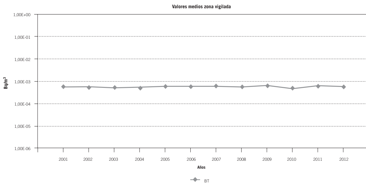
Figura 4.2.6.6.5. Aire. Evolución temporal del índice de actividad beta total. Central nuclear de Trillo
