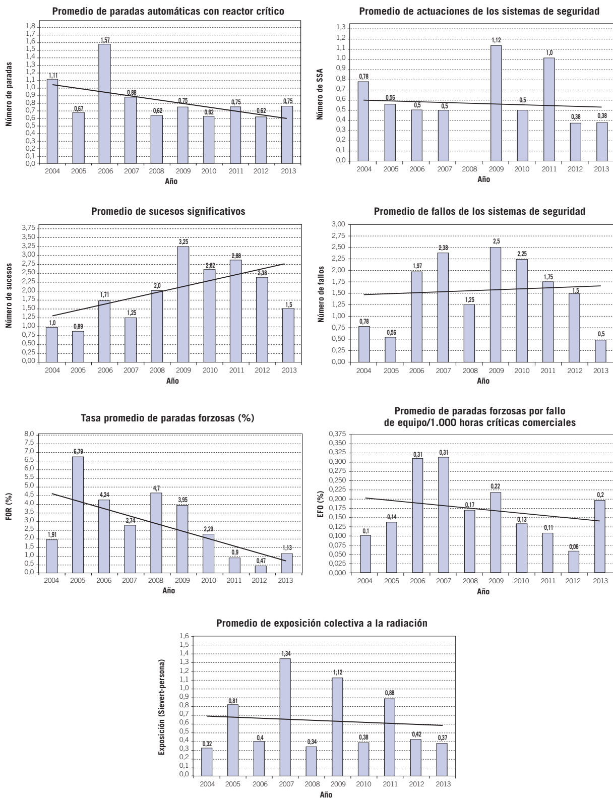
Figura 3.1.1.2.1. Indicadores de funcionamiento de las centrales nucleares
