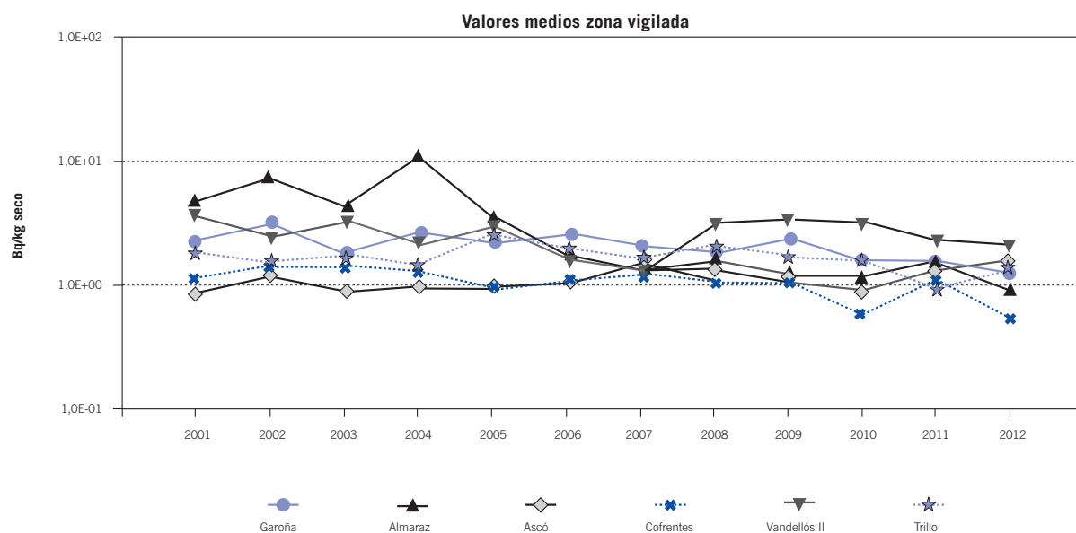
Figura 5.2.2.1.3. Muestras de suelo. Evolución temporal de Sr-90
