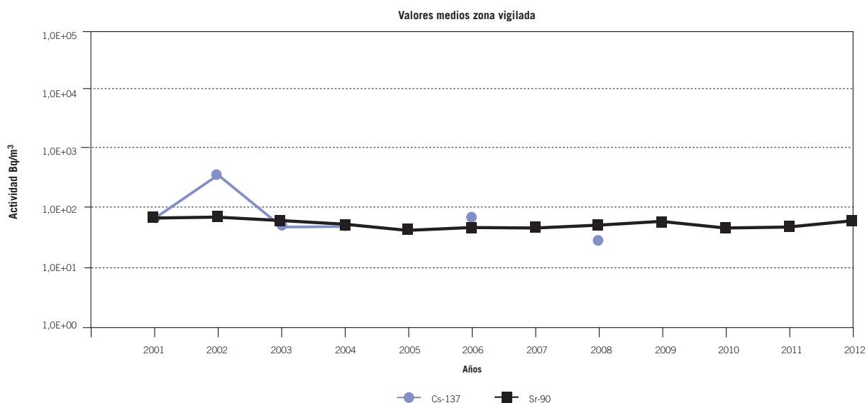
Figura 4.4.2.6. Resultados históricos de la vigilancia radiológica ambiental en leche en la central nuclear José Cabrera. Año 2012
