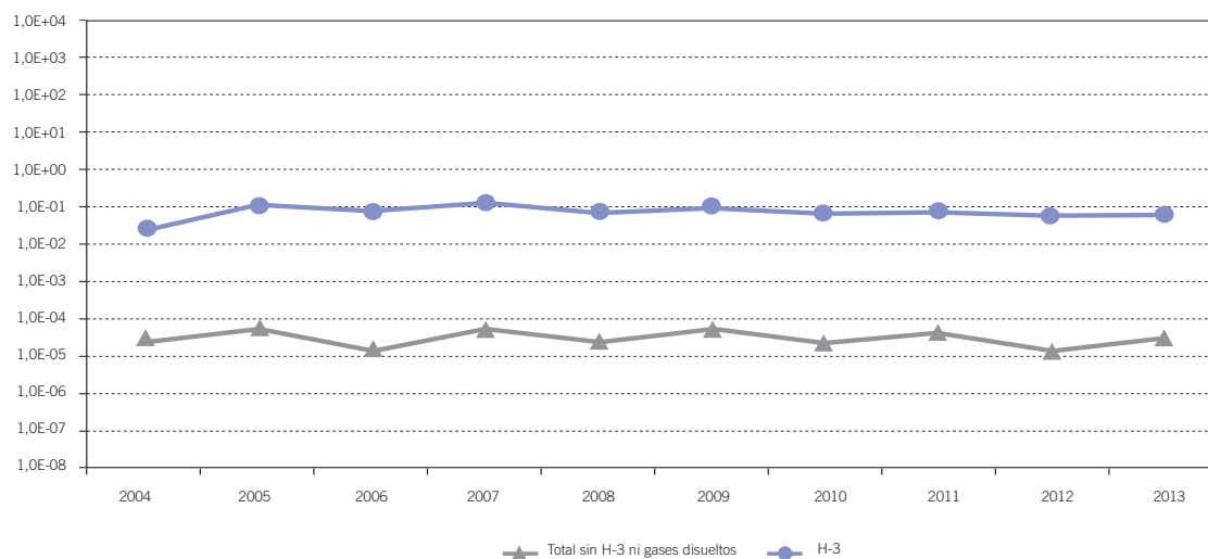
Figura 3.2.2.1.3. Efluentes radiactivos líquidos de centrales BWR. Actividad normalizada (GBq/GWh)
