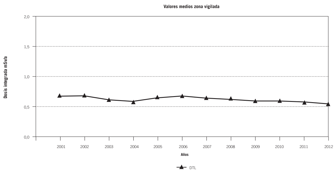
Figura 4.4.1.4. Evolución temporal de la tasa de radiación ambiental en la instalación Vandellós I
