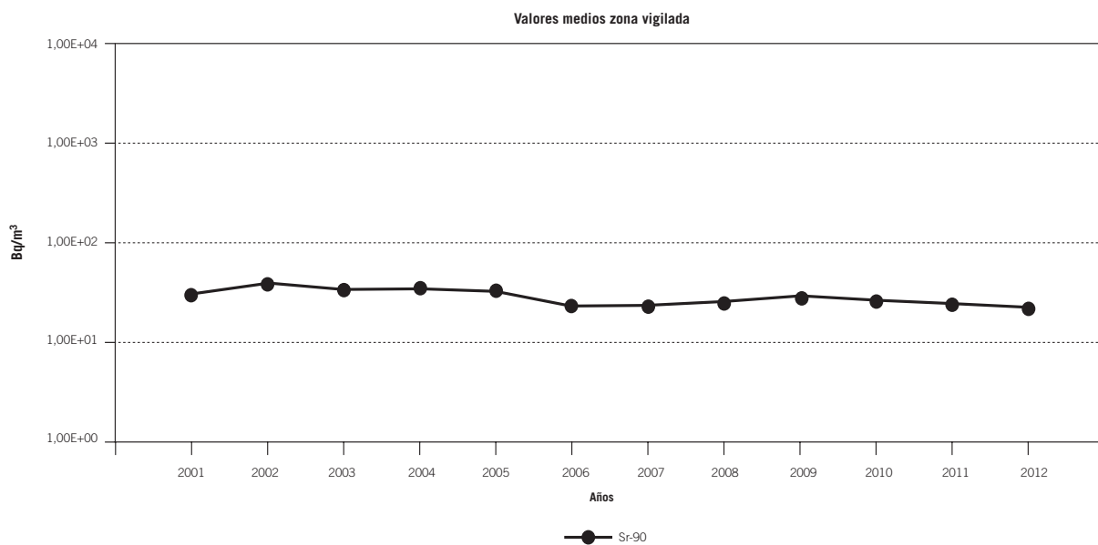
Figura 4.2.6.3.10. Muestras de leche. Evolución temporal de Sr-90. Central nuclear de Ascó
