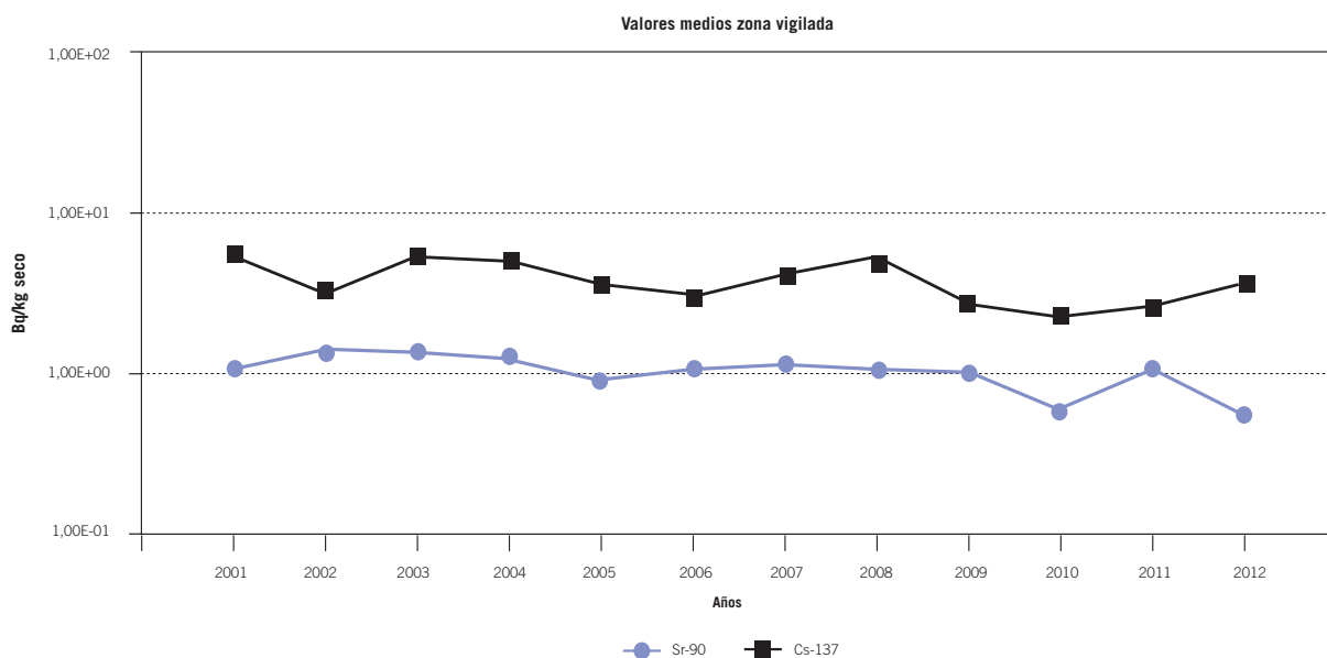
Figura 4.2.6.4.6. Muestras de suelo. Evolución temporal de Sr-90 y CS-137. Central nuclear de Cofrentes
