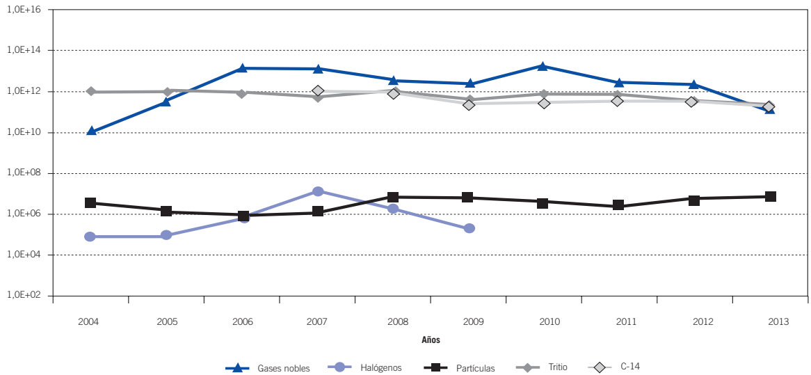
Figura 4.2.6.3.5. Central nuclear Ascó II. Actividad de efluentes radiactivos gaseosos (Bq)
