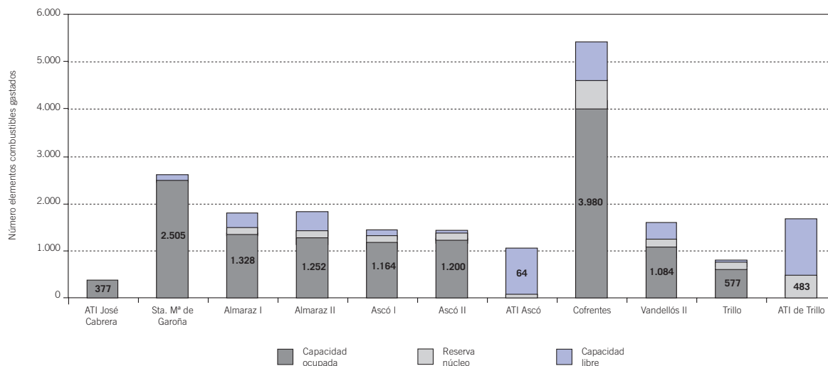
Figura 6.1.1.1. Situación de las instalaciones de almacenamiento de combustible irradiado en las centrales nucleares españolas a finales del año 2013
