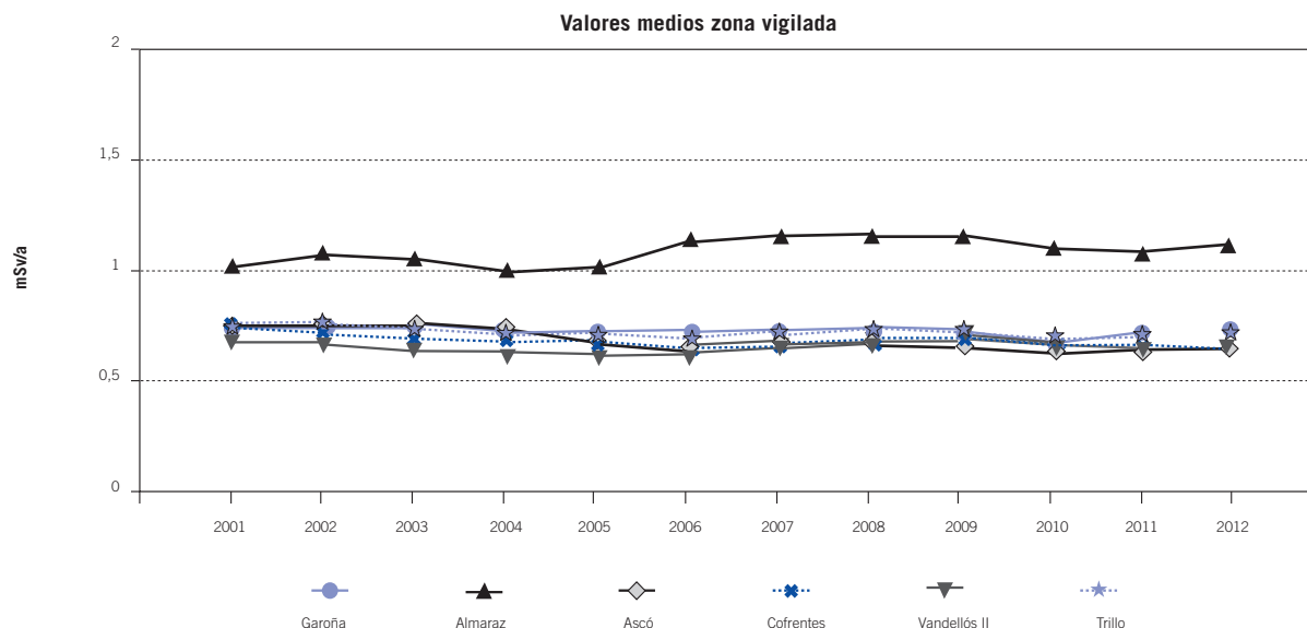
Figura 5.2.2.1.11. Radiación directa. Dosis integrada. Valores de los DTL
