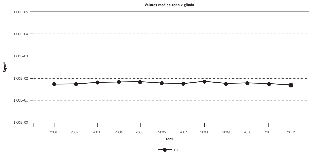
Figura 4.2.6.3.9. Muestras de agua potable. Evolución temporal de actividad beta total. Central nuclear de Ascó
