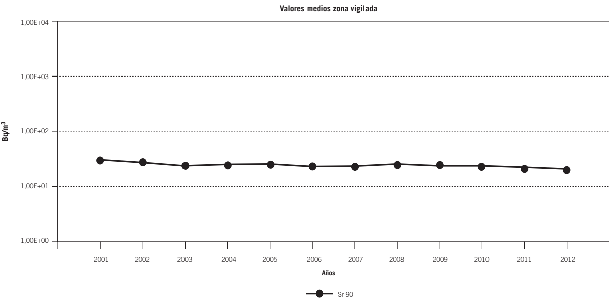
Figura 4.2.6.1.8. Muestras de leche. Evolución temporal de Sr-90. Central nuclear de Santa María de Garoña
