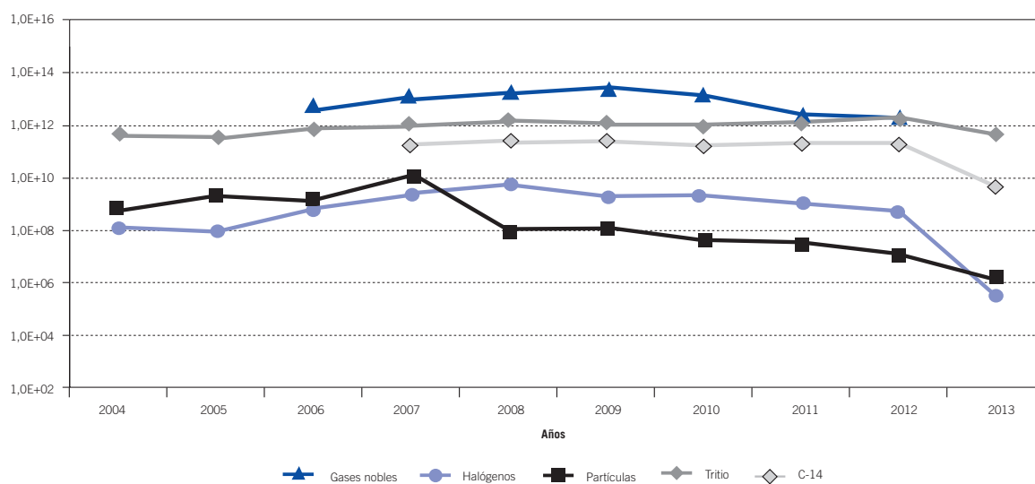
Figura 4.2.6.1.3. Central nuclear de Santa María de Garoña. Actividad de efluentes radiactivos gaseosos (Bq)
