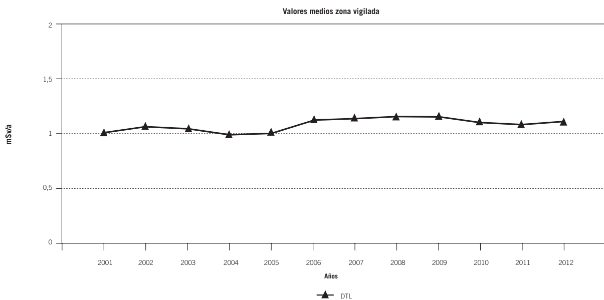
Figura 4.2.6.2.9. Radiación directa. Dosis integrada. Valores de los DTL. Central nuclear de Almaraz
