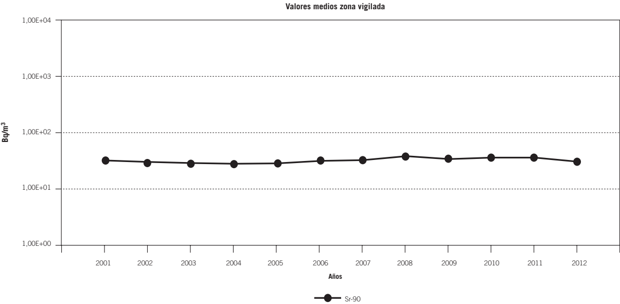
Figura 4.2.6.4.8. Muestras de leche. Evolución temporal de Sr-90. Central nuclear de Cofrentes
