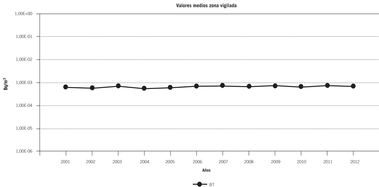
Figura 4.2.6.5.5. Aire. Evolución temporal del índice de actividad beta total. Central nuclear Vandellós II
