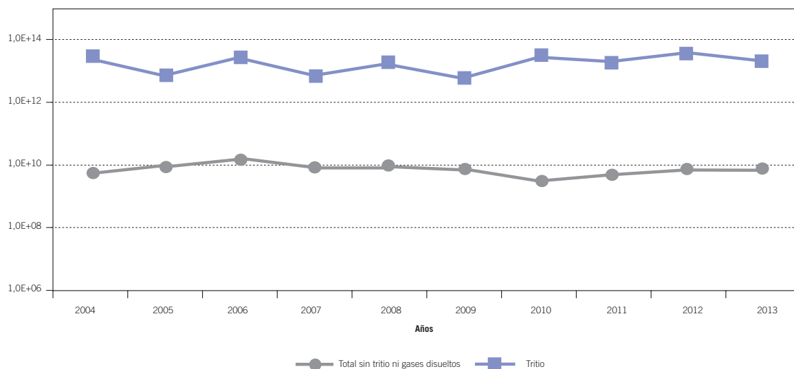
Figura 4.2.6.5.2. Central nuclear Vandellós II. Actividad de efluentes radiactivos líquidos (Bq)
