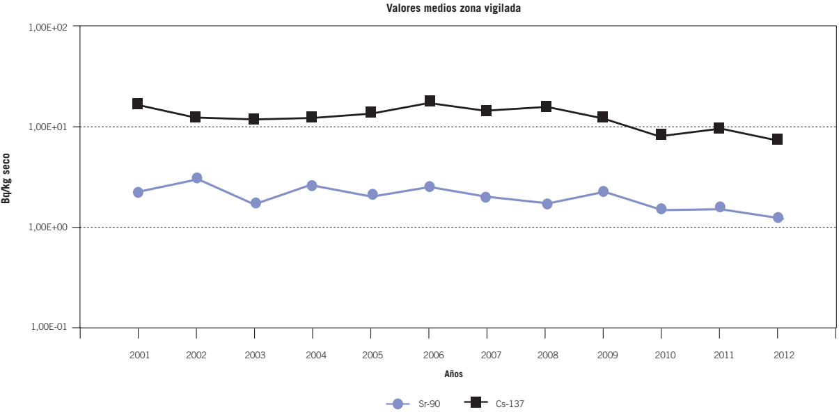
Figura 4.2.6.3.8. Muestras de suelo. Evolución temporal de Sr-90 y CS-137. Central nuclear de Ascó
