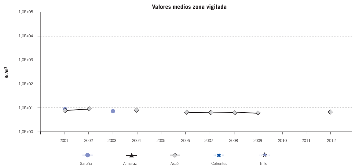
Figura 5.2.2.1.7. Muestras agua potable. Evolución temporal del Sr-90
