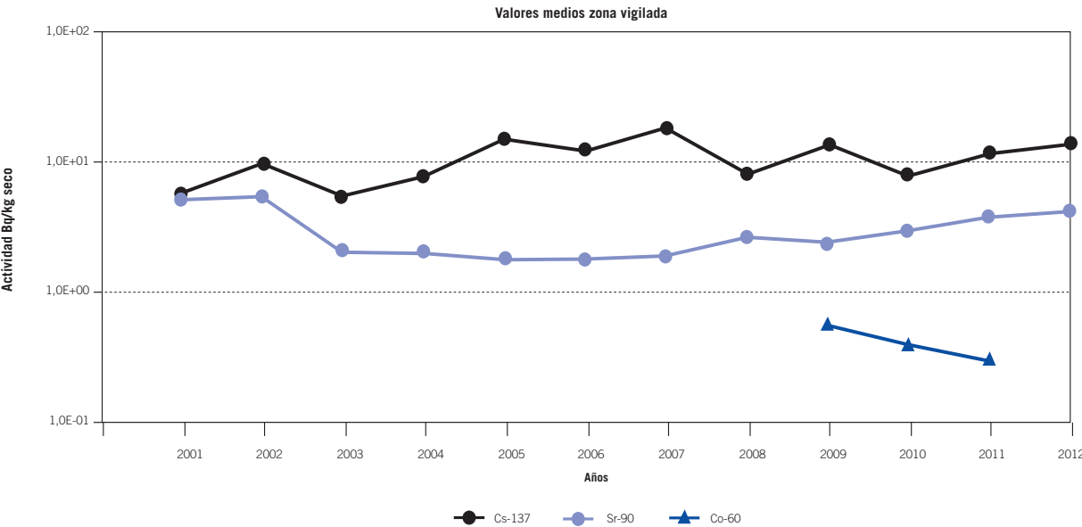
Figura 4.4.2.4. Resultados históricos de la vigilancia radiológica ambiental en el suelo en la central nuclear José Cabrera. Año 2012
