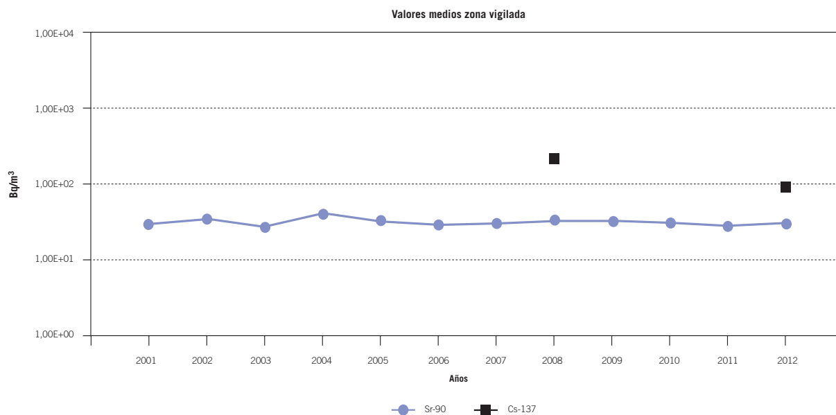
Figura 4.2.6.5.7. Muestras de leche. Evolución temporal de Sr-90 y Cs-137. Central nuclear Vandellós II
