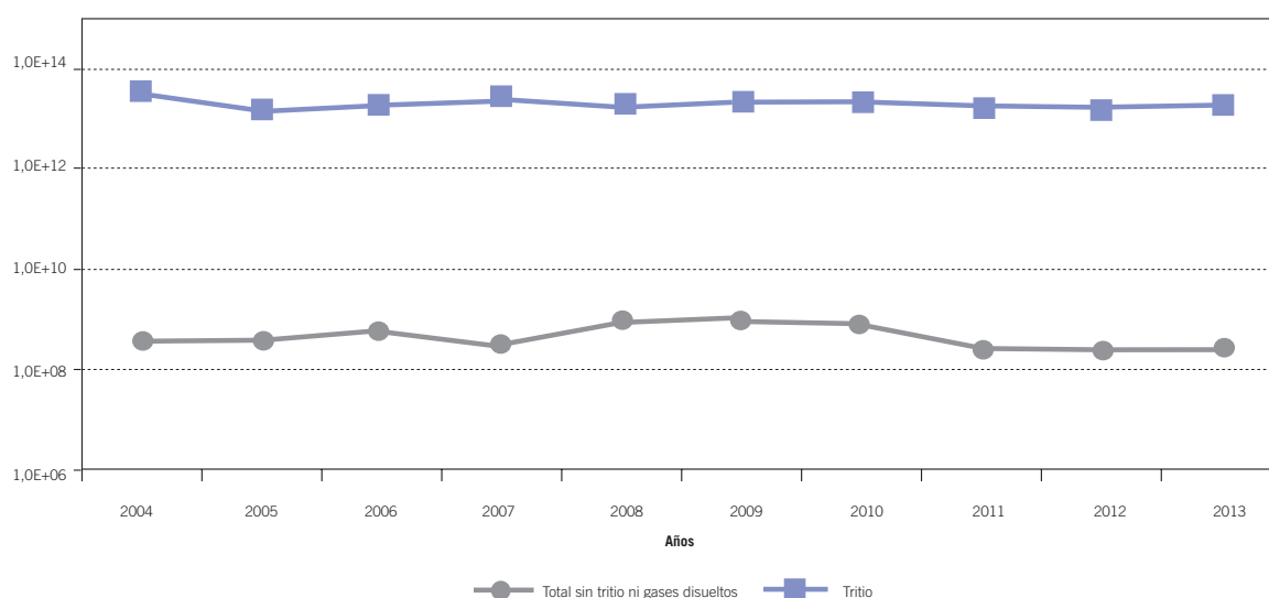
Figura 4.2.6.6.2. Central nuclear de Trillo. Actividad de efluentes radiactivos líquidos (Bq)
