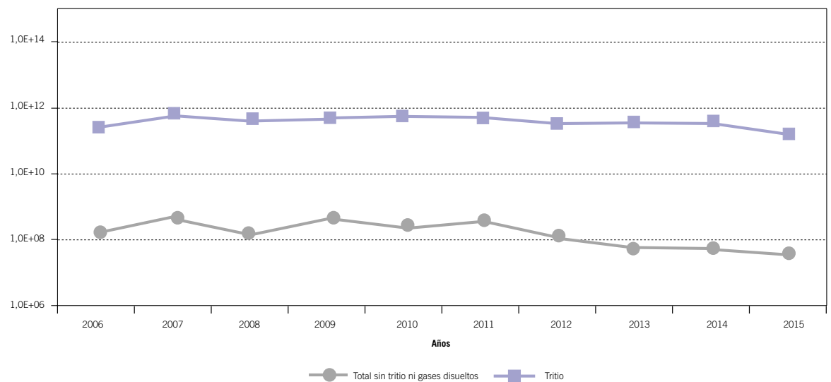
Figura 4.2.7.1.2. Central nuclear Santa María de Garoña. Actividad de efluentes radiactivos líquidos (Bq)
