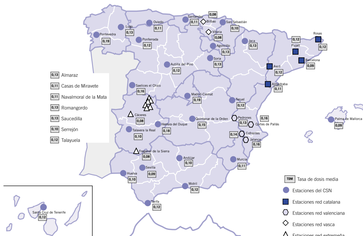
Figura 3.2.2.5. REA. Valores medios de tasa de dosis gamma. Año 2015 (microSievert/hora)
