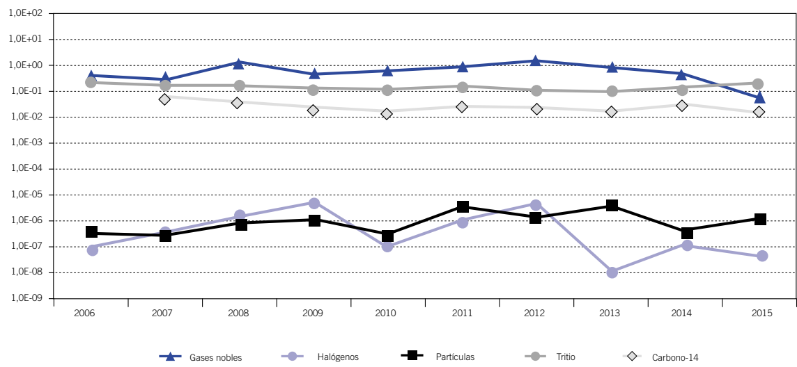
Figura 3.2.2.2. Efluentes radiactivos gaseosos de centrales PWR. Actividad normalizada (GBq/GWh)
