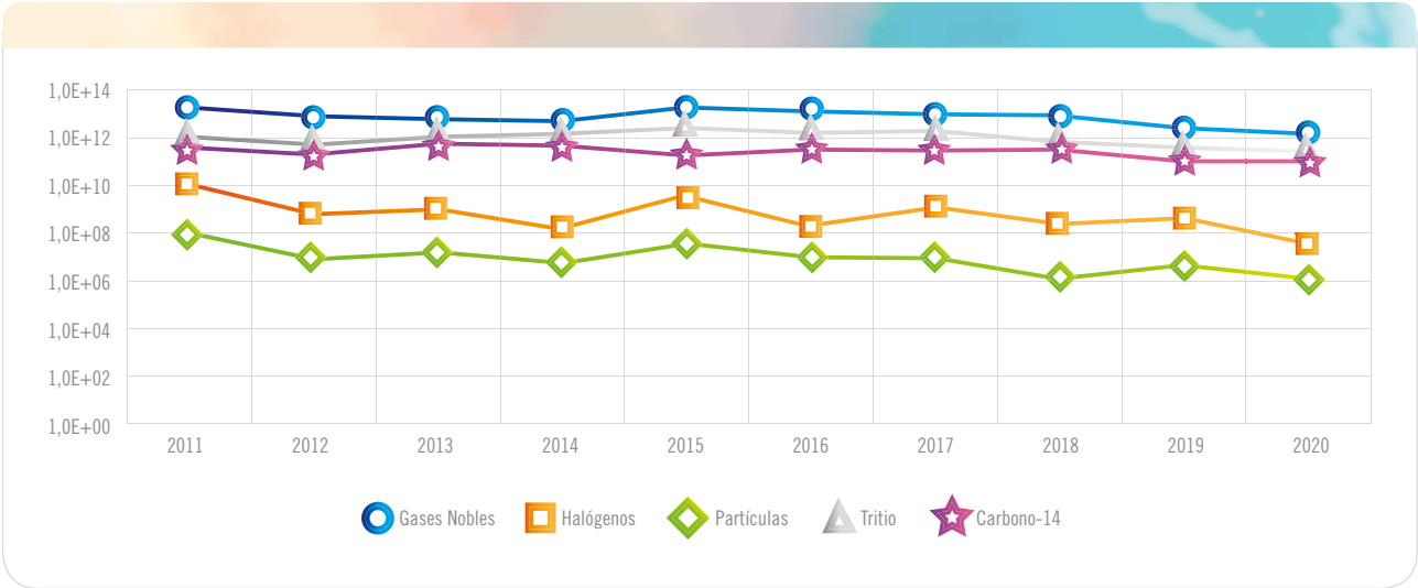
Gráfica 4.1.4.4.3. CN Cofrentes. Actividad de efluentes radiactivos gaseosos (Bq)
