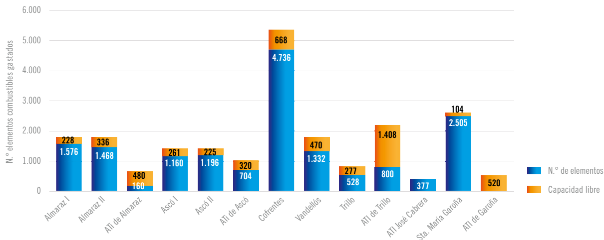
Gráfica 6.1.1.2. Inventario de metal pesado en las instalaciones de almacenamiento de combustible gastado en las centrales nucleares españolas a 31-12-2020 (en toneladas de uranio)
