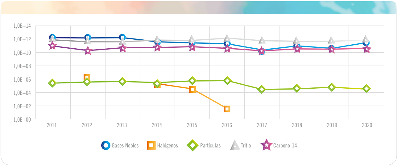
Gráfica 4.1.4.2.3. CN Almaraz. Actividad de los efluentes radiactivos gaseosos (Bq)
