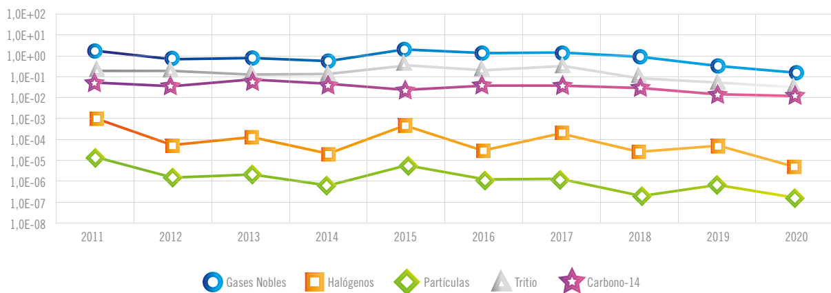
Gráfica 3.2.2.5. Efluentes radiactivos gaseosos de centrales BWR
