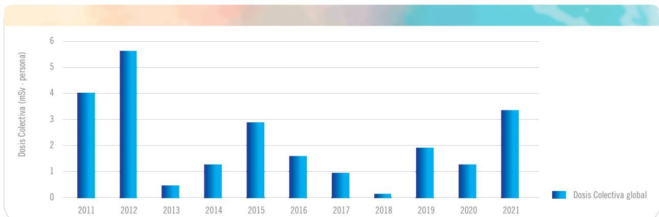
Gráfica 4.3.4.1. Evolución de la dosis colectiva en las instalaciones del Ciemat
