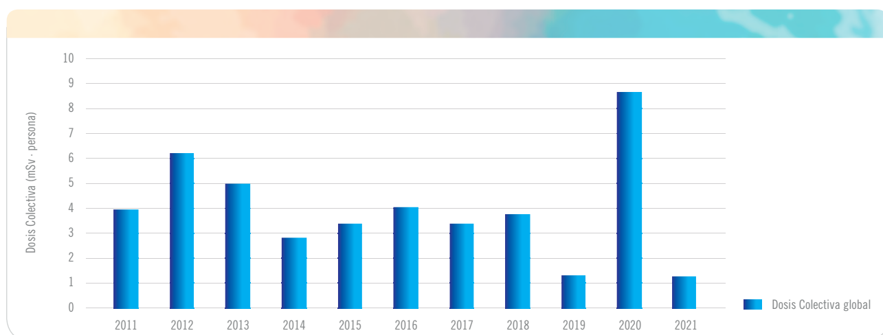
Gráfica 4.3.3.1. Evolución temporal de la dosis colectiva para el personal del Centro de Almacenamiento de Residuos Radiactivos de El Cabril
