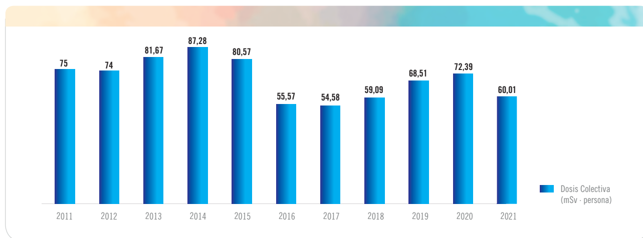
Gráfica 4.3.1.1. Evolución de la dosis colectiva en la fábrica de elementos combustibles de Juzbado desde al año 2011
