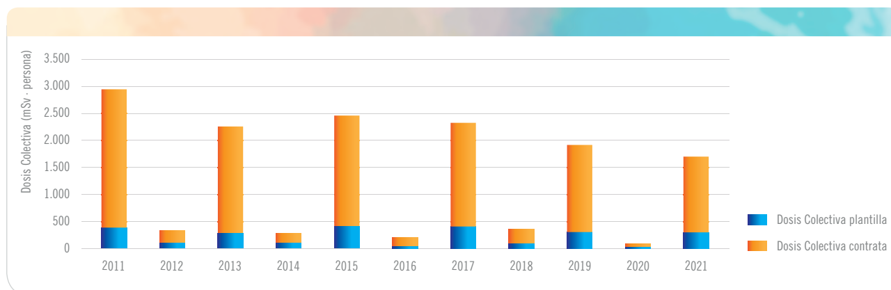
Gráfica 4.1.4.4.1. Evolución de la dosis colectiva en la central nuclear de Cofrentes desde el año 2011
