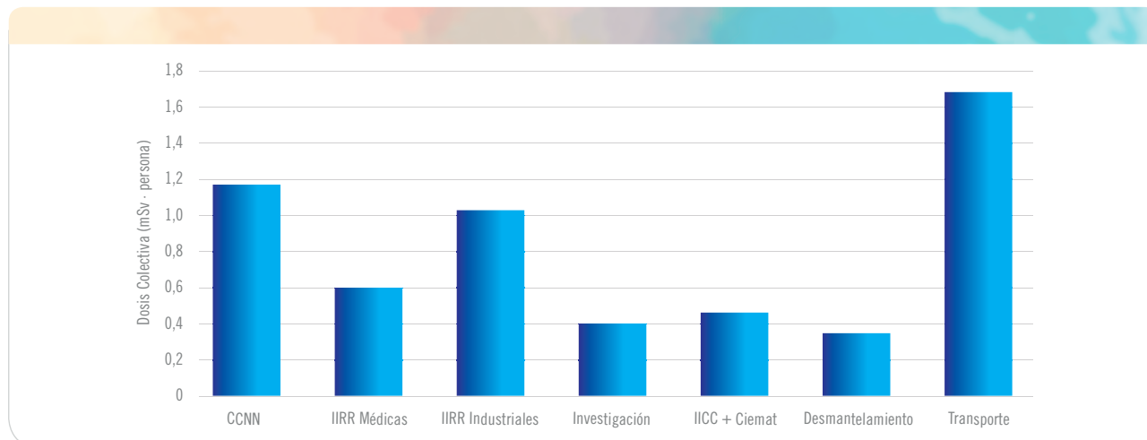
Gráfica 5.1.2.2. Dosis individual media por sectores. Año 2021
