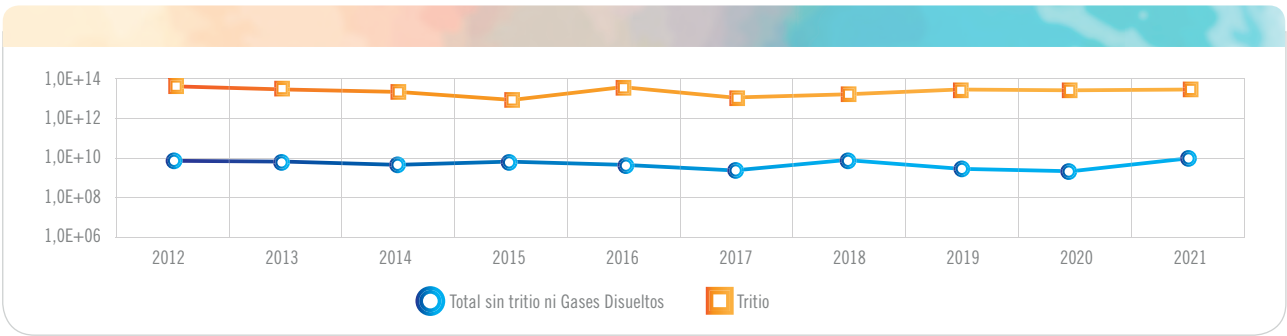
Gráfica 4.1.4.5.3. CN Vandellós II. Actividad de los efluentes radiactivos gaseosos (Bq)
