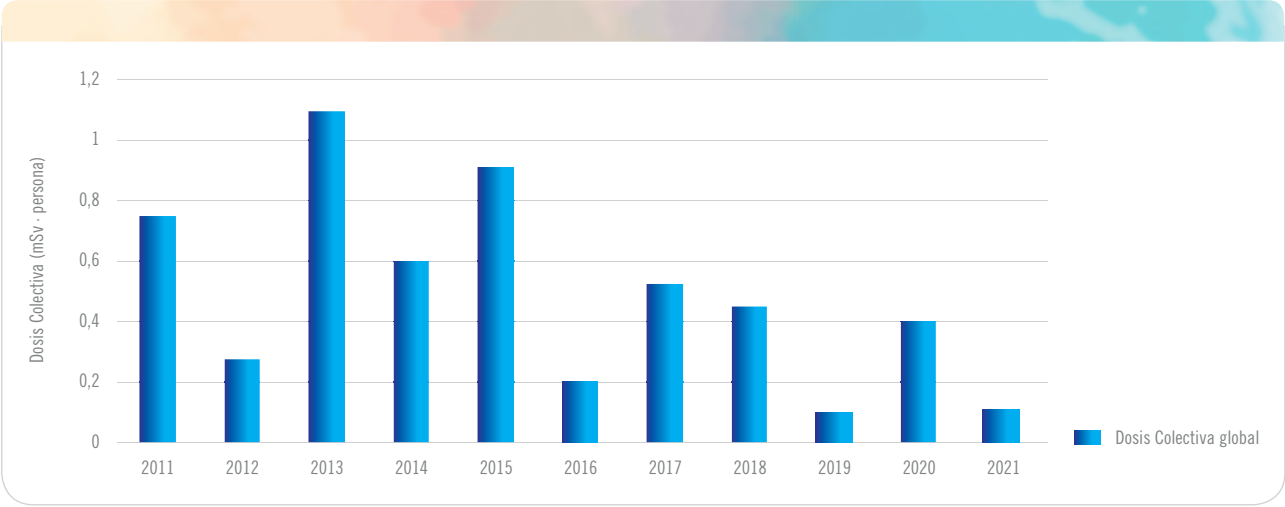
Gráfica 4.3.5.1.1. Evolución de la dosis colectiva en la planta Quercus de fabricación de concentrados de uranio
