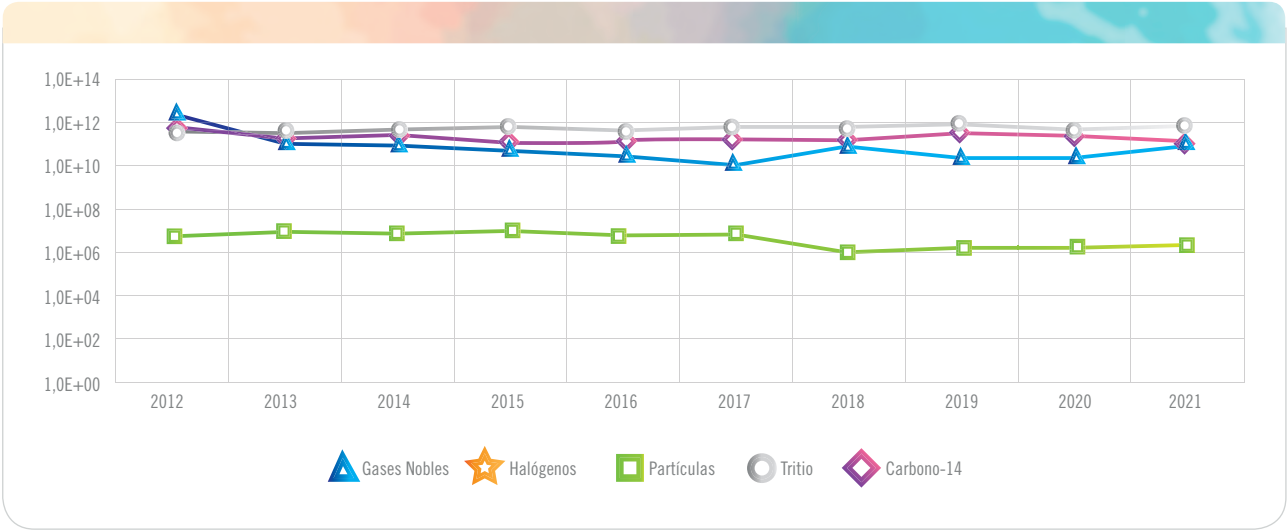
Gráfica 4.1.4.3.5. CN Ascó II. Actividad de efluentes radiactivos gaseosos (Bq)
