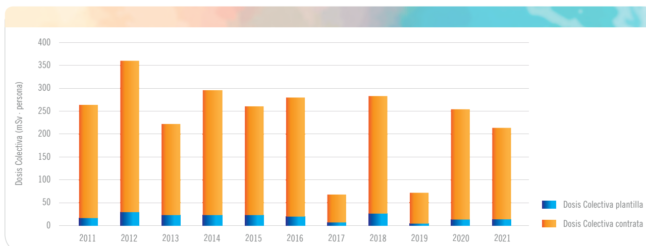
Gráfica 4.1.4.6.1. Evolución de la dosis colectiva en la central nuclear de Trillo desde el año 2011
