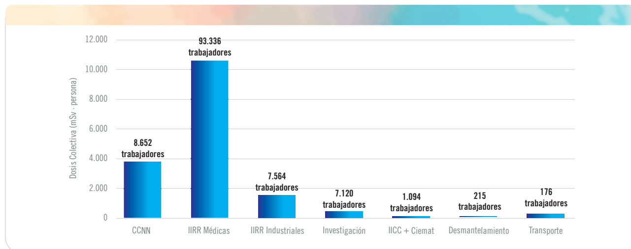
Gráfica 5.1.2.1. Dosis colectiva y nº de trabajadores expuestos por sectores. Año 2021
