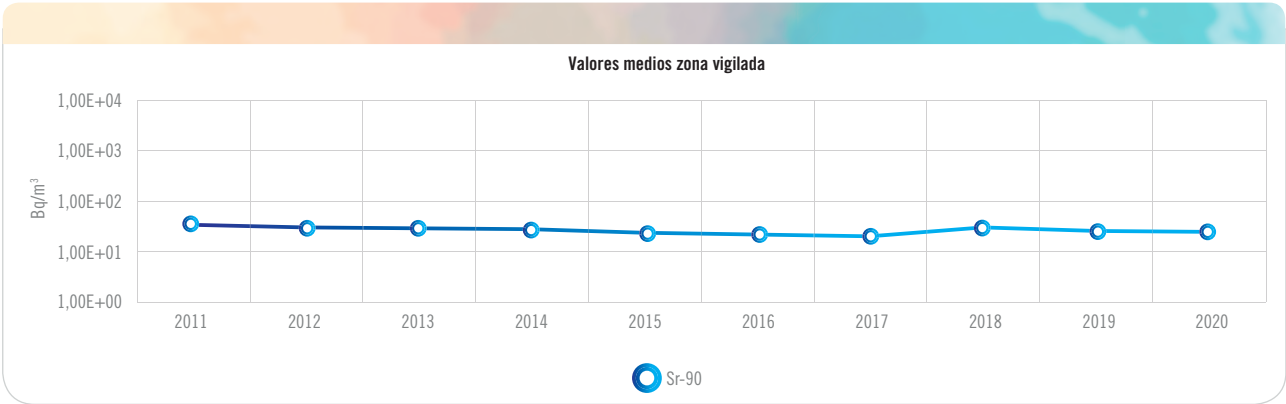
Gráfica 4.1.4.4.8. Leche. Evolución temporal de Sr-90. Central nuclear Cofrentes
