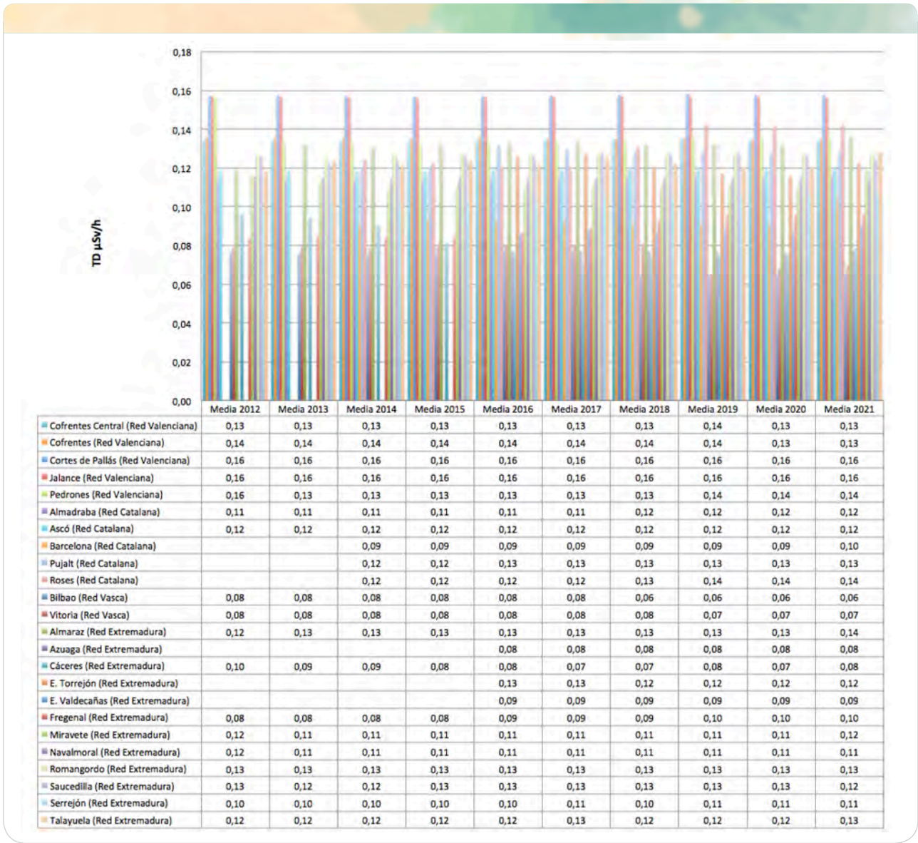
Gráfica 3.2.3.1. Valores medios anuales de tasa de dosis gamma (µSv/hora). Año 2021. REA de las CCAA
