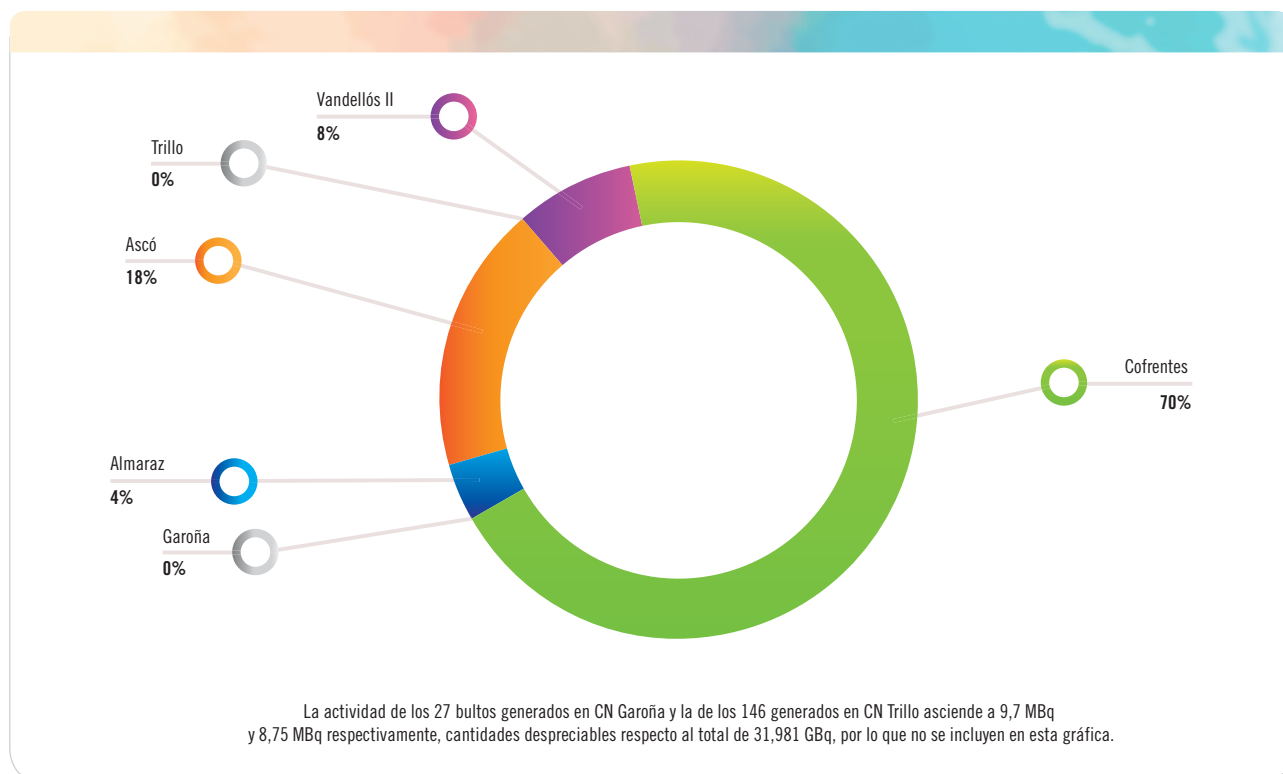
Gráfica 6.2.1.2. Distribución de la actividad (31,981 GBq) contenida en los bultos de residuos radiactivos (RBMA y RBBA) generados en 2021 en las centrales nucleares en explotación y en cese definitivo
