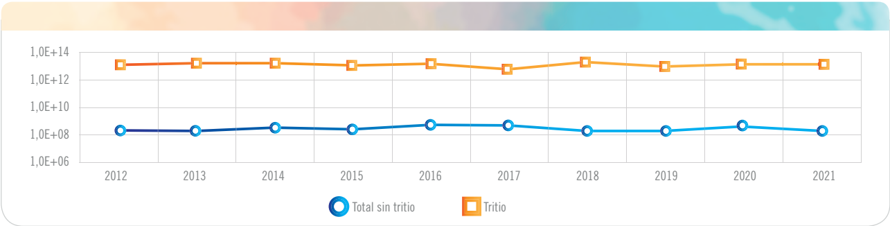
Gráfica 4.1.4.6.3. CN Trillo. Actividad de efluentes radiactivos gaseosos (Bq)
