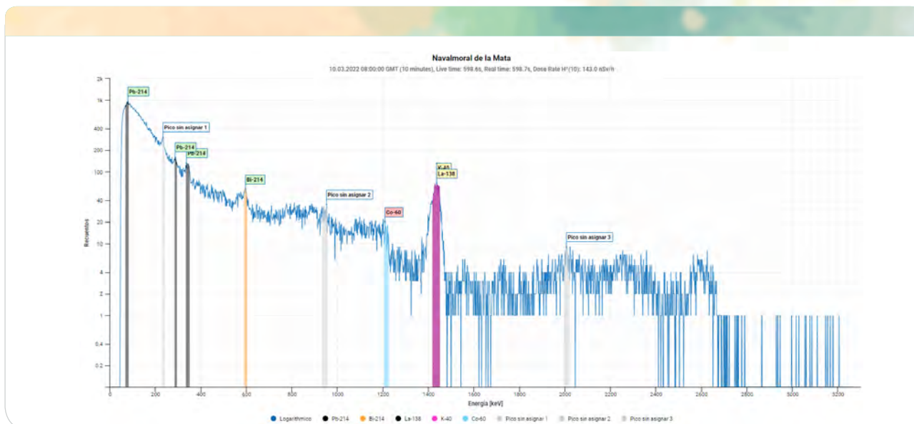
Figura 6. Espectro gamma de una medida realizada en una estación
