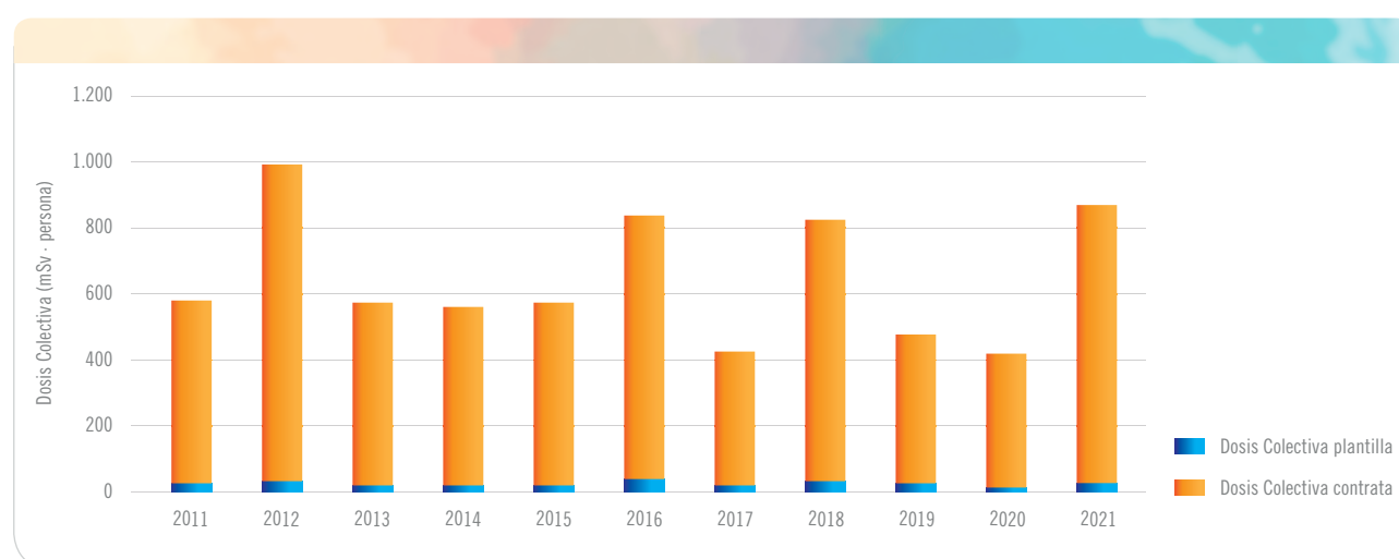
Gráfica 4.1.4.2.1. Evolución de la dosis colectiva en la central nuclear de Almaraz desde al año 2011
