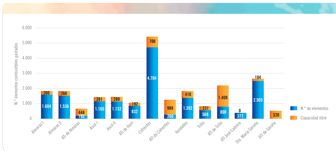
Gráfica 6.1.1. Inventario de las instalaciones de almacenamiento de combustible gastado en las centrales nucleares españolas a 31-12-2021 (en número de elementos combustibles)
