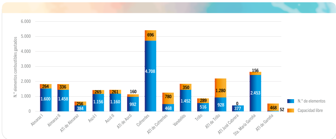
Gráfica 6.1.1.1. Inventario de las instalaciones de almacenamiento de combustible gastado en las centrales nucleares españolas a 31-12-2023 (en número de elementos combustibles)
