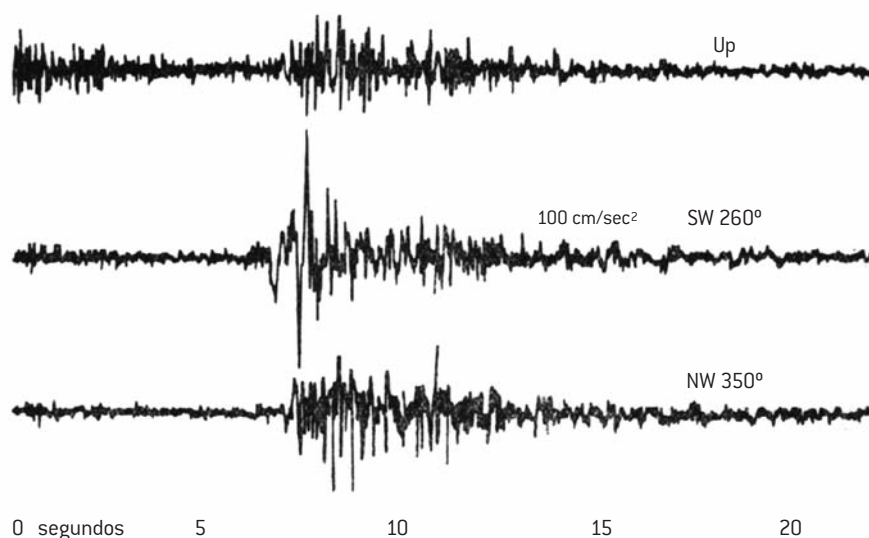
Figura 5. Acelerograma registrado en Santiago de Chile el 13 de septiembre de 1945.
