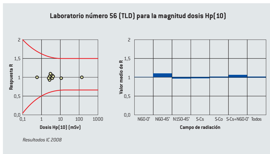
Figura 1. Resultados obtenidos por el CND en la intercomparación EURADOS 2008 (EURADOS Report 2012-01)
