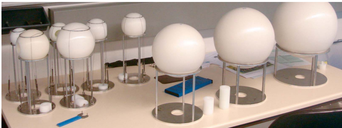
Sistema de esferas de Bonner para la caracterización del espectro neutrónico.
