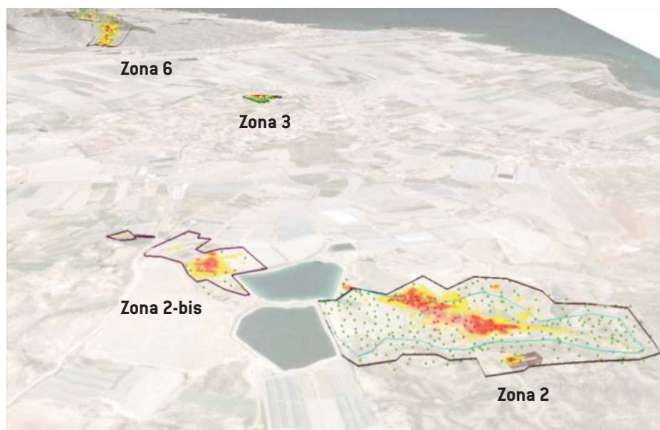
Este mapa de la zona de Palomares muestra las áreas con valores que superan los criterios de restricción de uso parcial (amarillo) y total (rojo) establecidos por el CSN.
