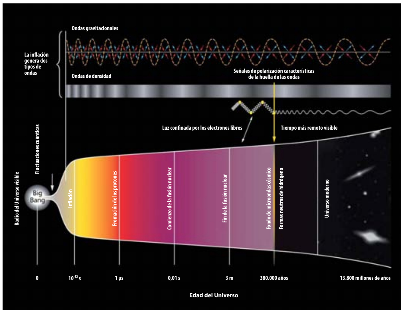
Esquema de la evolución del Universo.
