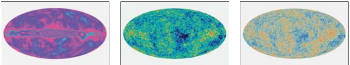
De izquierda a derecha, resolución de los telescopios Cobe, WMAP y Planck.
