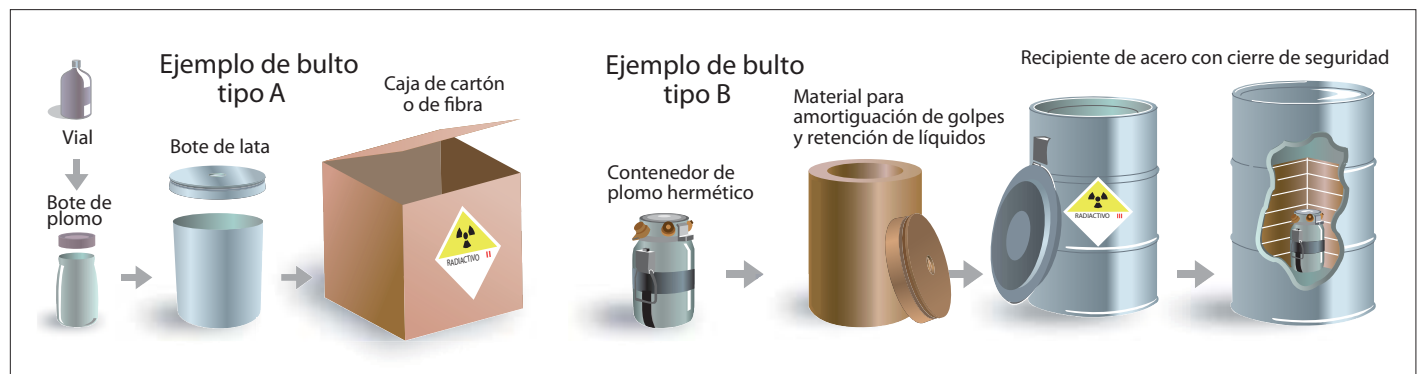
Características de los diferentes tipos de embalaje para la gestión de las fuentes radiactivas.
