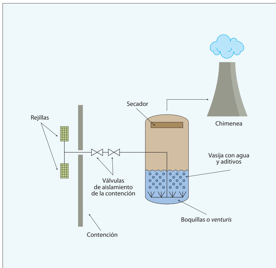
Figura 1. Sistema de venteo filtrado de la contención húmedo.
