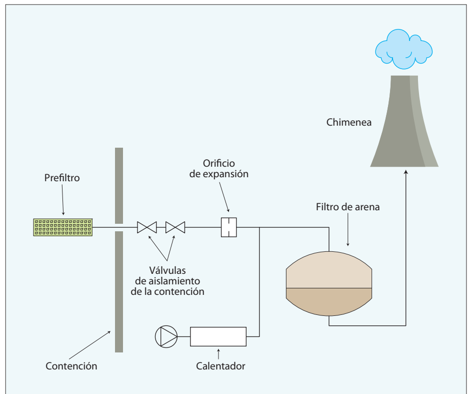
Figura 3. Sistema de venteo filtrado de la contención seco de lecho de arena.
