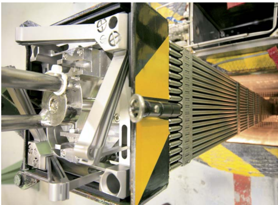
Elemento combustible en la factoría de Enusa.
