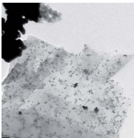
Imagen nanométrica de una superficie de grafito con nanopartículas de oro.
