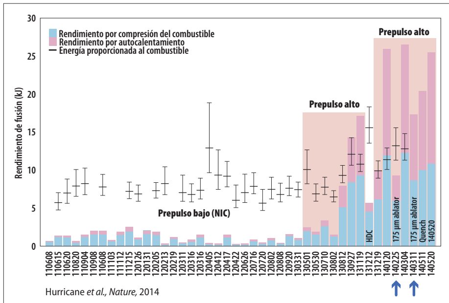
Figura 3. Resultados (rendimiento por fusión en cápsula de DT en kJ) obtenidos por los diferentes experimentos realizados en NIF.
