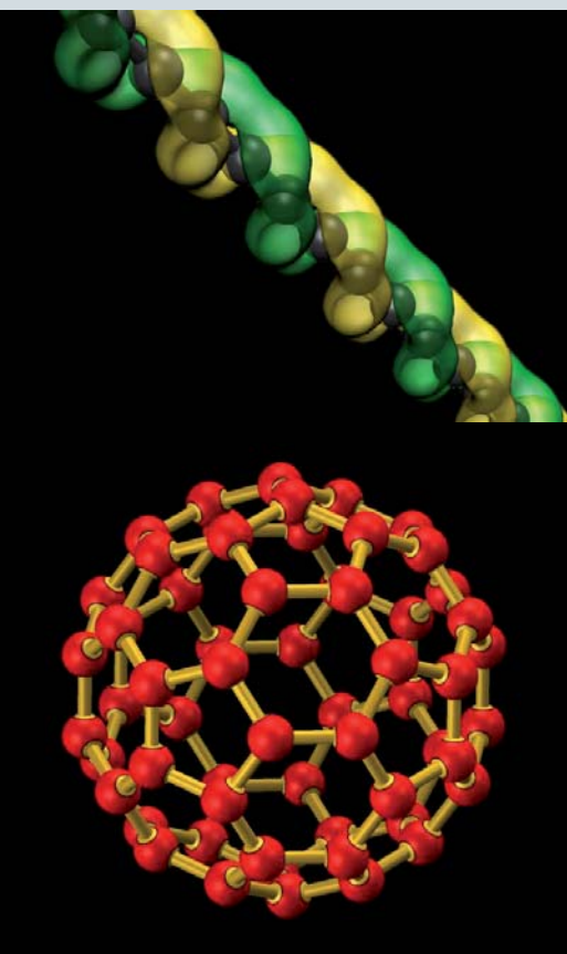
Carbino (arriba) y fullereno.
