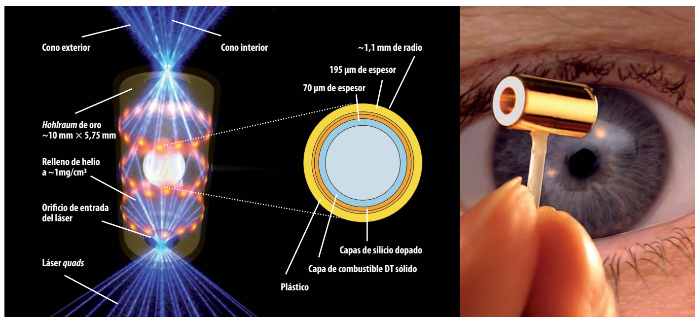
Figura 2. Entrada de la radiación láser e impacto sobre la esfera de combustible y corte de dicha esfera.
