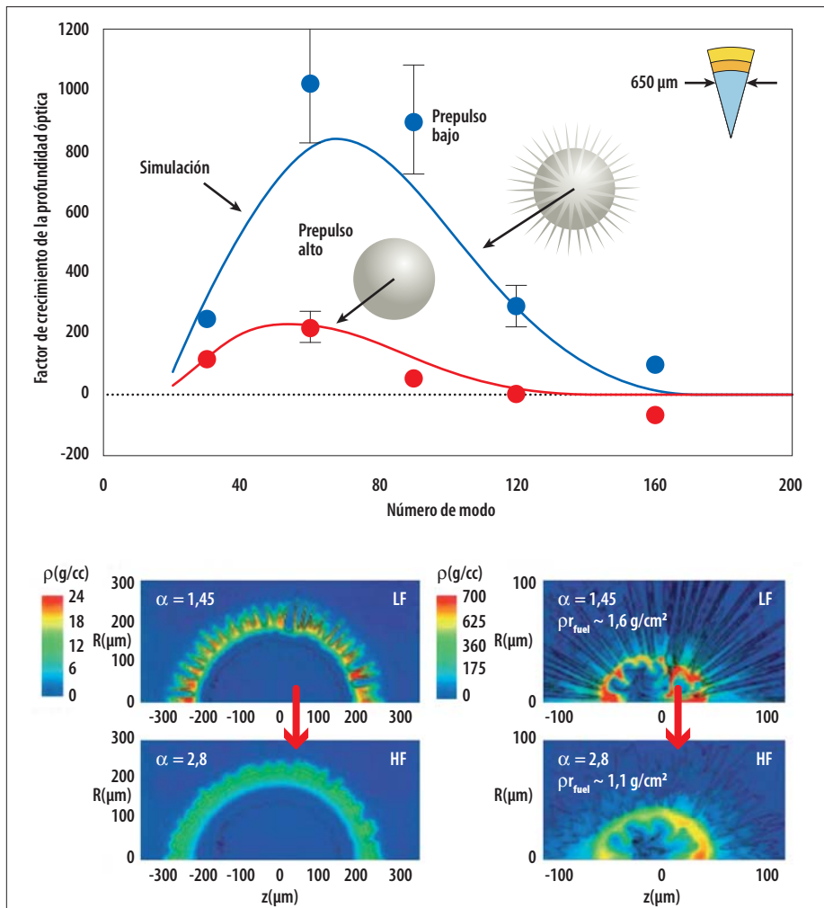
Figura 4.- Factor de crecimiento de inestabilidades para prepulso bajo (LF) y alto (HF), (arriba); y evolución del frente de ablación (abajo) durante implosión (izda.) y en máxima compresión (dcha.).
