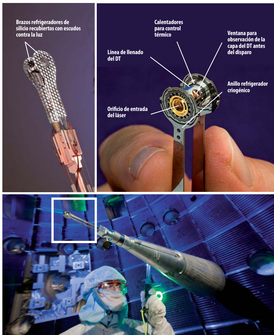
Figura 1. Detalle del cilindro o hohlraum donde va alojada la esfera de combustible.
