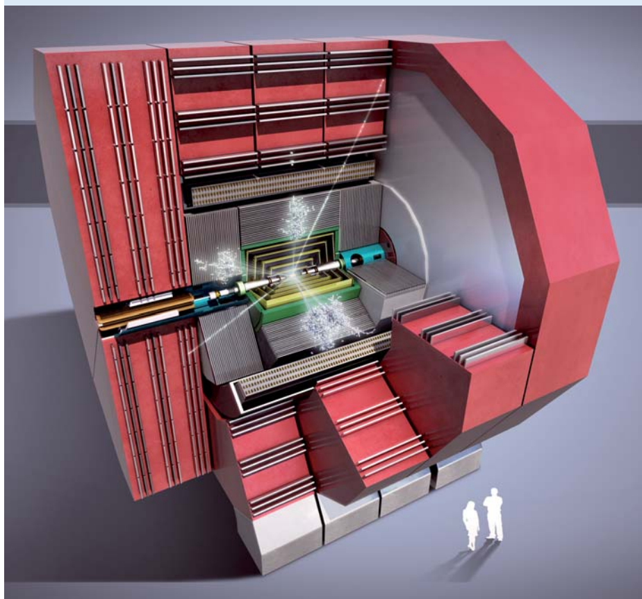
Simulación de una colisión de partículas en el futuro acelerador lineal CLIC.
