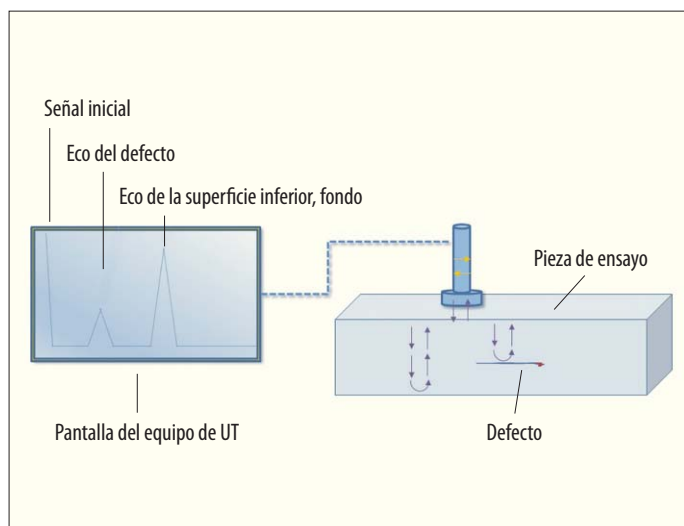
Figura 4. Esquema de un examen por ultrasonidos.
