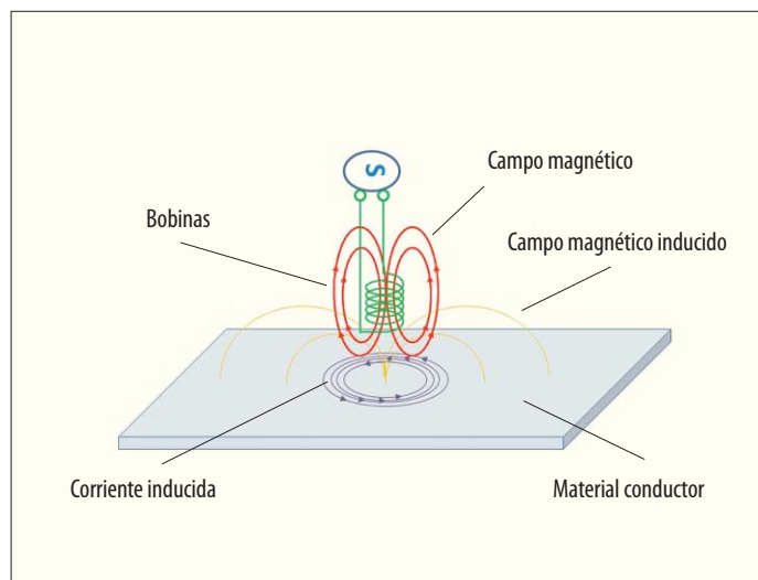
Figura 3. Corrientes inducidas.
