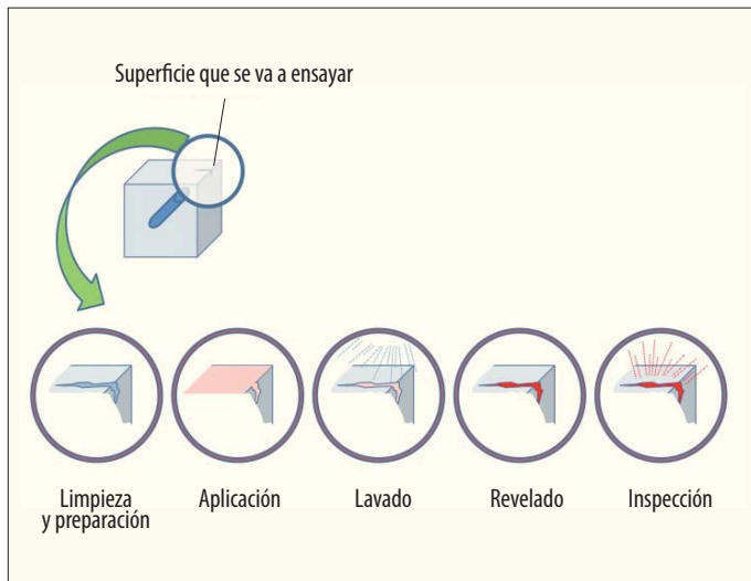
Figura 1. Proceso de líquidos penetrantes.
