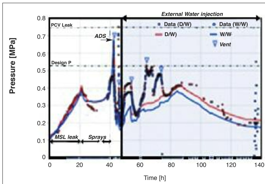
Figura 8. Evolución de la presión en la contención de la unidad 3.
