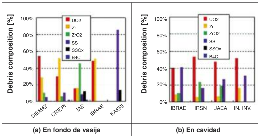
Figura 2. Localización y composición del corio en la Unidad 2.
