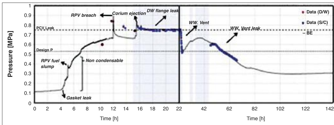
Figura 7. Evolución de la presión en la contención de la unidad 1.
