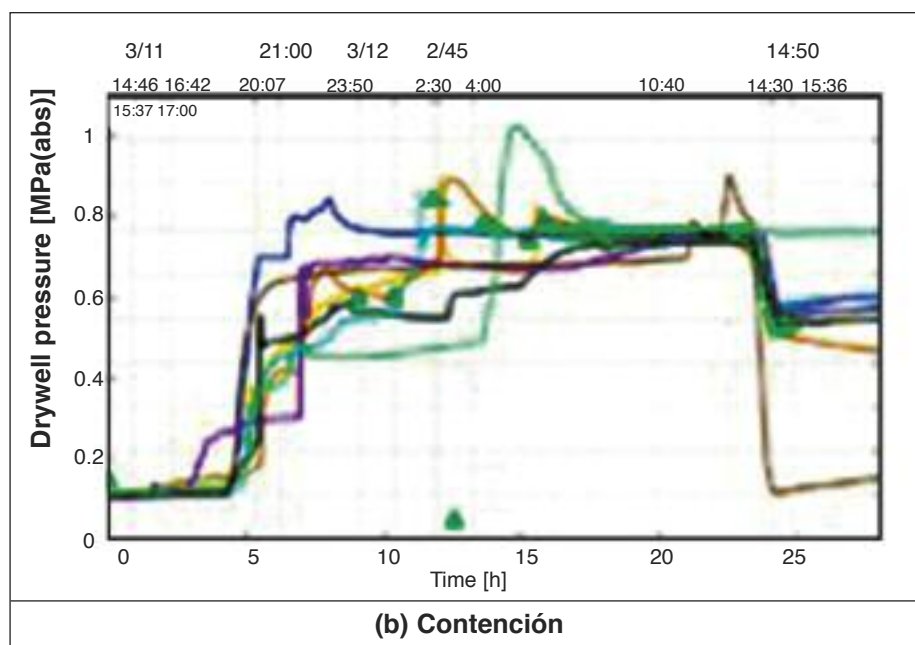
Figura 5. Evolución de la presión en la unidad 1.
