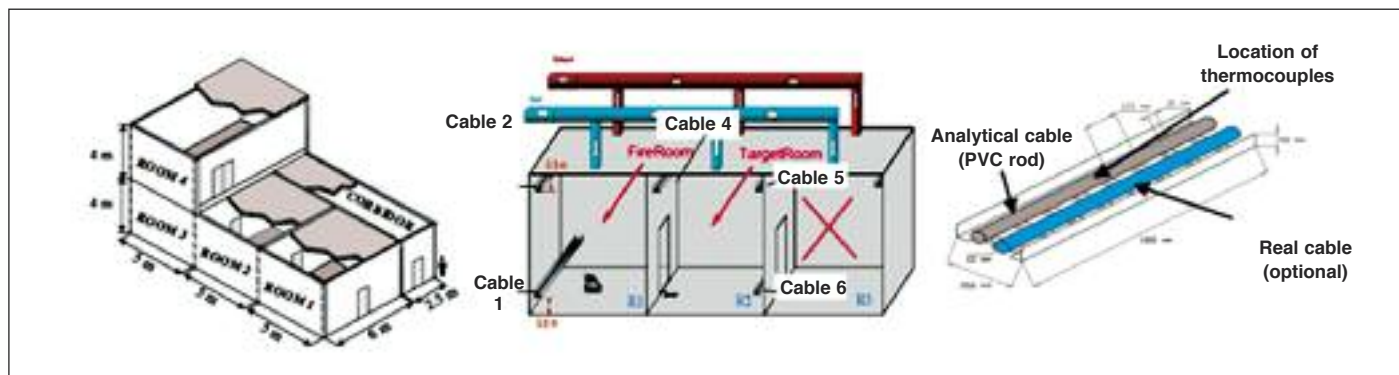
Figura 5.: Instalación DIVA (izda.). Escenario del ejercicio PRS_DI_D3 (centro). Bandejas de cables (dcha.)
