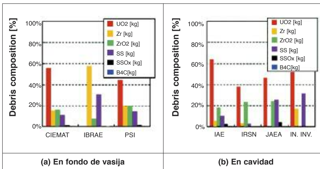
Figura 3. Localización y composición del corio en Unidad 3.
