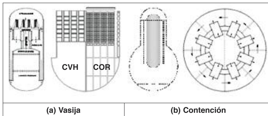
Figura 6. Modelo MELCOR 2.1 para las unidades 1-3 de Fukushima.
