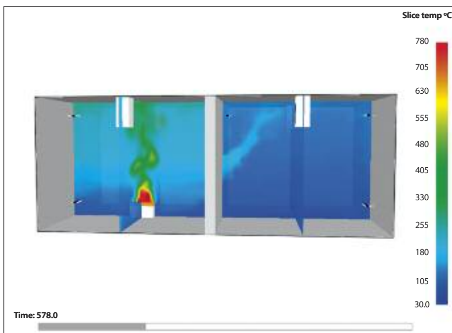
Figura 7. Simulación del escenario PRS_DI_D3 del proyecto PRISME con FDS.
