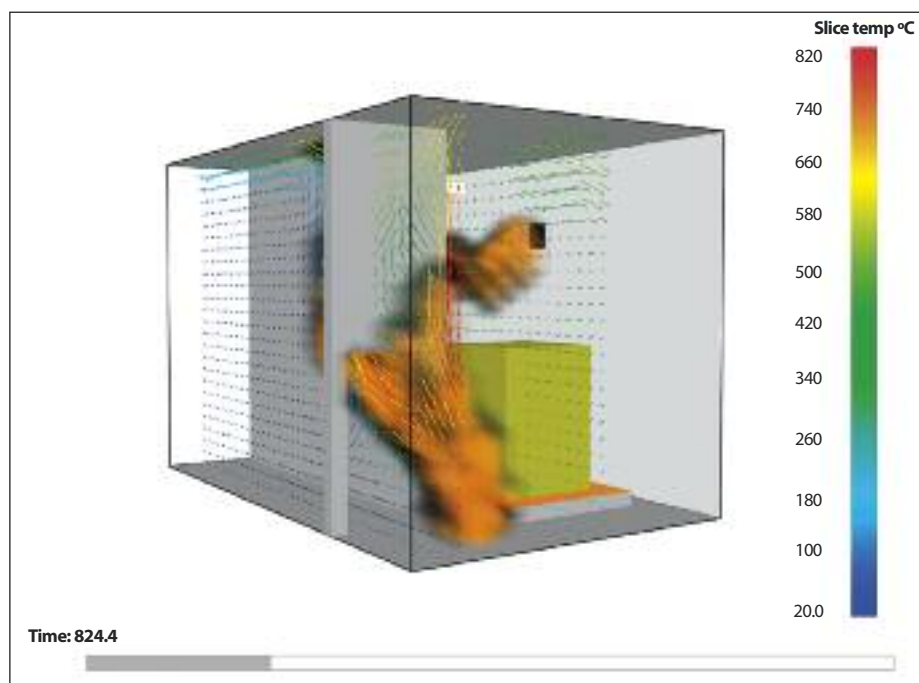
Figura 2. Escenario del incendio del aceite de lubricación en la sala de una bomba con FDS.
