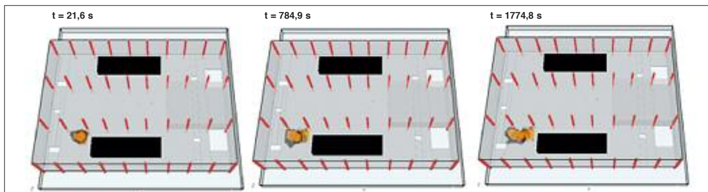
Figura 4. Evolución del incendio del aceite de lubricación de una turbina con FDS.
