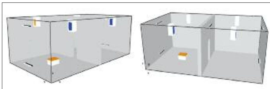
Figura 6. Escenarios simulados del ejercicio PRS_DI_D3 del proyecto PRISME.
