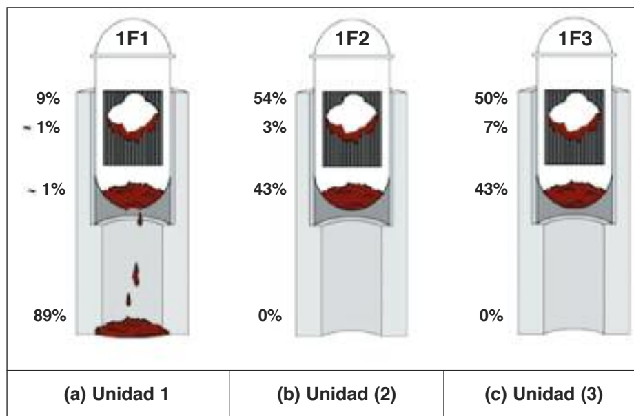
Figura 9. Localización del corio en las unidades según los cálculos de MELCOR 2.1.
