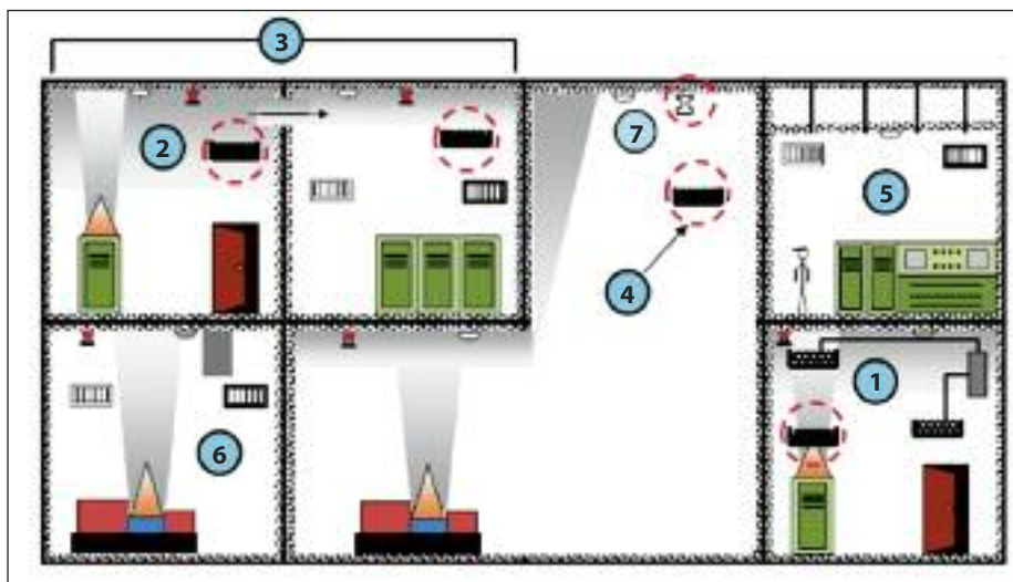
Figura 1. Esquema de escenarios prototipo de incendios en centrales nucleares. Fuente NUREG-1934 de la USNRC.
