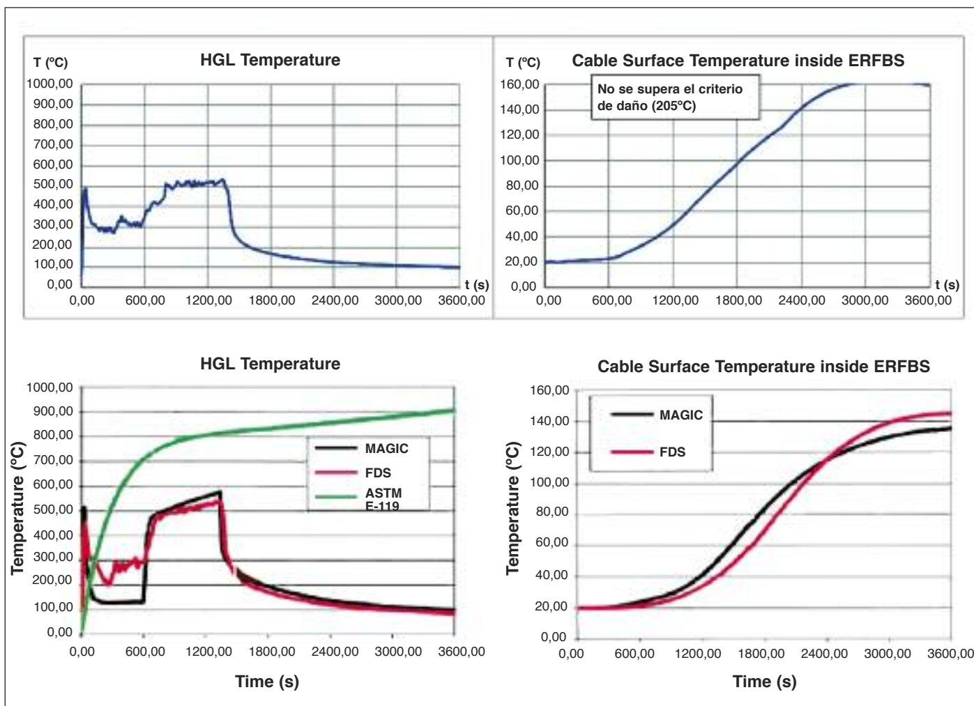
Figura 3. Validación de resultados del incendio del aceite de lubricación en la sala de una bomba con FDS.
