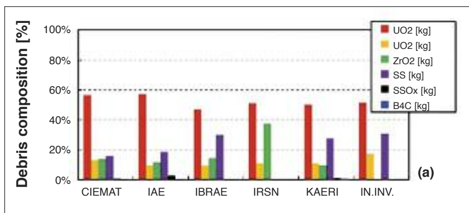
Figura 1. Composición del corio en la cavidad del reactor de la unidad 1.
