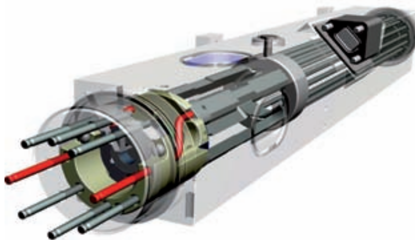
Esquema del Reloj Atómico de Espacio Profundo (DSAC).
