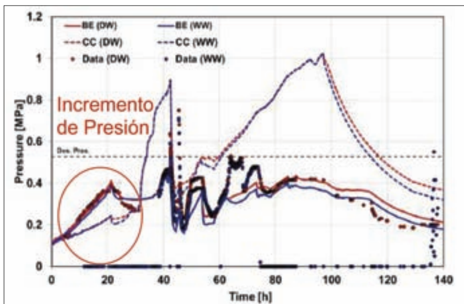
Figura 1. Evolución de presión en contención en Fukushima Dai-Ichi Unidad 3 (Fuente: Cálculo realizado por el Ciemat con el código MELCOR para el proyecto BSAF-1).
