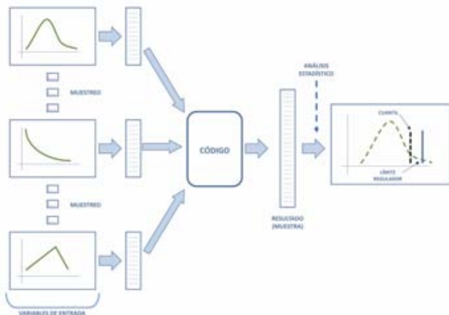
Figura 2: Propagación de incertidumbre en un análisis BEPU.
