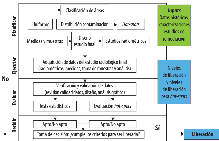
Diagrama de flujo de la metodología de MARSSIM.
