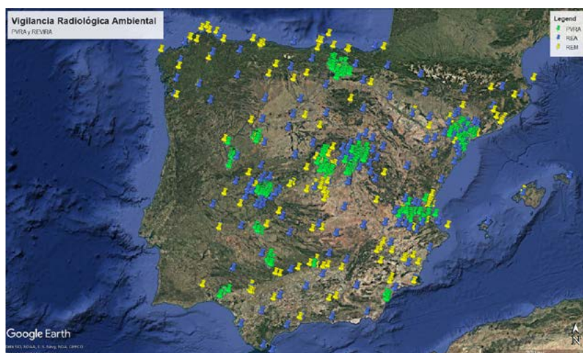
Figura 1. Estaciones de medida y muestreo del sistema de vigilancia radiológica ambiental en España
