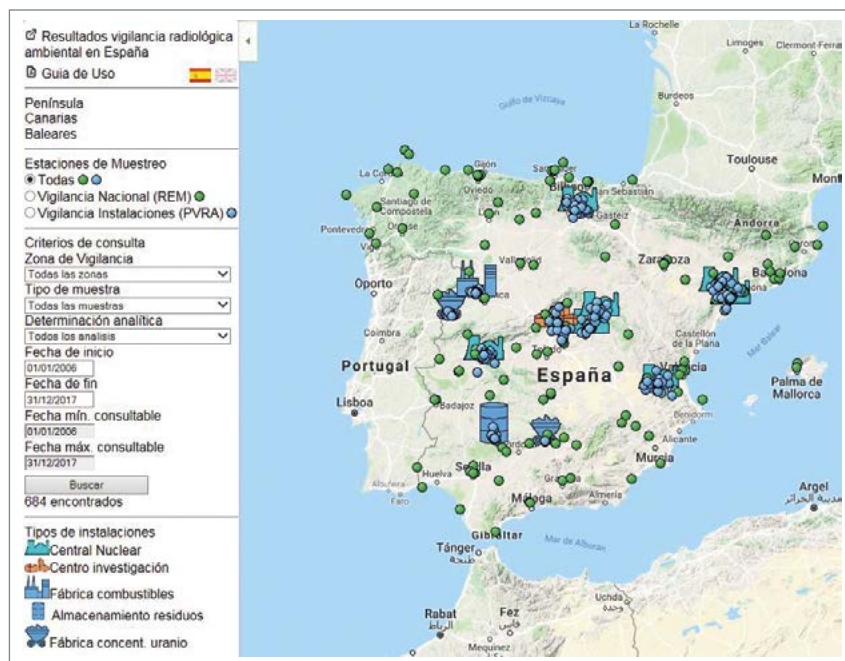
Figura 8. Aplicación KEEPER-WEB
