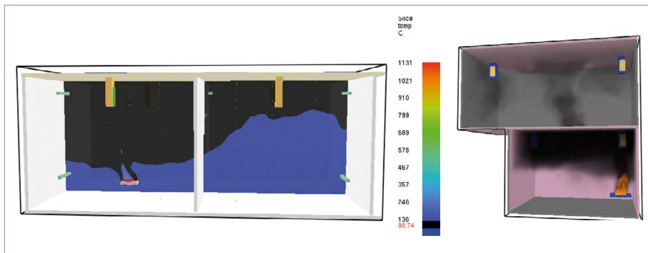
Figura 3. Simulaciones de incendios de validaciones internacionales de PRISME
