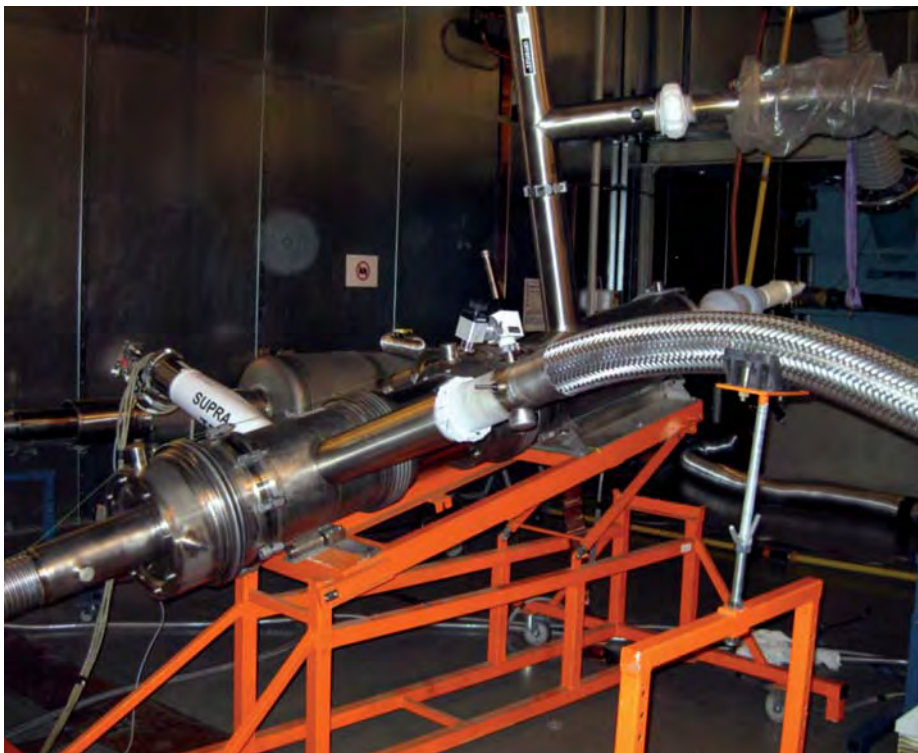
Realización de pruebas para estudiar el comportamiento del cable superconductor.
