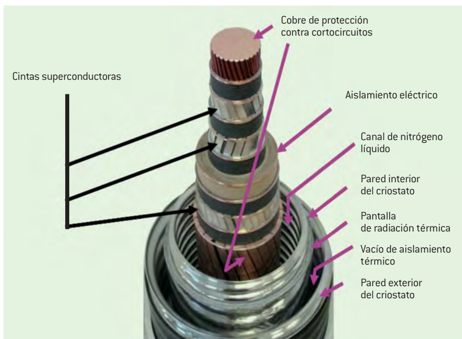
Estructura del cable superconductor del ICMB-CSIC.
