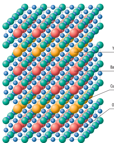
Estructura del compuesto denominado ybaco.
