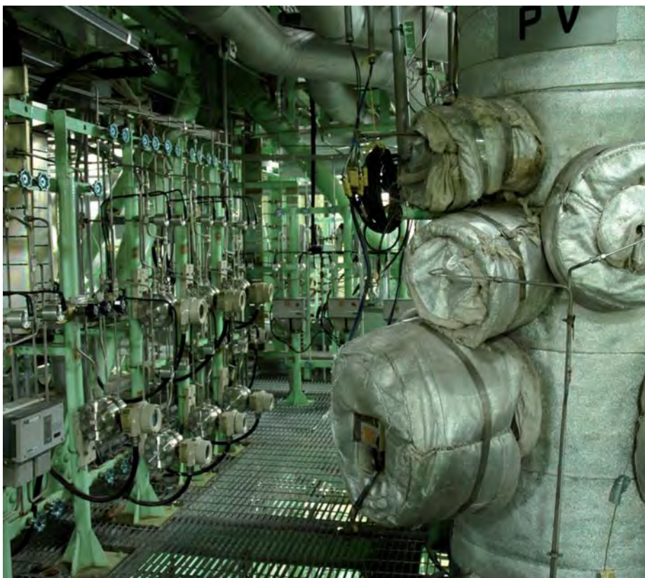
Vista de las instalaciones del proyecto de investigación ROSA, en Japón.
