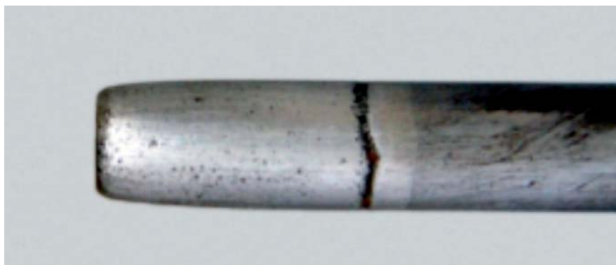
Figura 4. Estado de la varilla y de la zona de soldadura contenida en un equipo de medida de densidad y humedad en suelos.
