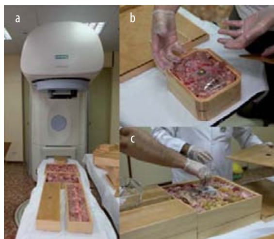
Figura 5. (a) Preparación del maniquí de tejido equivalente en la sala de tratamiento, (b) y (c) detalles de la composición y ubicación del detector en cabeza y abdomen.
