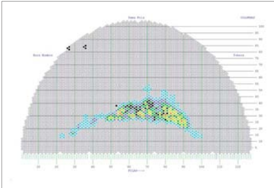
Figura 2. Ejemplo mapa de la distribución del denting en rama fría.
