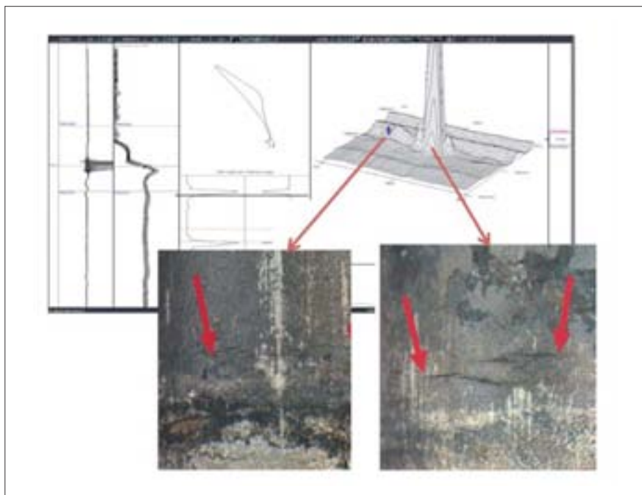
Figura 6. Indicación de grieta en tubo extraído.
