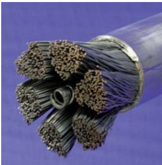
Detalle de los cables superconductores que envuelven el anillo toroidal. El tubo central alberga el helio líquido que enfría los cables.
