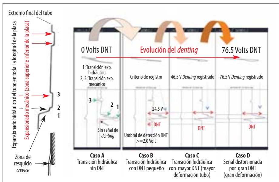
Figura 5. Caracterización y evolución del denting .
