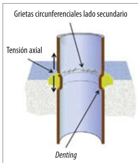
Figura 4. Detalle del posible efecto del denting .
