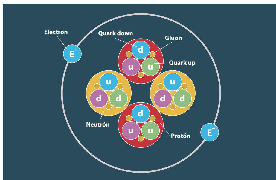
Estructura de un átomo de helio-4.
