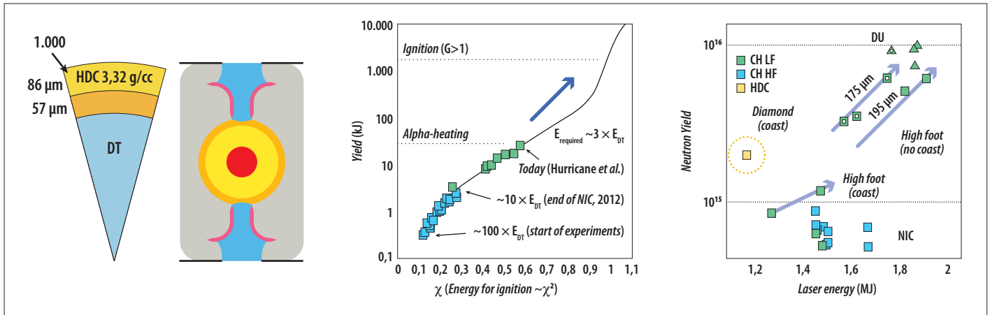
Figura 5. De izquierda a derecha, cápsula propuesta con capa de HDC y hohlraum con cuasivación interno, rendimiento del DT vs. parámetro de ignición ( 1 = \text{ignición} ) y rendimiento del DT vs. energía del láser.
