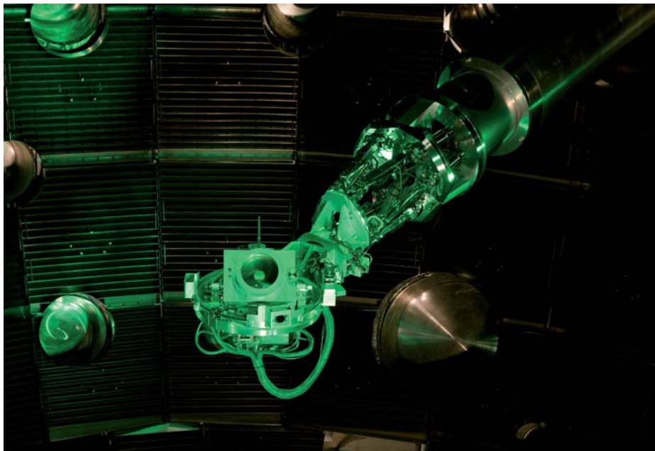
Mecanismo de evaluación por inspección óptica de los experimentos realizados en NIF.
