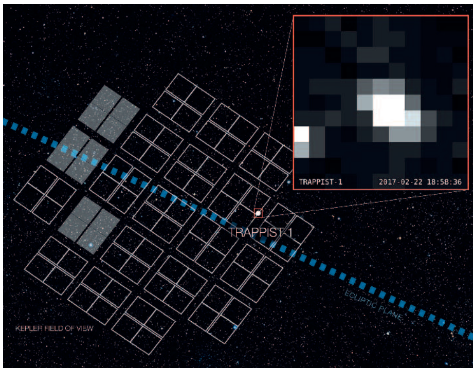
Localización de la estrella enana Trappist-1 en el campo de visión del telescopio espacial de la NASA Kepler y, en el recuadro, la cantidad de luz detectada por cada pixel en una pequeña sección de la cámara del telescopio. La luz captada de Trappist-1 se aprecia en el centro de la imagen. Los planetas alrededor de la estrella no son visibles. Crisis al Tetraedro del Fuego, debido a la incorporación de Internet y las Redes Sociales de manera masiva. NASA Ames/W. Stenzel
