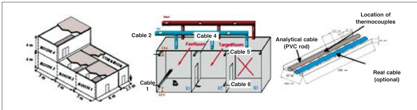
Figura 5.: Instalación DIVA (izda.). Escenario del ejercicio PRS_DI_D3 (centro). Bandejas de cables (dcha.)
