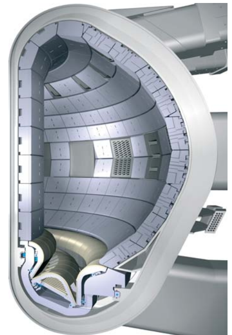
Sección de la cámara del reactor.
