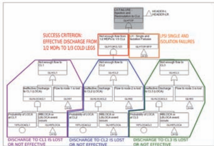
Figura 3. Top del FT del LPSI en el modelo genérico SPAR-CSN.
