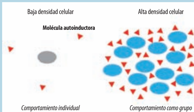
Mecanismo de Quorum Sensing .
