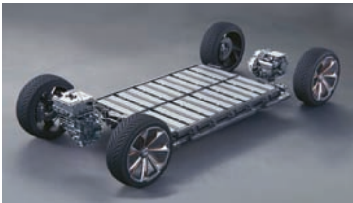
Batería de litio de un coche eléctrico y conexiones de alimentación. Derecha, batería de níquel de Tesla y la Universidad Dalhousie, montada en un prototipo.
