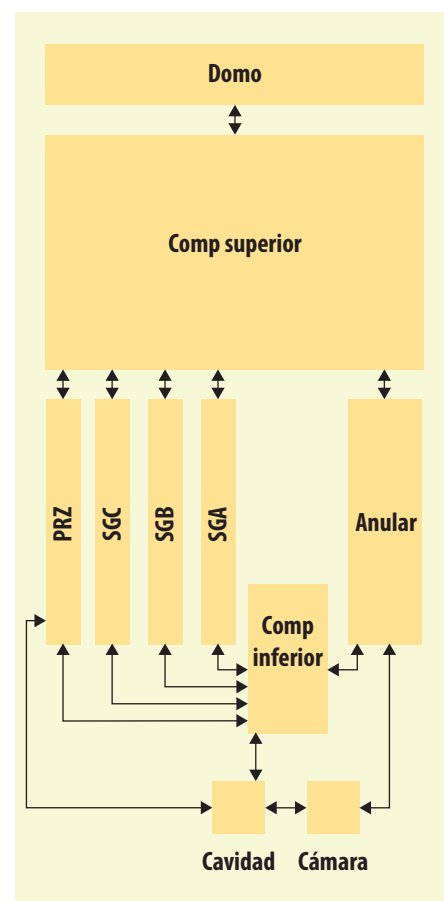
Figura 1. Nodalización del recinto de contención.
