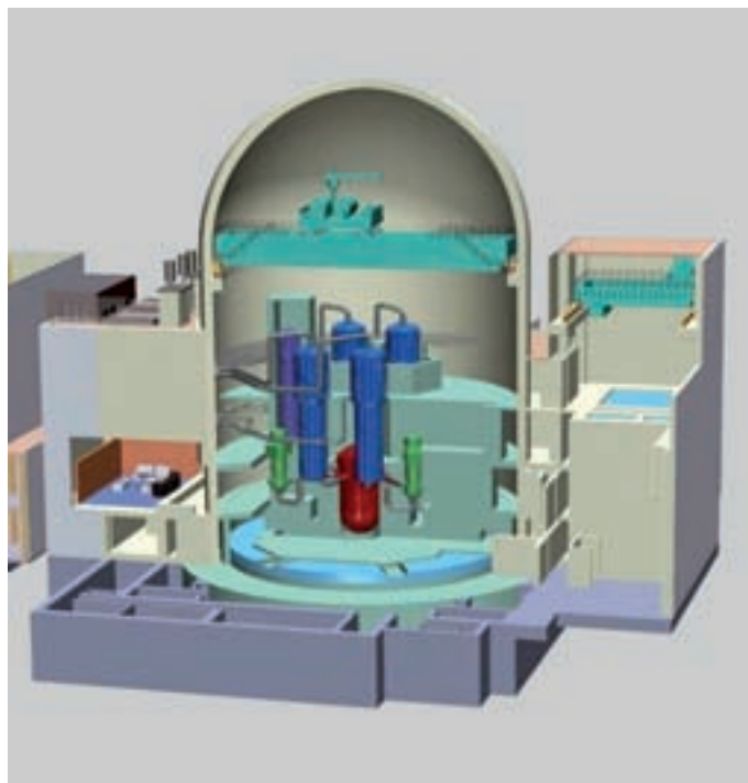
Sección transversal de un RC en un reactor PWR de tecnología americana.
