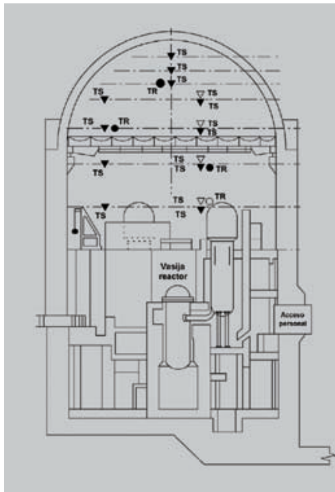
Situación de sensores de temperatura seca (TS) y de rocío (TR) en la parte superior del RC para una prueba ILRT
