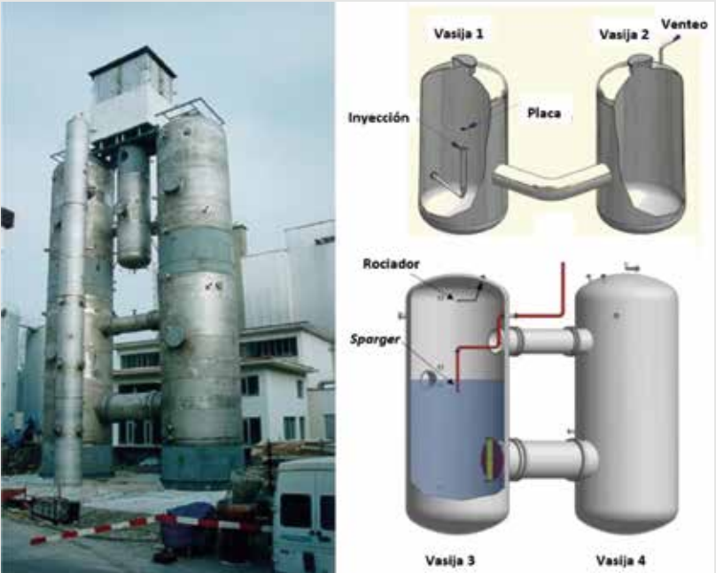
Figura 1. Instalación experimental PANDA. Fuente: PSI
