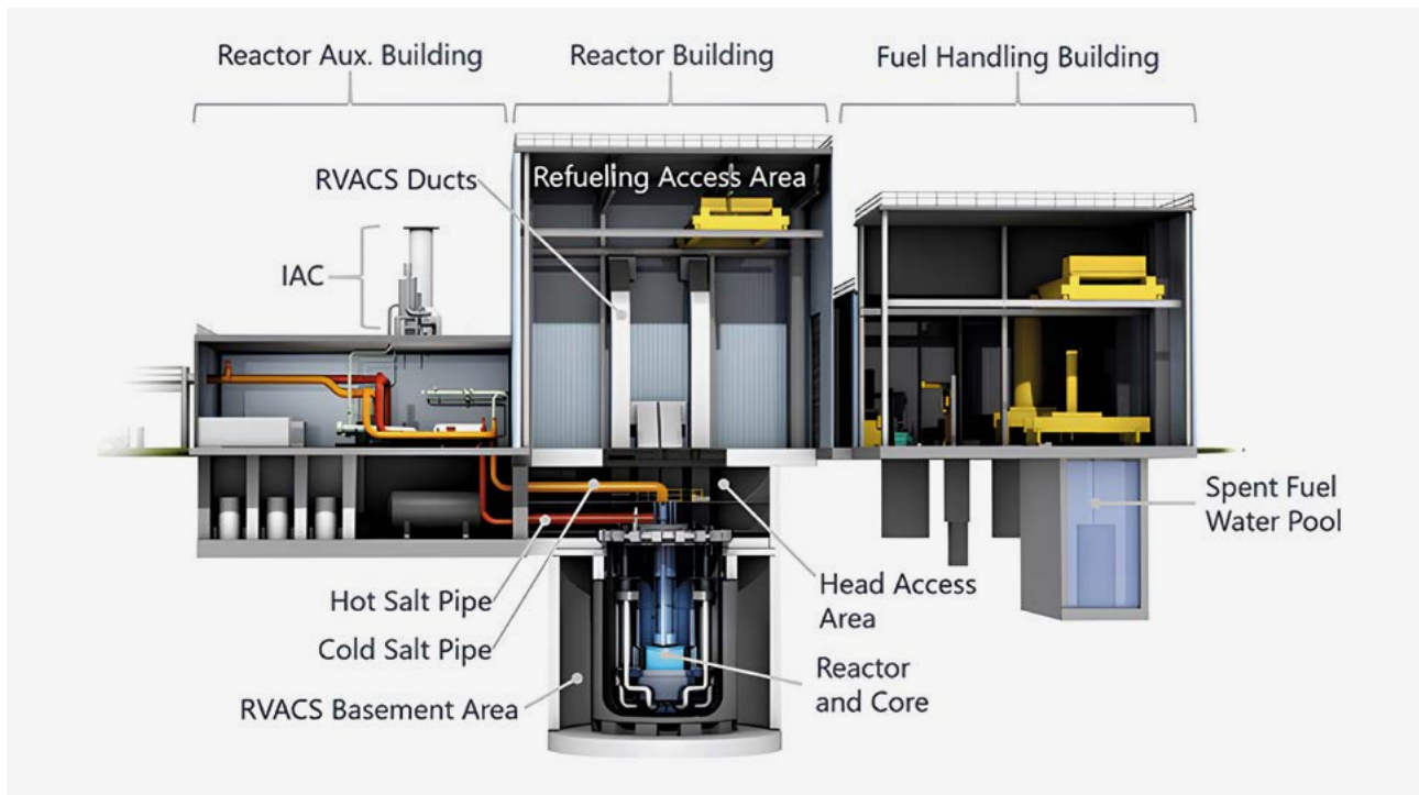
Figura 3. Esquema del reactor rápido de sodio Natrium
