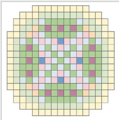
Figura 1. Geometría del reactor BIBLIS 2D donde se describen los distintos materiales que lo componen, con las secciones eficaces homogenizadas y dadas para dos grupos de energía.
