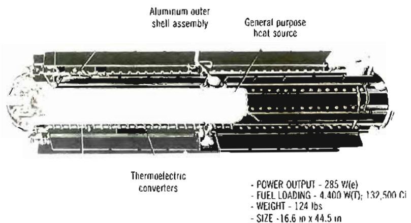
Figura 5. Generador de electricidad por radioisótopos para un cohete espacial.
