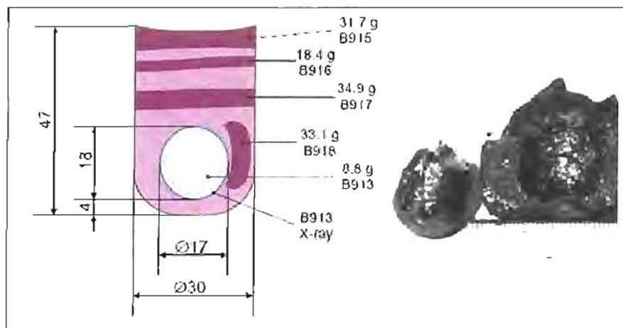
Figura 1. Esquema y fotografía del estado final del corium en el experimento STFM-Fe 10.
