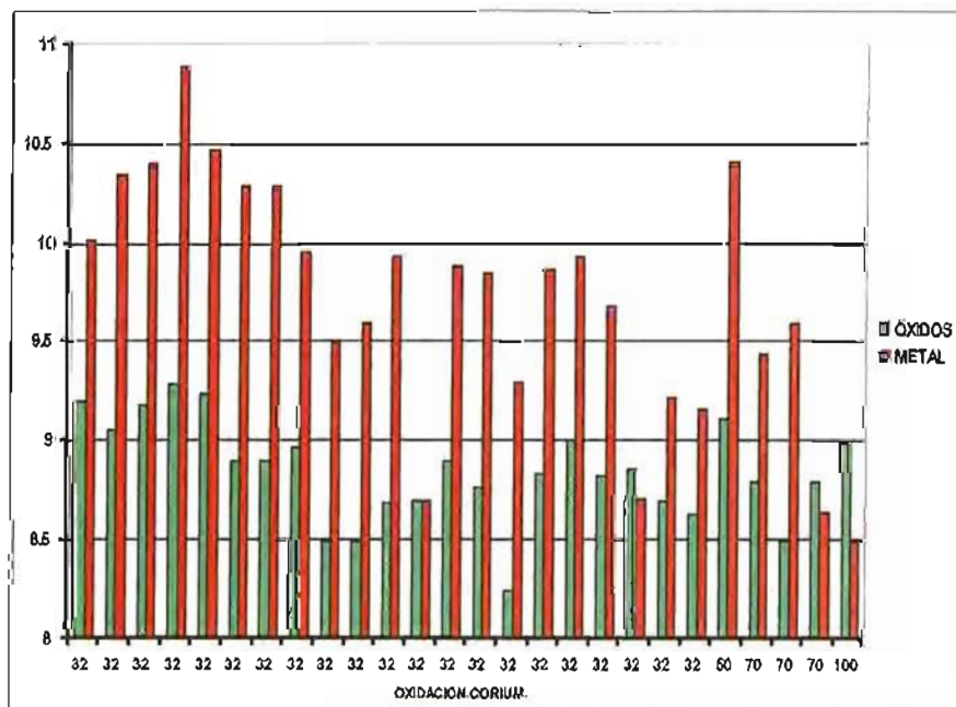
Figura 3. Densidad de las capas metálicas y de óxidos en los experimentos STFM-Ox (con atmósfera oxidante).
