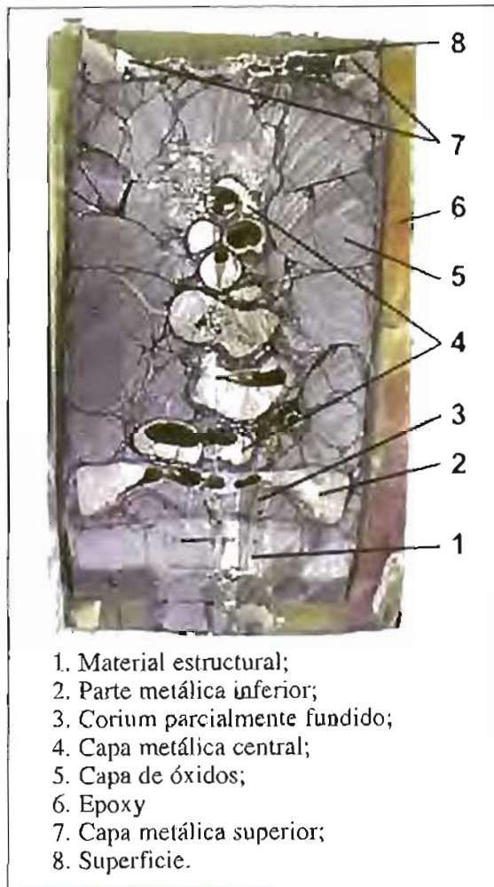
Figura 5. Estado final del corium en el experimento RCW-1
