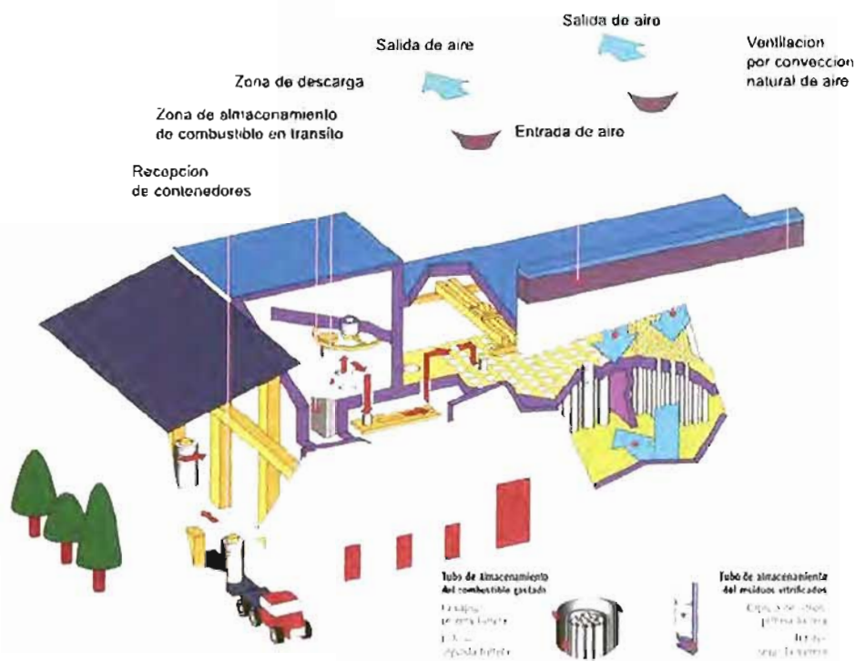
Ilustración del diseño conceptual del ATC en un edificio tipo bóveda con pozos o tubos metálicos.
