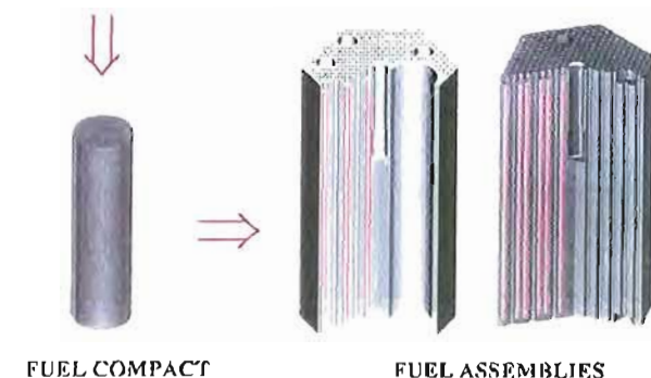
Figura 3. Combustible de un reactor de la generación IV.
