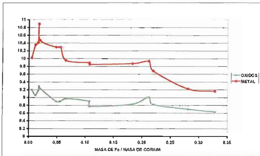
Figura 2. Densidad de las capas metálicas y de óxidos en los experimentos a pequeña escala STFM-Fe. Grado de oxidación del corium 32%.
