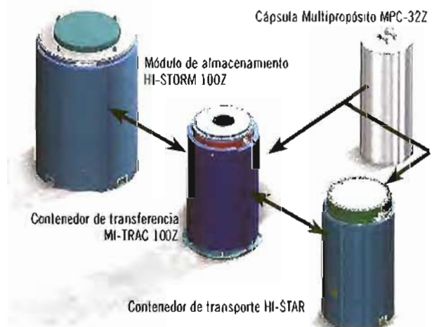
Figura 2. Componentes del sistema HI-STORM para la central nuclear José Cabrera.
