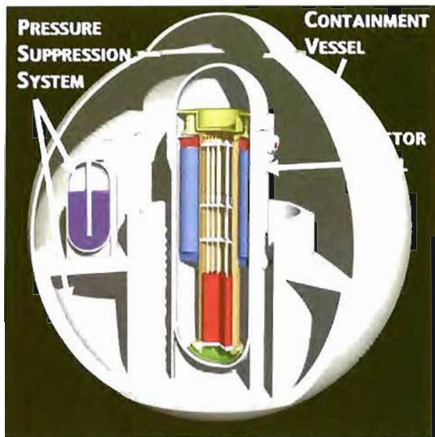
Figura 2. Esquema del recinto de contención del reactor IRIS.
