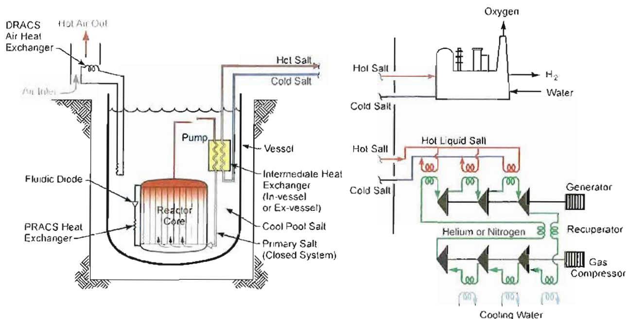
Figura 4. Esquema de un reactor de alta temperatura refrigerado por gas.
