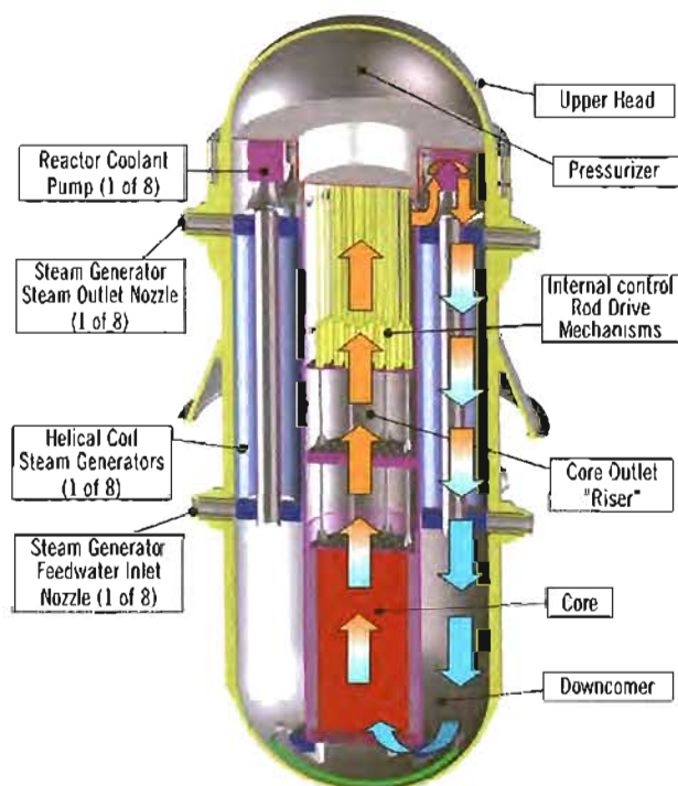
Figura 1. Diseño de la vasija del reactor IRIS.
