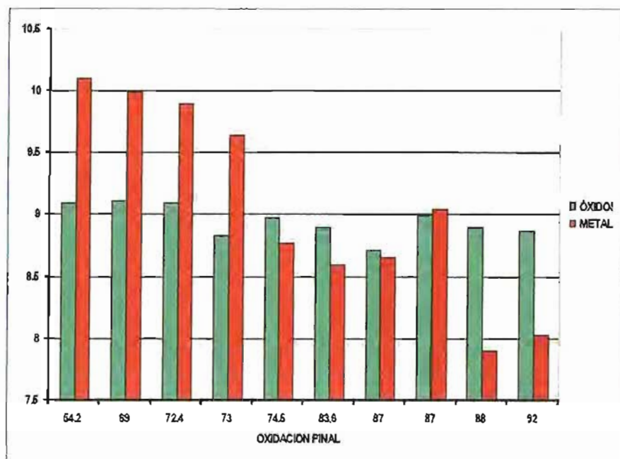
Figura 4. Densidad de las capas metálicas y de óxidos en los experimentos STFM-Ox (con atmósfera oxidante).
