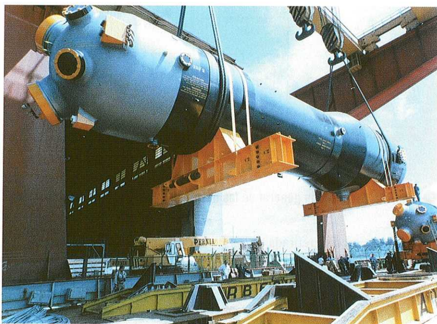
► Figura 4. Embarque de un generador de vapor para la central nuclear de Almaraz en la fábrica de Equipos Nucleares.
