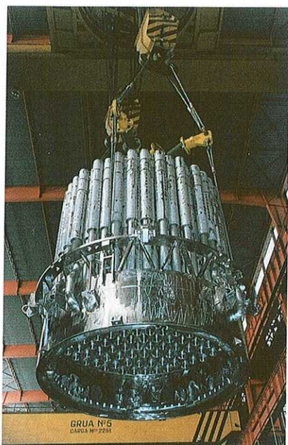
► Figura 5. Soporte del núcleo de la central nuclear de Olkiluoto (Finlandia).
