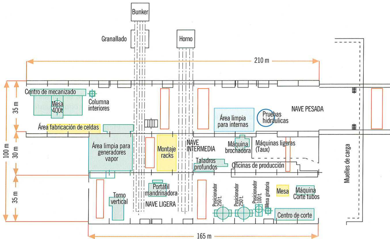
► Figura 3. Disposición general de las naves de producción de la fábrica de Equipos Nucleares.
