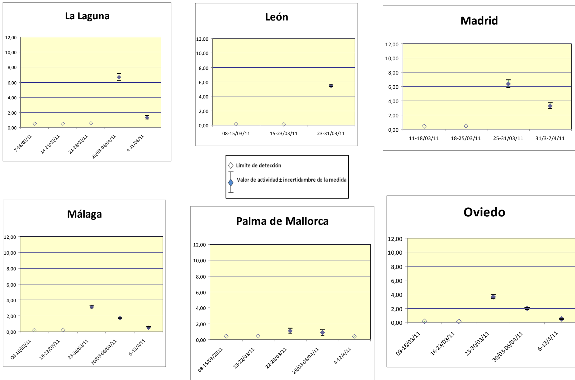
Figura 4/2. Evolución de las concentraciones de actividad de I-131 medidas en cartuchos de carbón activo de la red de estaciones de muestreo del CSN (Red densa) (miliBq/m 3 )
