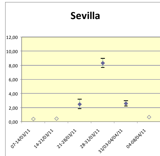
Figura 4/3. Evolución de las concentraciones de actividad de I-131 medidas en cartuchos de carbón activo de la red de estaciones de muestreo del CSN (Red densa) (miliBq/m 3 )
