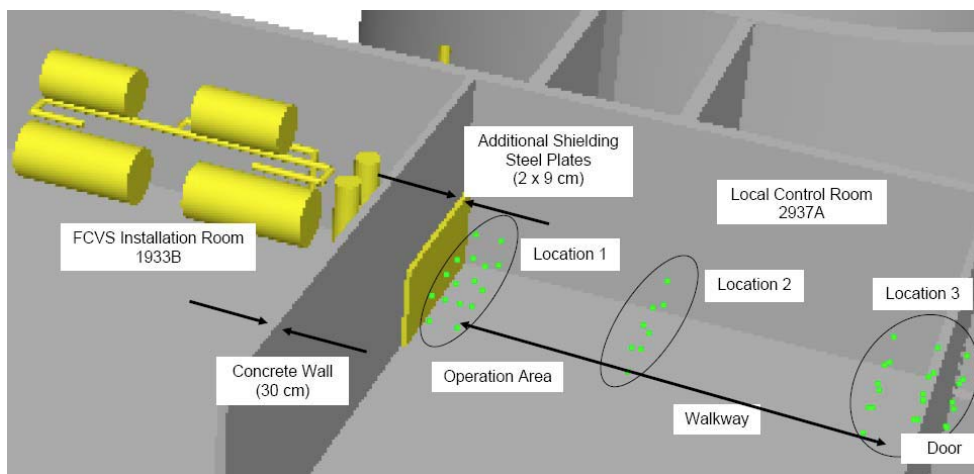
Figura 9. Acceso y blindaje del cuarto de control local
