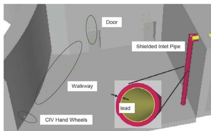
Figura 7. Acceso a los mandos a distancia para la abertura de las Válvulas aislamiento de la contención.
