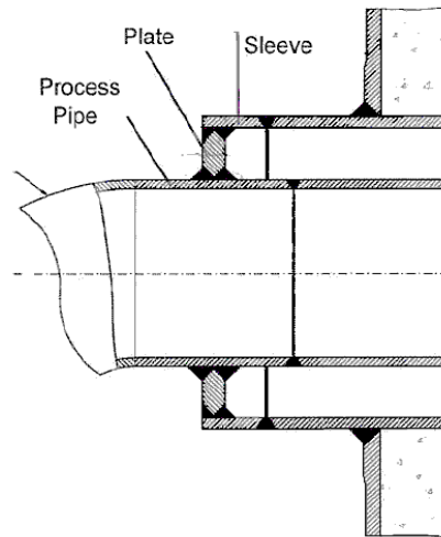
Figura 5. Diseño propuesto por el titular para la penetración del SVFC en CN Ascó II
