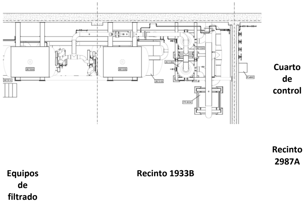
Figura 3. Conjunto de filtros en el edificio auxiliar y cuarto de control
