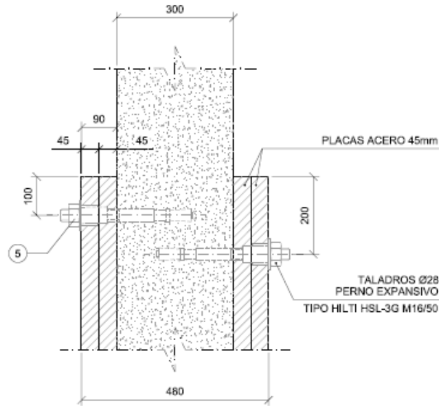
Figura 8. Blindaje pared separación entre filtros y el cuarto de control local
