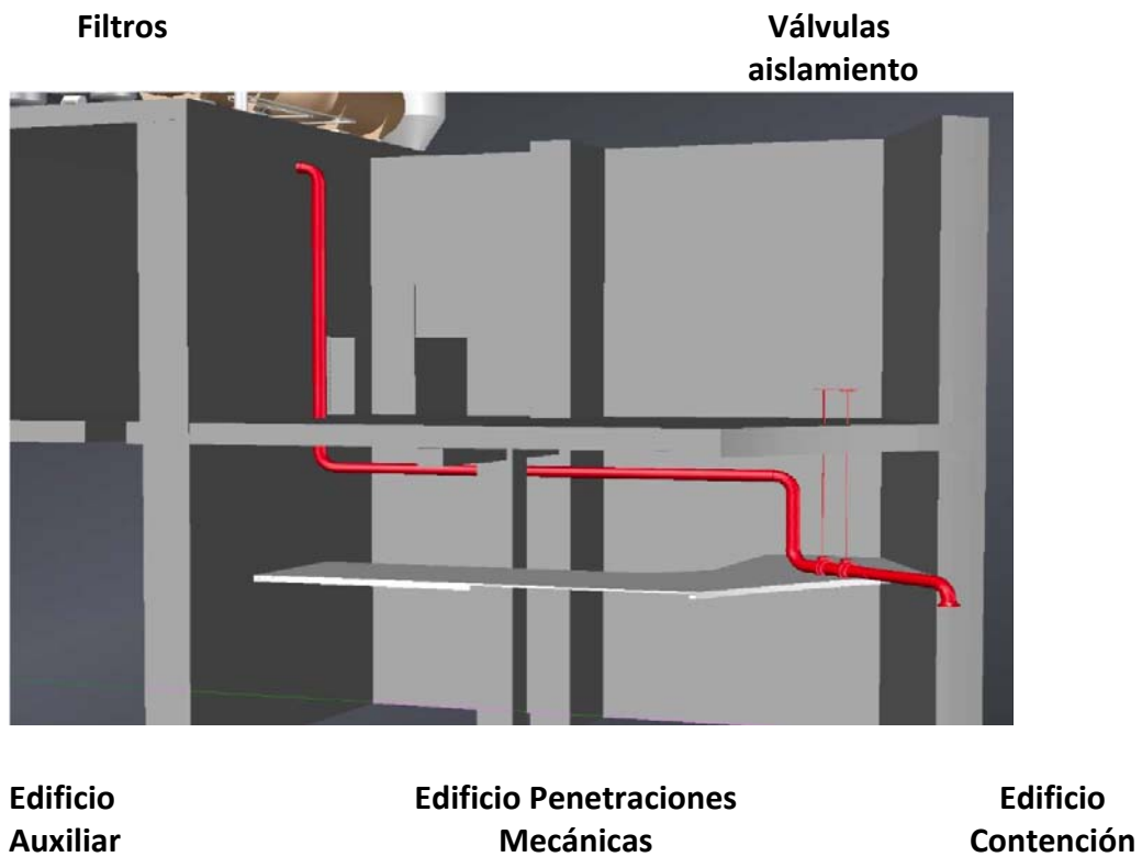
Figura 1. Válvulas de aislamiento de la contención y tramo de tubería hasta los filtros del SVCF
