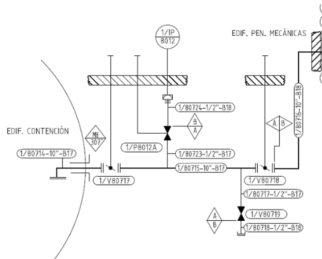
Figura 5. Diseño propuesto por el titular para la penetración del SVFC en CN Ascó II
