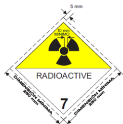
Placa-etiqueta 7D
