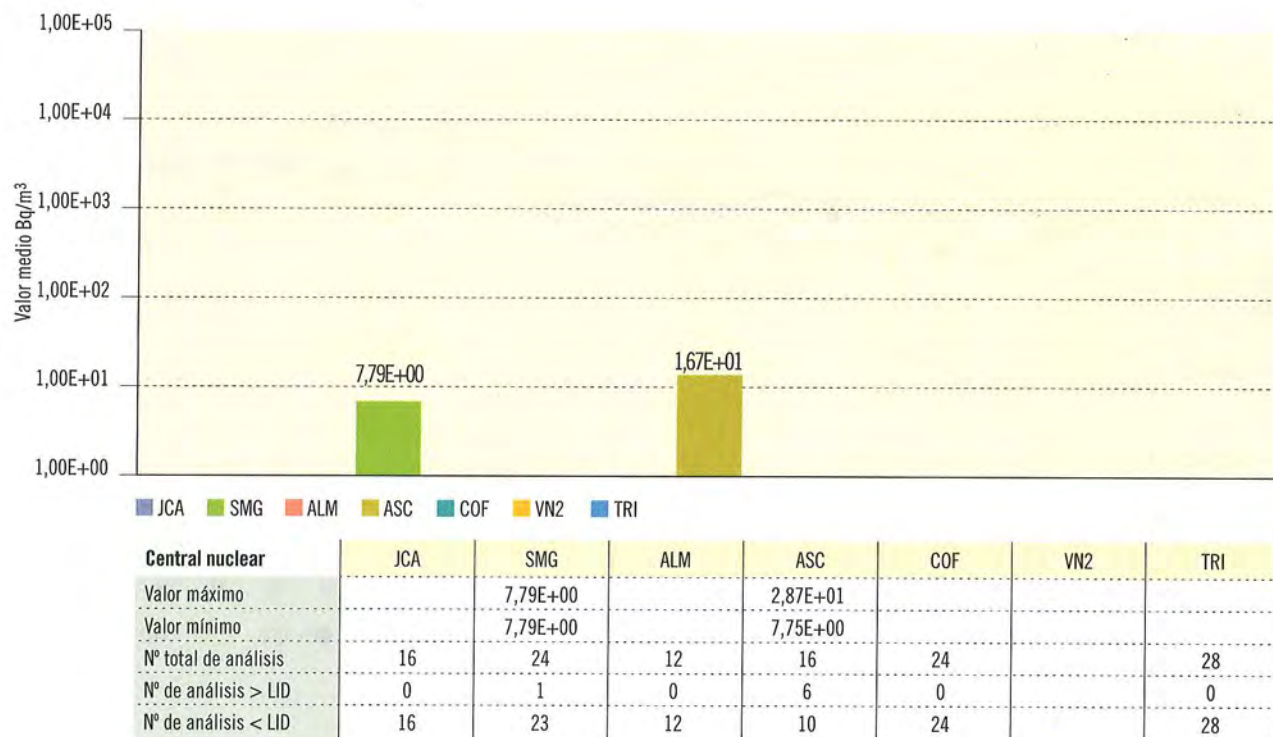
Figura 2.24b. Agua potable. Concentración de actividad de Sr-90 (Bq/m³)
