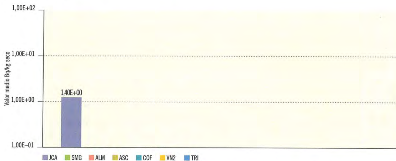
Figura 2.16b. Suelo. Concentración de actividad de Cs-134 (Bq/kg seco)
