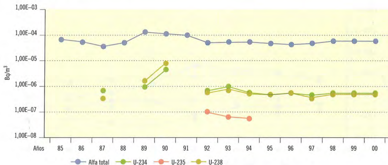
Figura 2.50. Juzbado. Partículas de polvo en el aire. Valores de concentración de actividad (Bq/m 3 )
