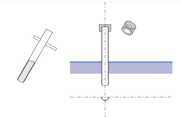
Figura 2. Cilindro de toma de muestras artesanal
