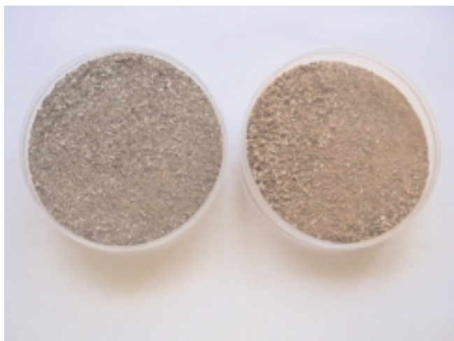
Figura 6. Diferencia de tonalidad de una muestra de sedimento seco (izquierda) y tras su calcinación a 600°C durante 24 horas (derecha)
