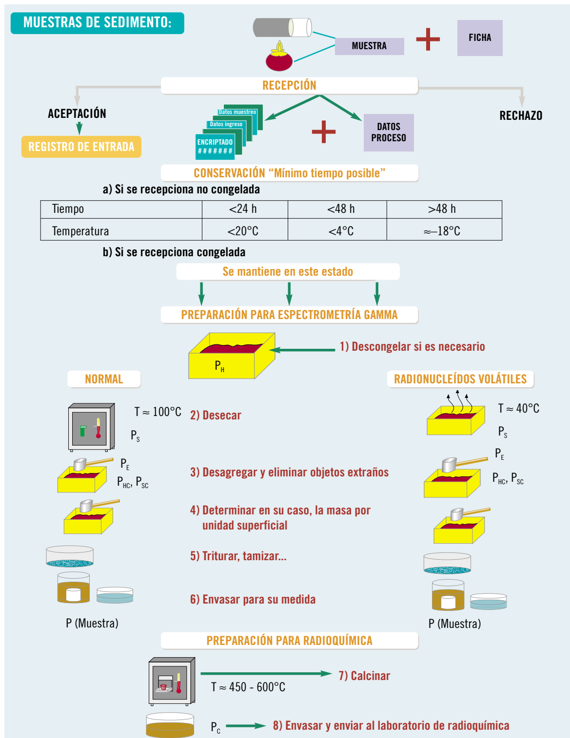
Figura 1. Esquema del procedimiento para la recepción, conservación y preparación de sedimentos
