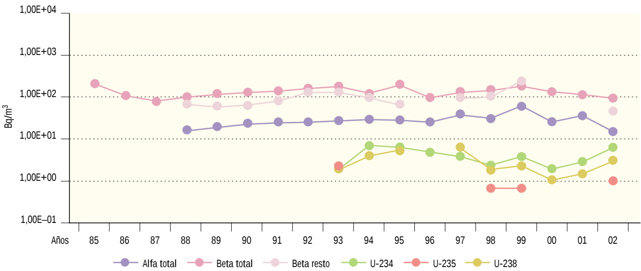
Figura 2.64. Juzbado. Agua potable. Valores de concentración de actividad (Bq/m³) Evolución temporal valores medios
