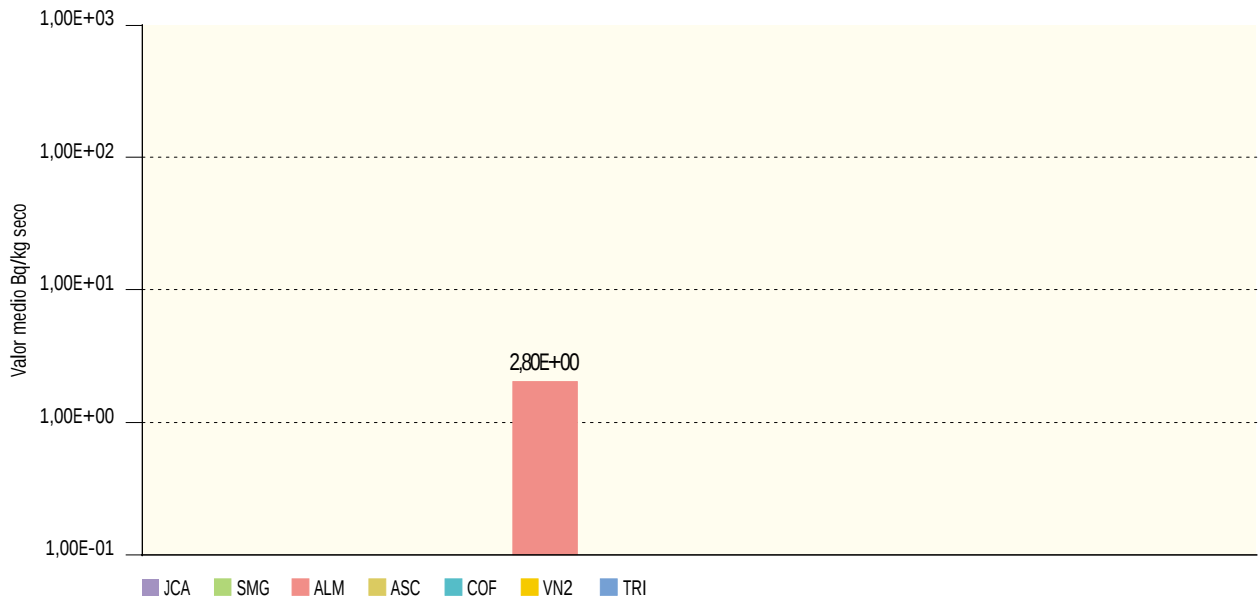
Figura 2.28b. Sedimentos de fondo. Concentración de actividad de Cs-134 (Bq/kg seco) Valores de la campaña de 2002
