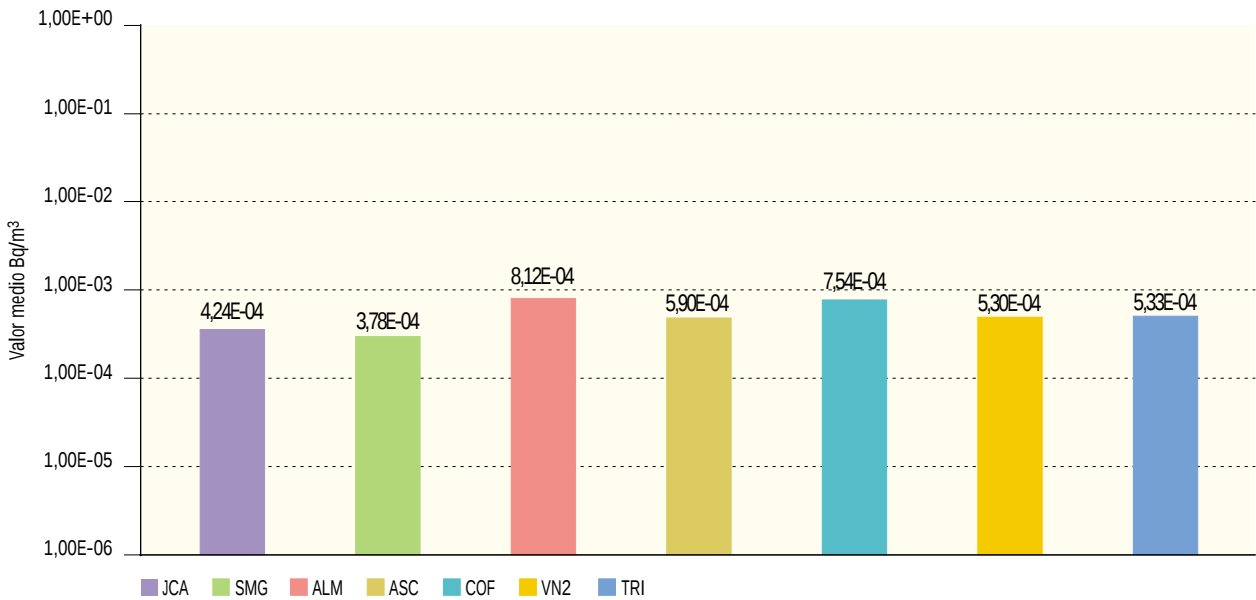
Figura 2.8b. Partículas de polvo en el aire. Concentración del índice de actividad beta total (Bq/m³) Valores de la campaña de 2002
