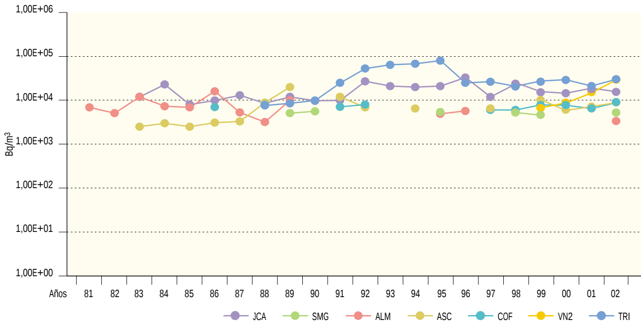
Figura 2.25b. Agua potable. Concentración de actividad de H-3 (Bq/m³) Valores de la campaña de 2002
