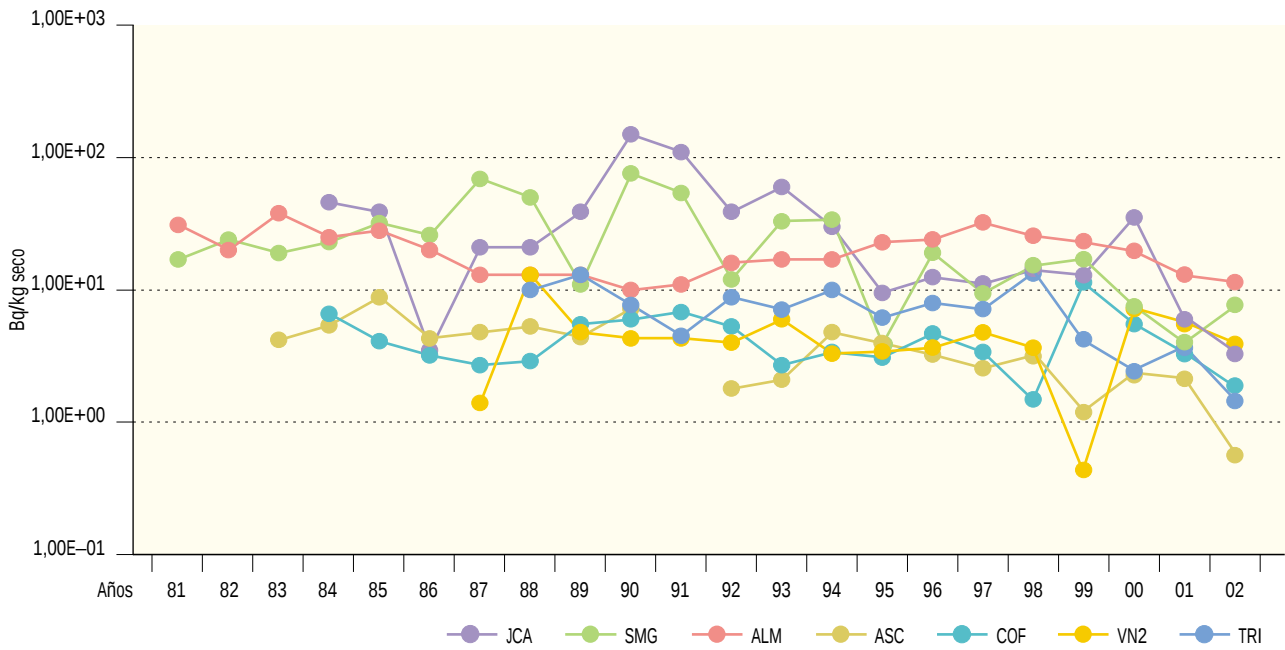
Figura 2.27b. Sedimentos de fondo. Concentración de actividad de Cs-137 (Bq/kg seco) Valores de la campaña de 2002
