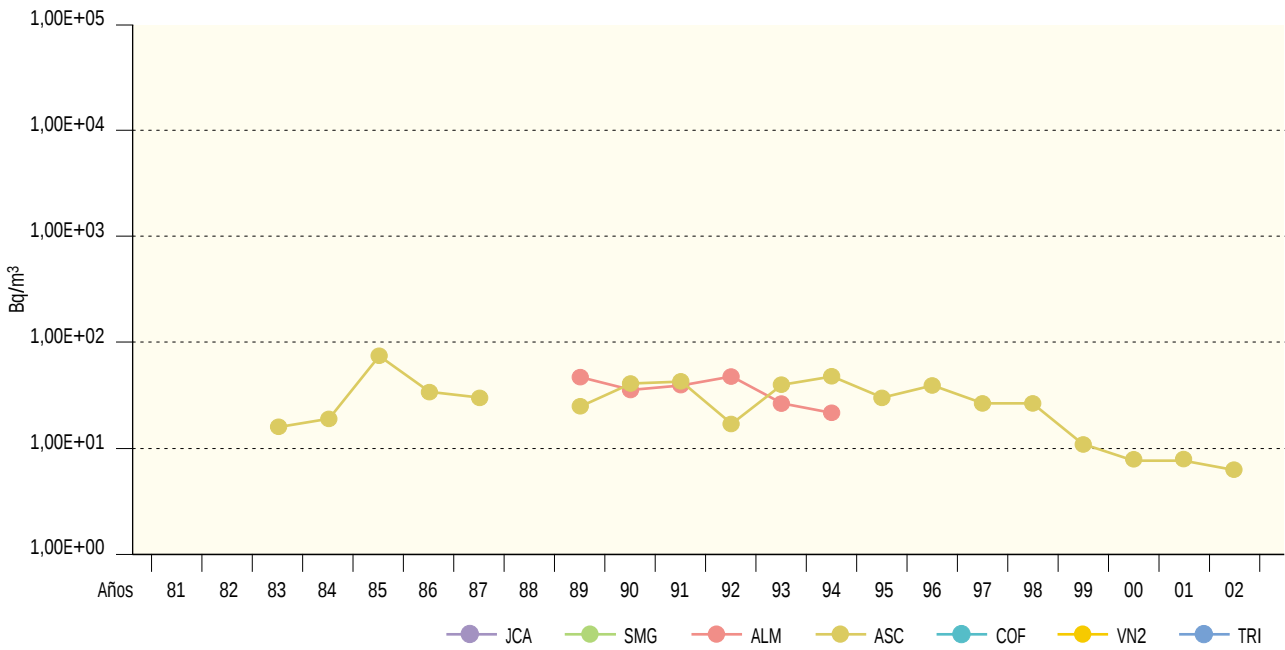
Figura 2.20a. Agua superficial. Evolución temporal de la concentración de actividad de Sr-90 Valores medios en la zona vigilada
