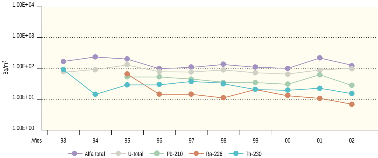
Figura 2.65. Quercus. Agua potable. Valores de concentración de actividad (Bq/m³) Evolución temporal valores medios
