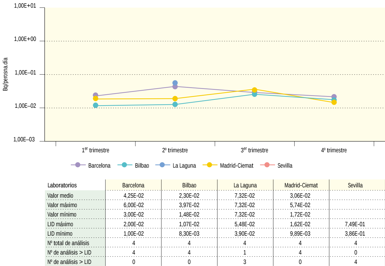
Figura 3.19. Dieta tipo. Concentración de actividad de Cs-137 (Bq/persona.día) Valores de la campaña de 2002
