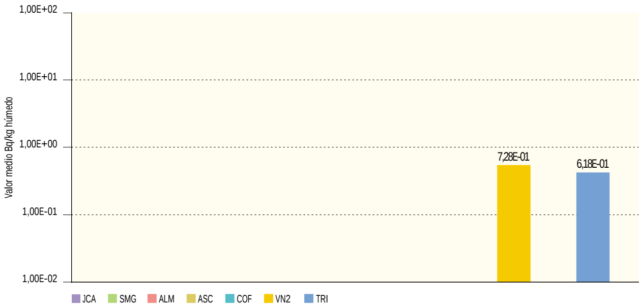
Figura 2.46b. Miel. Concentración de actividad de Cs-137 (Bq/kg húmedo)
