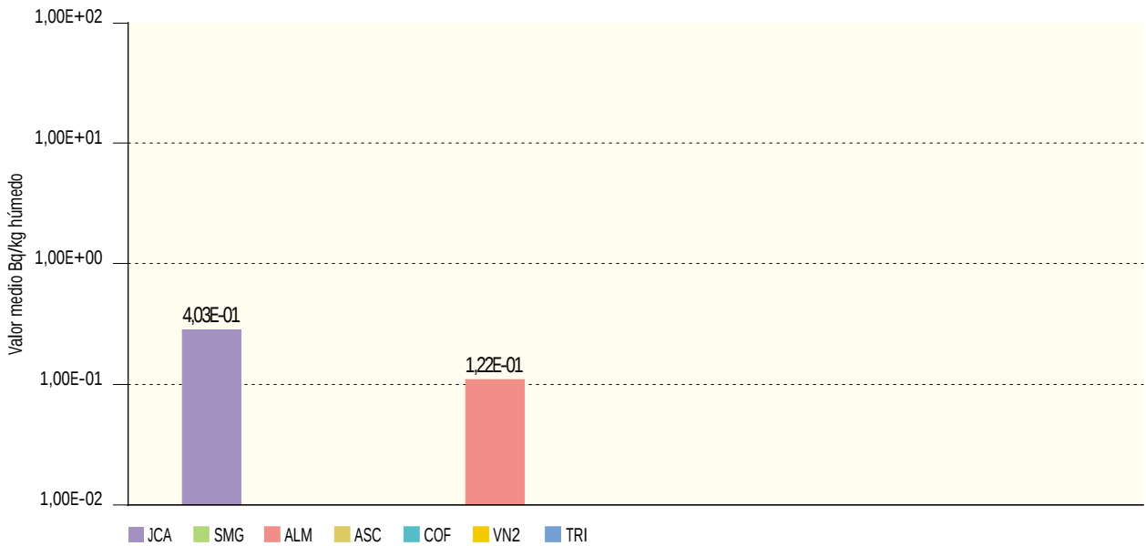
Figura 2.40b. Vegetales de hoja ancha. Concentración de actividad de Cs-137 (Bq/kg húmedo) Valores de la campaña de 2002
