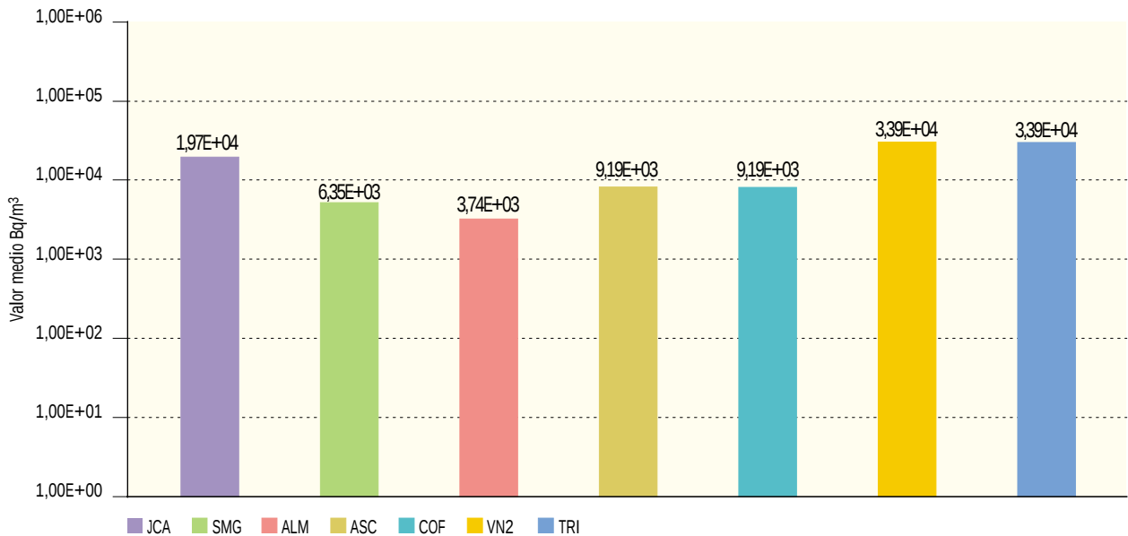
Figura 2.25b. Agua potable. Concentración de actividad de H-3 (Bq/m³) Valores de la campaña de 2002
