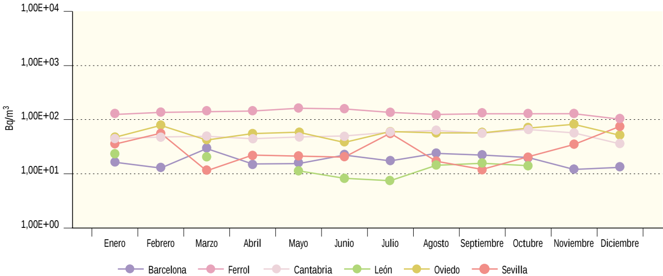
Figura 3.16. Leche. Concentración de actividad de Sr-90 (Bq/m³) Valores de la campaña de 2002
