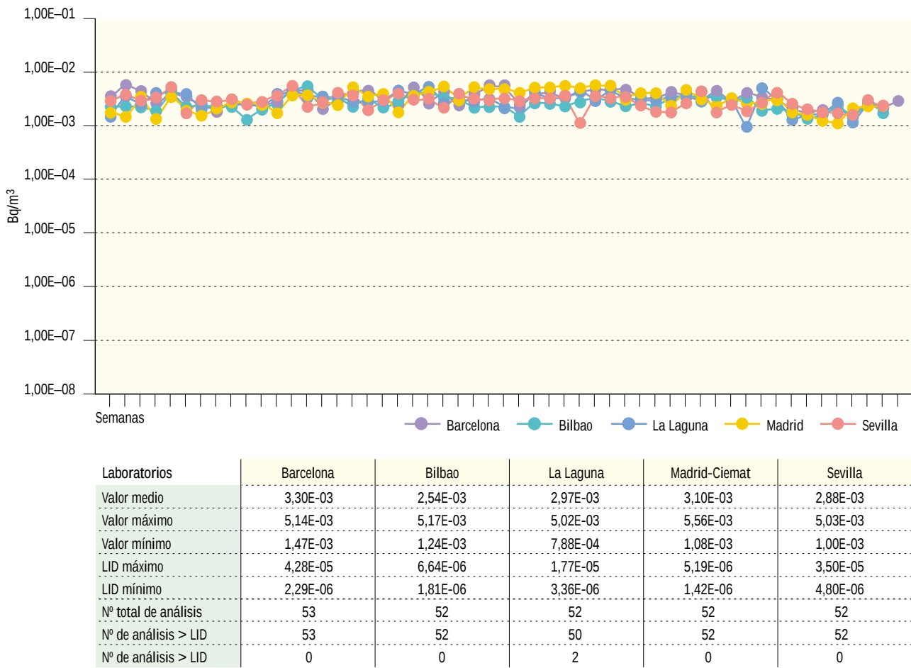
Figura 3.6. Partículas de polvo en el aire. Muestreador alto flujo Concentración de actividad de Be-7 (Bq/m³). Valores de la campaña de 2002
