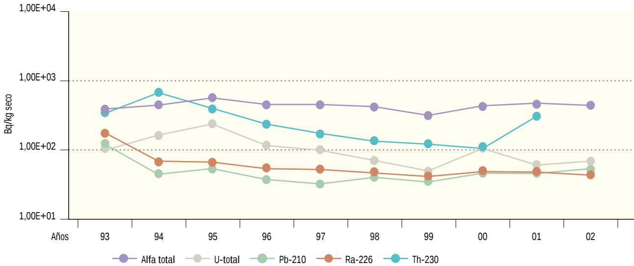
Figura 2.59. Quercus. Suelo. Valores de concentración de actividad (Bq/kg seco) Evolución temporal valores medios
