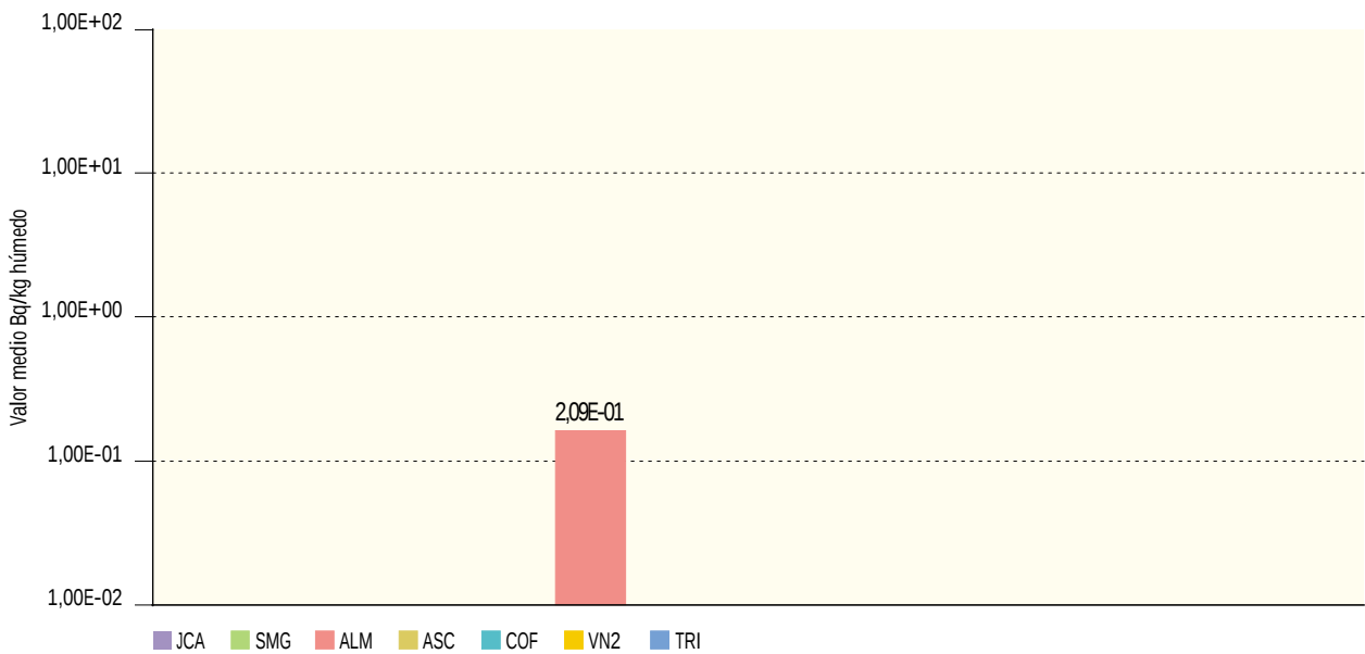
Figura 2.44b. Carne y aves. Concentración de actividad de Cs-137 (Bq/kg húmedo) Valores de la campaña de 2002
