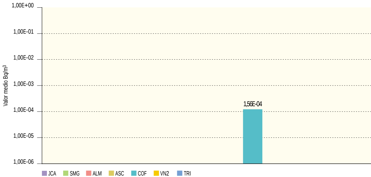
Figura 2.11b. Partículas de polvo en el aire. Concentración de actividad de Co-60 (Bq/m³) Valores de la campaña de 2002
