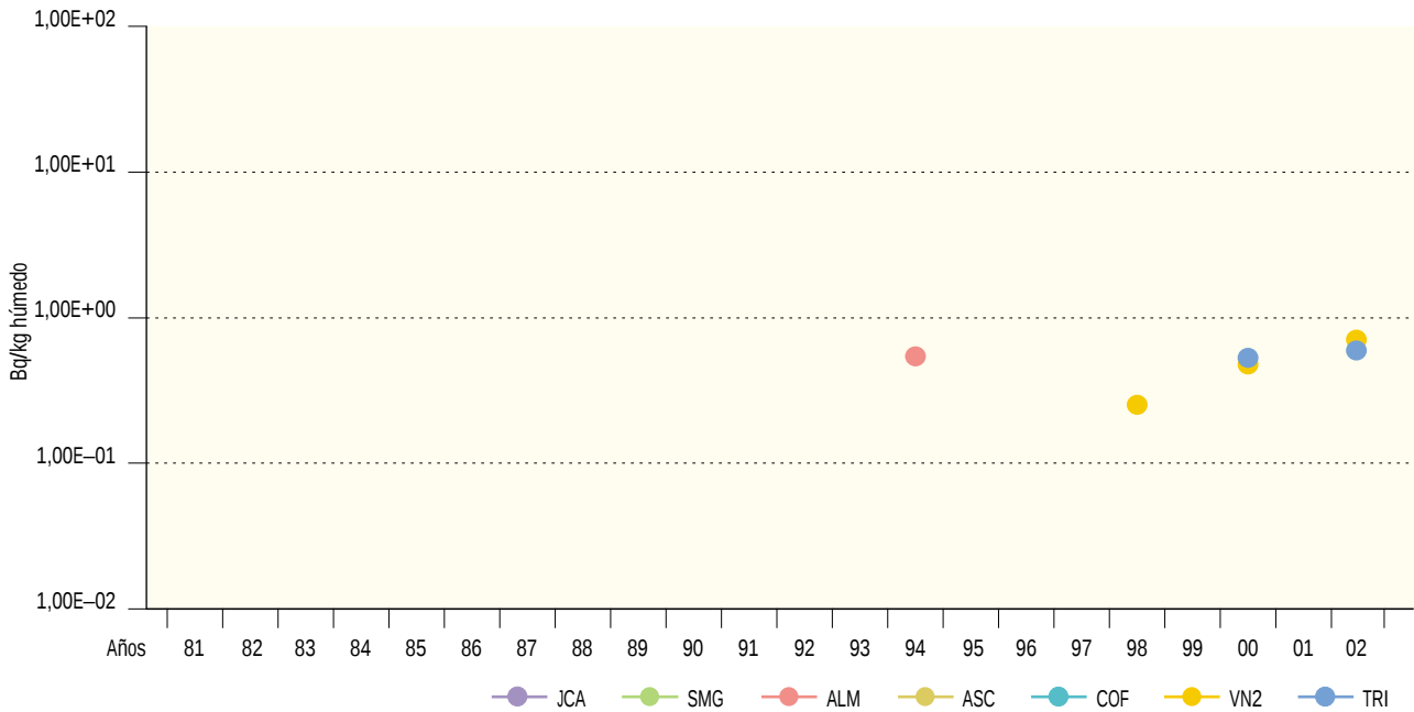
Figura 2.46b. Miel. Concentración de actividad de Cs-137 (Bq/kg húmedo)
