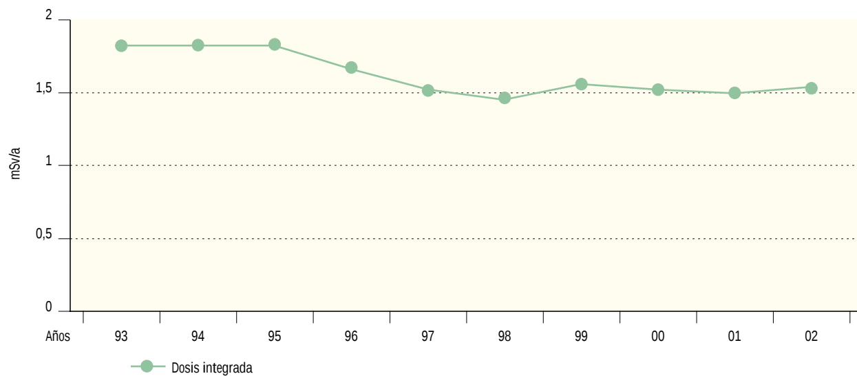
Figura 2.56. Quercus. Radiación directa. Dosis integrada (DTL) (mSv/a)
