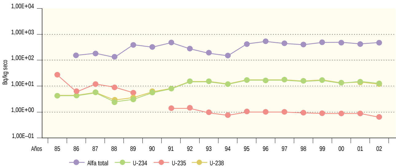
Figura 2.58. Juzbado. Suelo. Valores de concentración de actividad (Bq/kg seco) Evolución temporal valores medios
