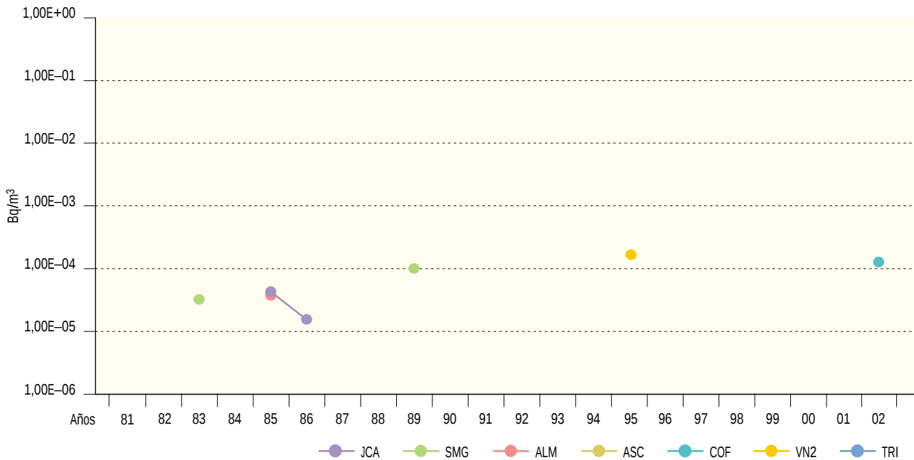
Figura 2.11b. Partículas de polvo en el aire. Concentración de actividad de Co-60 (Bq/m³) Valores de la campaña de 2002
