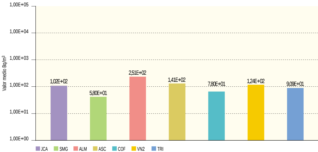
Figura 2.22b. Agua potable. Concentración del índice de actividad beta total (Bq/m³) Valores de la campaña de 2002
