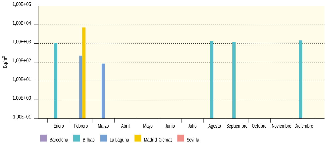
Figura 3.14. Agua potable. Concentración de actividad de H-3 (Bq/m³) Valores de la campaña de 2002
