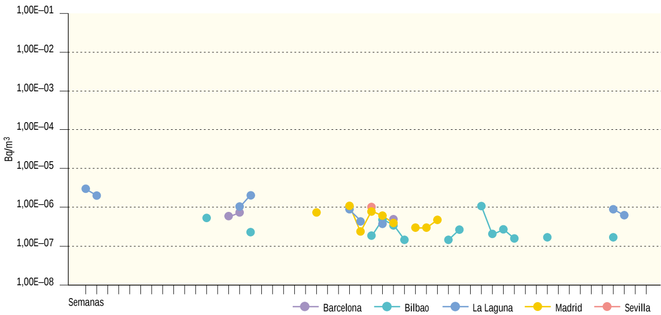
Figura 3.5. Partículas de polvo en el aire. Muestreador alto flujo Concentración de actividad de Cs-137 (Bq/m³). Valores de la campaña de 2002
