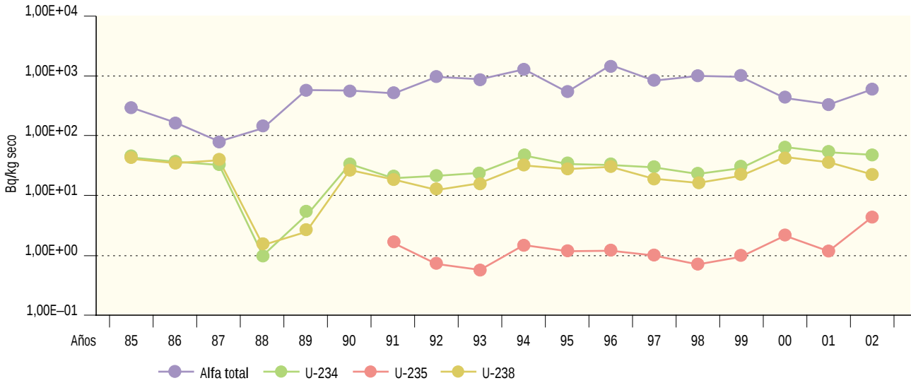
Figura 2.66. Juzbado. Sedimentos de fondo. Valores de concentración de actividad (Bq/kg seco) Evolución temporal valores medios
