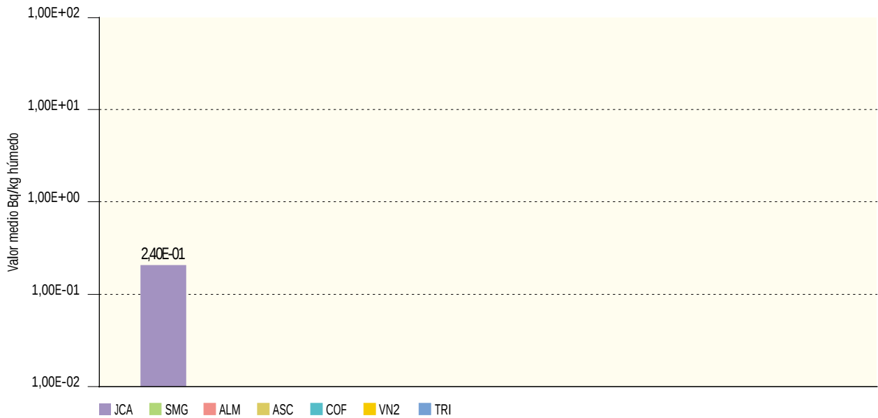
Figura 2.43b. Vegetales de hoja no ancha. Concentración de actividad de Cs-137 (Bq/kg húmedo) Valores de la campaña de 2002
