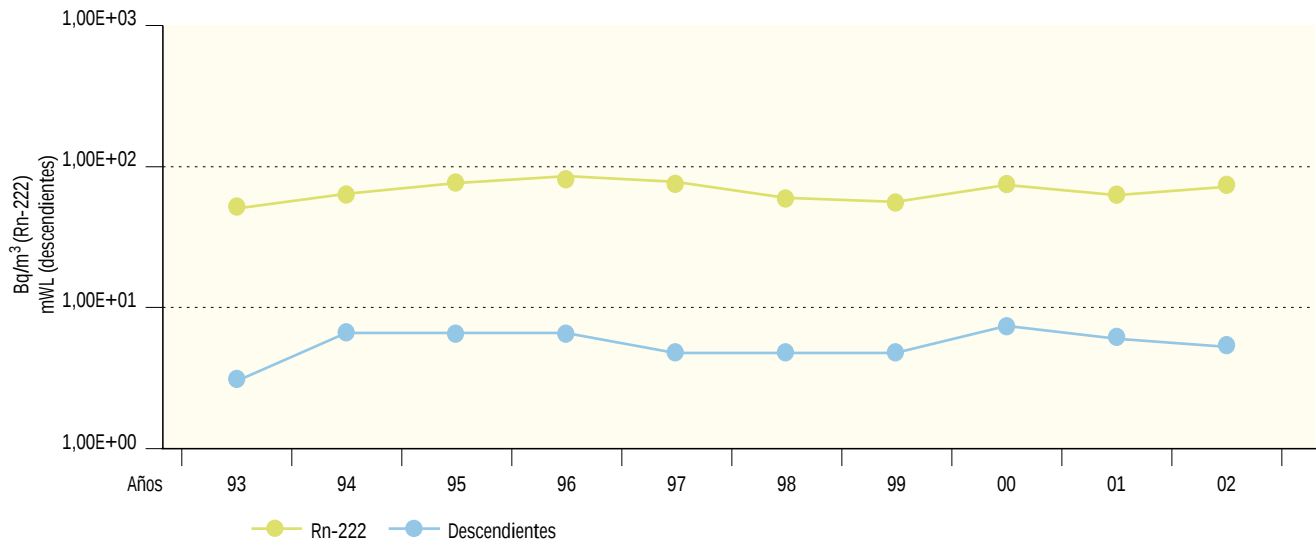
Figura 2.53. Quercus. Radón en el aire. Valores de concentración de actividad Rn-222 (Bq/m³). Descendientes (mWL) Evolución temporal valores medios
