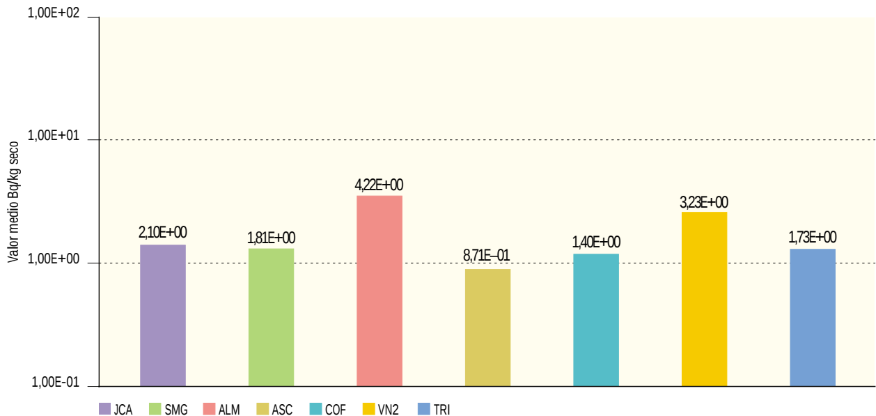
Figura 2.13b. Suelo. Concentración de actividad de Sr-90 (Bq/kg seco) Valores de la campaña de 2003
