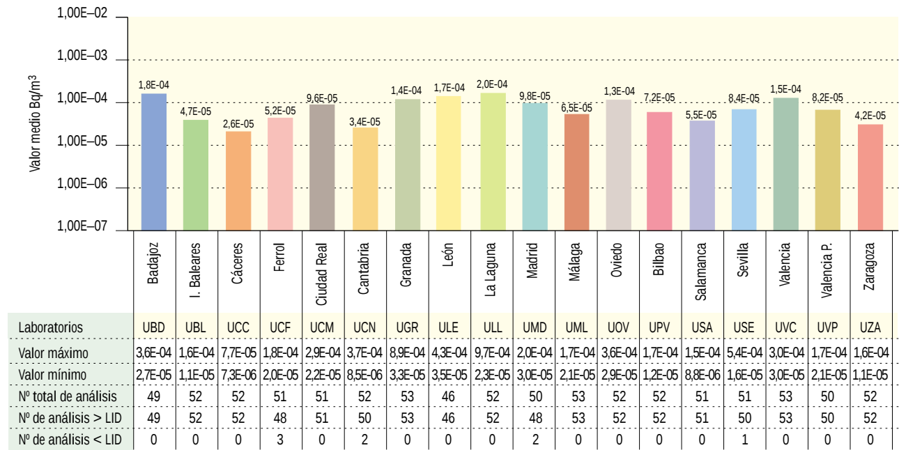
Figura 3.2b. Partículas de polvo en el aire. Concentración del índice de actividad alfa total (Bq/m³) Valores de la campaña de 2003
