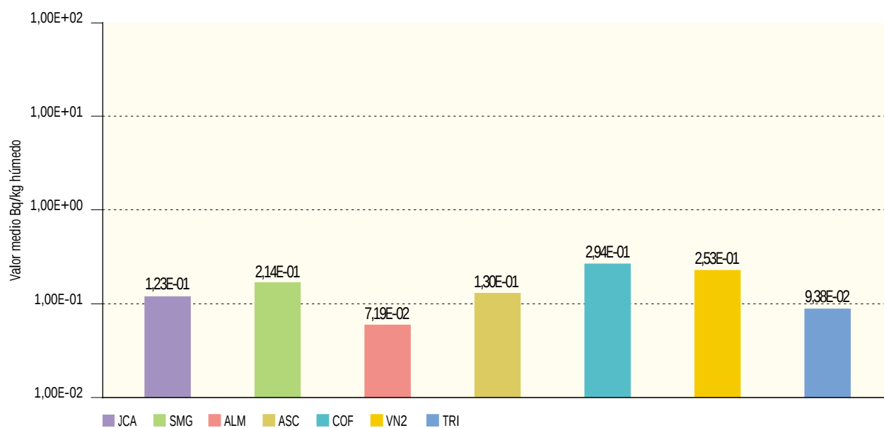
Figura 2.37b. Vegetales de hoja no ancha. Concentración de actividad de Sr-90 (Bq/kg húmedo)
