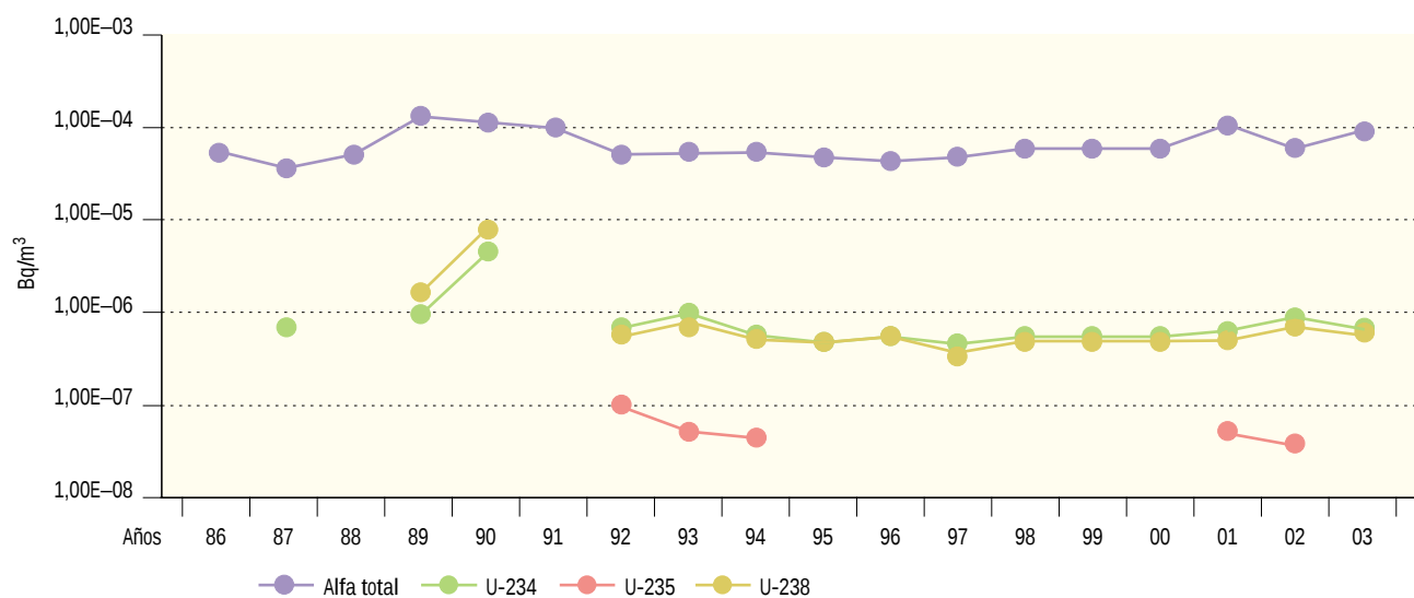
Figura 2.44. Juzbado. Partículas de polvo en el aire. Valores de concentración de actividad ( \text{Bq}/\text{m}^3 )
