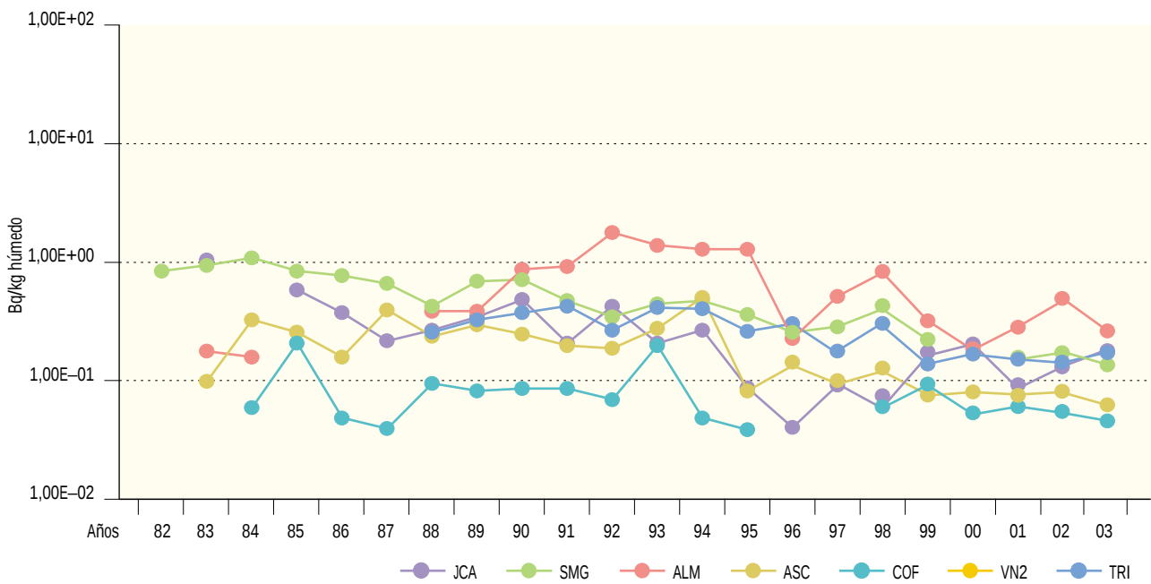
Figura 2.36b. Vegetales de hoja ancha. Concentración de actividad de Sr-90 (Bq/kg húmedo) Valores de la campaña de 2003
