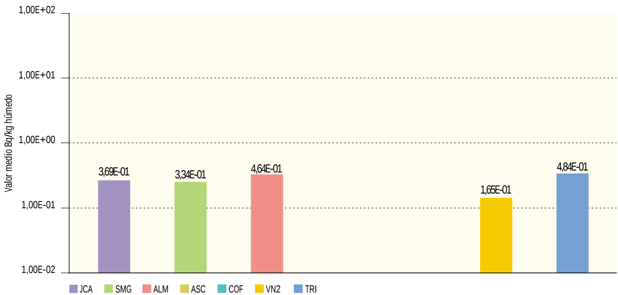
Figura 2.40b. Peces y mariscos. Concentración de actividad de Cs-137 (Bq/kg húmedo) Valores de la campaña de 2003
