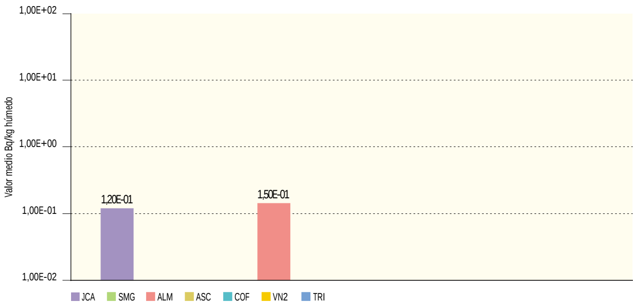
Figura 2.38b. Vegetales de hoja no ancha. Concentración de actividad de Cs-137 (Bq/kg húmedo) Valores de la campaña de 2003
