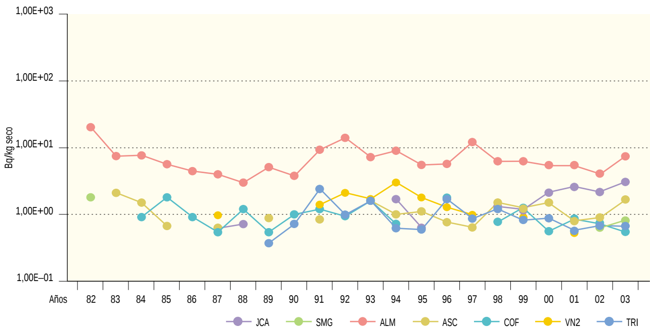
Figura 2.23b. Sedimentos de fondo. Concentración de actividad de Sr-90 (Bq/kg seco) Valores de la campaña de 2003
