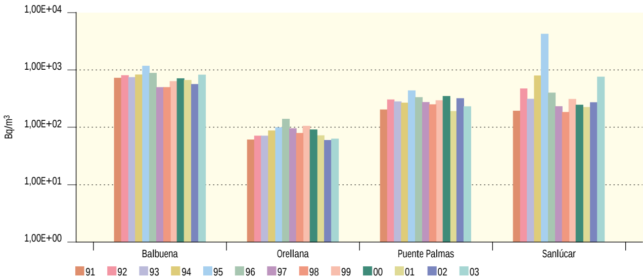
Figura 3.38. Río Gadiana Evolución temporal del índice de actividad beta total
