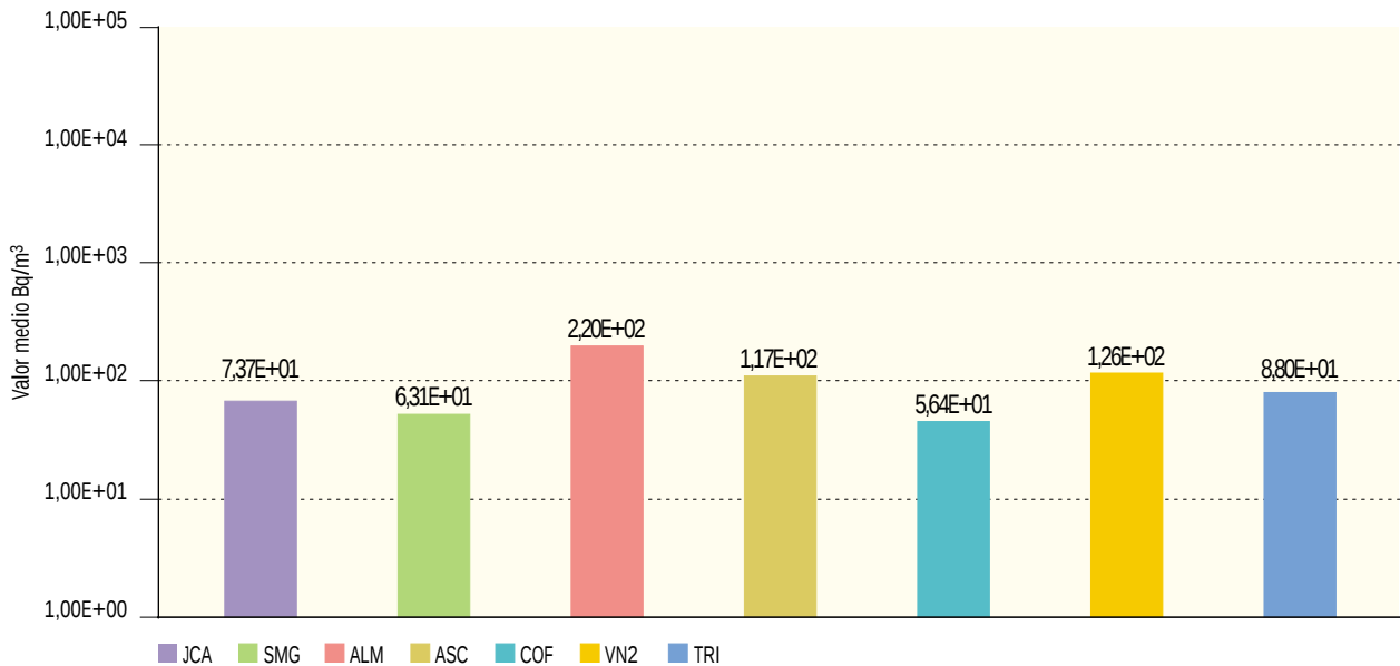
Figura 2.19b. Agua potable. Concentración del índice de actividad beta total (Bq/m³) Valores de la campaña de 2003
