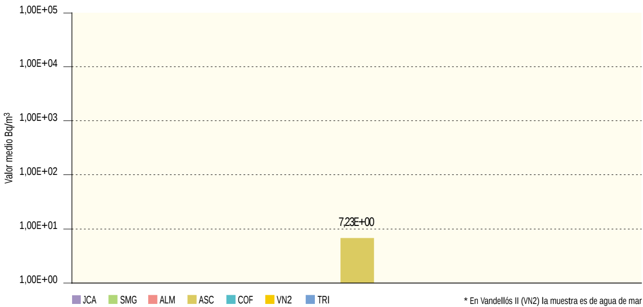
Figura 2.17b. Agua superficial. Concentración de actividad de Sr-90 (Bq/m³) Valores de la campaña de 2003
