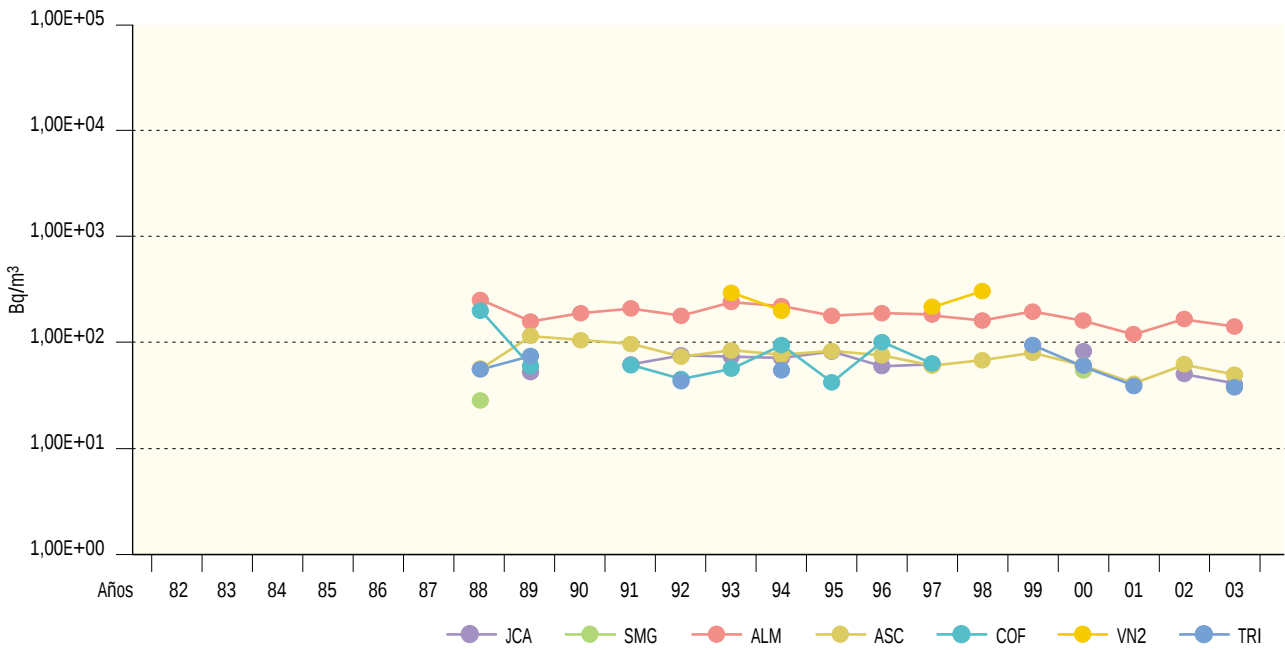
Figura 2.20b. Agua potable. Concentración del índice de actividad beta resto (Bq/m³) Valores de la campaña de 2003
