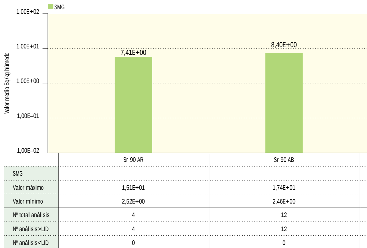
Figura 2.33b. Fauna terrestre. Concentración de actividad (Bq/kg húmedo)
