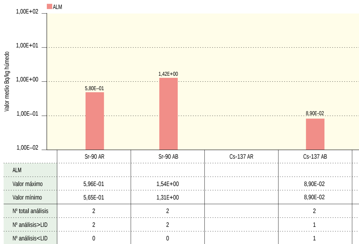
Figura 2.31b. Plantas terrestres. Concentración de actividad (Bq/kg húmedo)
