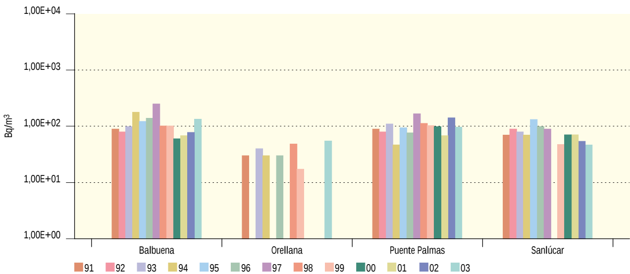
Figura 3.37. Río Gadiana Evolución temporal del índice de actividad alfa total
