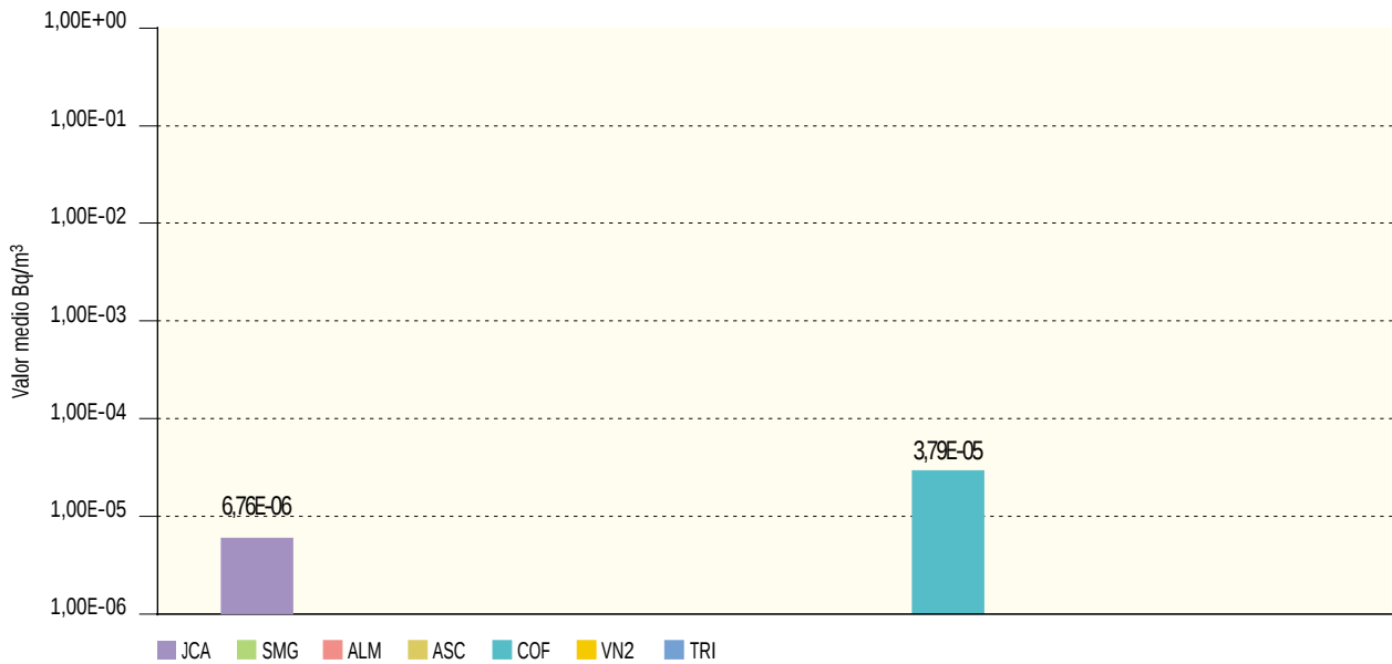
Figura 2.11b. Partículas de polvo en el aire. Concentración de actividad de Co-60 (Bq/m³) Valores de la campaña de 2003
