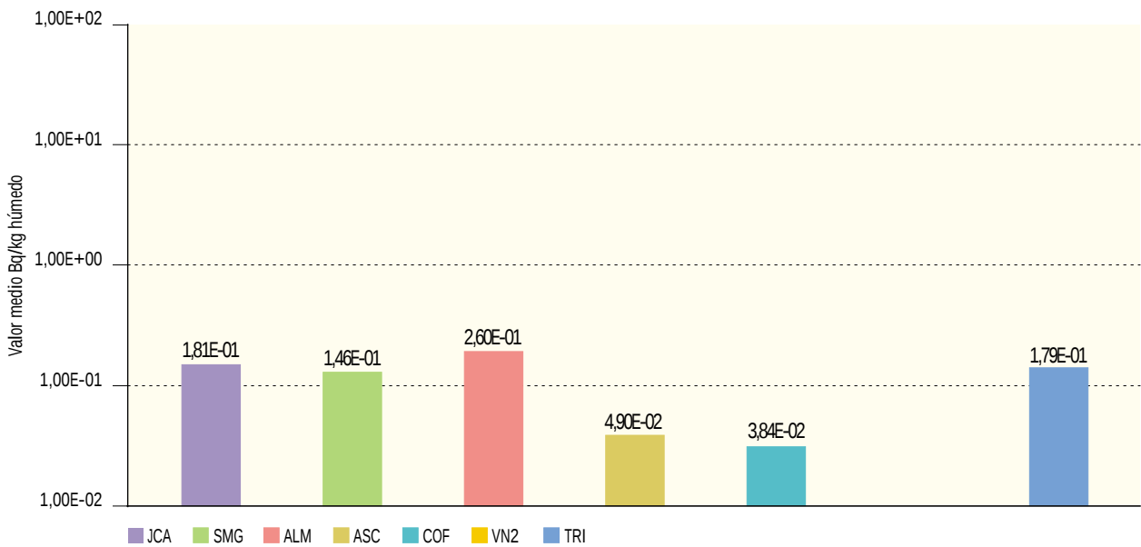
Figura 2.36b. Vegetales de hoja ancha. Concentración de actividad de Sr-90 (Bq/kg húmedo) Valores de la campaña de 2003
