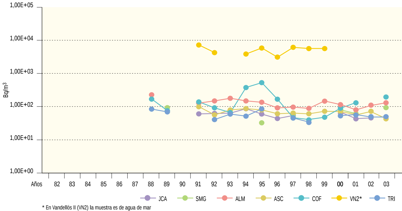
Figura 2.16b. Agua superficial. Concentración del índice de actividad beta resto (Bq/m³) Valores de la campaña de 2003
