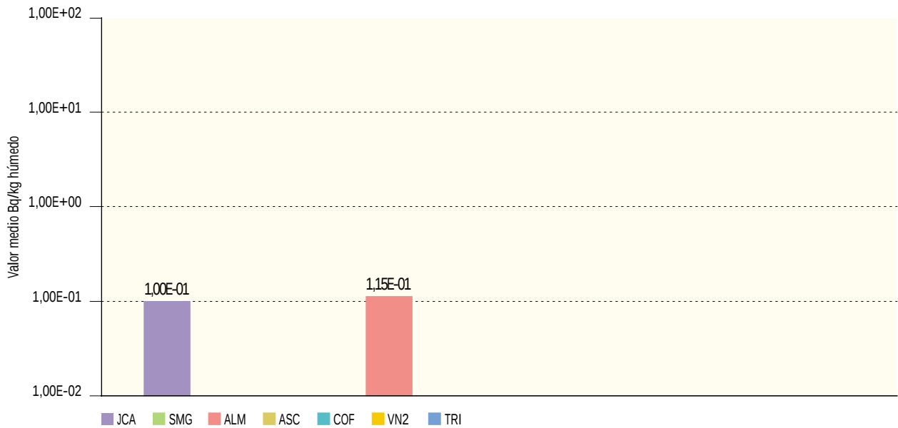
Figura 2.39b. Carne y aves. Concentración de actividad de Cs-137 (Bq/kg húmedo) Valores de la campaña de 2003
