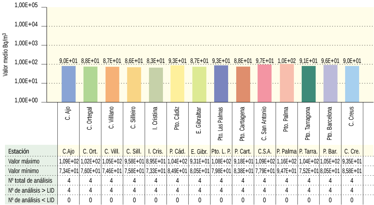
Figura 3.62b. Agua de mar. Concentración del índice de actividad alfa total (Bq/m³) Valores de la campaña de 2003
