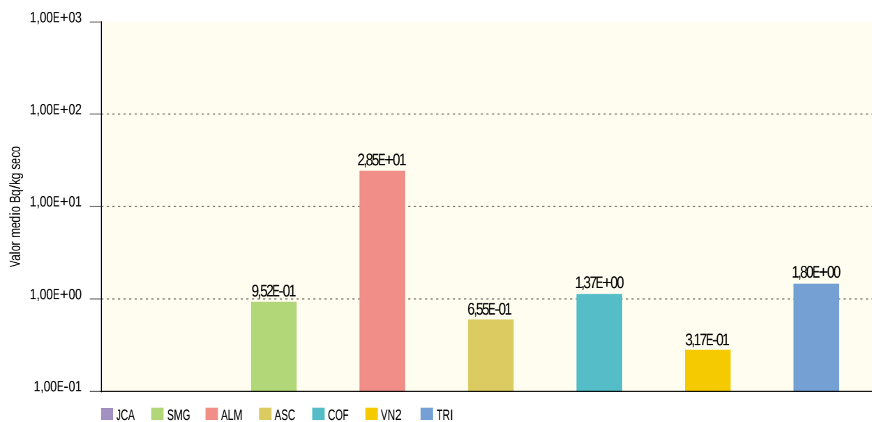
Figura 2.26b. Sedimentos de fondo. Concentración de actividad de Co-60 (Bq/kg seco)
