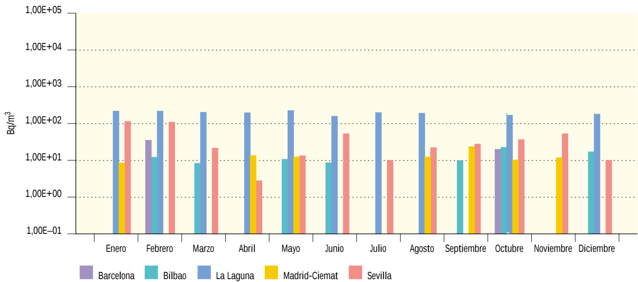
Figura 3.12. Agua potable. Concentración de actividad de beta resto (Bq/m³) Valores de la campaña de 2003
