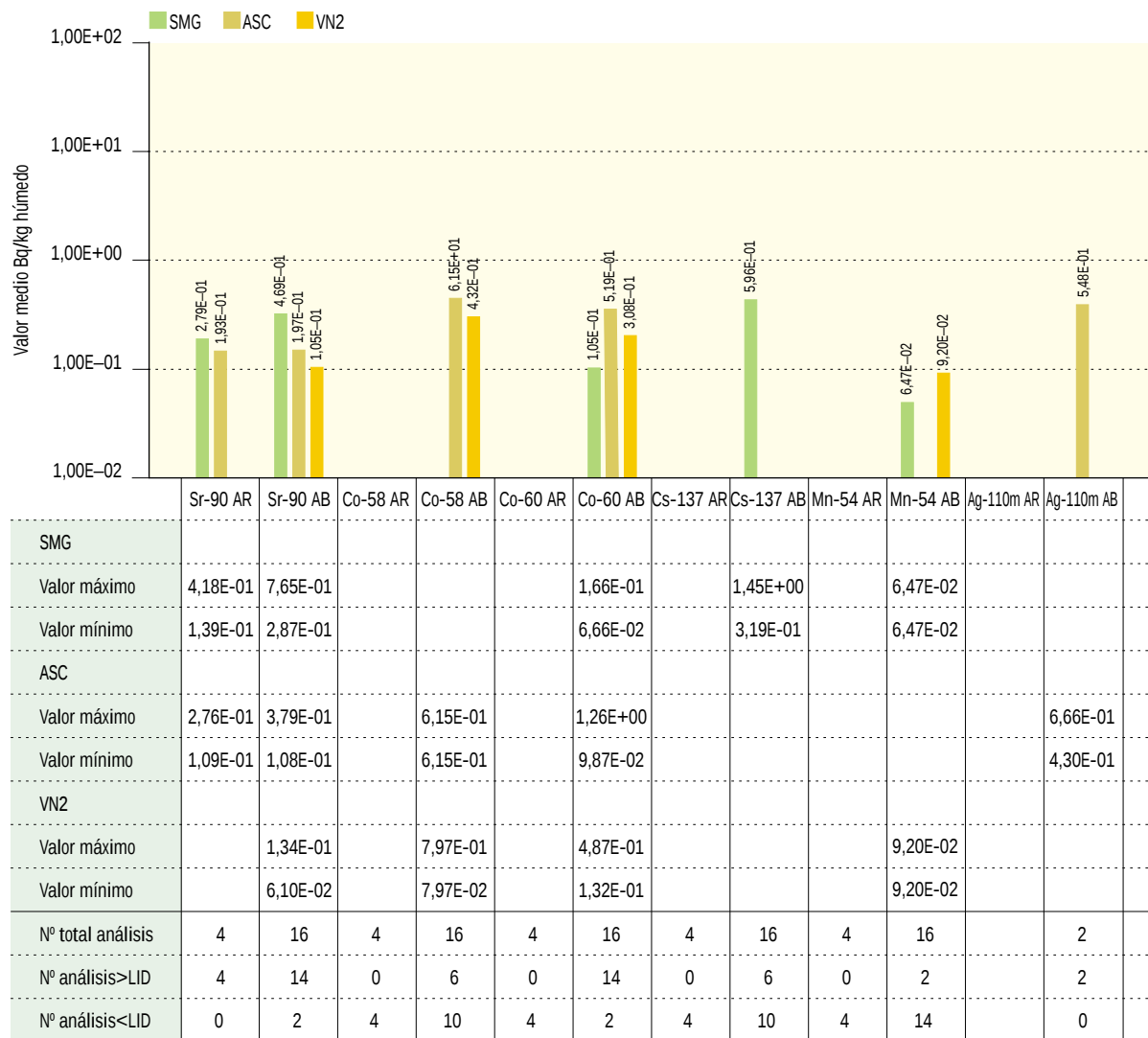
Figura 2.29b. Plantas acuáticas. Concentración de actividad (Bq/kg húmedo)
