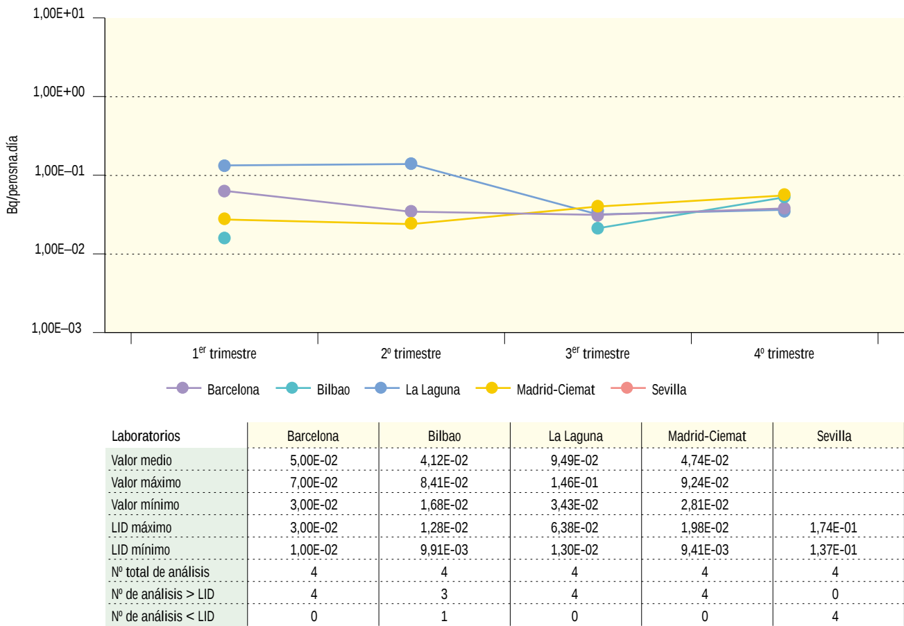
Figura 3.19. Dieta tipo. Concentración de actividad de Cs-137 (Bq/persona.día) Valores de la campaña de 2003
