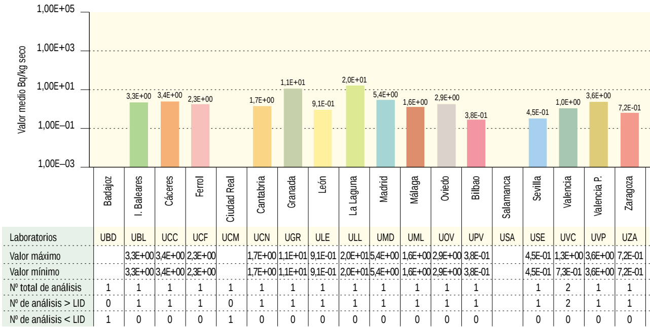
Figura 3.8b. Suelo. Concentración de actividad de Sr-90 (Bq/kg seco) Valores de la campaña de 2003
