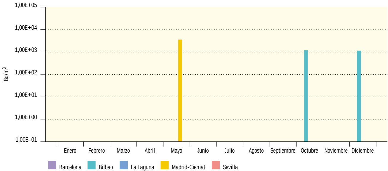
Figura 3.14. Agua potable. Concentración de actividad de H-3 (Bq/m³) Valores de la campaña de 2003
