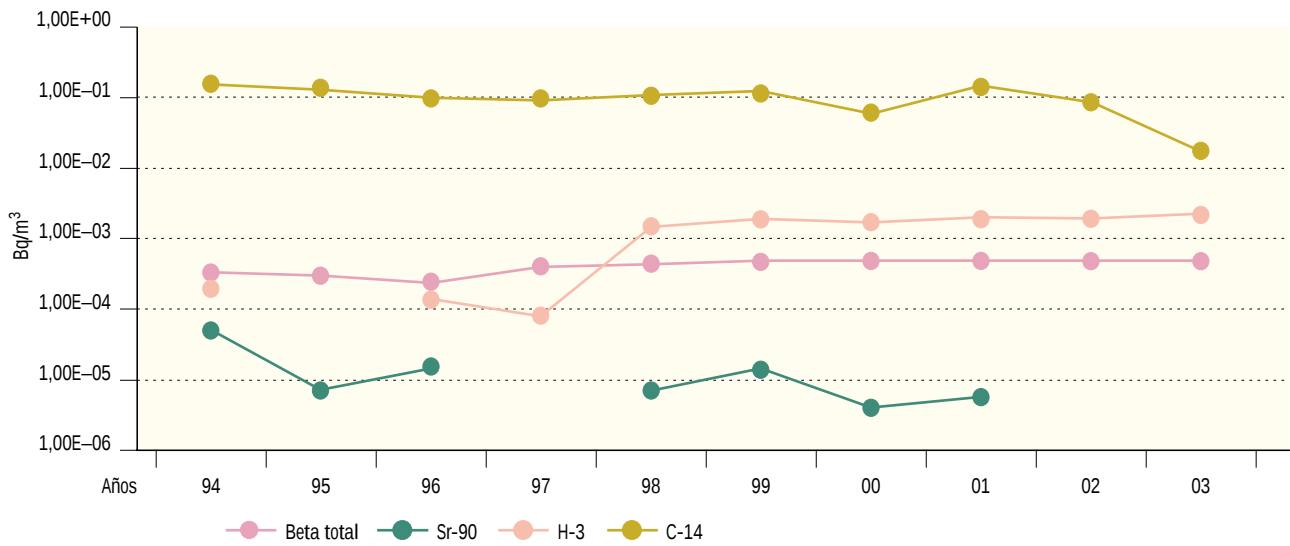
Figura 2.45. El Cabril. Aire. Valores de concentración de actividad (Bq/m³) Evolución temporal valores medios
