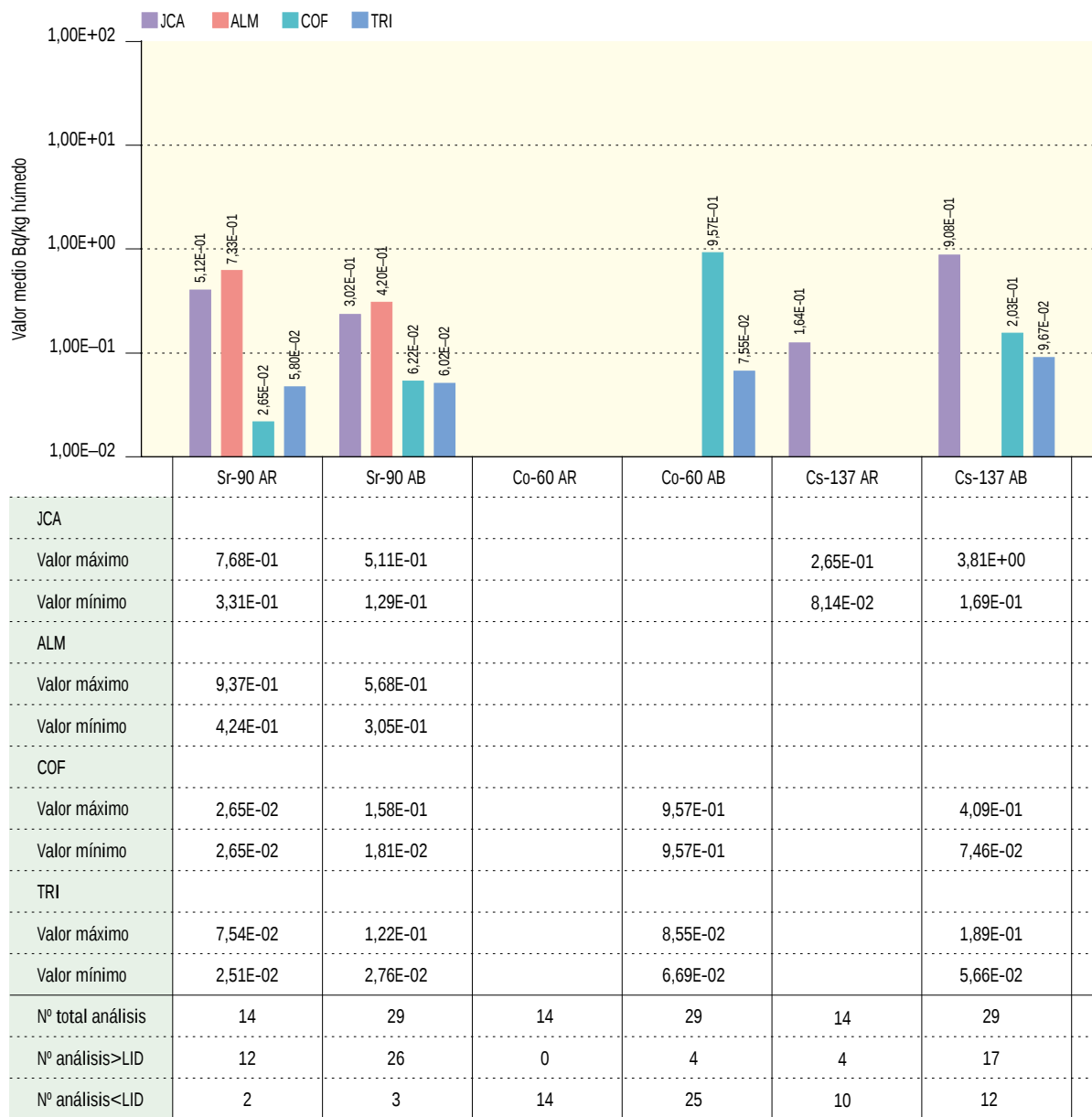
Figura 2.30b. Plantas de orilla. Concentración de actividad (Bq/kg húmedo)
