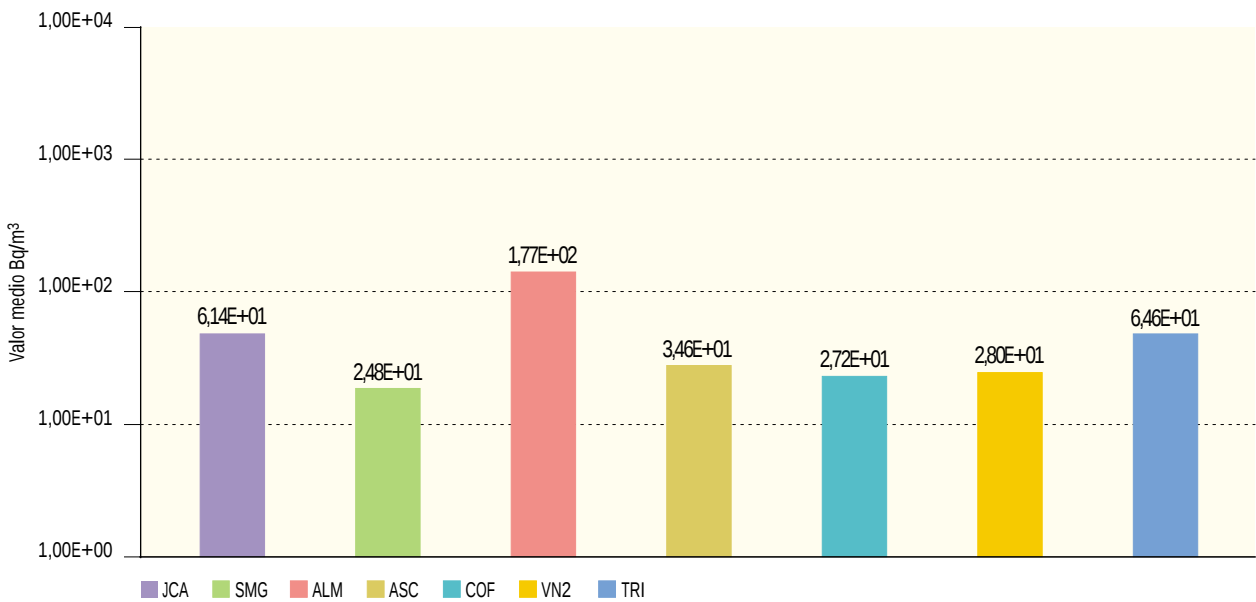
Figura 2.34b. Leche. Concentración de actividad de Sr-90 (Bq/m³) Valores de la campaña de 2003
