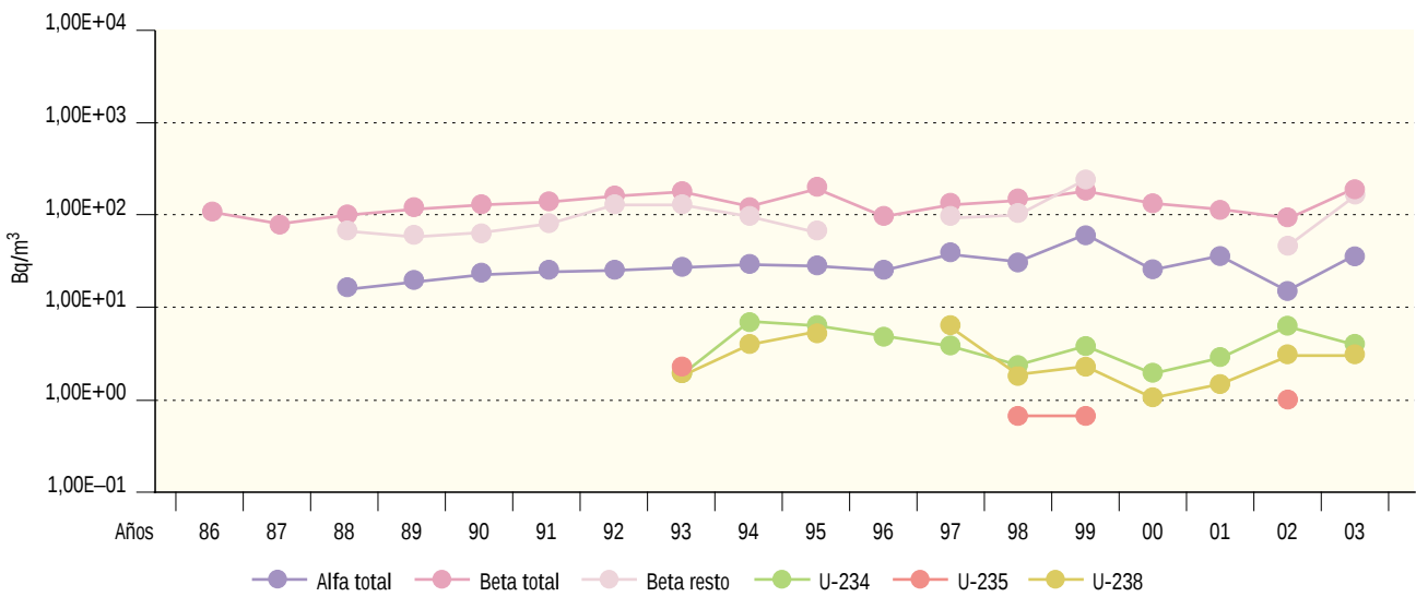
Figura 2.52. Juzbado. Agua potable. Valores de concentración de actividad (Bq/m³) Evolución temporal valores medios
