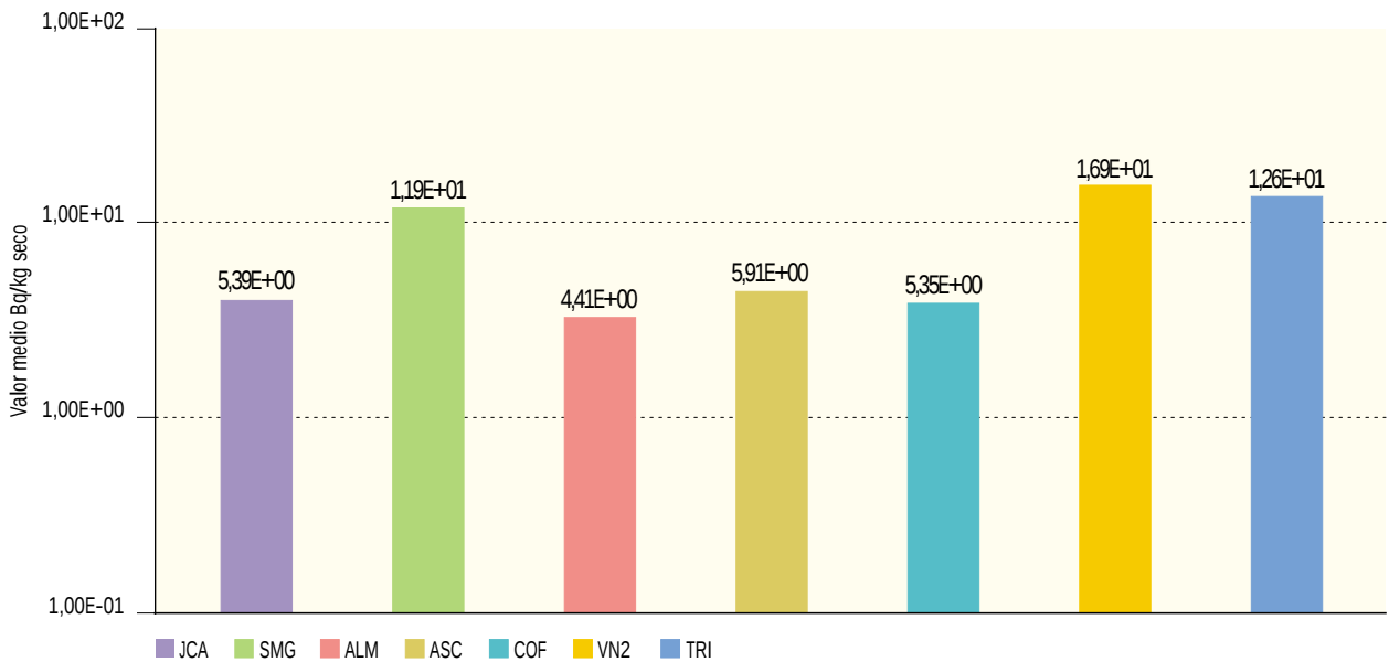
Figura 2.14b. Suelo. Concentración de actividad de Cs-137 (Bq/kg seco) Valores de la campaña de 2003
