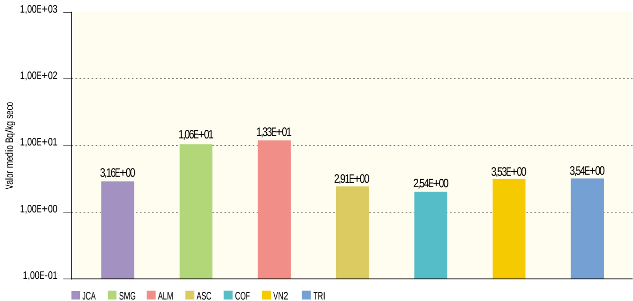
Figura 2.24b. Sedimentos de fondo. Concentración de actividad de Cs-137 (Bq/kg seco) Valores de la campaña de 2003
