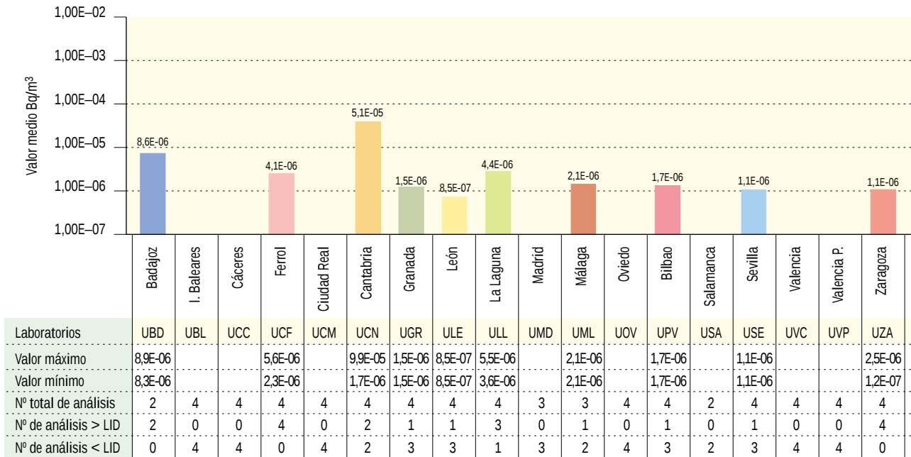
Figura 3.4b. Partículas de polvo en el aire. Concentración de actividad de Sr-90 (Bq/m³) Valores de la campaña de 2003
