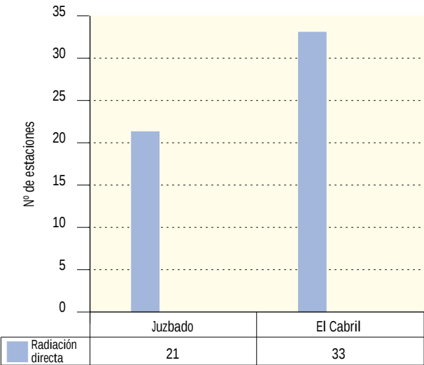
Figura 2.41. Número de estaciones de muestreo en los PVRA de las instalaciones del ciclo de combustible Aire y deposición húmeda y seca
