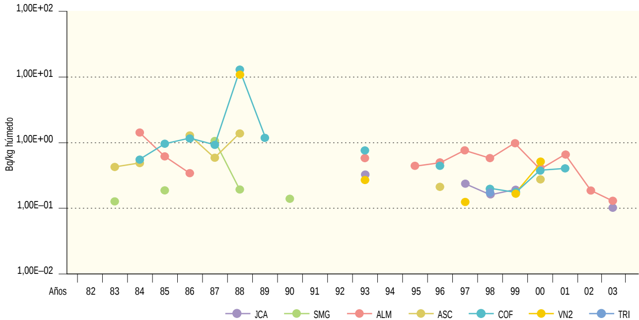
Figura 2.39b. Carne y aves. Concentración de actividad de Cs-137 (Bq/kg húmedo) Valores de la campaña de 2003
