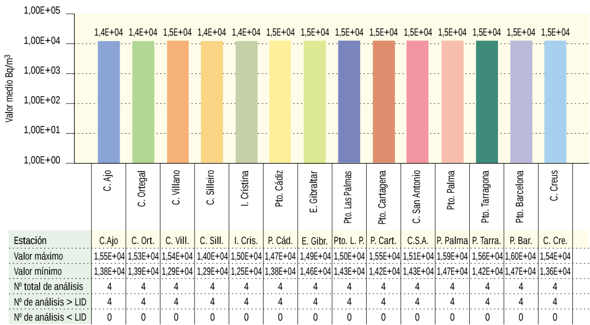
Figura 3.63b. Agua de mar. Concentración del índice de actividad beta total (Bq/m³) Valores de la campaña de 2003
