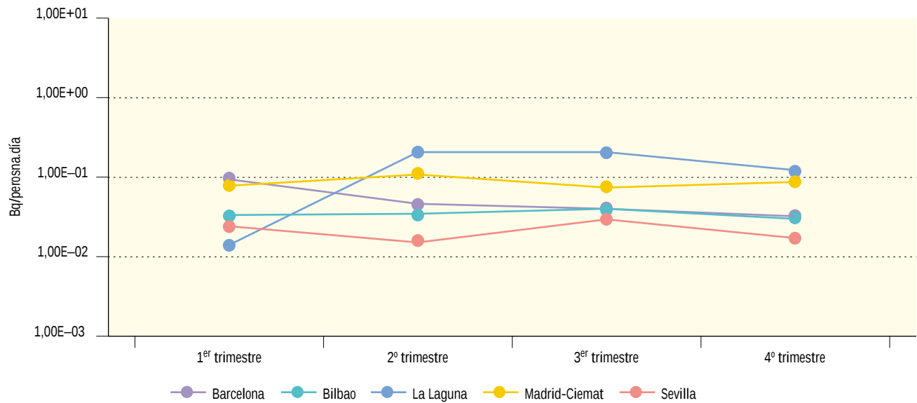
Figura 3.18. Dieta tipo. Concentración de actividad de Sr-90 (Bq/persona.día) Valores de la campaña de 2003
