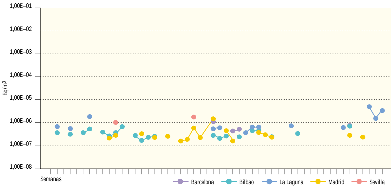
Figura 3.5. Partículas de polvo en el aire. Muestreador alto flujo Concentración de actividad de Cs-137 (Bq/m³). Valores de la campaña de 2003
