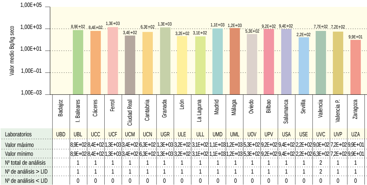
Figura 3.7b. Suelo. Concentración del índice de actividad beta total (Bq/kg seco) Valores de la campaña de 2003
