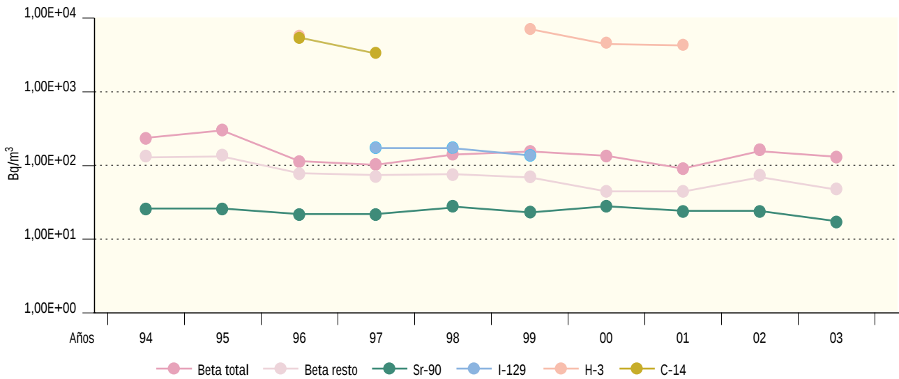
Figura 2.51. El Cabril. Agua superficial. Valores de concentración de actividad (Bq/m³) Evolución temporal valores medios
