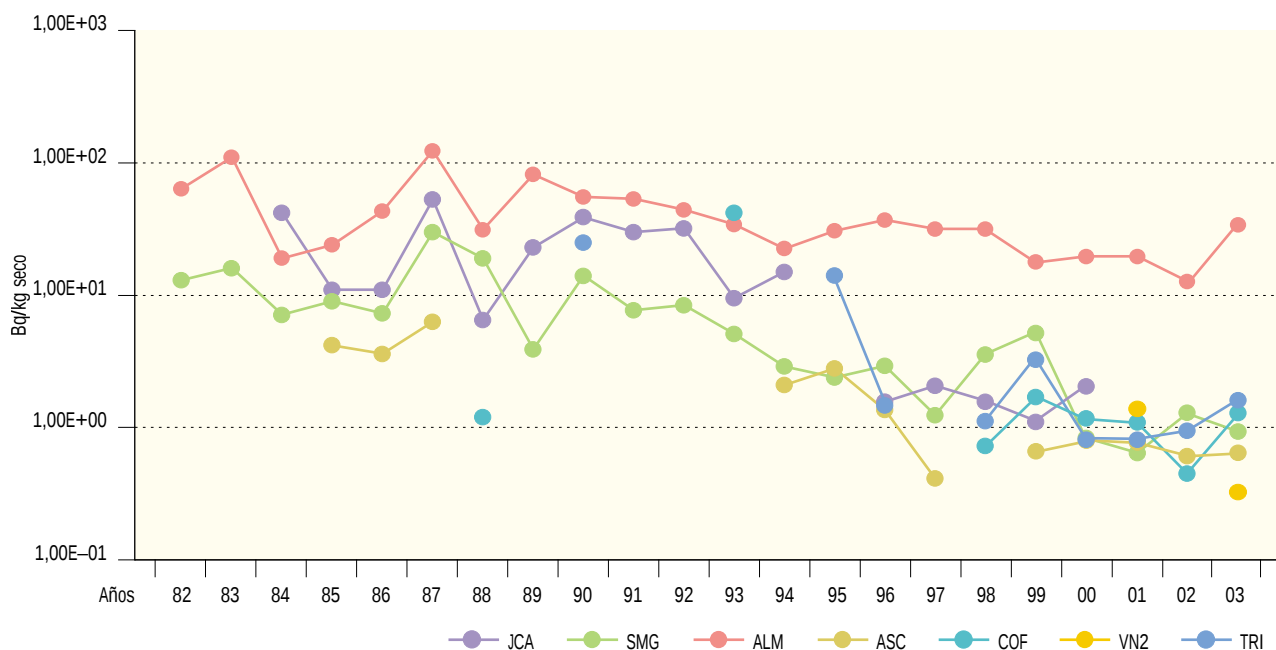
Figura 2.26b. Sedimentos de fondo. Concentración de actividad de Co-60 (Bq/kg seco)
