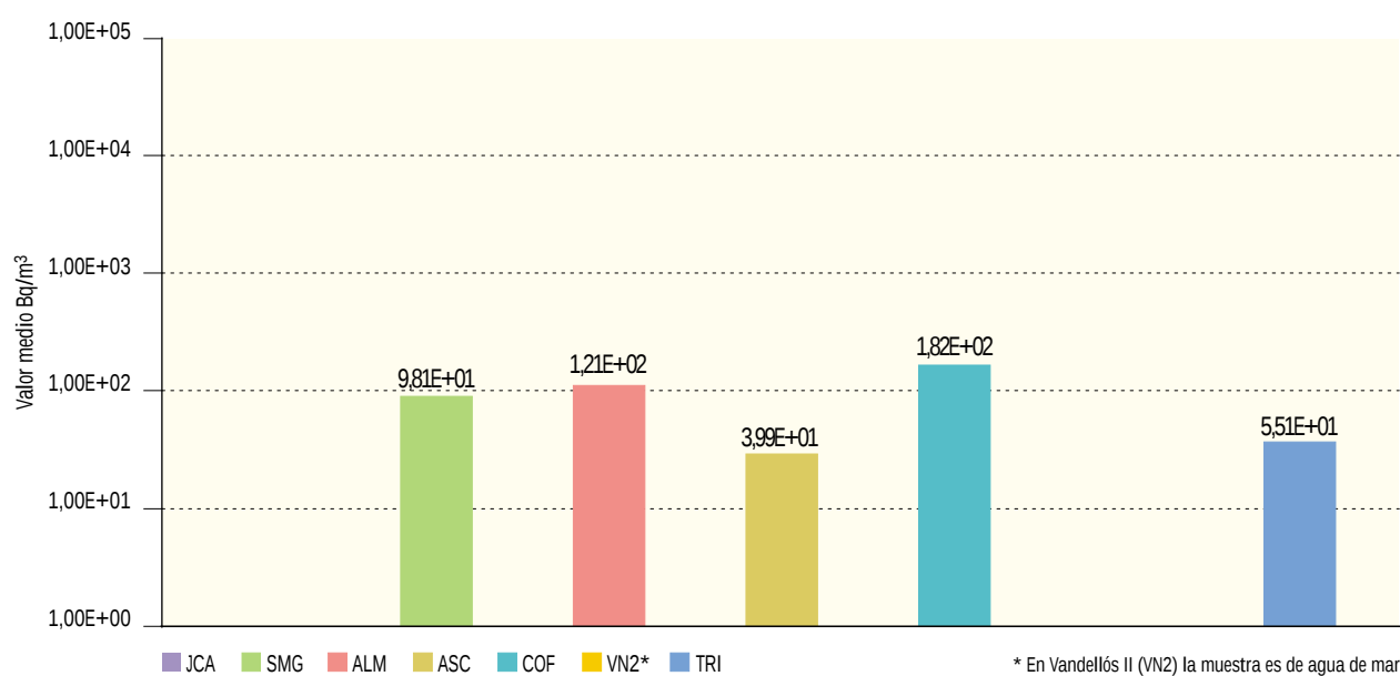
Figura 2.16b. Agua superficial. Concentración del índice de actividad beta resto (Bq/m³) Valores de la campaña de 2003
