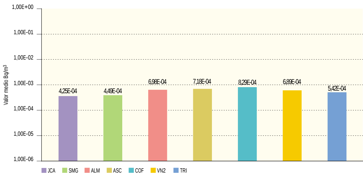
Figura 2.8b. Partículas de polvo en el aire. Concentración del índice de actividad beta total (Bq/m³) Valores de la campaña de 2003
