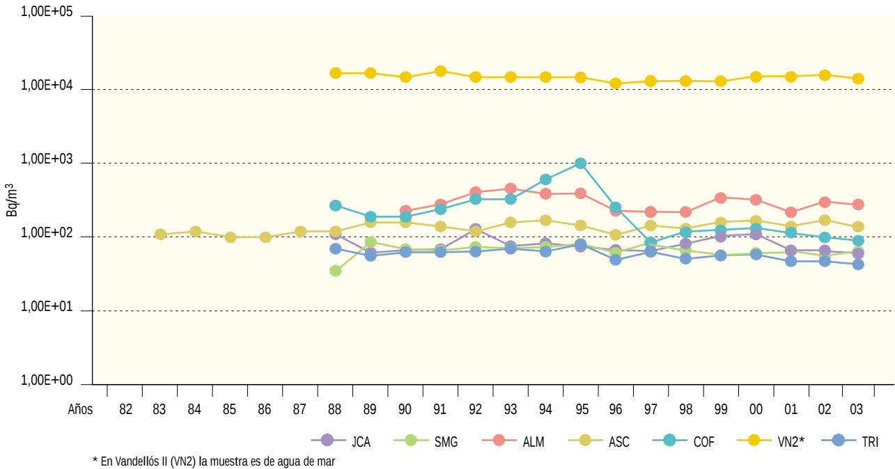
Figura 2.15b. Agua superficial. Concentración del índice de actividad beta total (Bq/m³) Valores de la campaña de 2003
