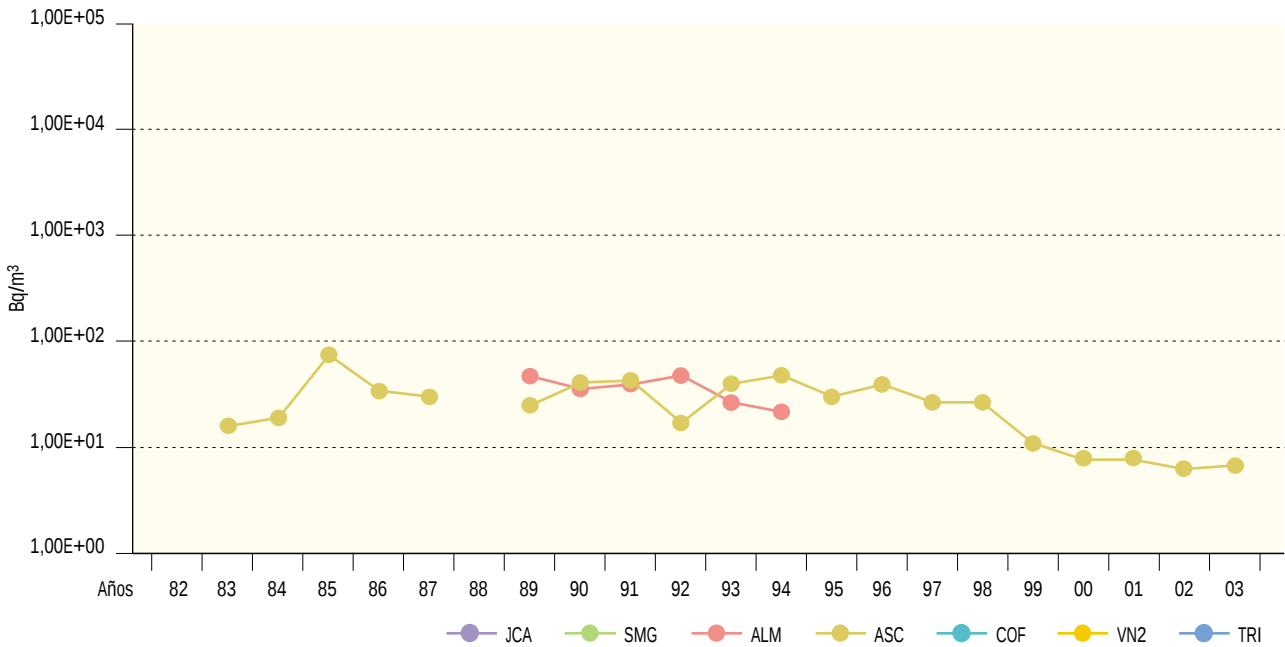
Figura 2.17b. Agua superficial. Concentración de actividad de Sr-90 (Bq/m³) Valores de la campaña de 2003
