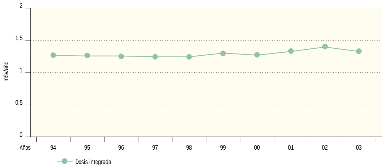
Figura 2.47. El Cabril. Radiación directa. Dosis integrada (DTL) (mSv/año) Valores medios en la zona vigilada
