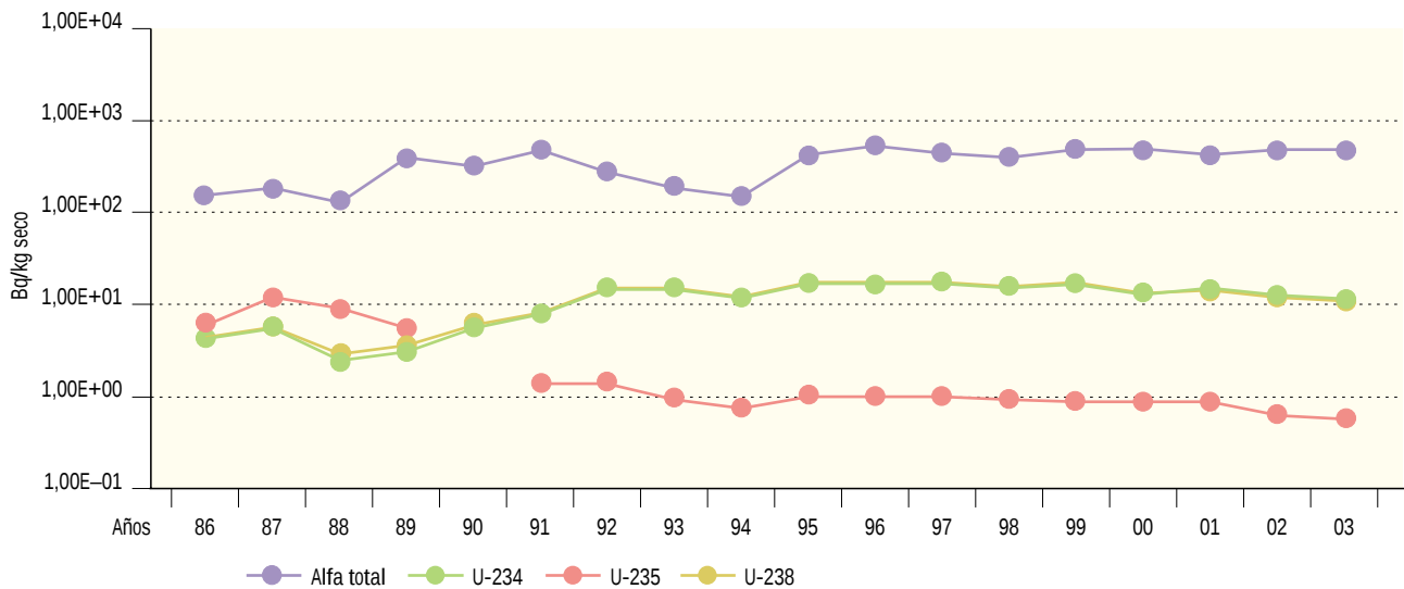
Figura 2.48. Juzbado. Suelo. Valores de concentración de actividad (Bq/kg seco)
