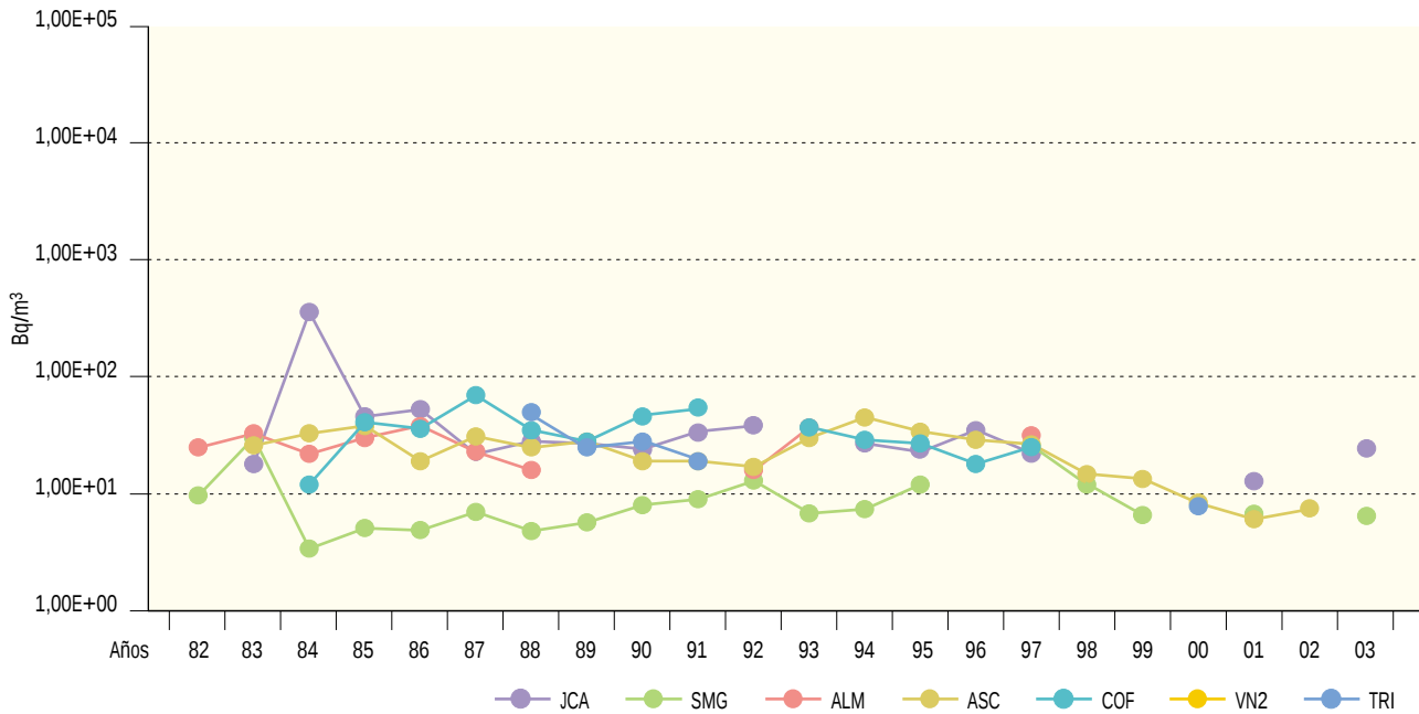
Figura 2.21b. Agua potable. Concentración de actividad de Sr-90 (Bq/m³) Valores de la campaña de 2003
