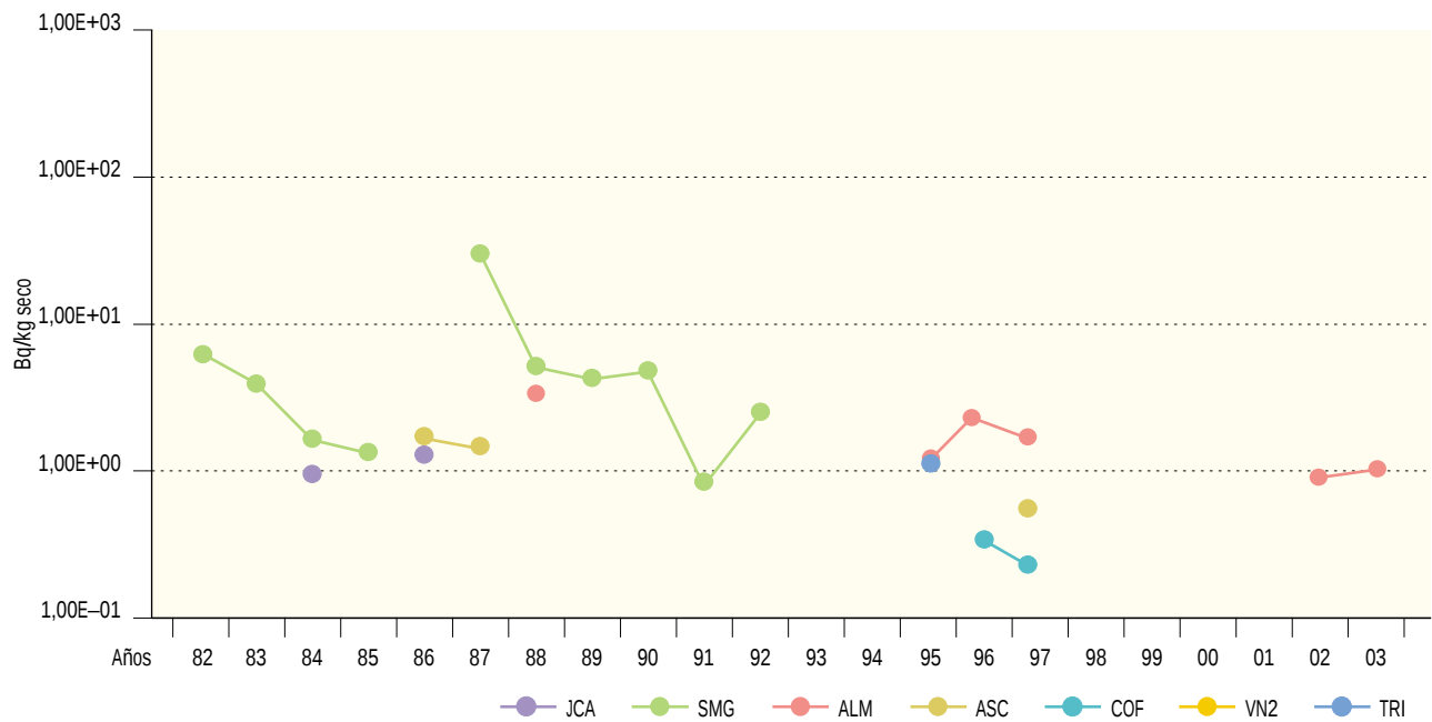
Figura 2.28b. Sedimentos de fondo. Concentración de actividad de Mn-54 (Bq/kg seco) Valores de la campaña de 2003
