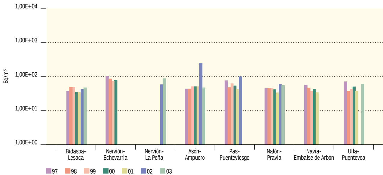
Figura 3.23. Cuencas del norte de España Evolución temporal del índice de actividad beta resto
