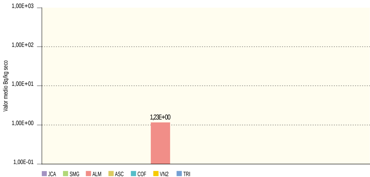
Figura 2.28b. Sedimentos de fondo. Concentración de actividad de Mn-54 (Bq/kg seco) Valores de la campaña de 2003
