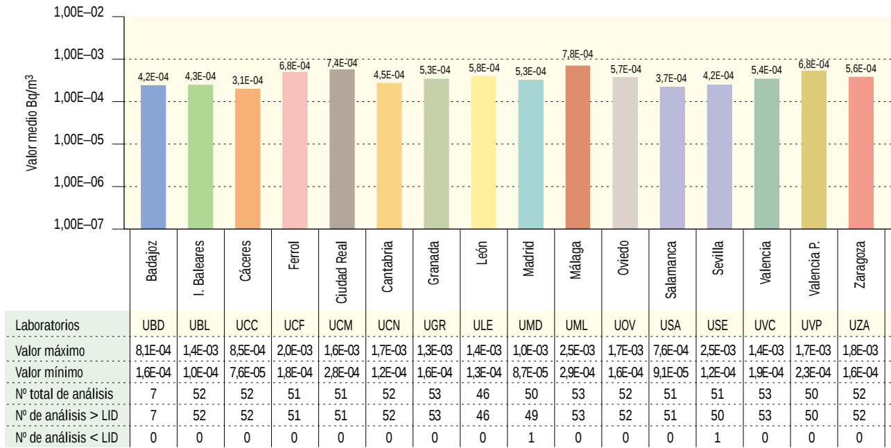
Figura 3.3b. Partículas de polvo en el aire. Concentración del índice de actividad beta total (Bq/m³) Valores de la campaña de 2003
