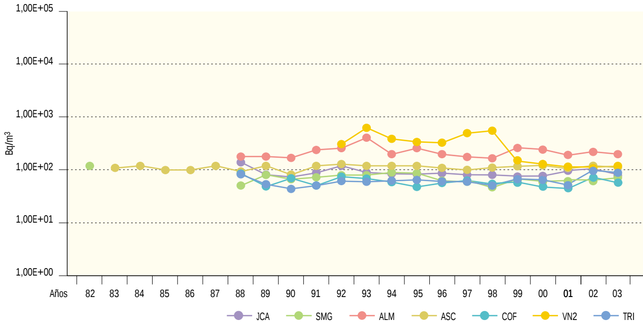
Figura 2.19b. Agua potable. Concentración del índice de actividad beta total (Bq/m³) Valores de la campaña de 2003
