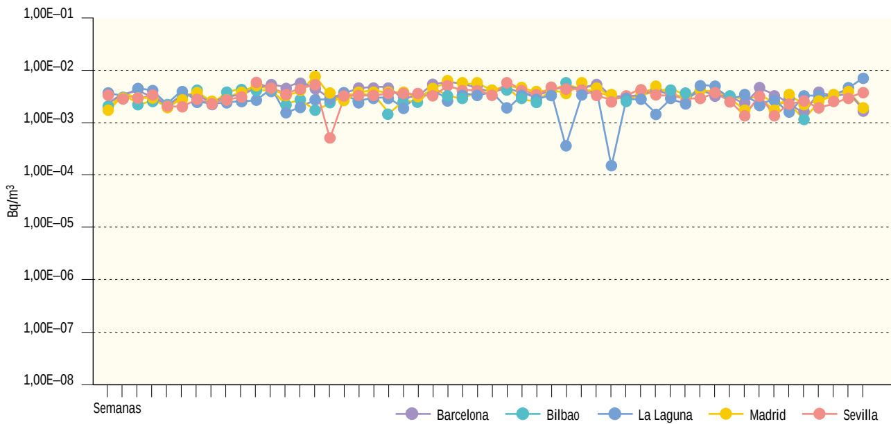
Figura 3.6. Partículas de polvo en el aire. Muestreador alto flujo Concentración de actividad de Be-7 (Bq/m³). Valores de la campaña de 2003
