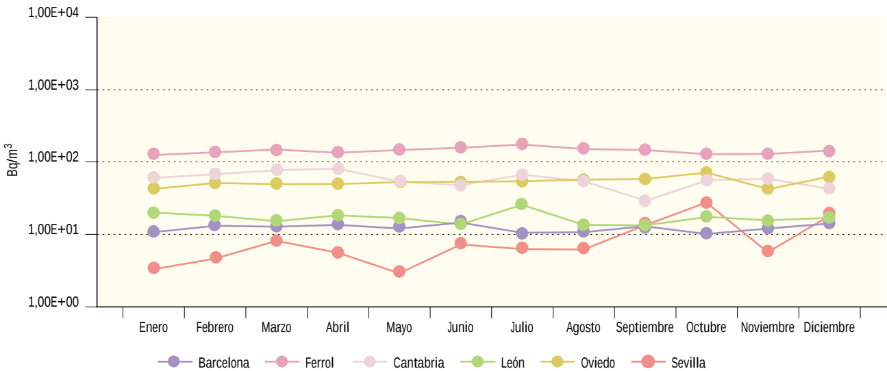
Figura 3.16. Leche. Concentración de actividad de Sr-90 (Bq/m³) Valores de la campaña de 2003
