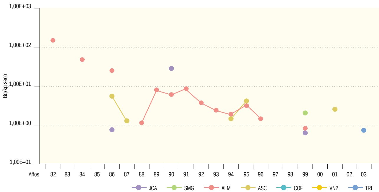
Figura 2.27b. Sedimentos de fondo. Concentración de actividad de Co-58 (Bq/kg seco) Valores de la campaña de 2003
