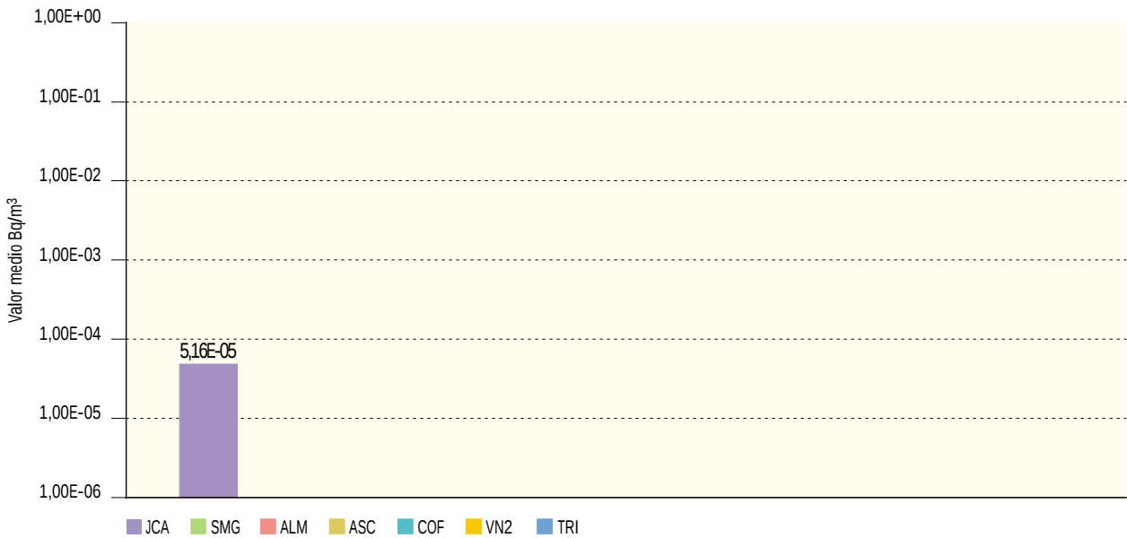
Figura 2.10b. Partículas de polvo en el aire. Concentración de actividad de Cs-137 (Bq/m³) Valores de la campaña de 2003
