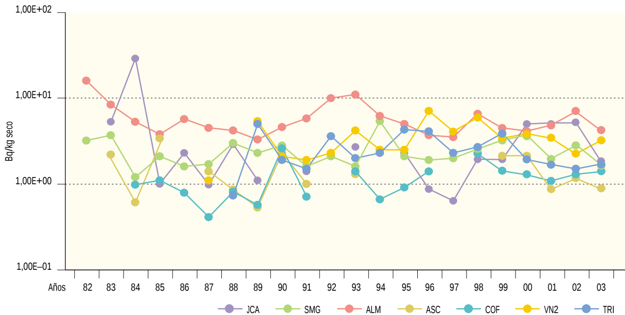
Figura 2.13b. Suelo. Concentración de actividad de Sr-90 (Bq/kg seco) Valores de la campaña de 2003
