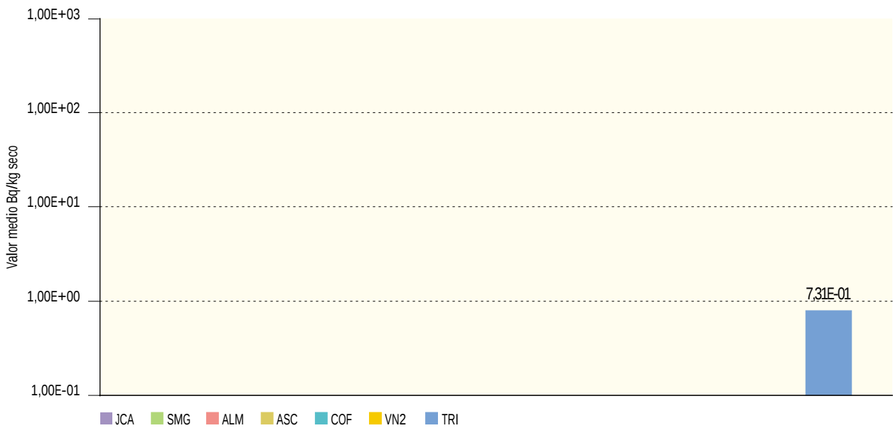
Figura 2.27b. Sedimentos de fondo. Concentración de actividad de Co-58 (Bq/kg seco) Valores de la campaña de 2003
