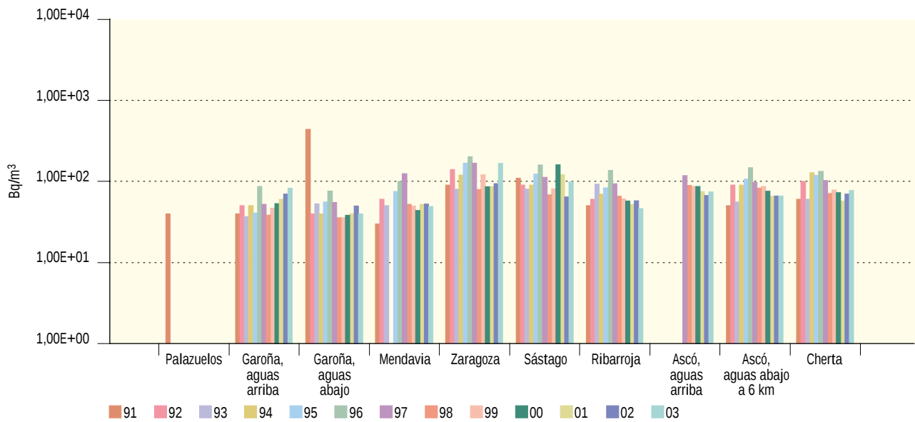
Figura 3.55. Río Ebro Evolución temporal del índice de actividad beta resto
