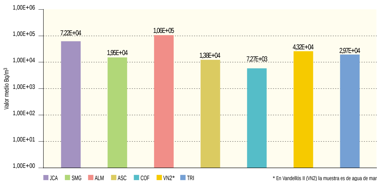
Figura 2.18b. Agua superficial. Concentración de actividad de H-3 (Bq/m³)
