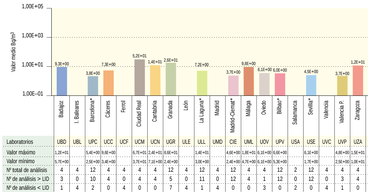
Figura 3.13b. Agua potable. Concentración de actividad de Sr-90 (Bq/m³) Valores de la campaña de 2003
