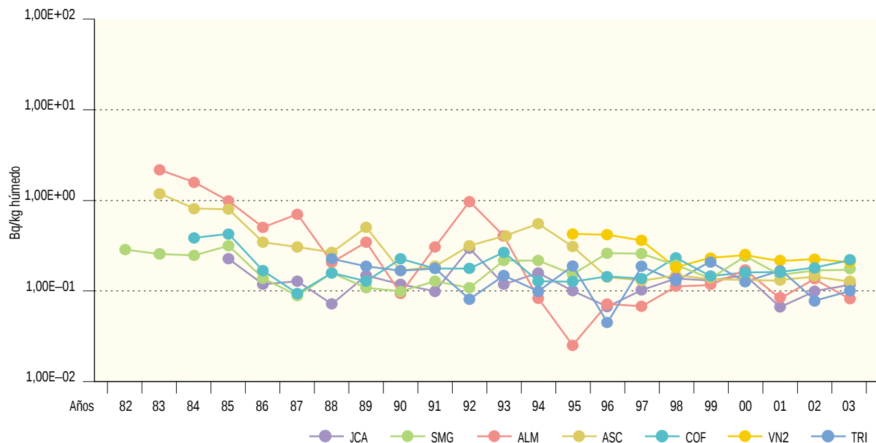
Figura 2.37b. Vegetales de hoja no ancha. Concentración de actividad de Sr-90 (Bq/kg húmedo)
