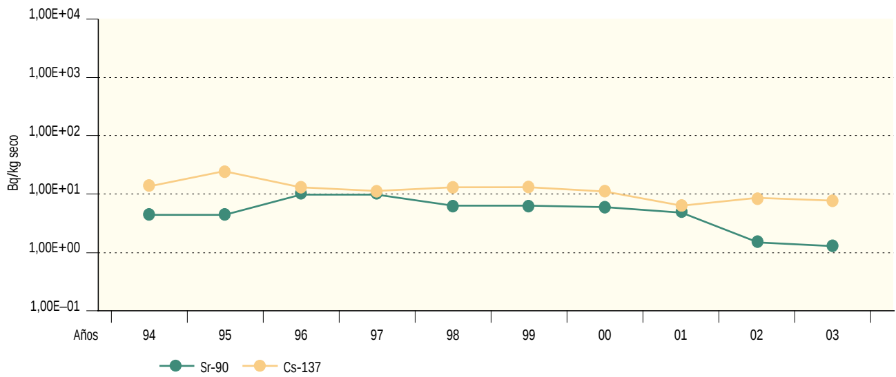
Figura 2.49. El Cabril. Suelo. Valores de concentración de actividad (Bq/kg seco) Evolución temporal valores medios
