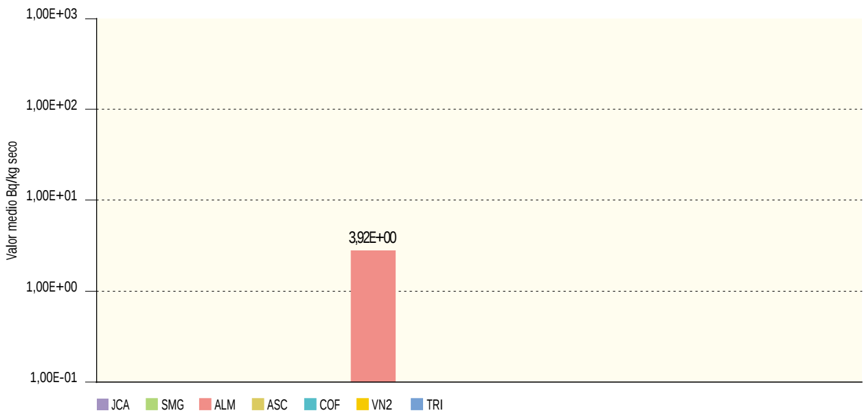
Figura 2.25b. Sedimentos de fondo. Concentración de actividad de Cs-134 (Bq/kg seco) Valores de la campaña de 2003
