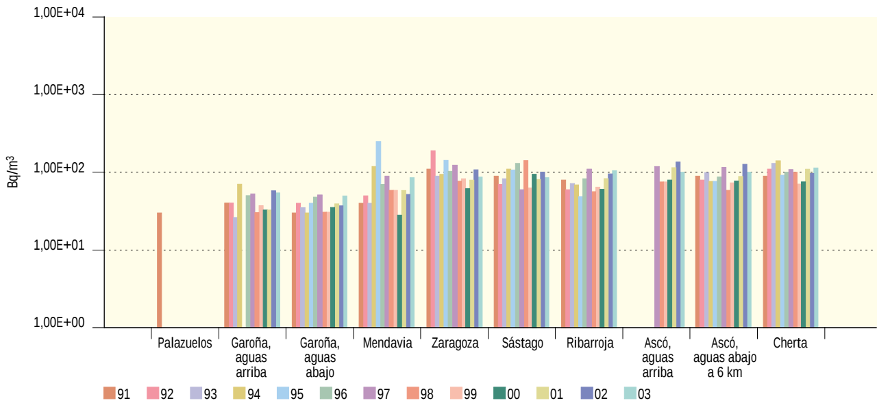
Figura 3.53. Río Ebro Evolución temporal del índice de actividad alfa total
