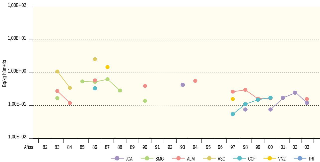
Figura 2.38b. Vegetales de hoja no ancha. Concentración de actividad de Cs-137 (Bq/kg húmedo) Valores de la campaña de 2003
