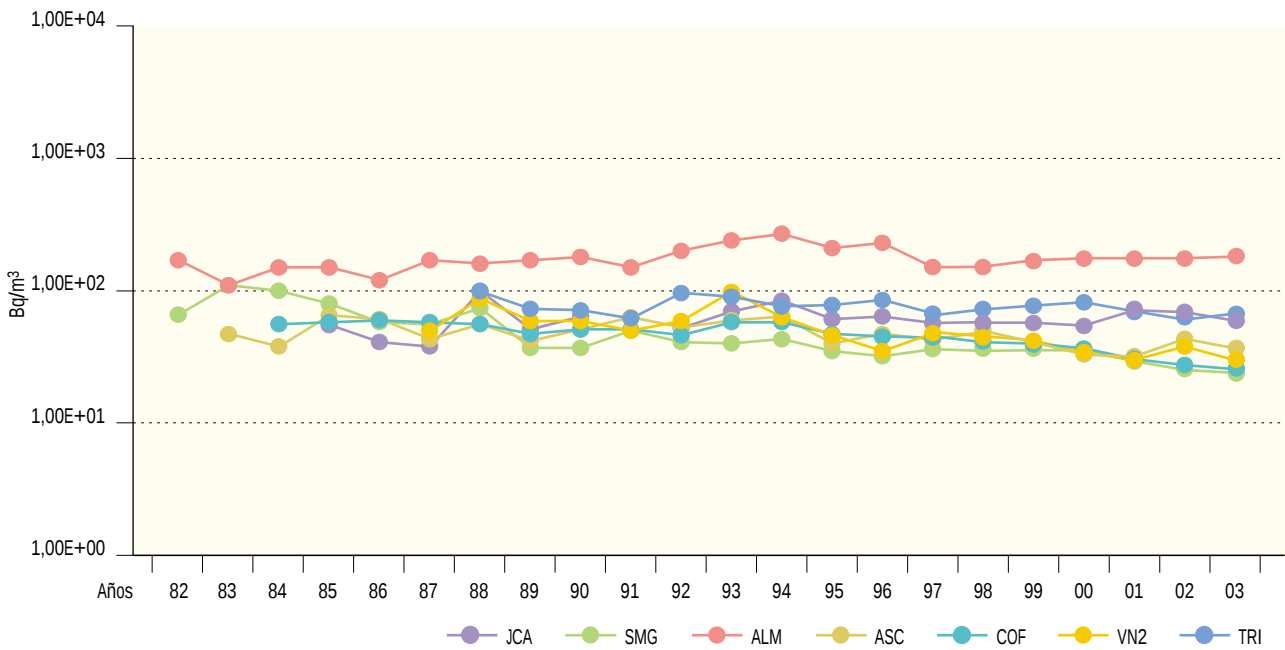
Figura 2.34b. Leche. Concentración de actividad de Sr-90 (Bq/m³) Valores de la campaña de 2003
