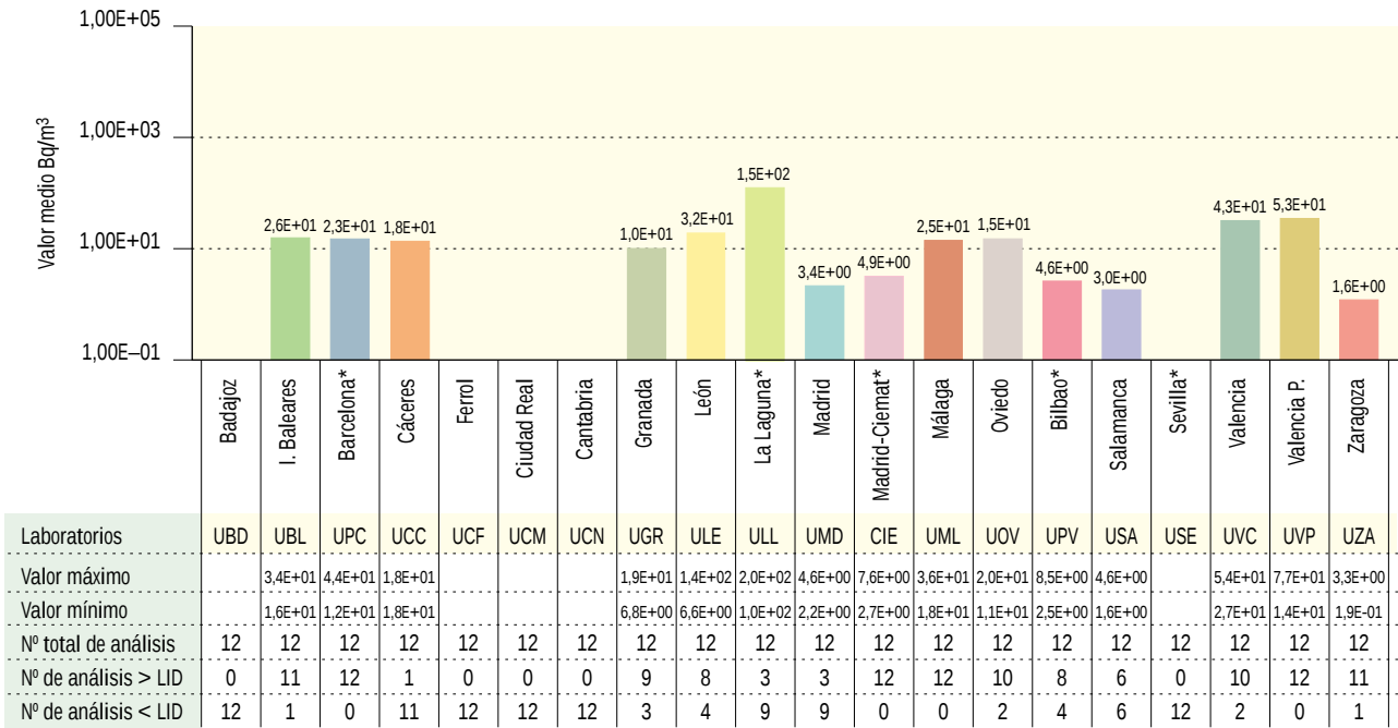
Figura 3.10b. Agua potable. Concentración de actividad de alfa total (Bq/m³) Valores de la campaña de 2003
