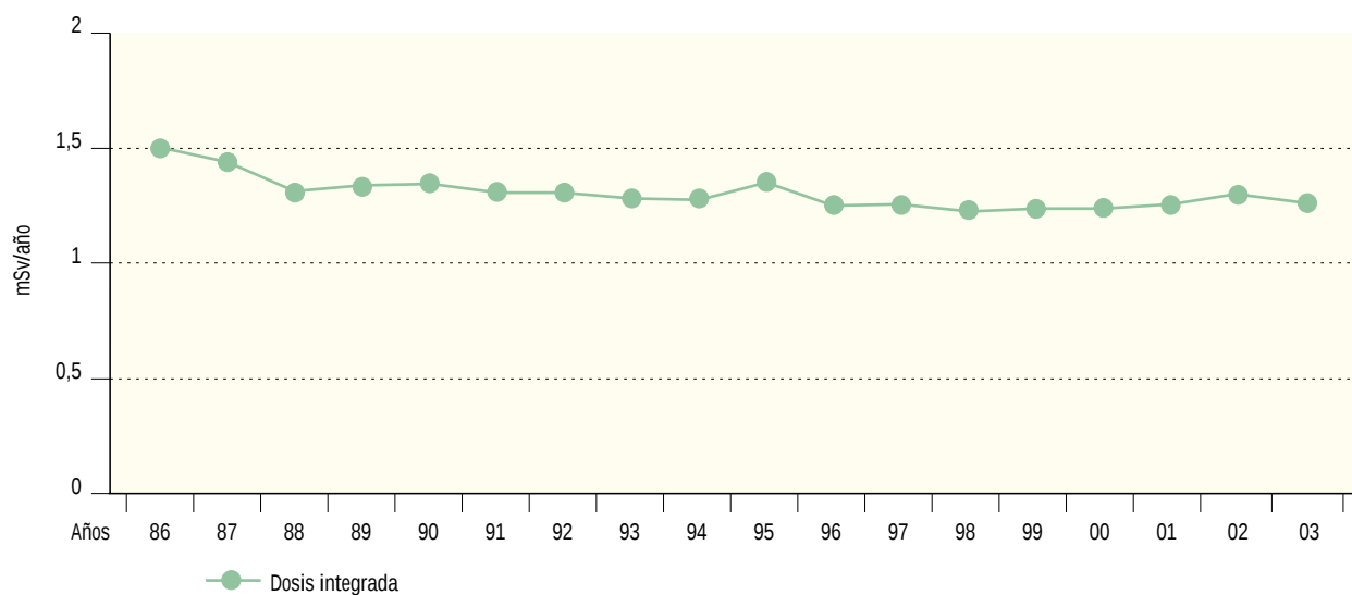
Figura 2.46. Juzbado. Radiación directa. Dosis integrada (DTL) (mSv/año)
