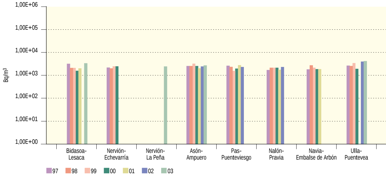
Figura 3.24. Cuencas del norte de España Evolución temporal de la concentración de actividad de H-3
