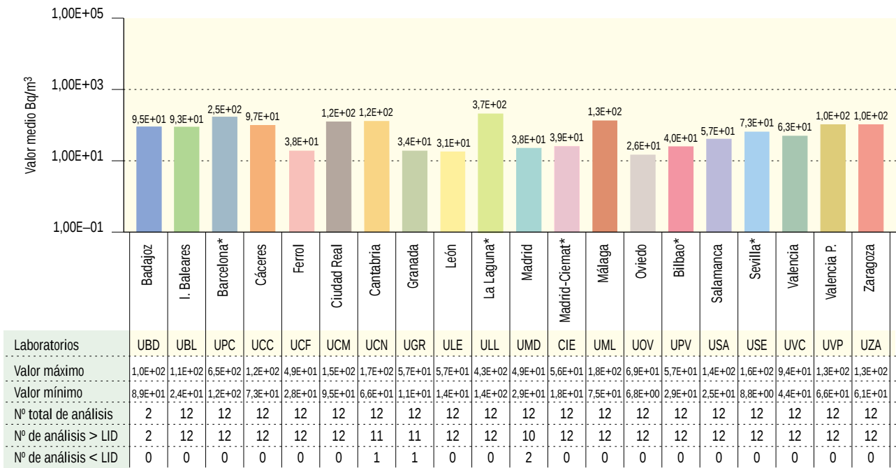
Figura 3.11b. Agua potable. Concentración de actividad de beta total (Bq/m³) Valores de la campaña de 2003
