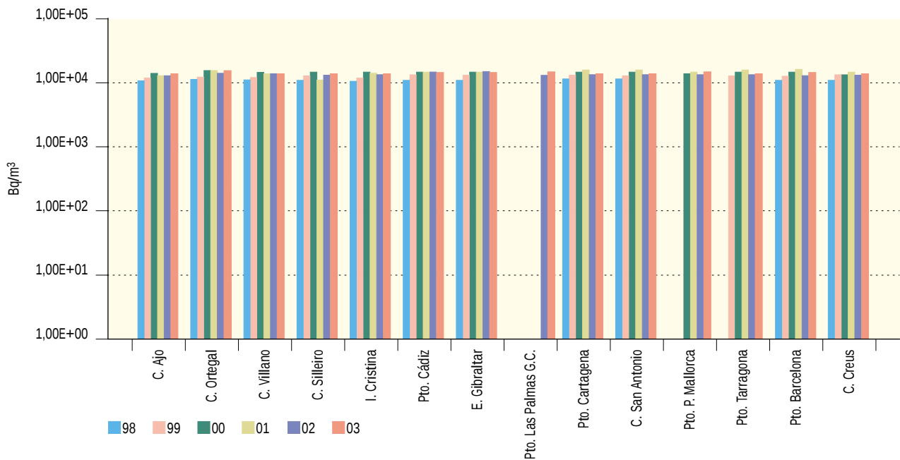
Figura 3.63a. Agua de mar Evolución temporal del índice de actividad beta total
