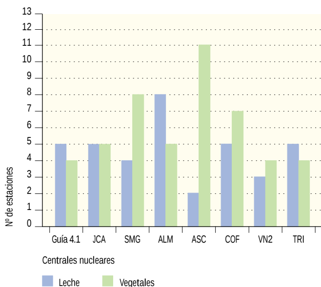
Figura 2.7. Número de estaciones de muestreo en los PVRA de las centrales nucleares. Año 2003.
