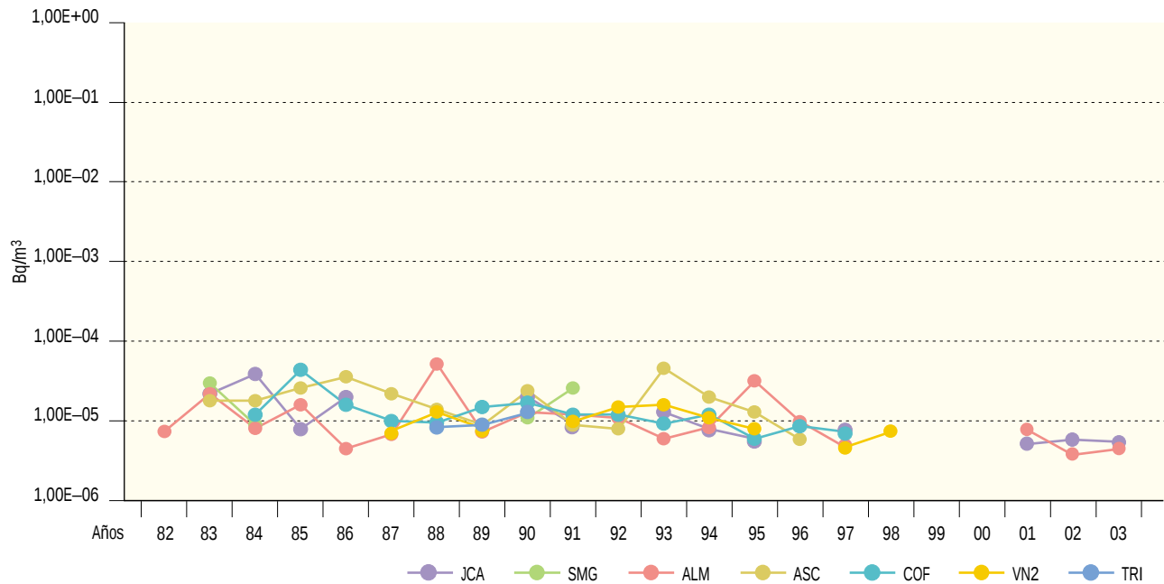
Figura 2.9b. Partículas de polvo en el aire. Concentración de actividad de Sr-90 (Bq/m³) Valores de la campaña de 2003
