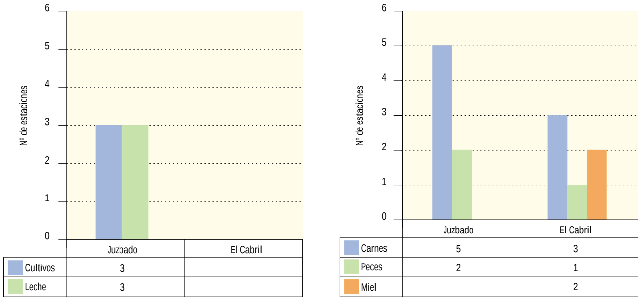
Figura 2.43. Número de estaciones de muestreo en los PVRA de las instalaciones del ciclo de combustible
