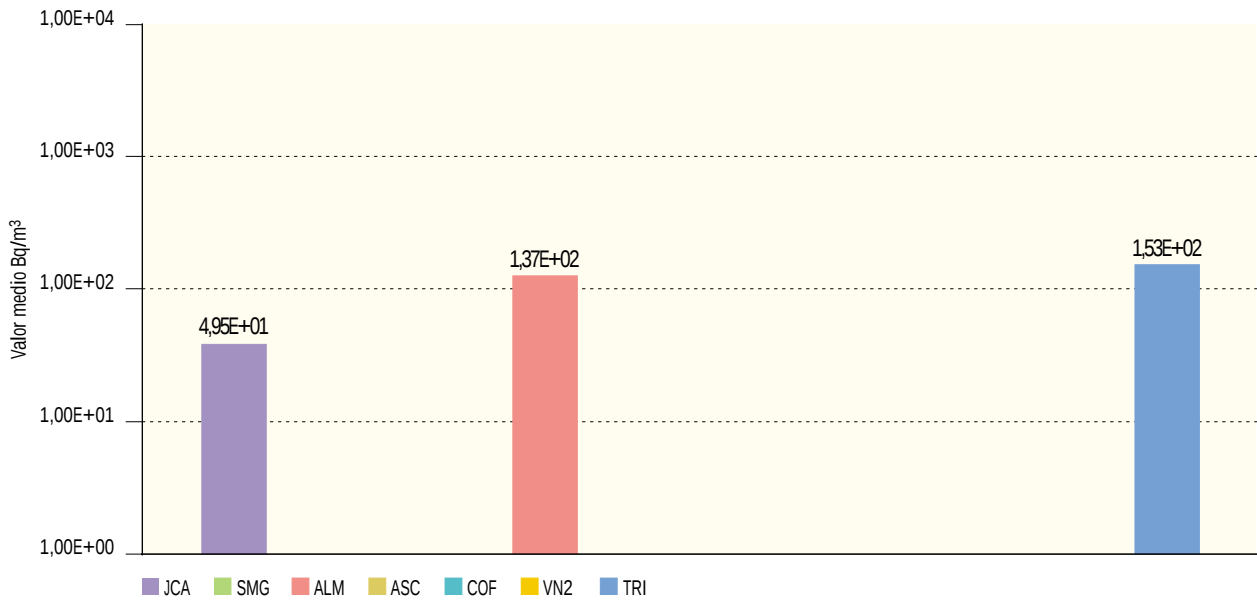
Figura 2.35b. Leche. Concentración de actividad de Cs-137 (Bq/m³) Valores de la campaña de 2003
