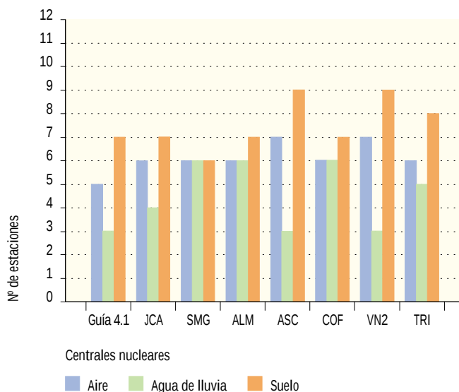
Figura 2.3. Número de estaciones de muestreo en los PVRA de las centrales nucleares. Año 2003.
