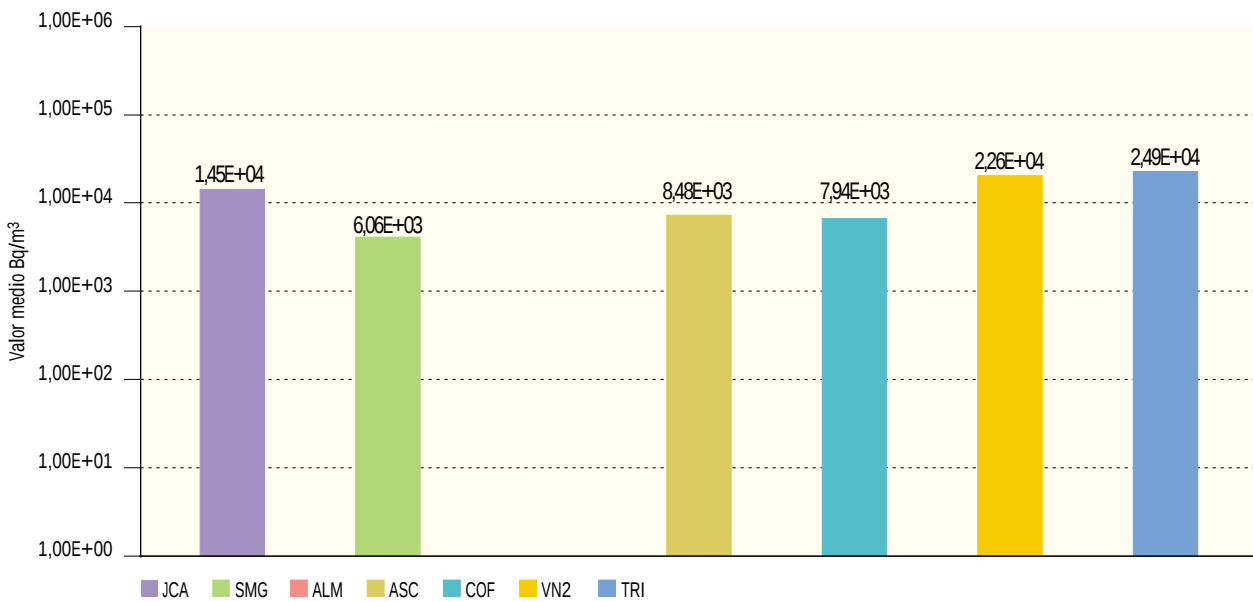
Figura 2.22b. Agua potable. Concentración de actividad de H-3 (Bq/m³) Valores de la campaña de 2003
