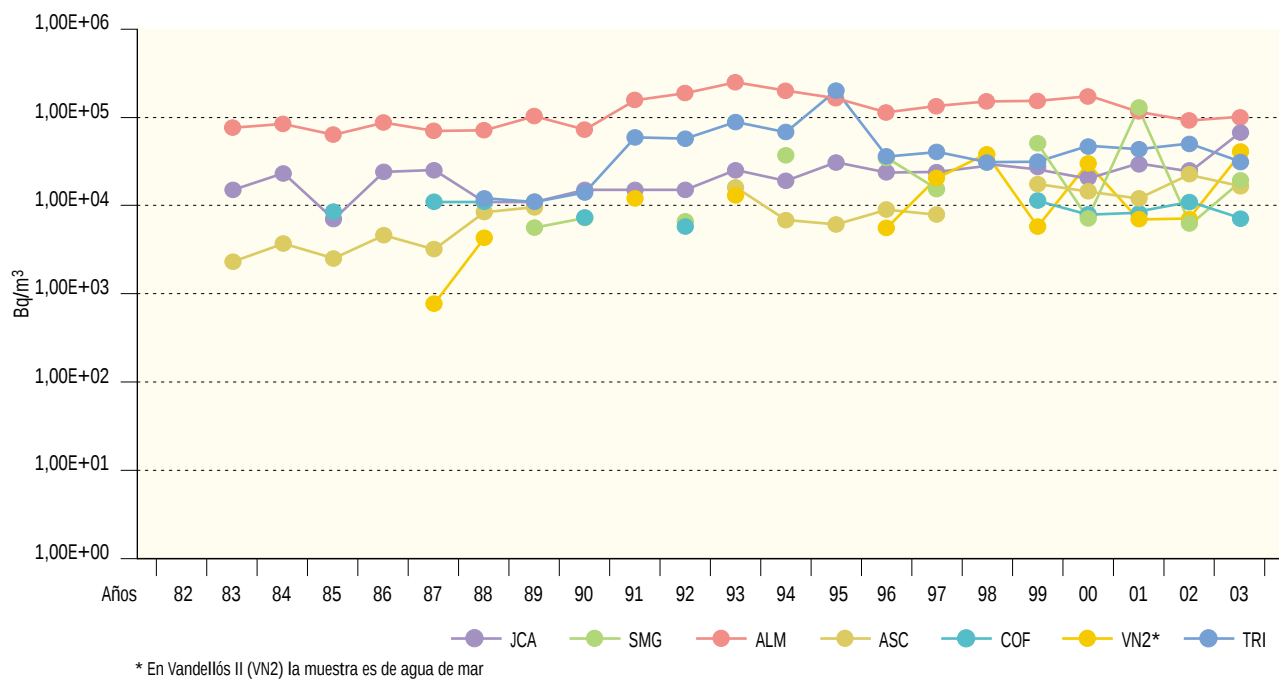
Figura 2.18b. Agua superficial. Concentración de actividad de H-3 (Bq/m³)
