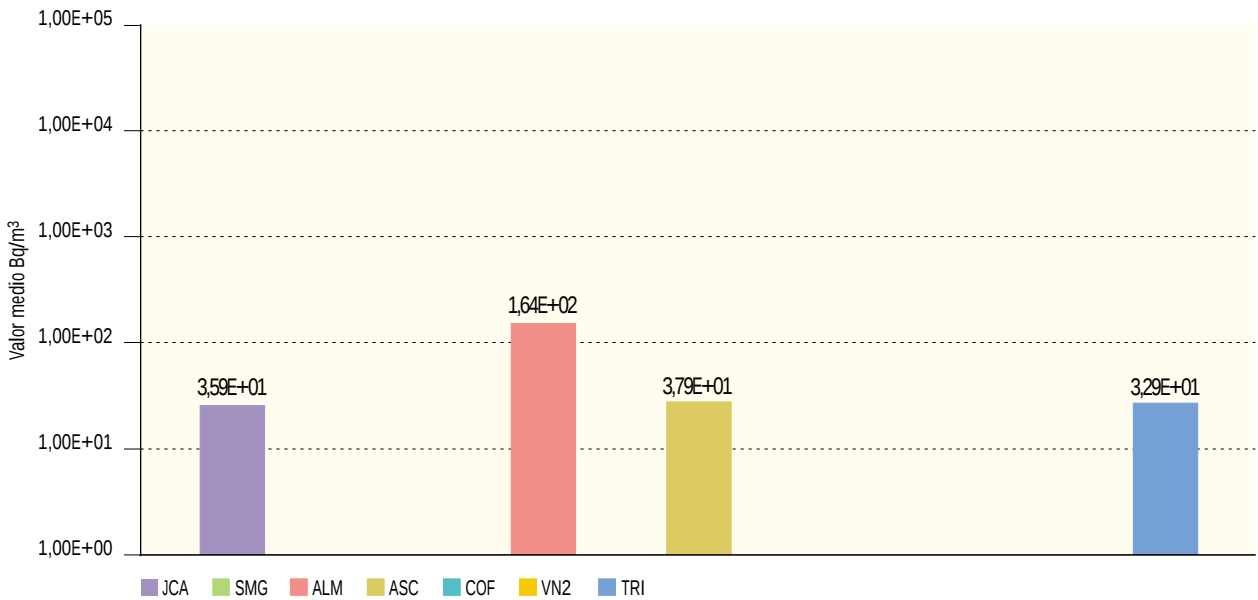
Figura 2.20b. Agua potable. Concentración del índice de actividad beta resto (Bq/m³) Valores de la campaña de 2003
