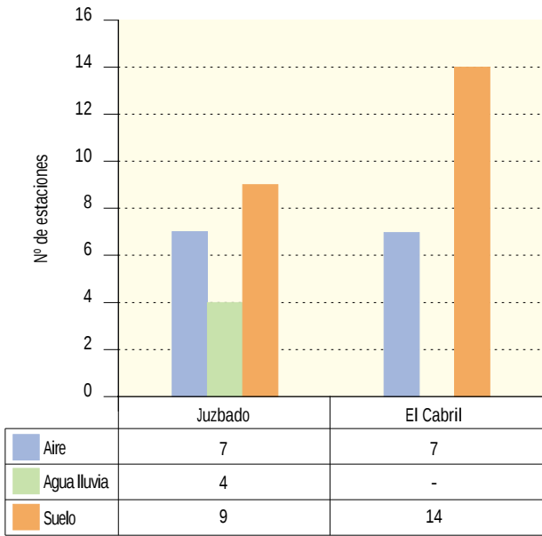
Figura 2.41. Número de estaciones de muestreo en los PVRA de las instalaciones del ciclo de combustible Aire y deposición húmeda y seca
