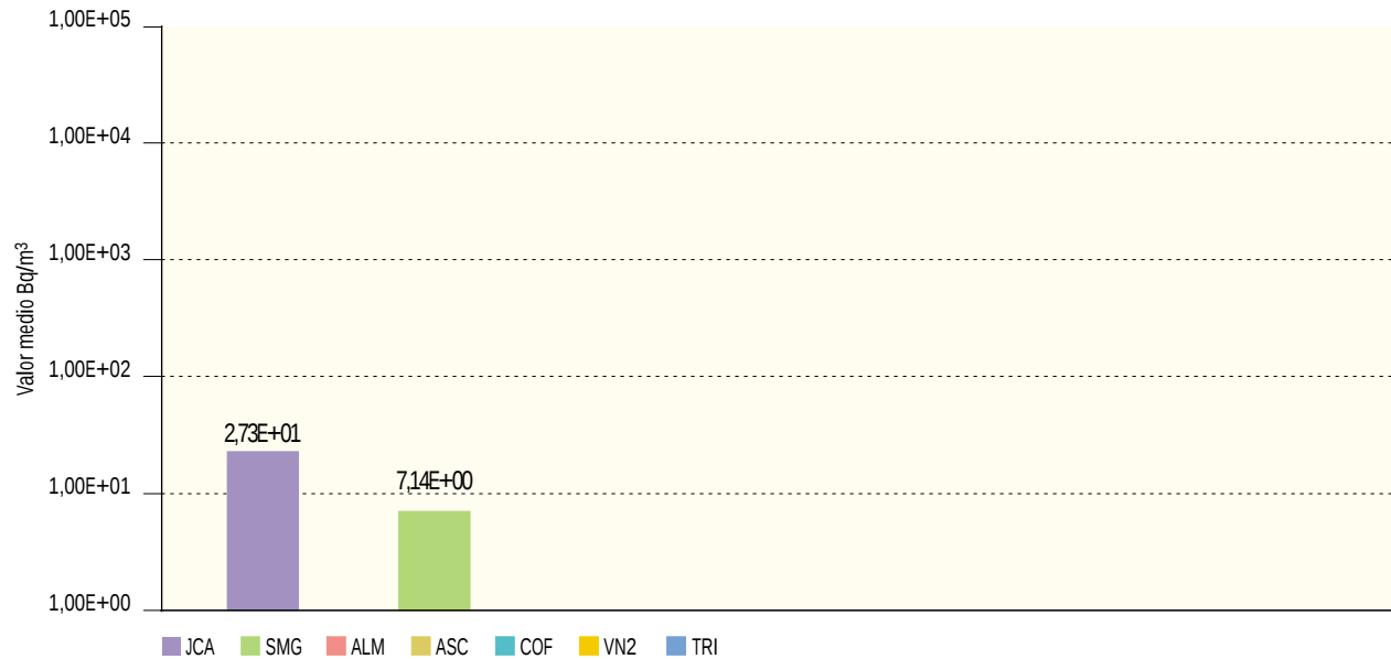
Figura 2.21b. Agua potable. Concentración de actividad de Sr-90 (Bq/m³) Valores de la campaña de 2003
