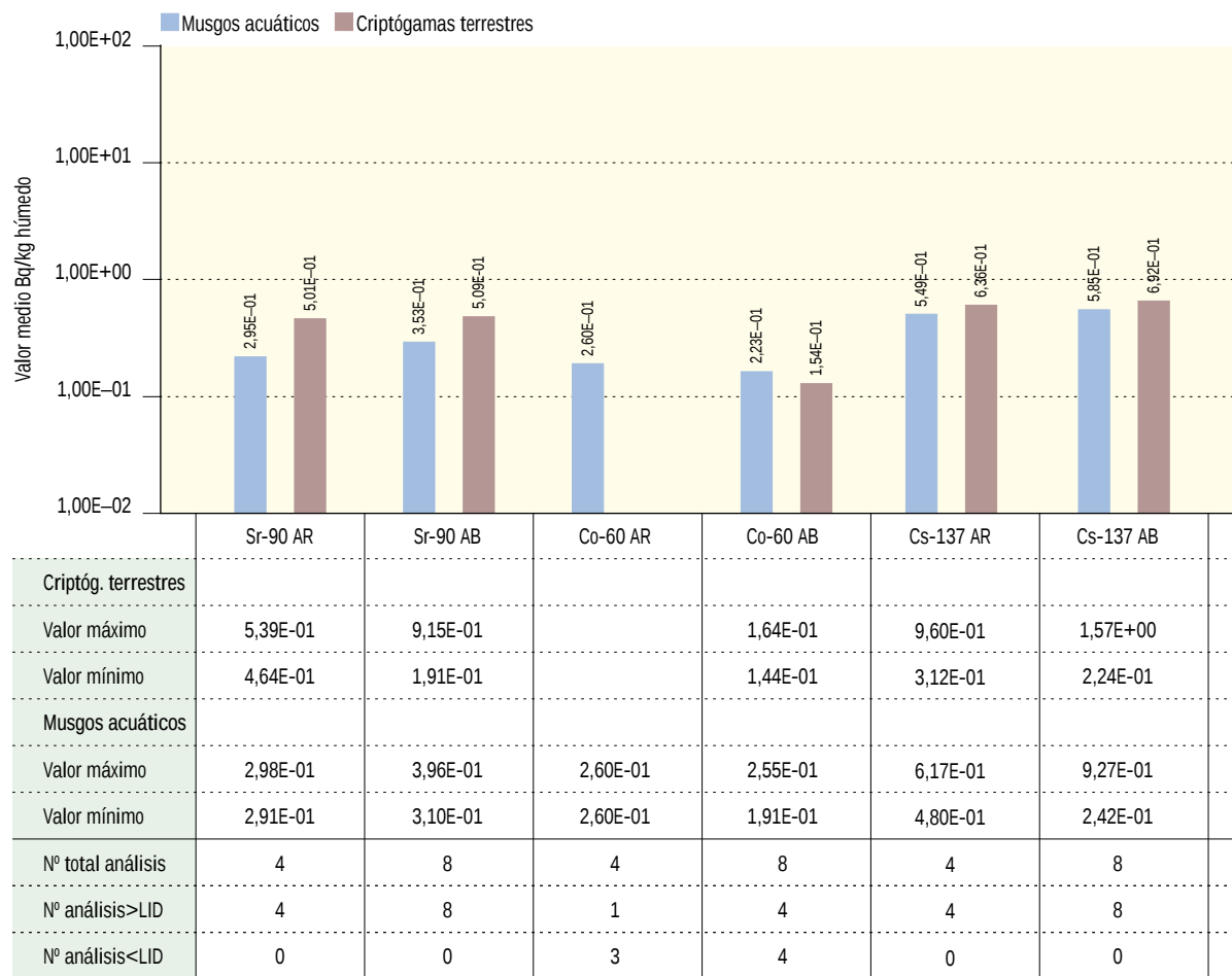
Figura 2.32b. Criptógamas. Central nuclear Santa María de Garoña. Concentración de actividad (Bq/kg húmedo)
