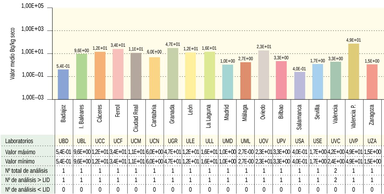
Figura 3.9b. Suelo. Concentración de actividad de Cs-137 (Bq/kg seco) Valores de la campaña de 2003
