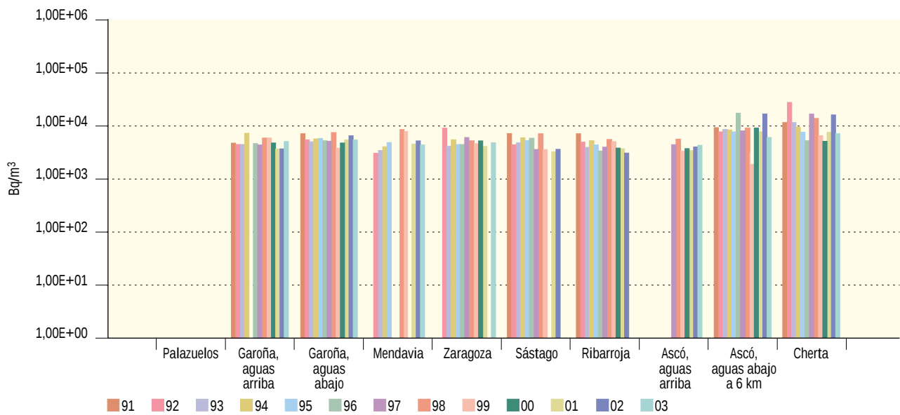
Figura 3.56. Río Ebro Evolución temporal de la concentración de actividad de H-3
