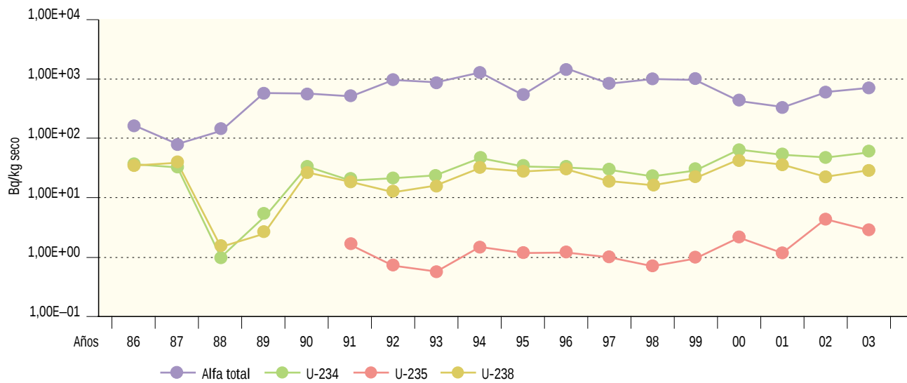
Figura 2.53. Juzbado. Sedimentos de fondo. Valores de concentración de actividad (Bq/kg seco) Evolución temporal valores medios
