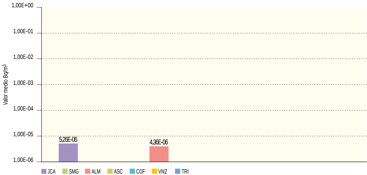
Figura 2.9b. Partículas de polvo en el aire. Concentración de actividad de Sr-90 (Bq/m³) Valores de la campaña de 2003
