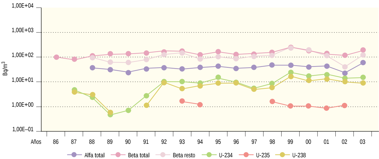
Figura 2.50. Juzbado. Agua superficial. Valores de concentración de actividad (Bq/m³) Evolución temporal valores medios
