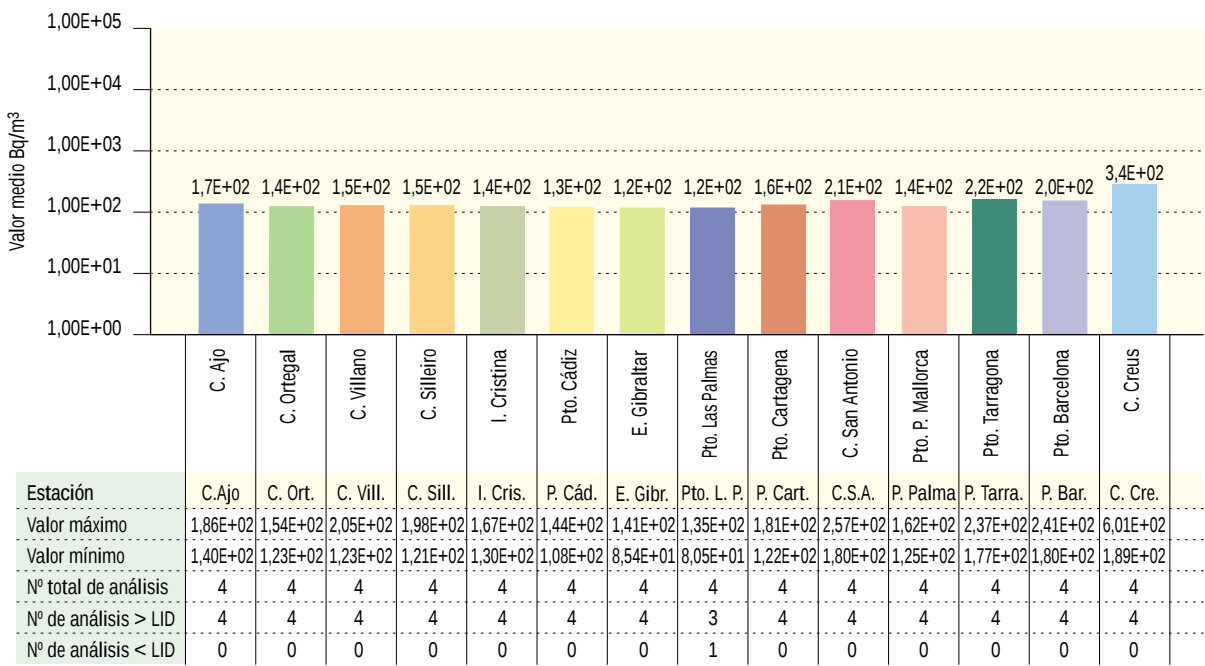
Figura 3.64b. Agua de mar. Concentración del índice de actividad de H-3 (Bq/m³) Valores de la campaña de 2003
