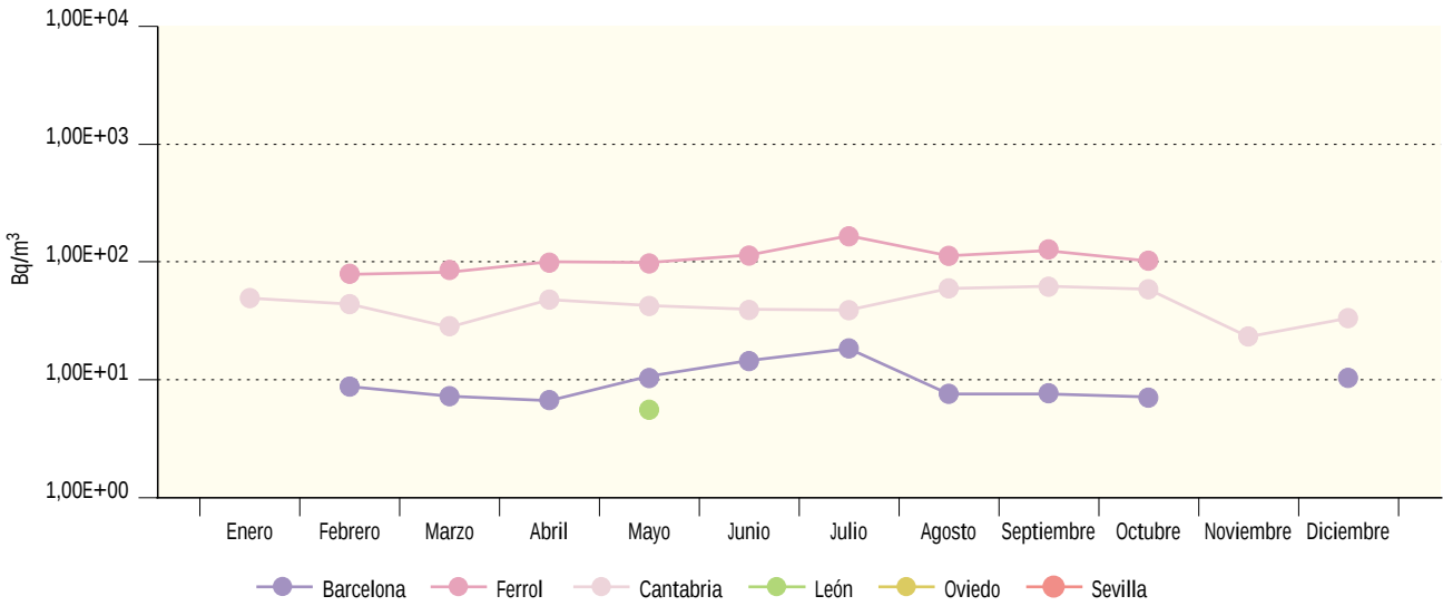
Figura 3.17. Leche. Concentración de actividad de Cs-137 (Bq/m³) Valores de la campaña de 2003
