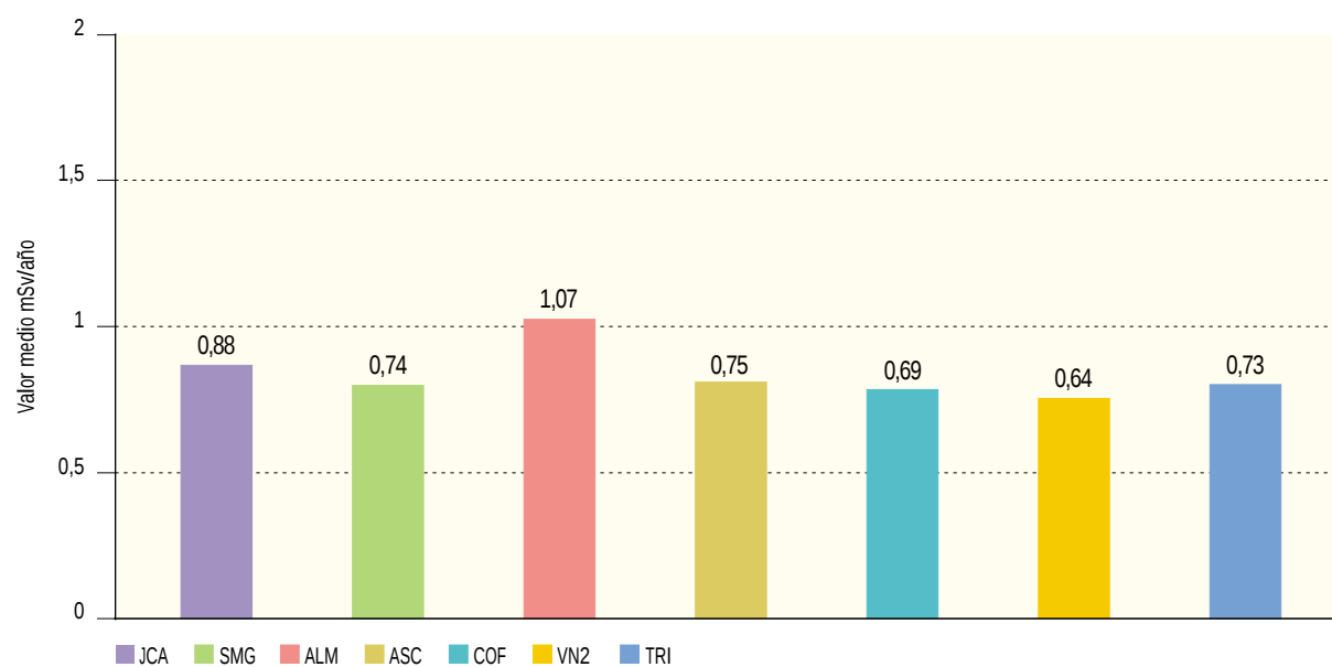
Figura 2.12b. Radiación directa. Dosis integrada (DTL) (mSv/año)
