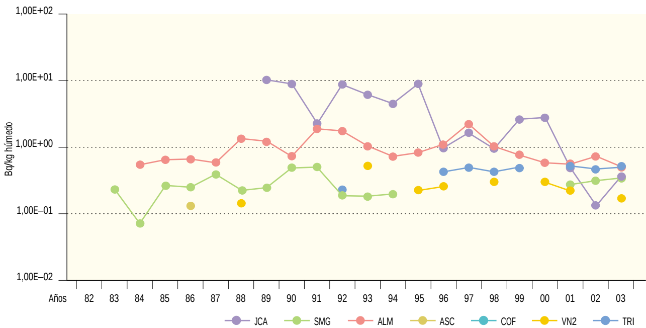
Figura 2.40b. Peces y mariscos. Concentración de actividad de Cs-137 (Bq/kg húmedo) Valores de la campaña de 2003
