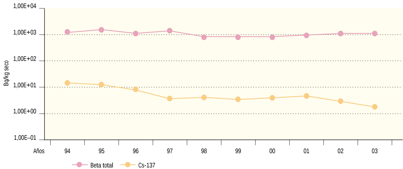
Figura 2.54. El Cabril. Sedimentos de fondo. Valores de concentración de actividad (Bq/kg seco) Evolución temporal valores medios
