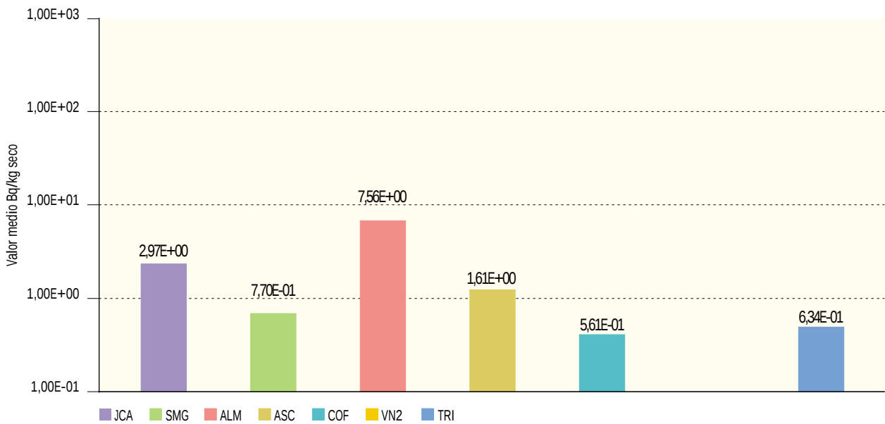
Figura 2.23b. Sedimentos de fondo. Concentración de actividad de Sr-90 (Bq/kg seco) Valores de la campaña de 2003
