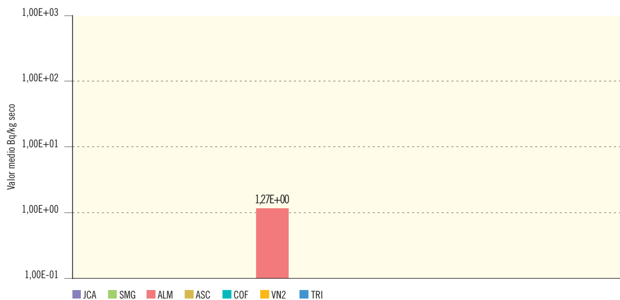
Figura 2.27b. Sedimentos de fondo. Concentración de actividad de Mn-54 (Bq/kg seco)
