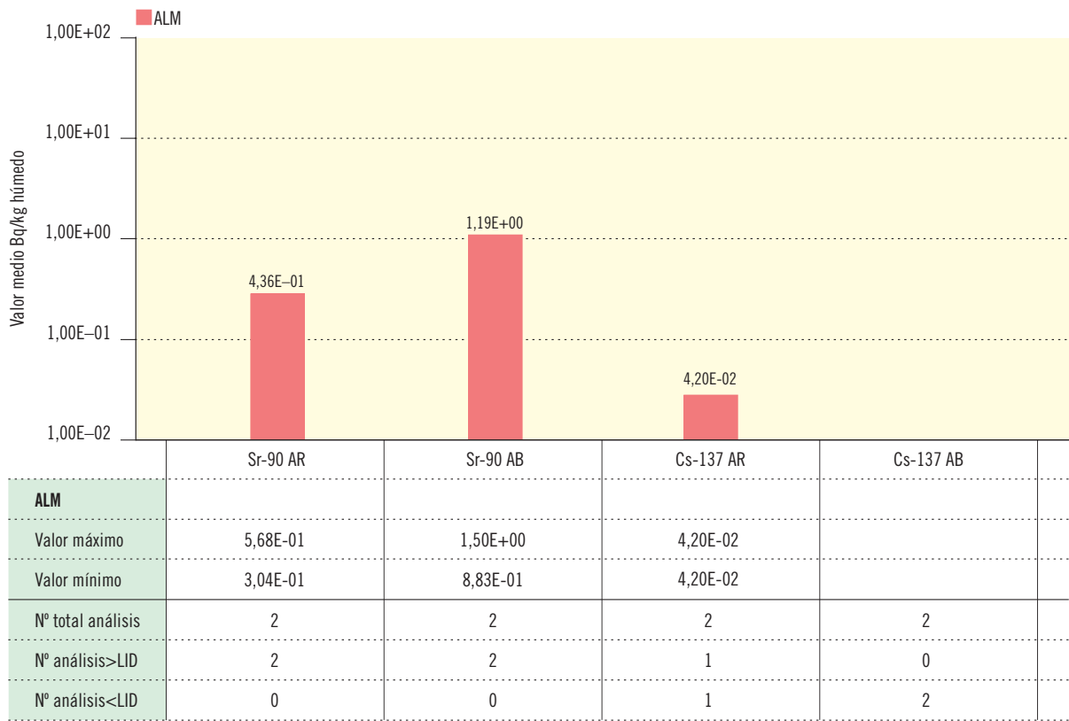
Figura 2.30b. Plantas terrestres. Concentración de actividad (Bq/kg húmedo)
