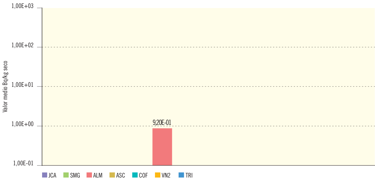
Figura 2.26b. Sedimentos de fondo. Concentración de actividad de Co-58 (Bq/kg seco)
