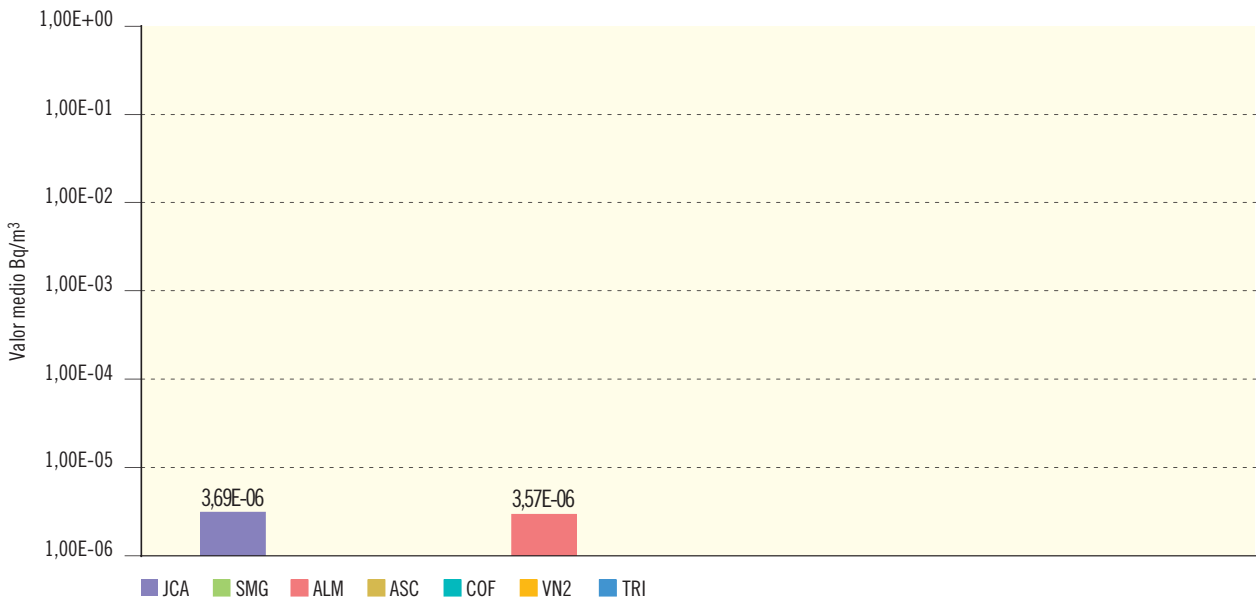
Figura 2.9b. Partículas de polvo en aire. Concentración de actividad de Sr-90 (Bq/m³)
