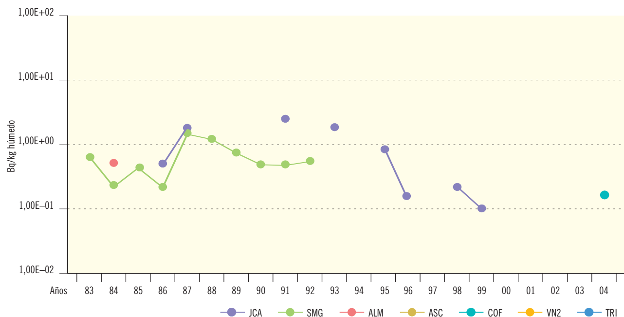
Figura 2.40b. Peces y mariscos. Concentración de actividad de de Co-60 (Bq/kg húmedo)
