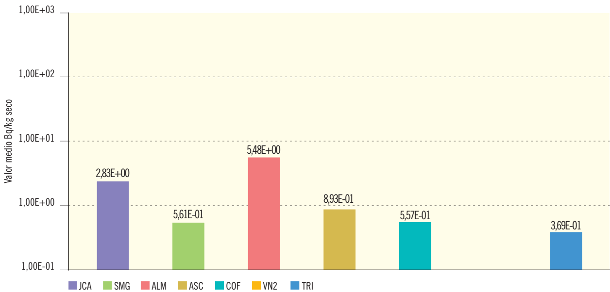
Figura 2.22b. Sedimentos de fondo. Concentración de actividad de Sr-90 (Bq/kg seco)
