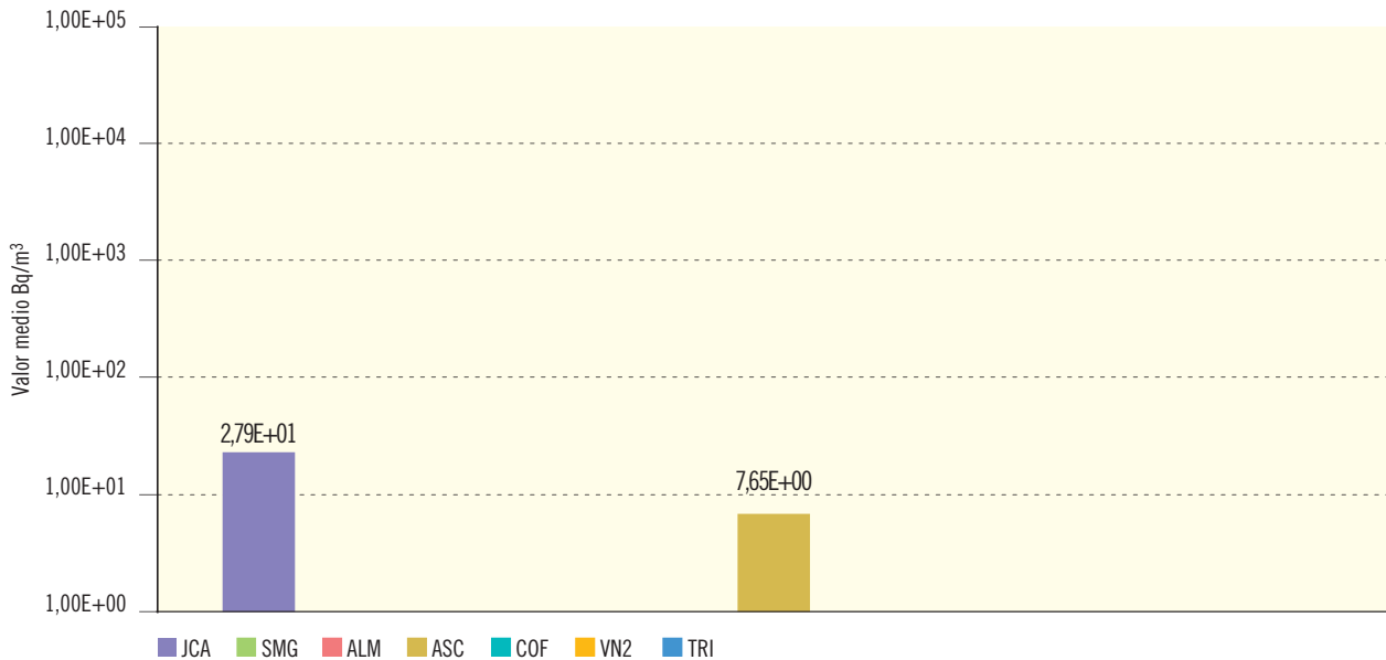
Figura 2.20b. Agua potable. Concentración de actividad de Sr-90 (Bq/m³)
