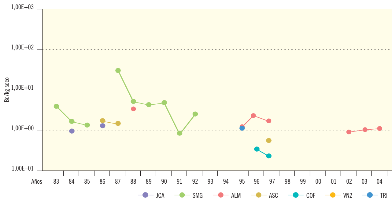
Figura 2.27b. Sedimentos de fondo. Concentración de actividad de Mn-54 (Bq/kg seco)
