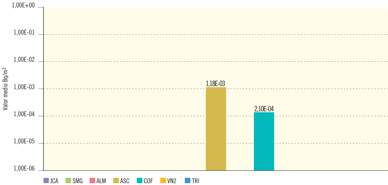
Figura 2.10b. Radiyodos en el aire. Concentración de actividad de I-131 (Bq/m³)
