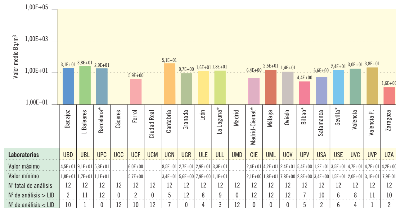
Figura 3.10b. Agua potable. Concentración de actividad de alfa total (Bq/m³)
