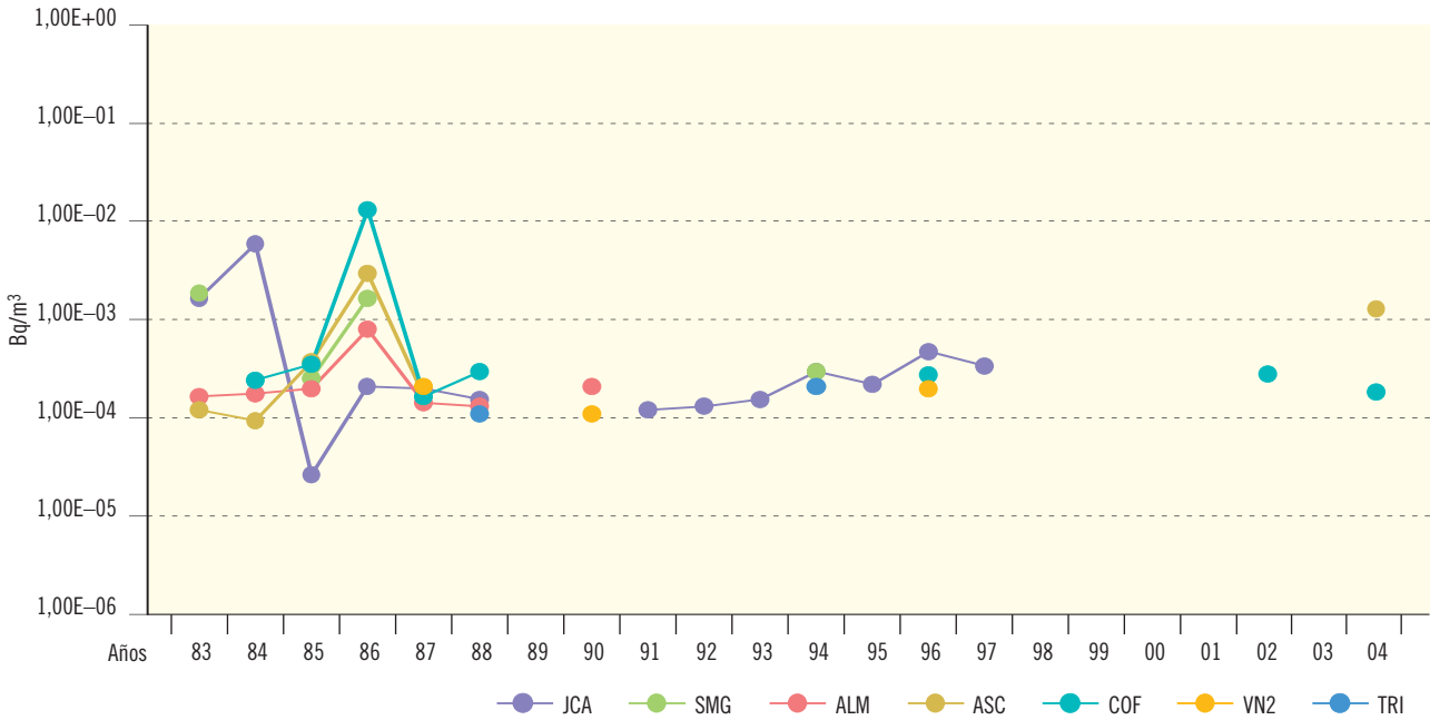
Figura 2.10b. Radiyodos en el aire. Concentración de actividad de I-131 (Bq/m³)
