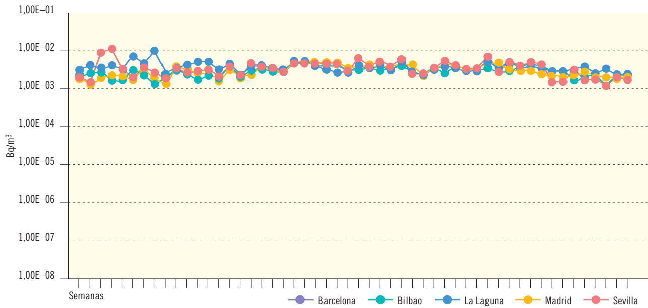
Figura 3.6b. Partículas de polvo en el aire. Muestreador alto flujo Concentración de actividad de Be-7 (Bq/m³). Valores de la campaña de 2004
