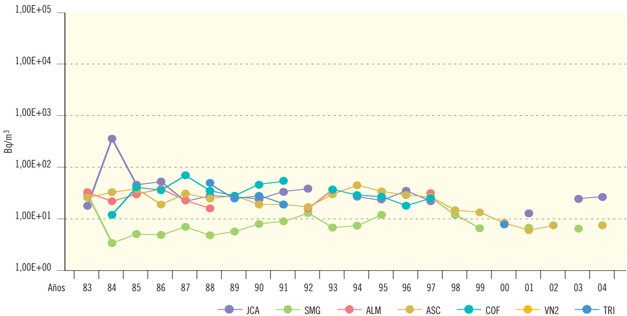
Figura 2.20b. Agua potable. Concentración de actividad de Sr-90 (Bq/m³)
