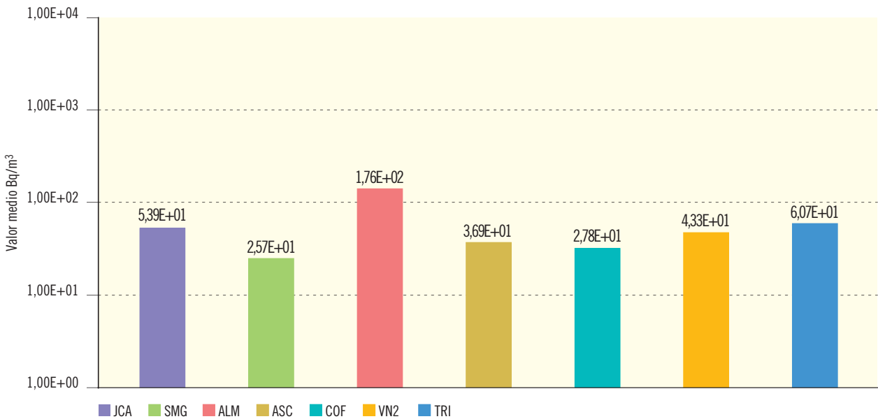
Figura 2.33b. Leche. Concentración de actividad de Sr-90 (Bq/m³)
