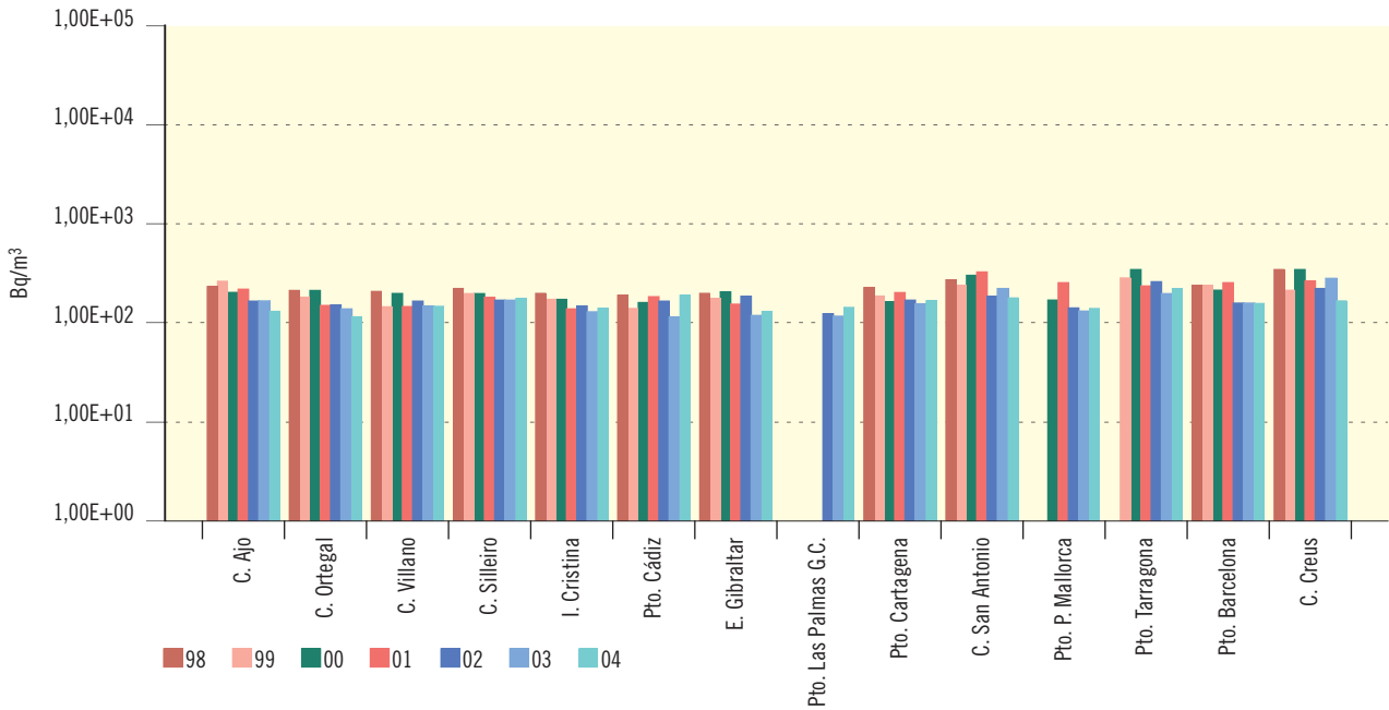
Figura 3.64a. Agua de mar
