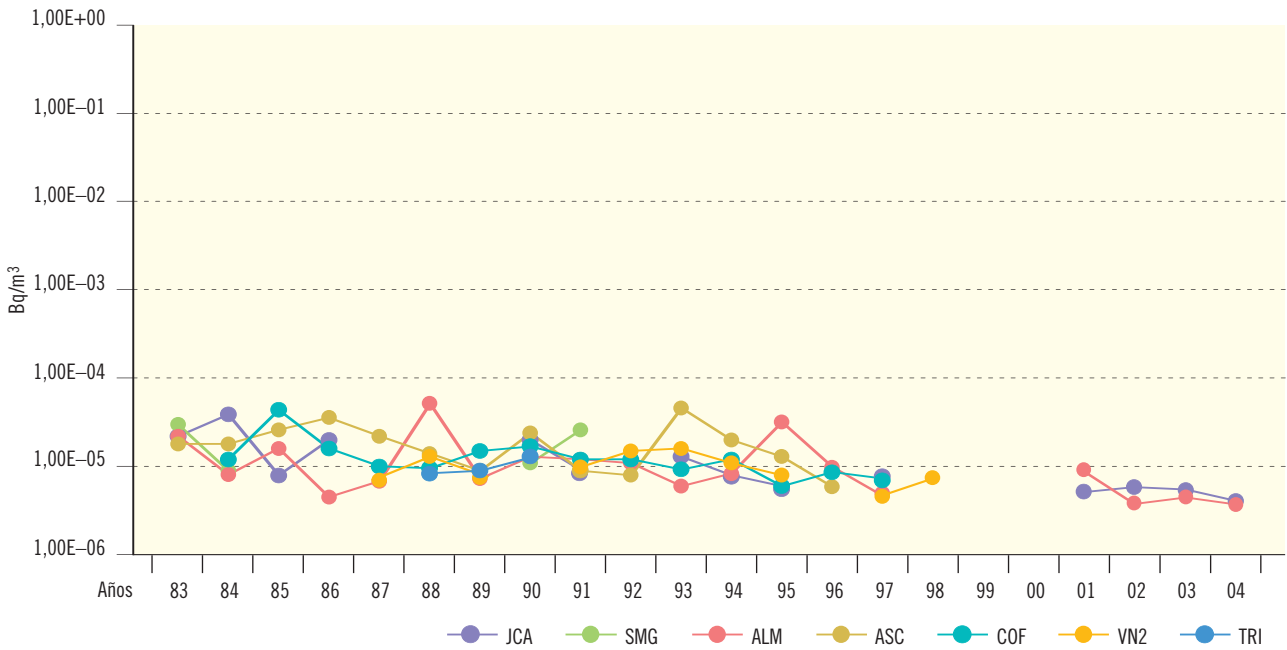
Figura 2.9b. Partículas de polvo en aire. Concentración de actividad de Sr-90 (Bq/m³)
