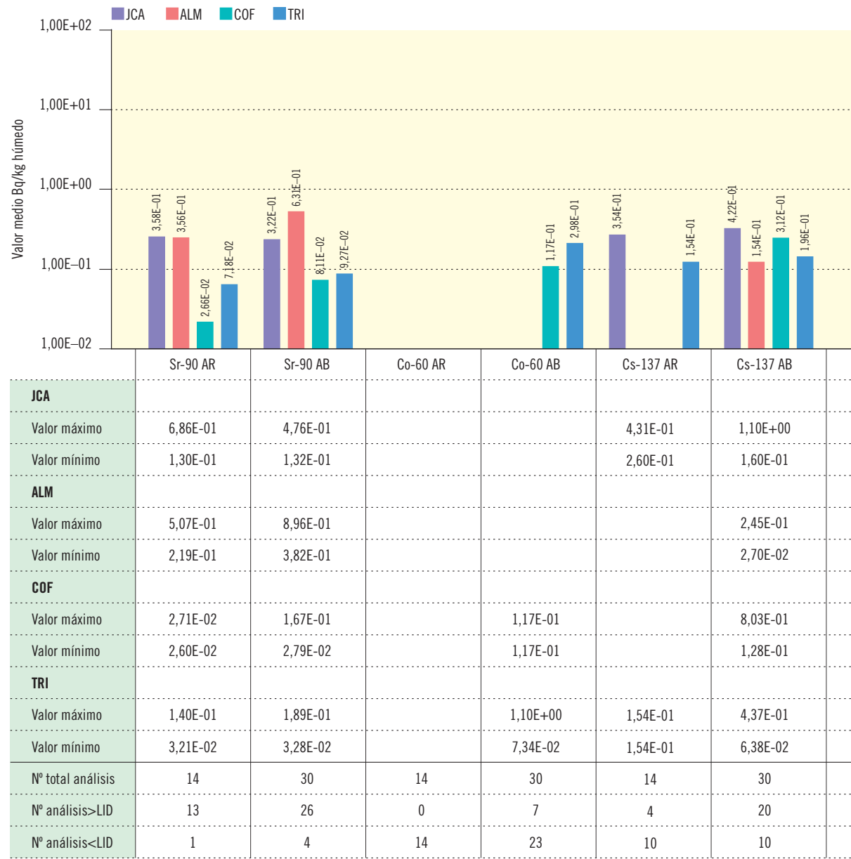
Figura 2.29b. Plantas de orilla. Concentración de actividad (Bq/kg húmedo)
