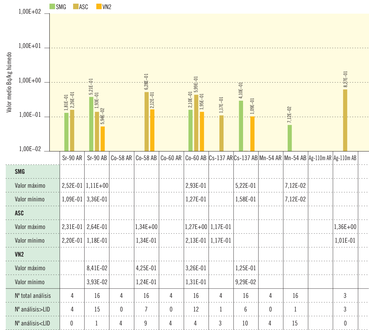
Figura 2.28b. Plantas acuáticas. Concentración de actividad (Bq/kg húmedo)
