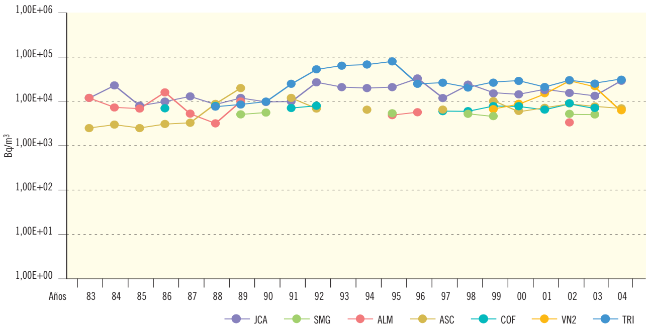
Figura 2.21b. Agua potable. Concentración de actividad de H-3 (Bq/m³)
