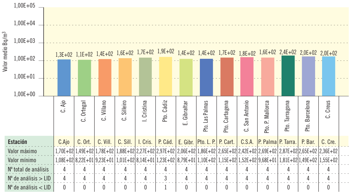
Figura 3.64b. Agua de mar. Concentración del índice de actividad de H-3 (Bq/m³)
