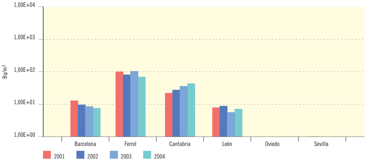
Figura 3.17b. Leche. Concentración de actividad de Cs-137 (Bq/m³)
