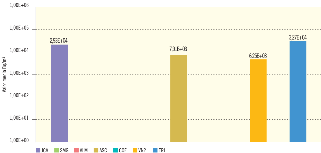
Figura 2.21b. Agua potable. Concentración de actividad de H-3 (Bq/m³)
