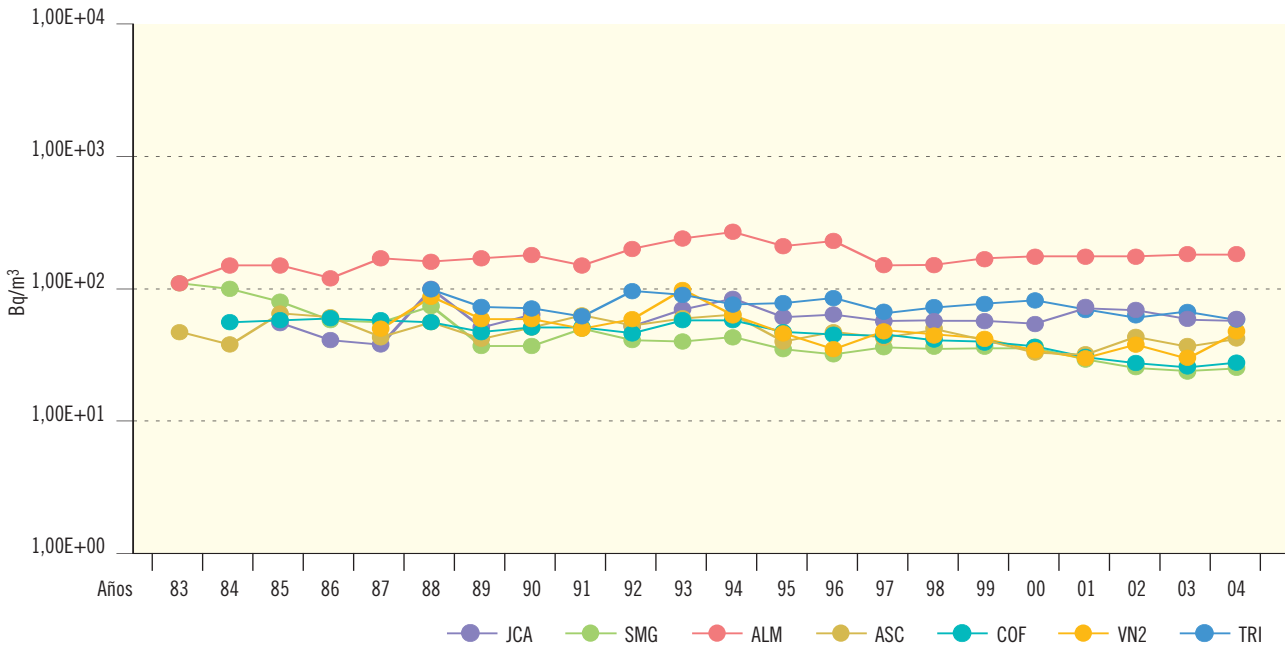
Figura 2.33b. Leche. Concentración de actividad de Sr-90 (Bq/m³)
