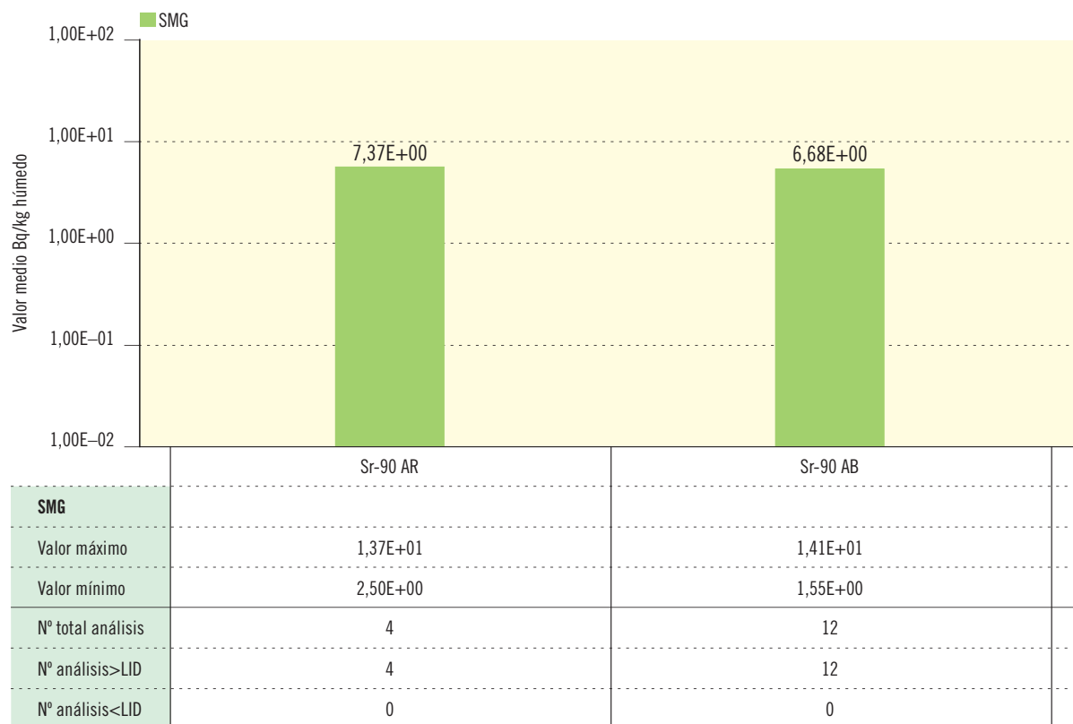
Figura 2.32b. Fauna terrestre. Concentración de actividad (Bq/kg húmedo)
