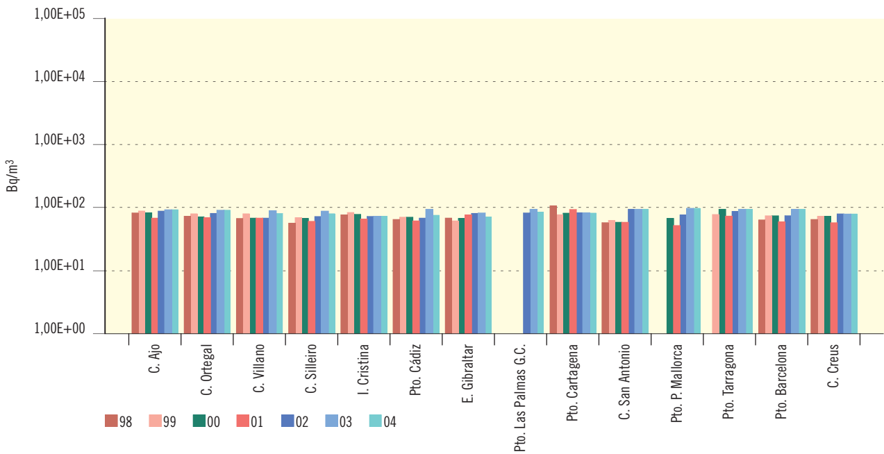
Figura 3.62a. Agua de mar
