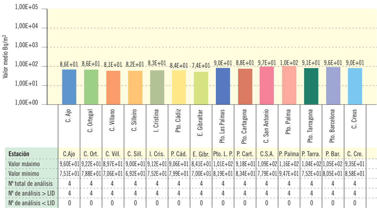
Figura 3.62b. Agua de mar. Concentración del índice de actividad alfa total (Bq/m³)
