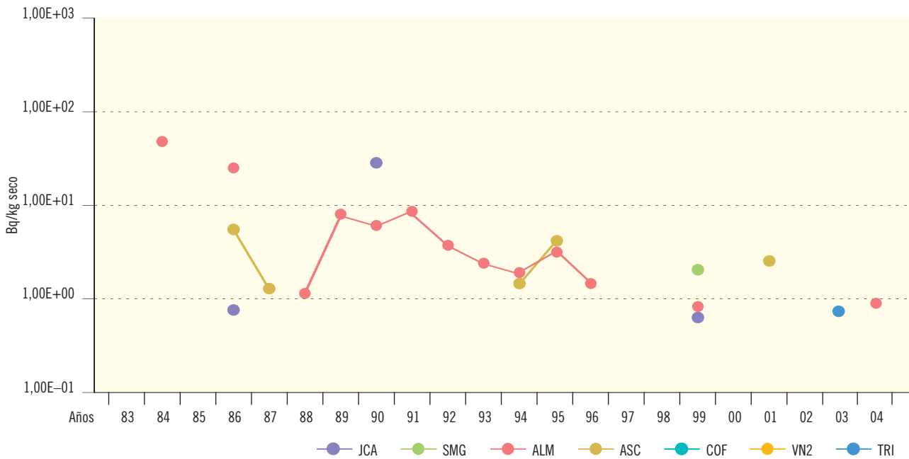
Figura 2.26b. Sedimentos de fondo. Concentración de actividad de Co-58 (Bq/kg seco)
