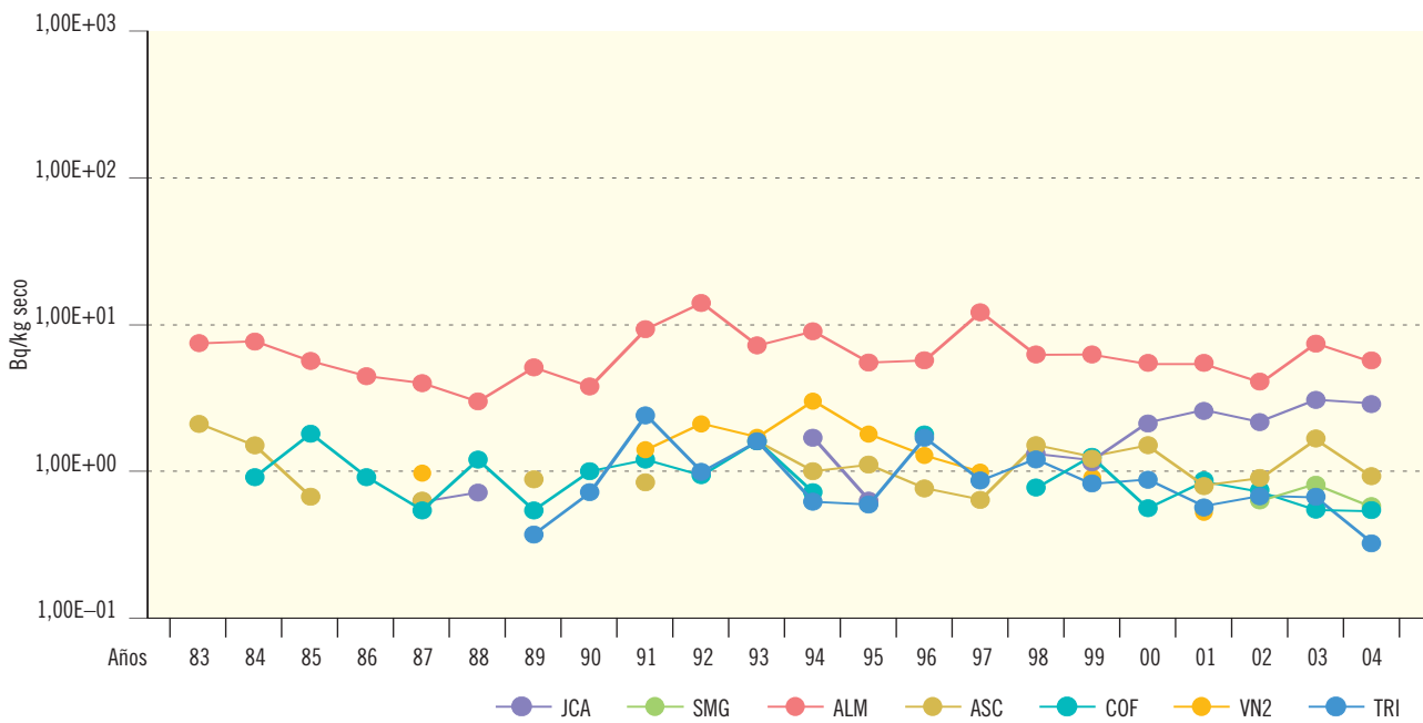
Figura 2.22b. Sedimentos de fondo. Concentración de actividad de Sr-90 (Bq/kg seco)
