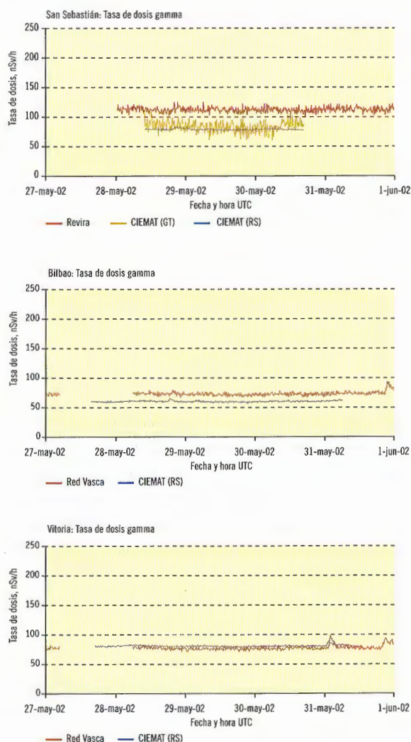
Figura 3.7. Resultados de las medidas de la tasa de dosis gamma ambiental en las estaciones del País Vasco (San Sebastián, Bilbao y Vitoria)
