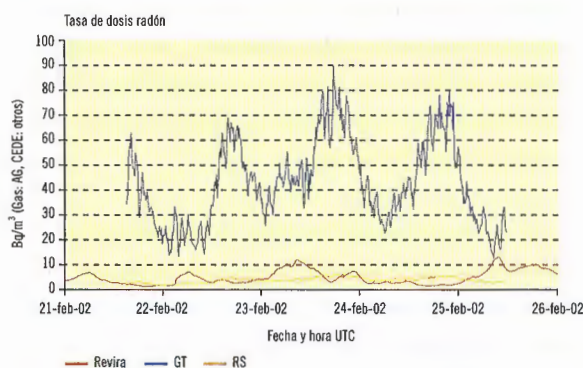
Figura 3.4. Resultados de las medidas comparadas de radón en la estación REA de Autilla
