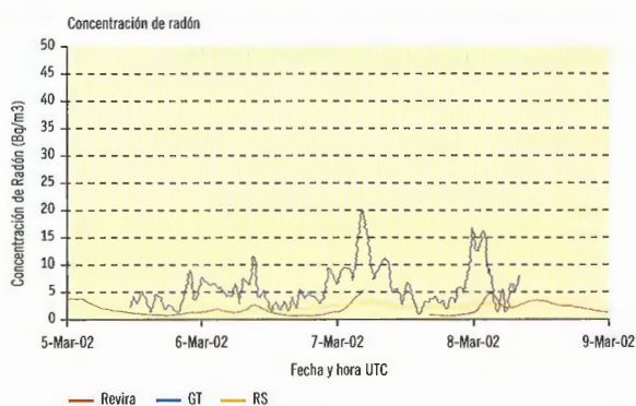
Figura 3.6. Resultados de las medidas comparadas de la tasa de radón en la estación de REA de Lugo
