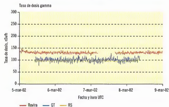
Figura 3.5. Resultados de las medidas comparadas de la tasa de dosis gamma en la estación REA de Lugo
