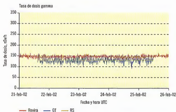
Figura 3.3. Resultados de las medidas comparadas de la tasa de dosis gamma en la REA de Autilla
