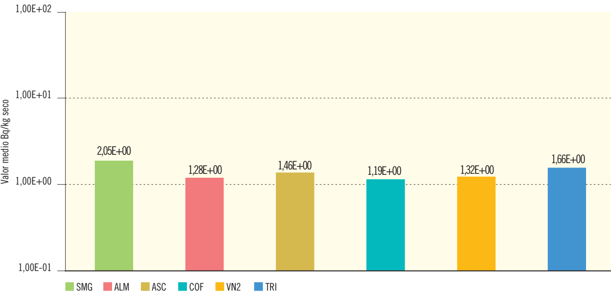
Figura 2.11b. Suelo. Concentración de actividad de Sr-90 (Bq/kg seco)
