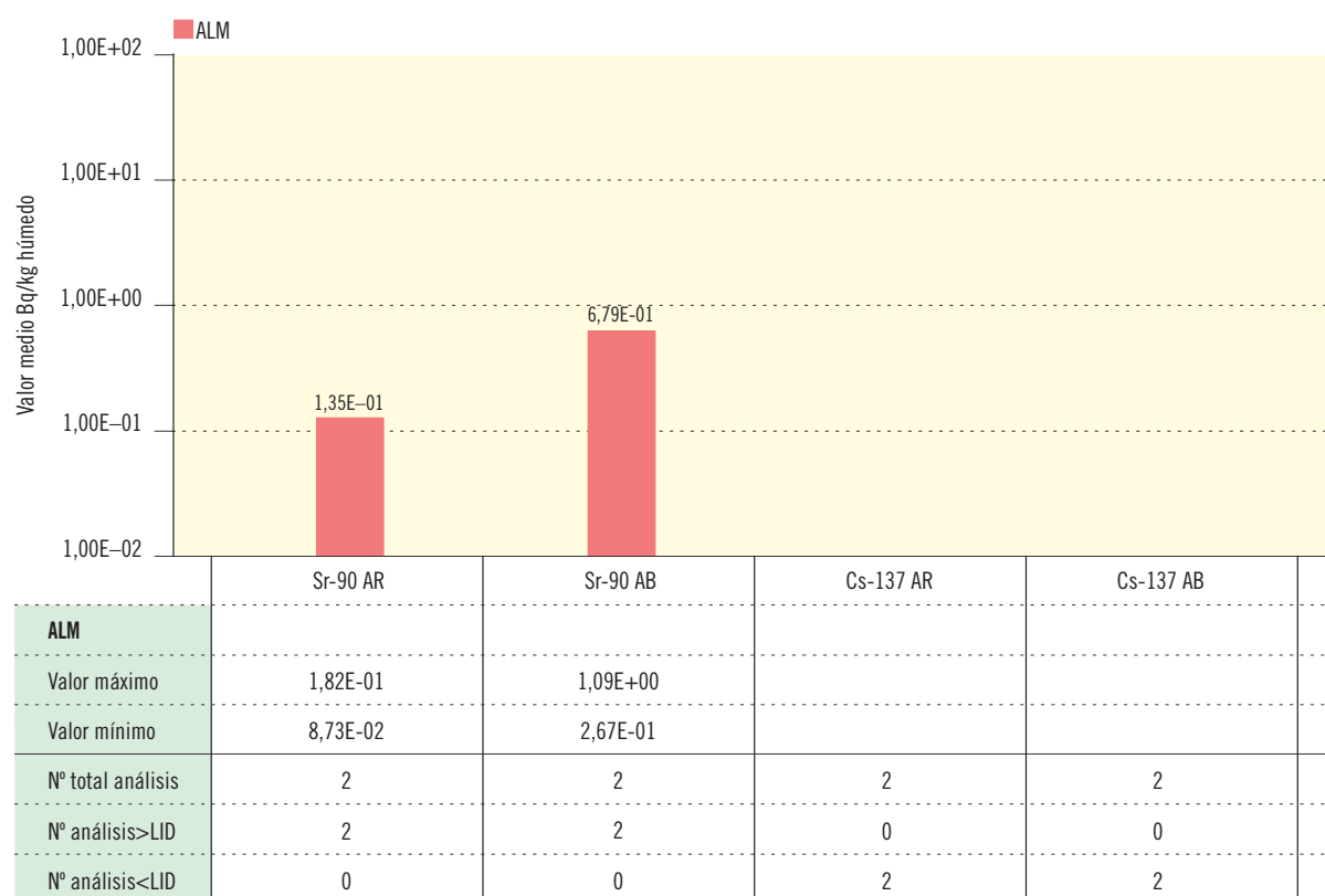
Figura 2.29b. Plantas terrestres. Concentración de actividad (Bq/kg húmedo)
