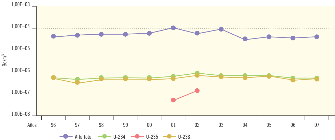
Figura 2.39. Juzbado. Partículas de polvo en el aire. Valores de concentración de actividad (Bq/m³)
