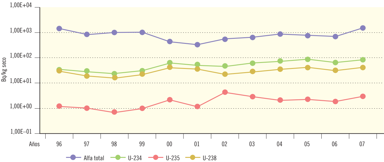
Figura 2.48. Juzbado. Sedimentos de fondo. Valores de concentración de actividad (Bq/kg seco)
