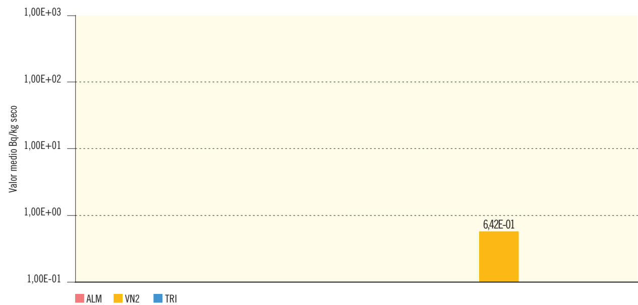
Figura 2.26b. Sedimentos de orilla. Concentración de actividad de Cs-137 (Bq/kg seco)
