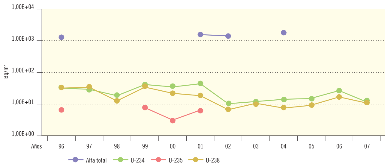
Figura 2.56. Juzbado. Leche. Valores de concentración de actividad (Bq/m³)
