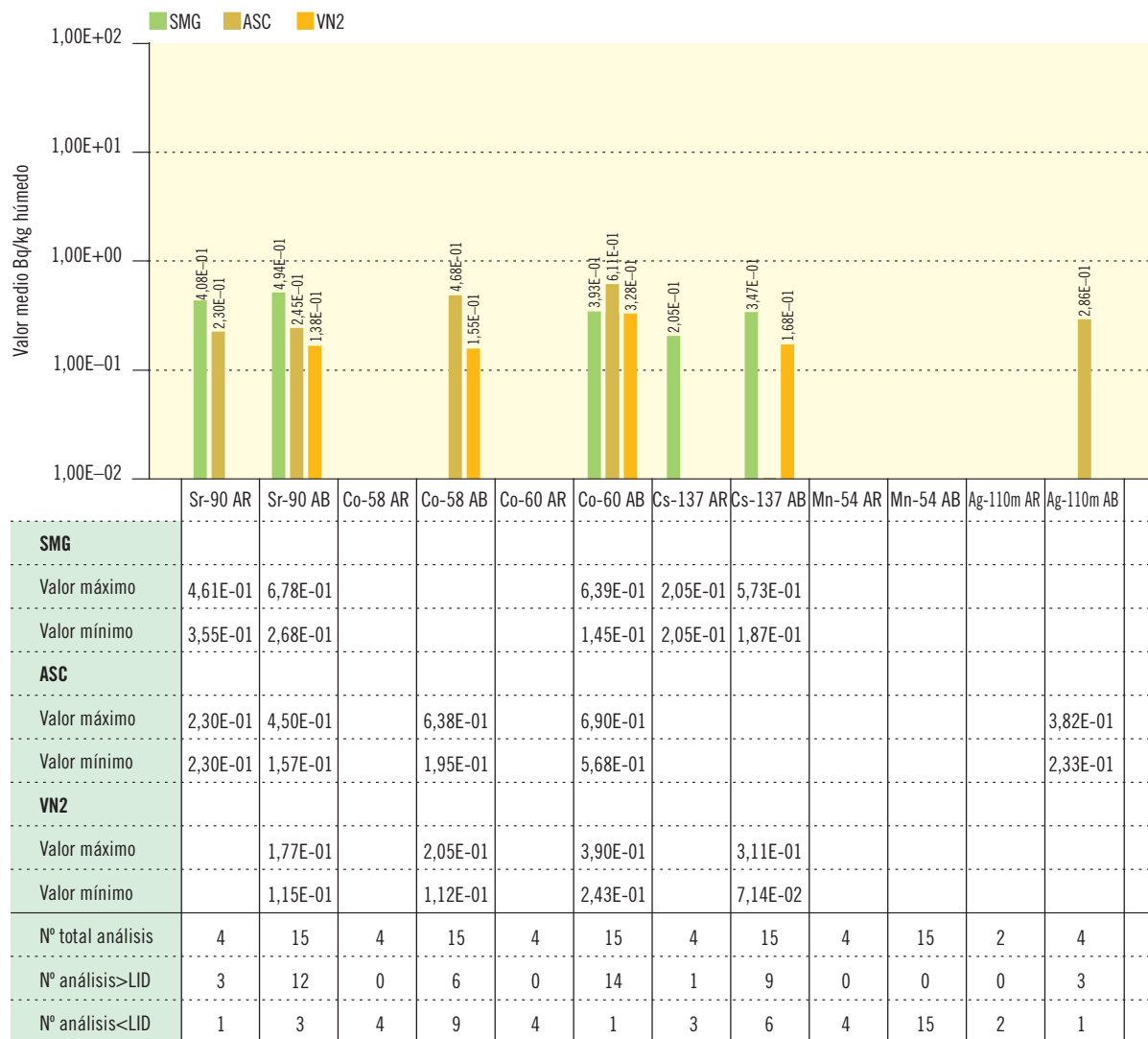
Figura 2.27b. Plantas acuáticas. Concentración de actividad (Bq/kg húmedo)
