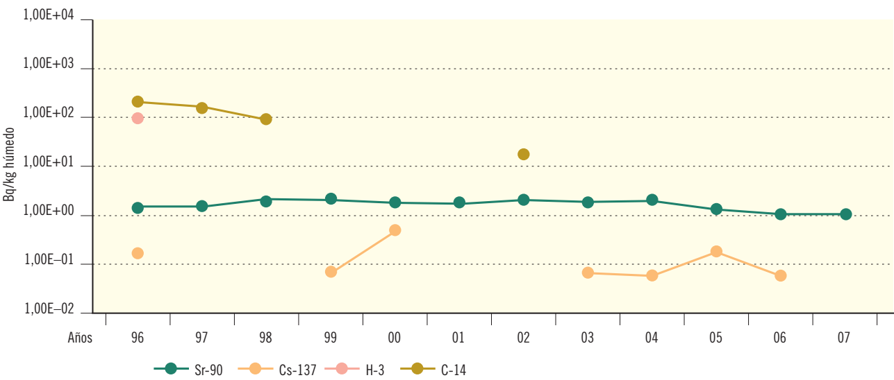
Figura 2.57. El Cabril. Plantas terrestres. Valores de concentración de actividad (Bq/kg húmedo)
