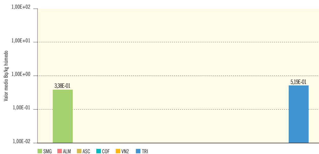
Figura 2.37b. Peces y mariscos. Concentración de actividad de Cs-137 (Bq/kg húmedo)
