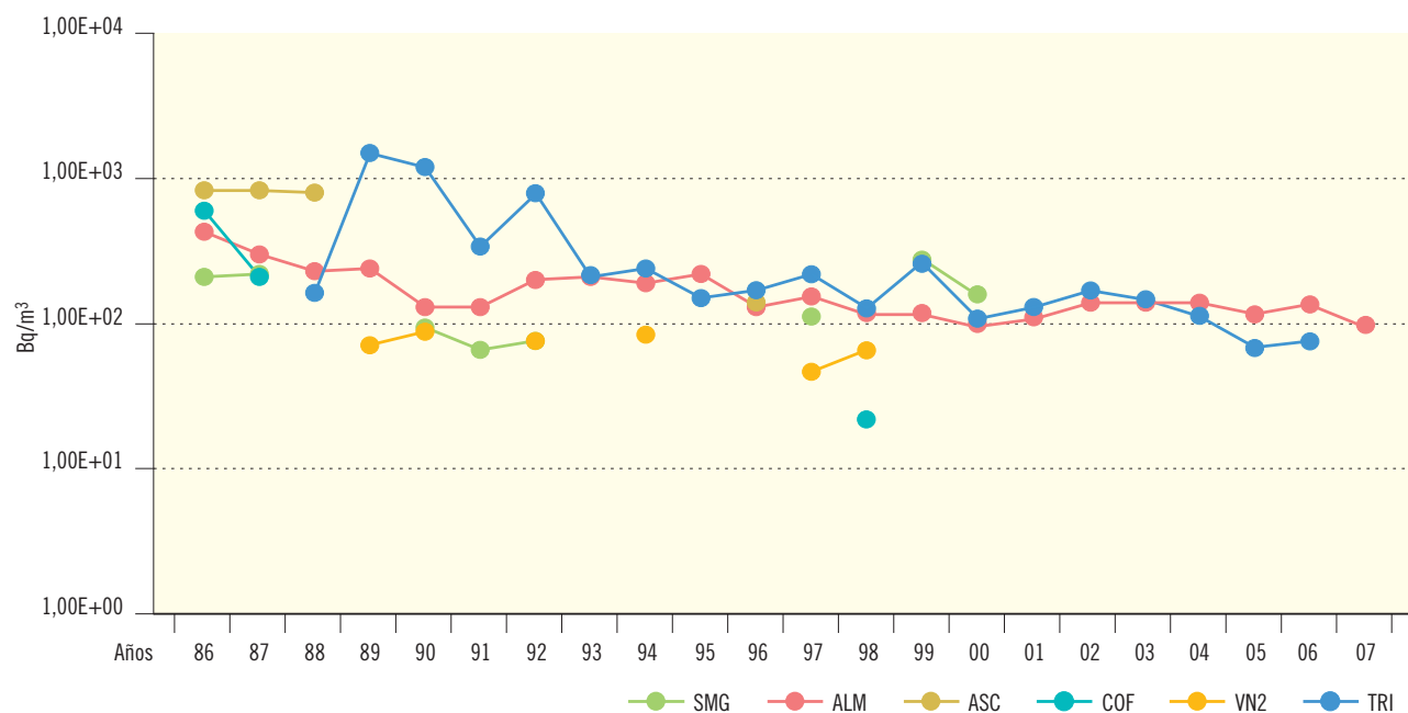
Figura 2.33b. Leche. Concentración de actividad de Cs-137 (Bq/m³)
