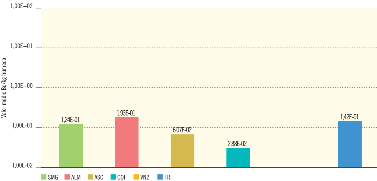
Figura 2.34b. Vegetales de hoja ancha. Concentración de actividad de Sr-90 (Bq/kg húmedo)
