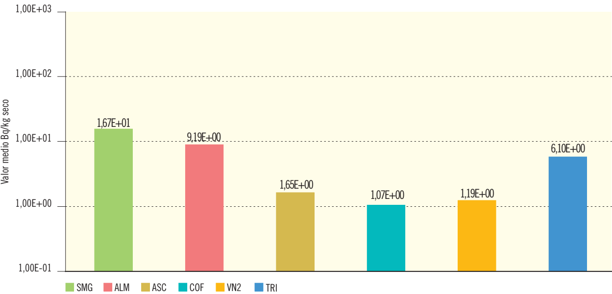
Figura 2.24b. Sedimentos de fondo. Concentración de actividad de Cs-137 (Bq/kg seco)
