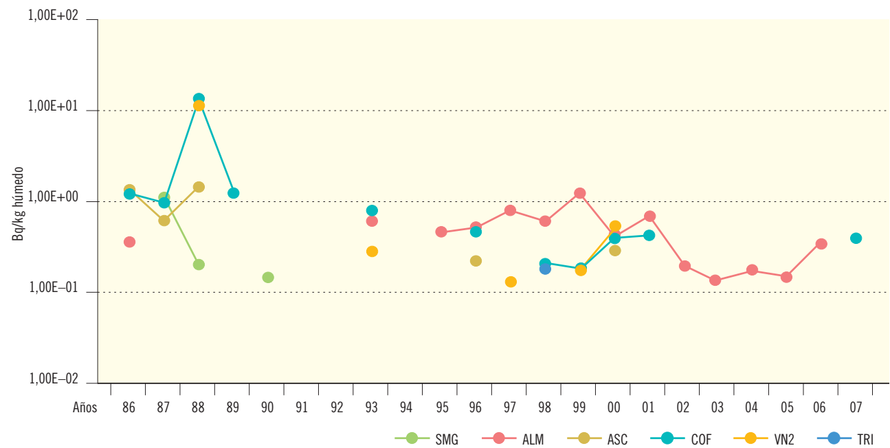
Figura 2.36b. Carne y aves. Concentración de actividad de Cs-137 (Bq/kg húmedo)
