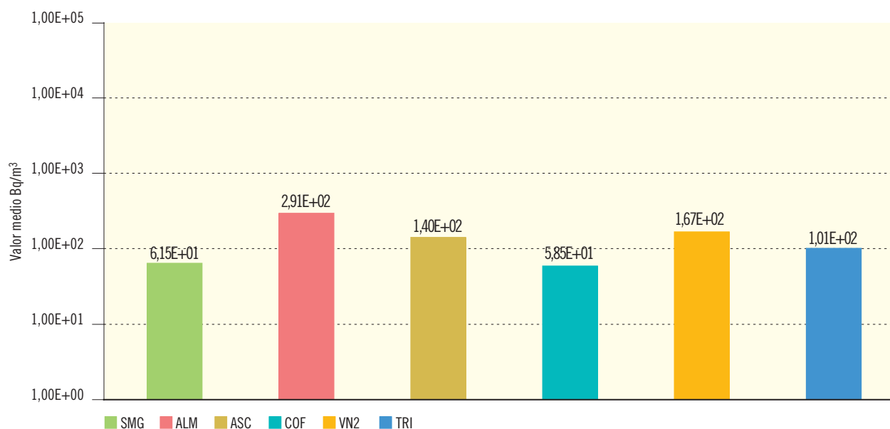
Figura 2.19b. Agua potable. Concentración del índice de actividad beta total (Bq/m³)
