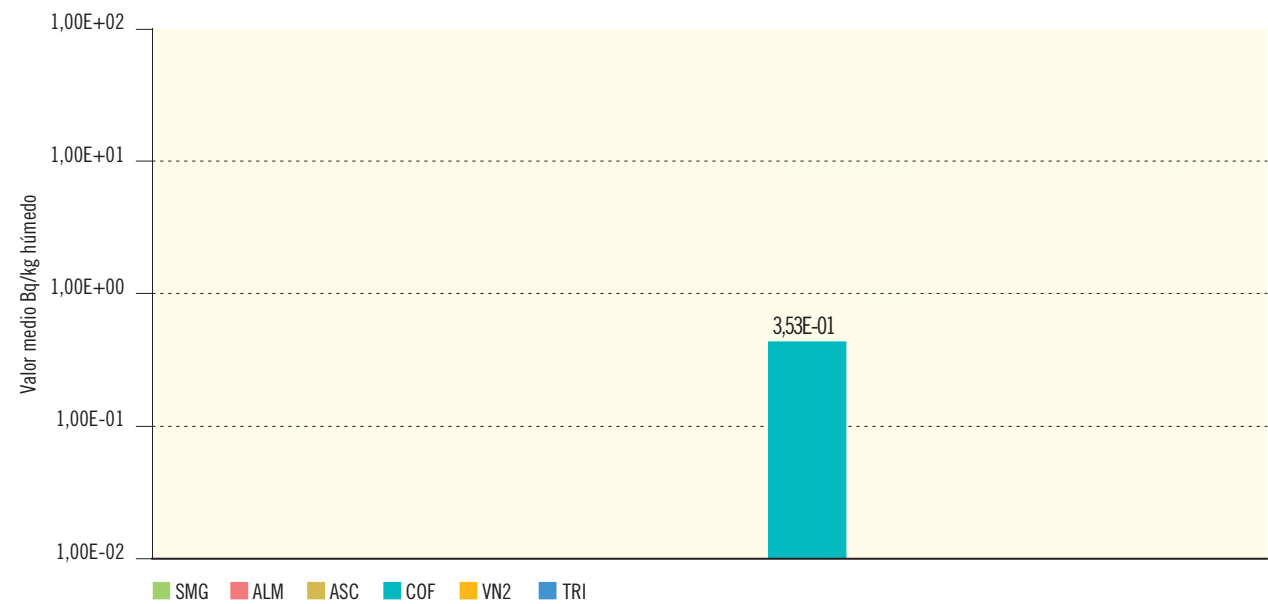
Figura 2.36b. Carne y aves. Concentración de actividad de Cs-137 (Bq/kg húmedo)
