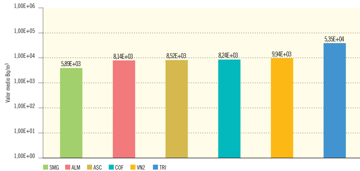
Figura 2.22b. Agua potable. Concentración de actividad de H-3 (Bq/m³)
