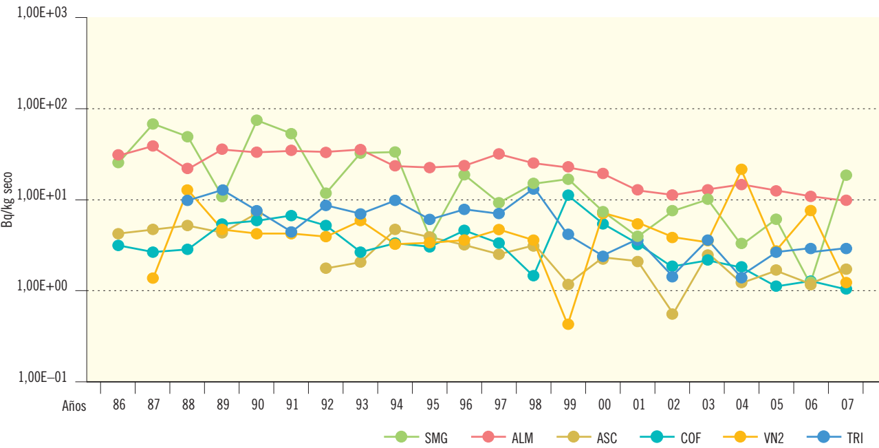
Figura 2.24b. Sedimentos de fondo. Concentración de actividad de Cs-137 (Bq/kg seco)
