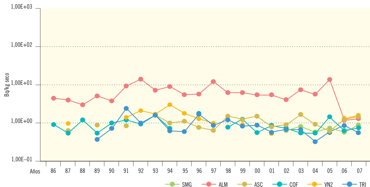
Figura 2.23b. Sedimentos de fondo. Concentración de actividad de Sr-90 (Bq/kg seco)
