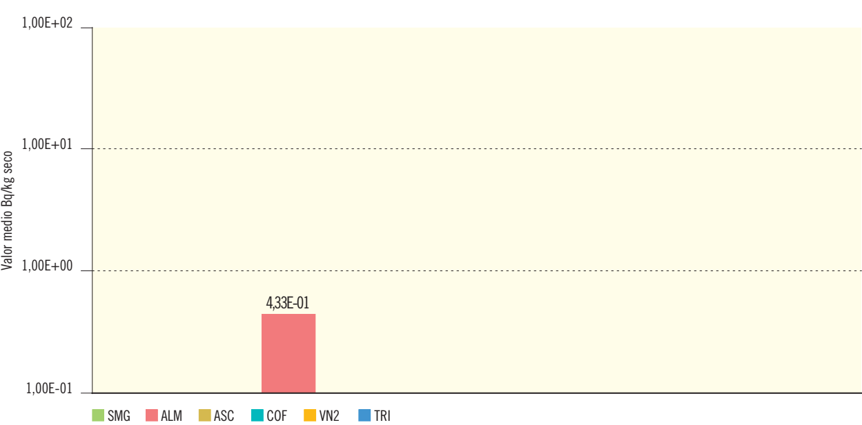
Figura 2.13b. Suelo. Concentracion de actividad de Co-60 (Bq/kg seco)
