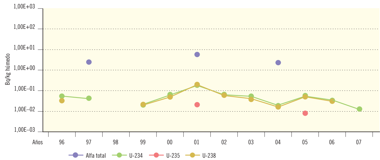
Figura 2.53. Juzbado. Vegetales de hoja ancha. Valores de concentración de actividad (Bq/kg húmedo)
