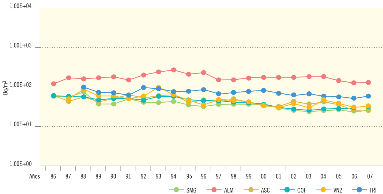
Figura 2.32b. Leche. Concentración de actividad de Sr-90 (Bq/m³)
