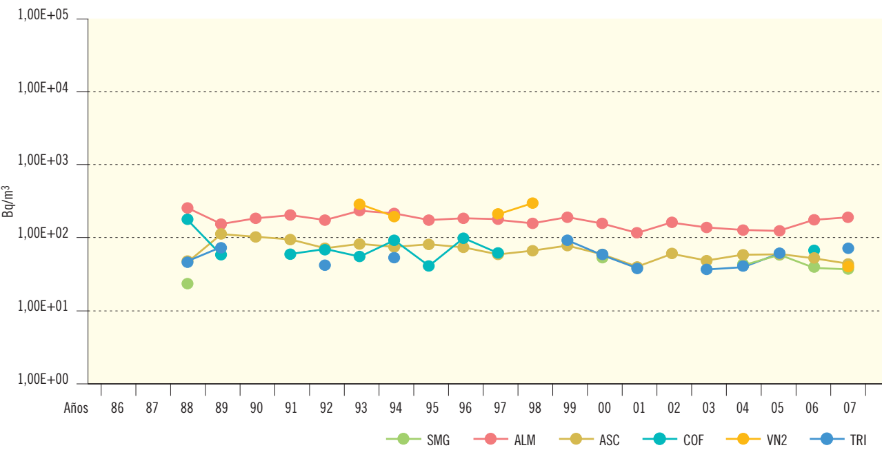
Figura 2.20b. Agua potable. Concentración del índice de actividad beta resto (Bq/m³) Valores de la campaña de 2007
