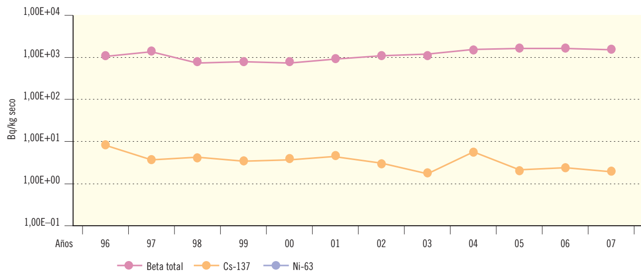
Figura 2.49. El Cabril. Sedimentos de fondo. Valores de concentración de actividad (Bq/kg seco)
