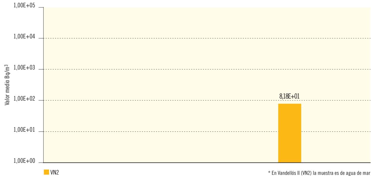
Figura 2.18b. Agua superficial. Concentración de actividad de Cs-137 (Bq/m³)
