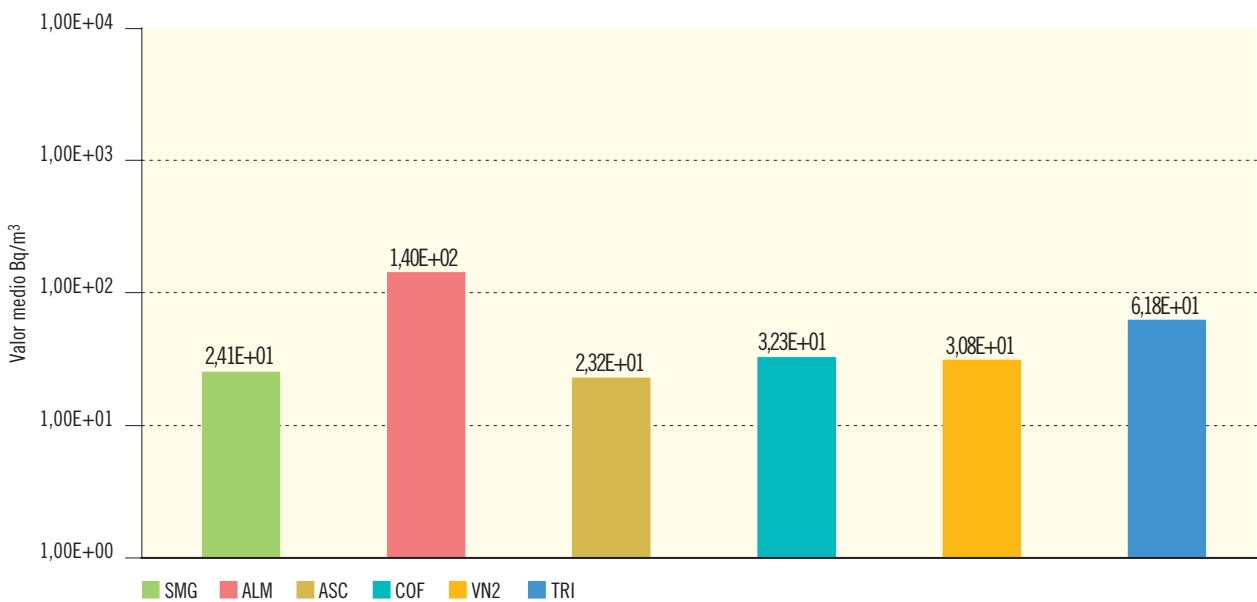
Figura 2.32b. Leche. Concentración de actividad de Sr-90 (Bq/m³)
