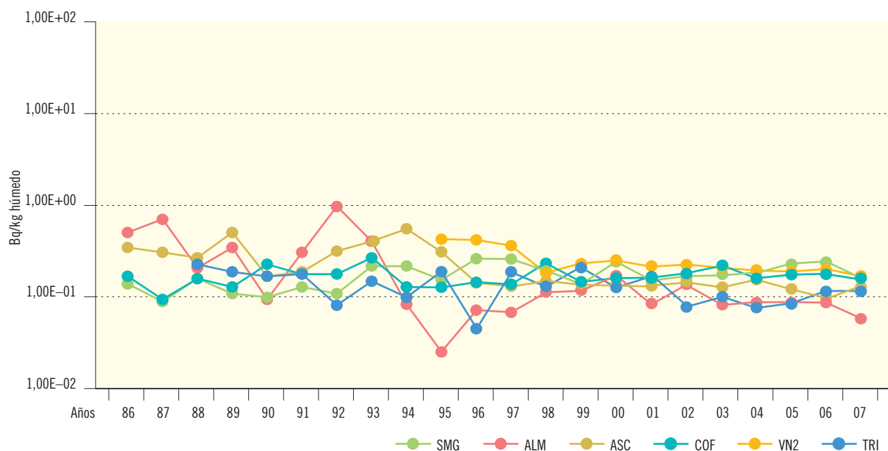
Figura 2.35b. Vegetales de hoja no ancha. Concentración de actividad de Sr-90 (Bq/kg húmedo)
