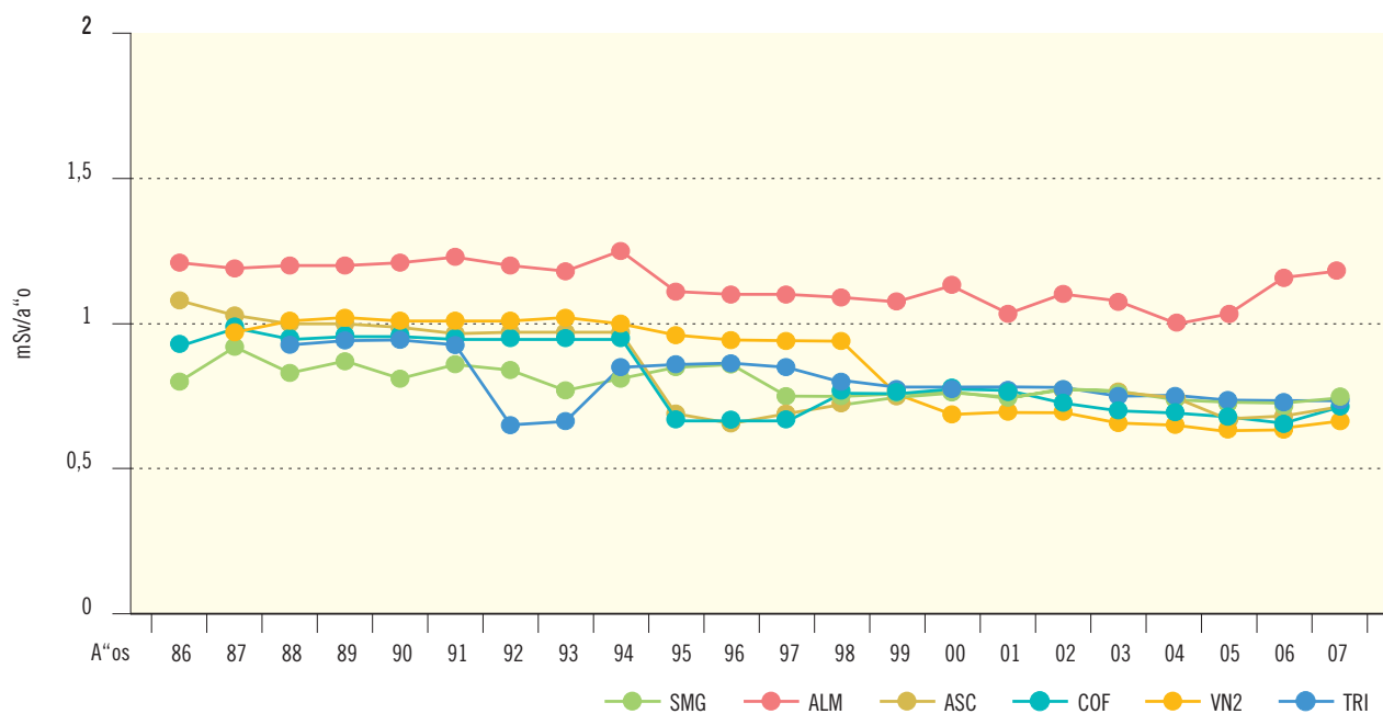
Figura 2.10b. Radiación directa. Dosis integrada (DTL) (mSv/año)
