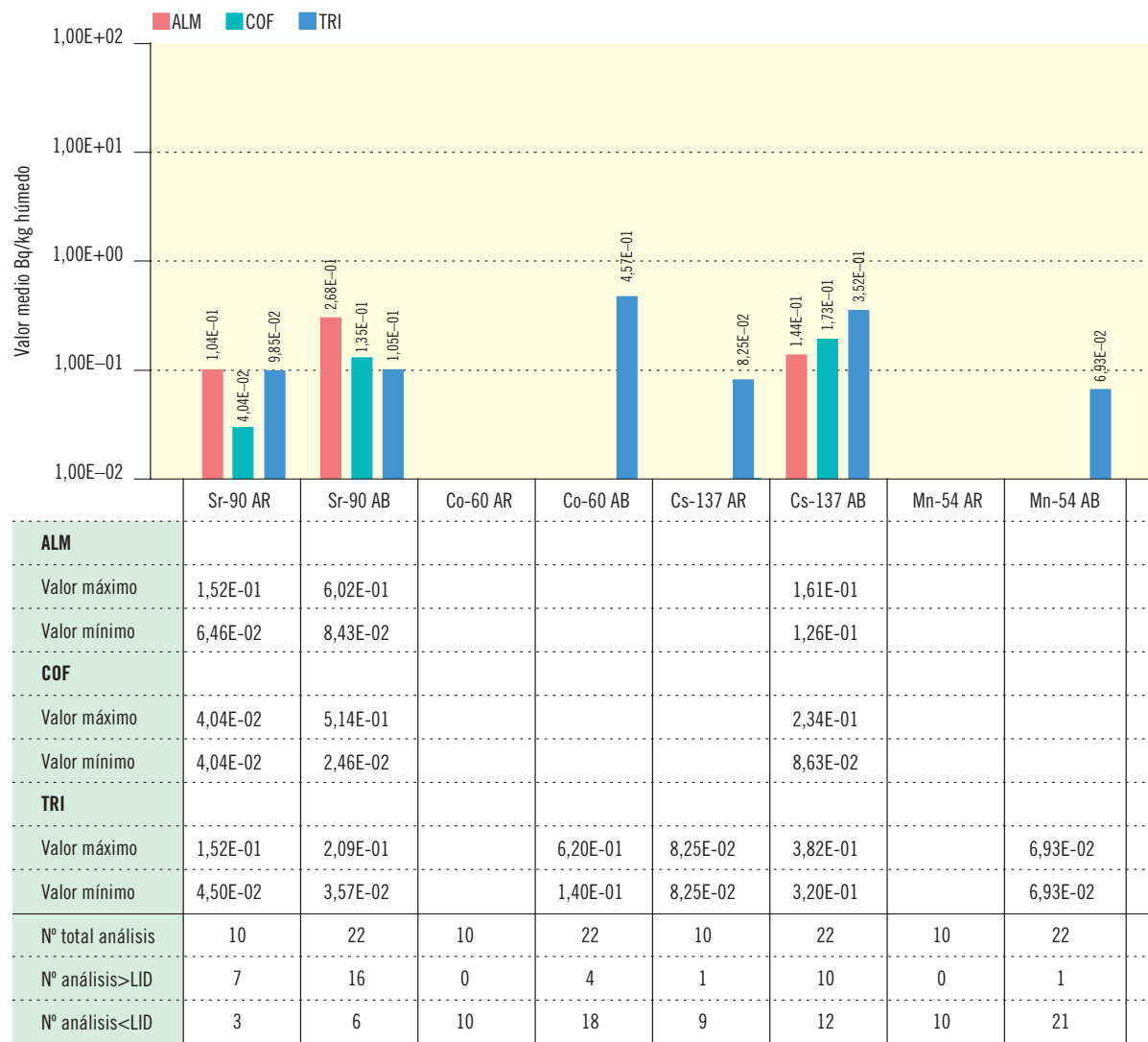
Figura 2.28b. Plantas de orilla. Concentración de actividad (Bq/kg húmedo)
