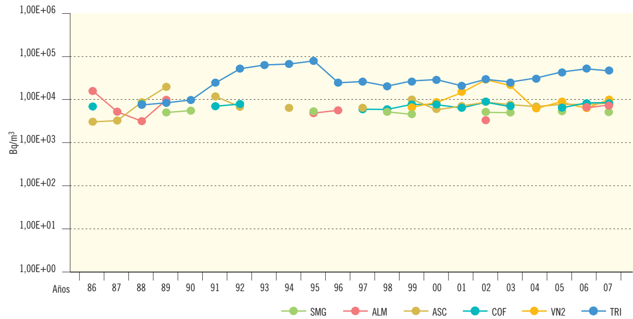
Figura 2.22b. Agua potable. Concentración de actividad de H-3 (Bq/m³)
