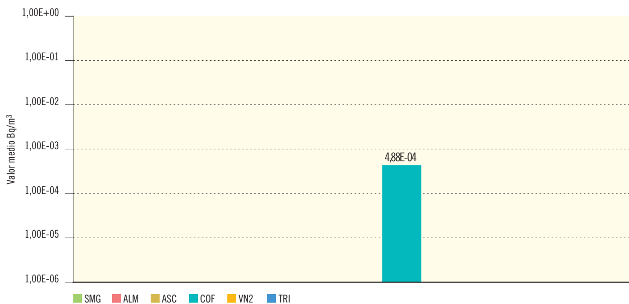
Figura 2.9b. Radioyodos en aire. Concentración de actividad I-131 (Bq/m³)
