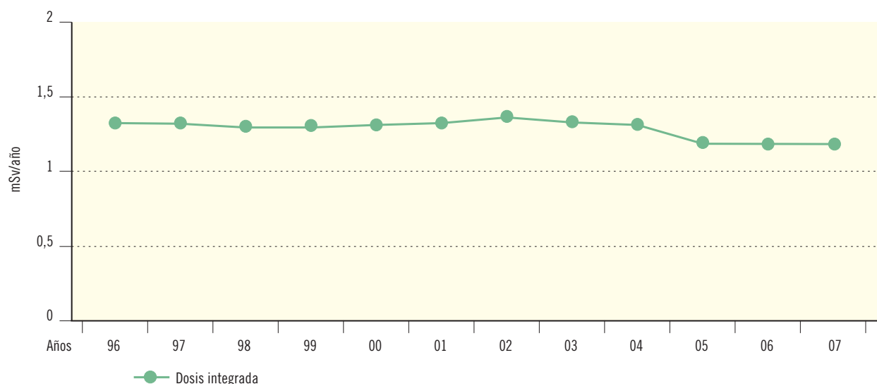
Figura 2.41. Juzbado. Radiación directa. Dosis integrada (DTL) (mSv/año) Evolución temporal valores medios
