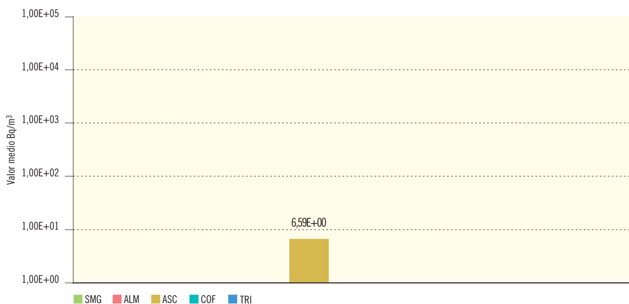
Figura 2.21b. Agua potable. Concentración de actividad de Sr-90 (Bq/m³)
