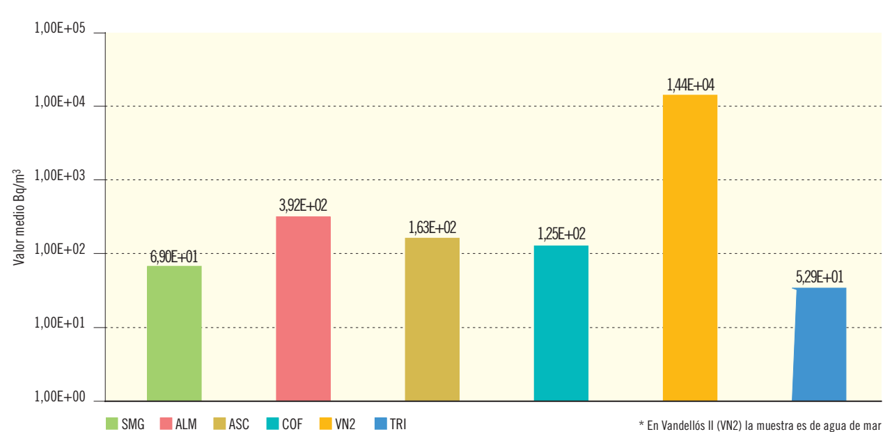
Figura 2.14b. Agua superficial. Concentración del índice de actividad beta total (Bq/m³)
