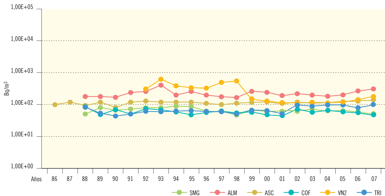
Figura 2.19b. Agua potable. Concentración del índice de actividad beta total (Bq/m³)
