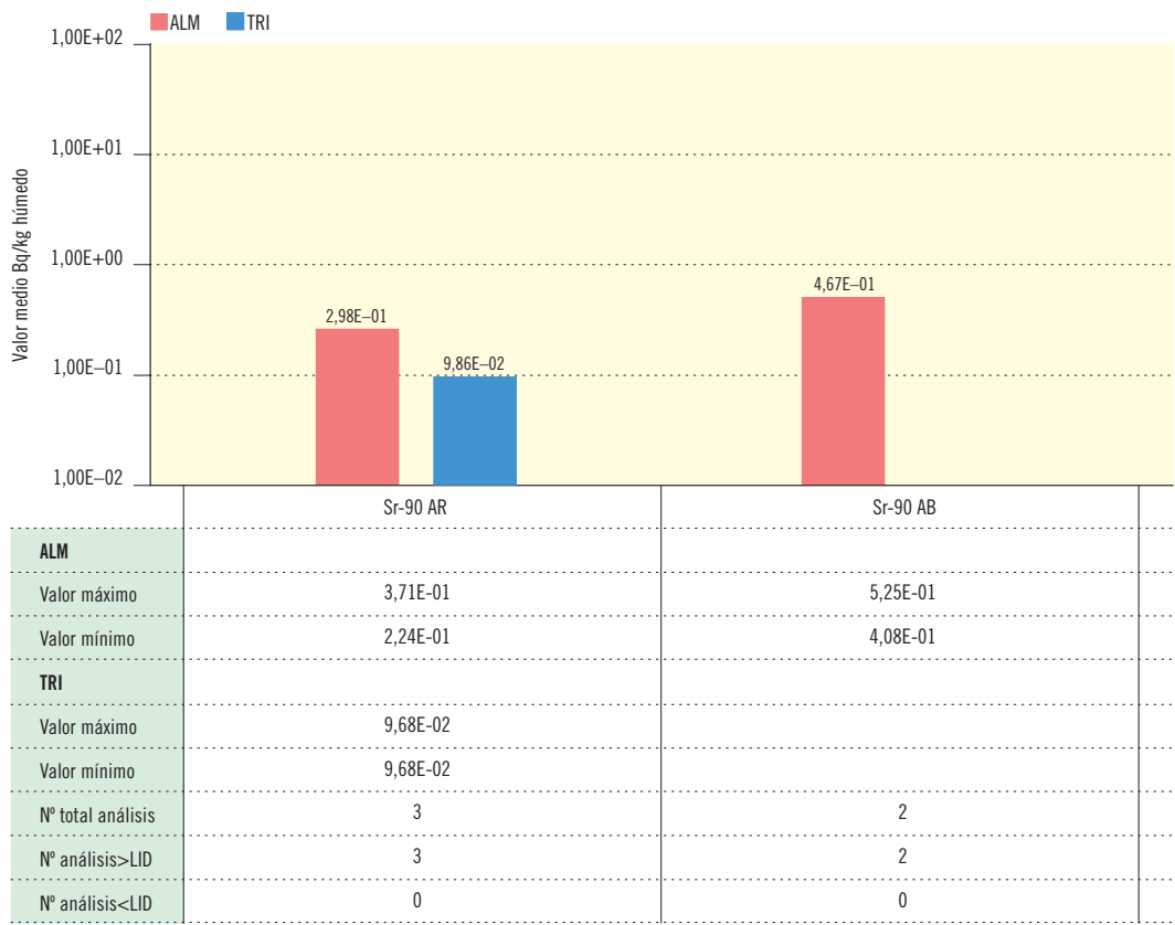
Figura 2.25b. Plantas terrestres. Concentración de actividad (Bq/kg húmedo) Valores de la campaña de 2014
