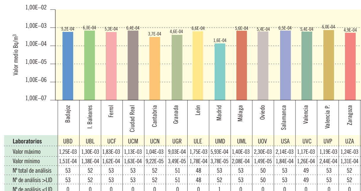
Figura 3.3b. Partículas de polvo en aire. Concentración del índice de actividad beta total (Bq/m³)
