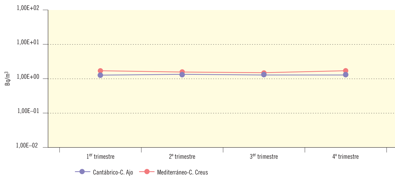
Figura 3.67b. Red de alta sensibilidad. Agua de mar. Concentración de actividad de Cs-137 (Bq/m³)
