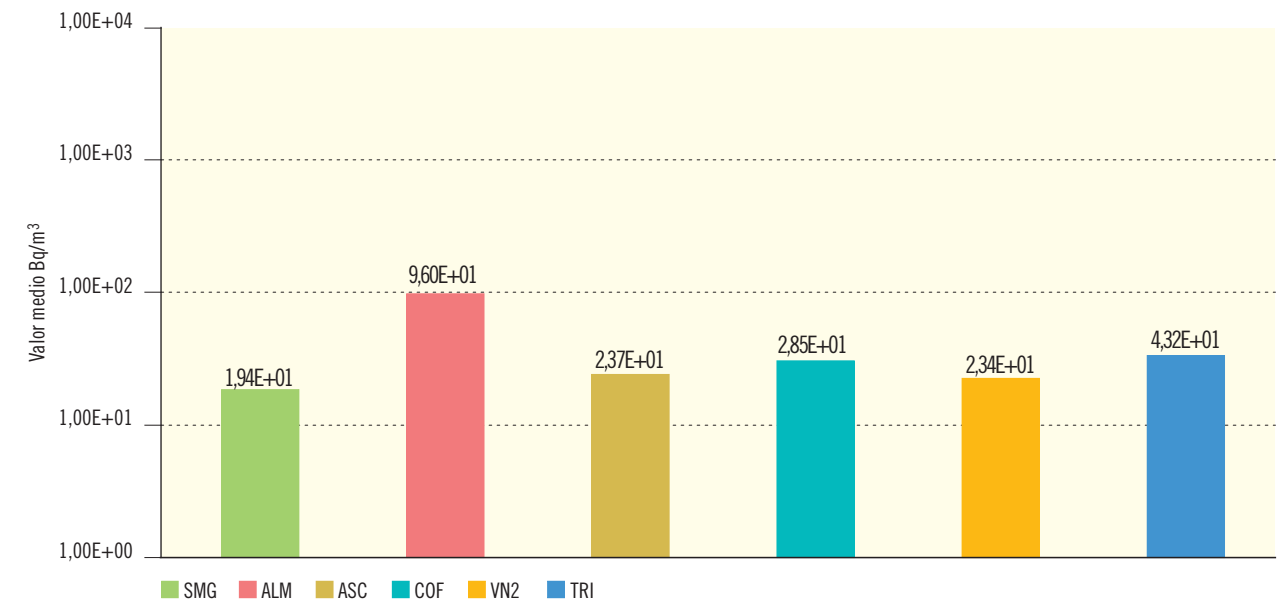
Figura 2.28b. Leche. Concentración de actividad de Sr-90 (Bq/m³)
