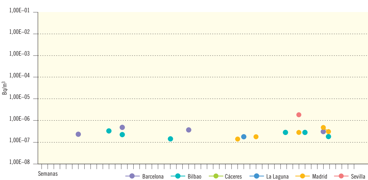
Figura 3.5b. Red de alta sensibilidad. Partículas de polvo en aire. Muestreador de alto flujo
