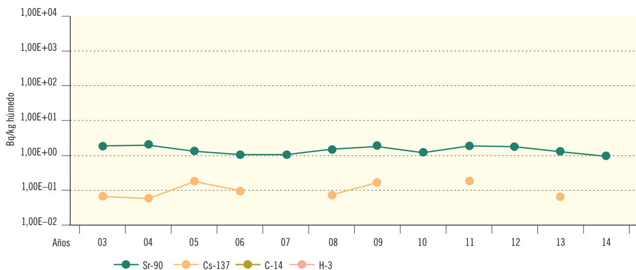
Figura 2.53. El Cabril. Plantas terrestres. Valores de concentración de actividad (Bq/kg húmedo)
