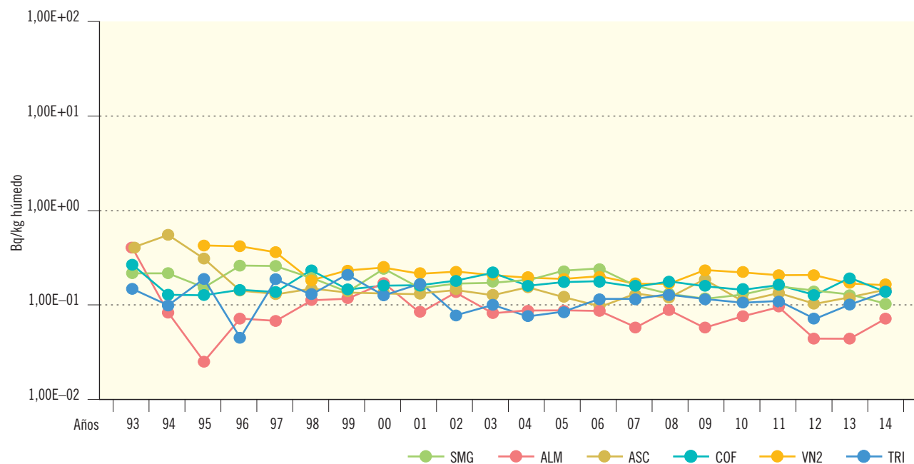
Figura 2.31b. Vegetales de hoja no ancha. Concentración de actividad de Sr-90 (Bq/kg húmedo)
