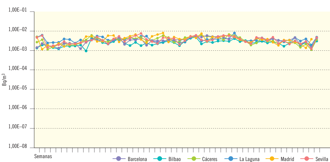
Figura 3.6b. Red de alta sensibilidad. Partículas de polvo en aire. Muestreador de alto flujo
