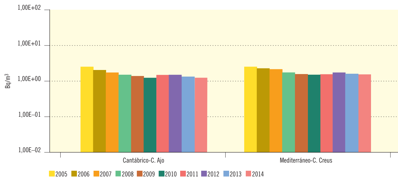
Figura 3.67a. Red de alta sensibilidad. Agua de mar
