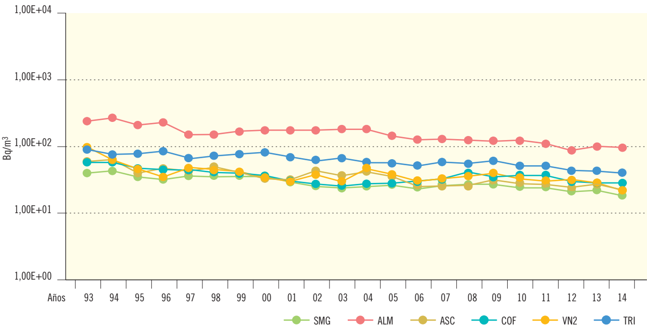
Figura 2.28b. Leche. Concentración de actividad de Sr-90 (Bq/m³)
