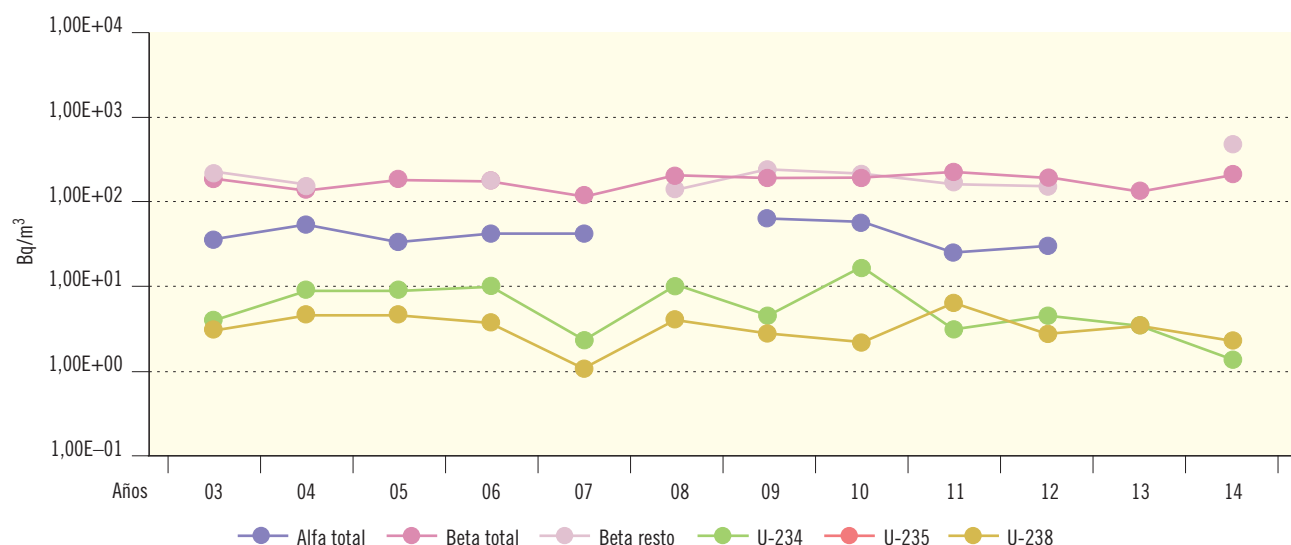
Figura 2.43. Juzbado. Agua potable. Valores de concentración de actividad ( \text{Bq/m}^3 )
