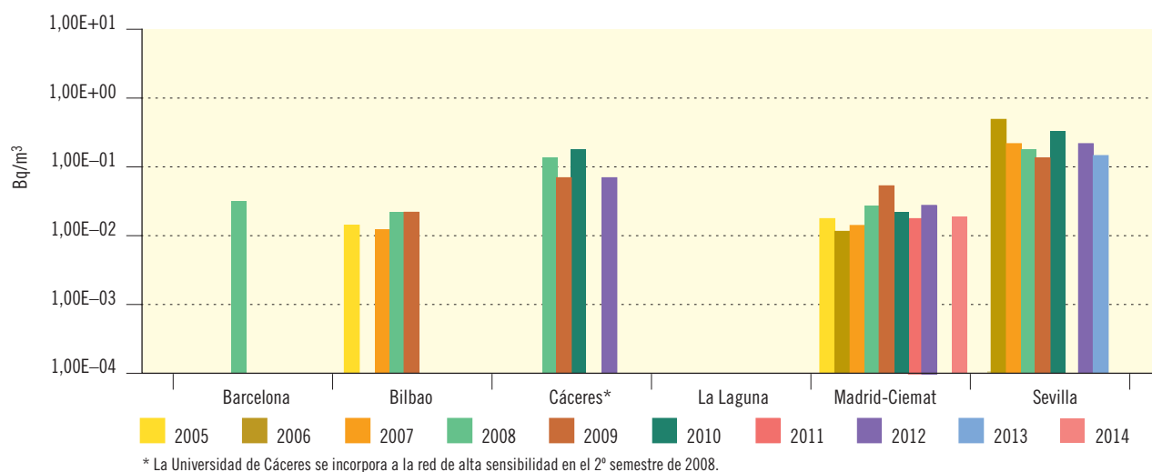
Figura 3.15b. Red de alta sensibilidad. Agua potable. Concentración de actividad de Cs-137 (Bq/m³)
