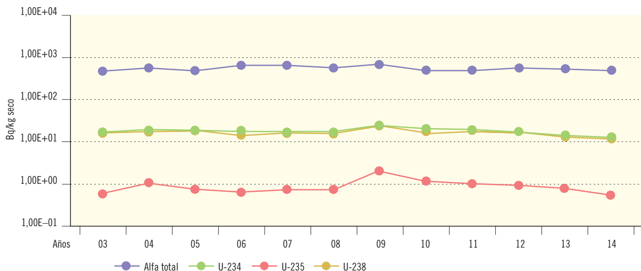
Figura 2.39. Juzbado. Suelo. Valores de concentración de actividad (Bq/kg seco)
