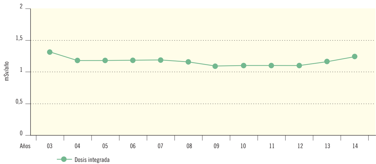
Figura 2.38. El Cabril. Radiación directa. Dosis integrada (DTL) (mSv/año)
