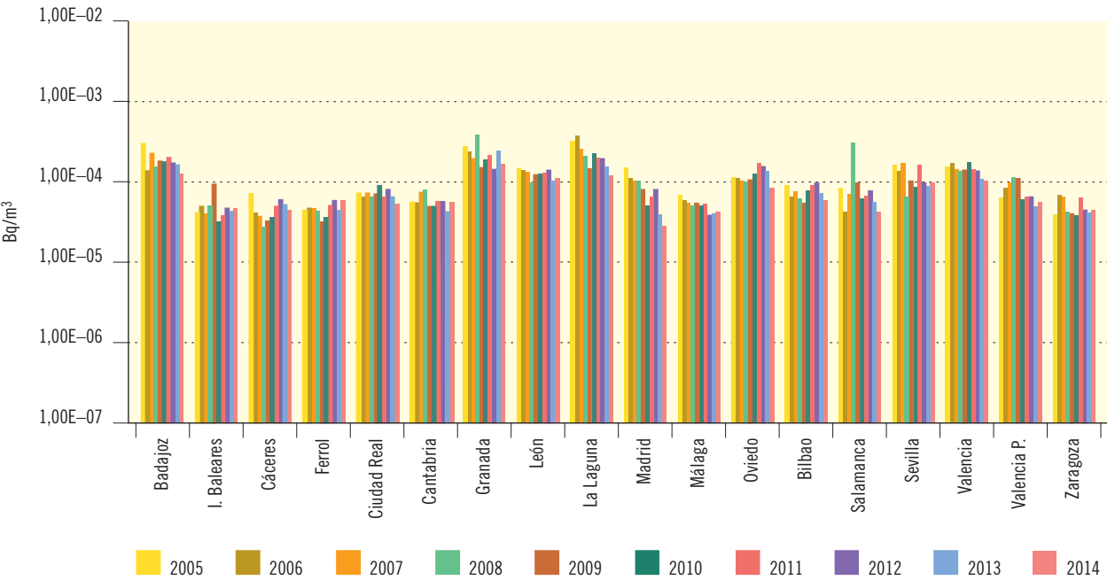
Figura 3.2a. Partículas de polvo en aire
