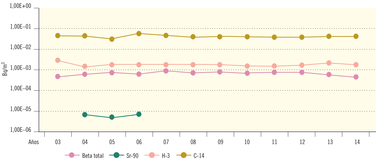
Figura 2.36. El Cabril. Partículas de polvo en aire. Valores de concentración de actividad (Bq/m³)
