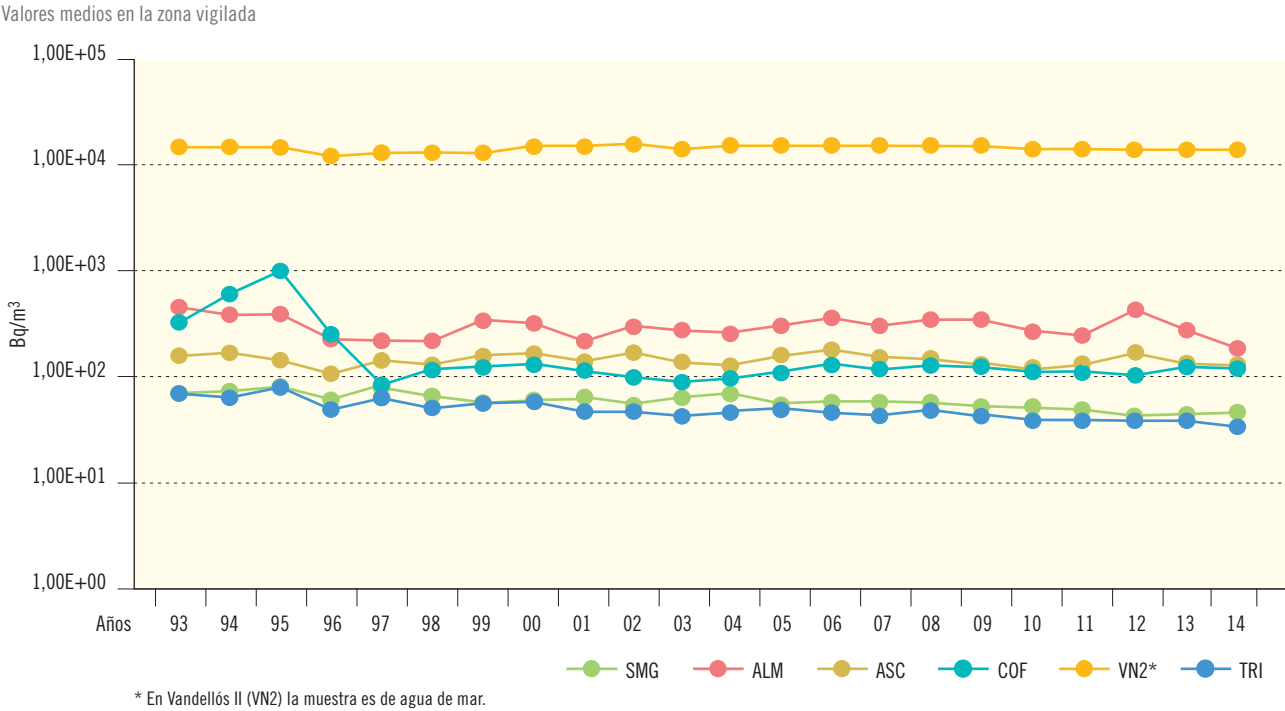
Figura 2.12a. Agua superficial. Evolución temporal del índice de actividad beta total
