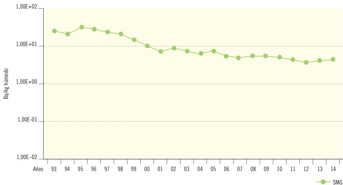
Figura 2.27b. Fauna terrestre. Concentración de actividad (Bq/kg húmedo)
