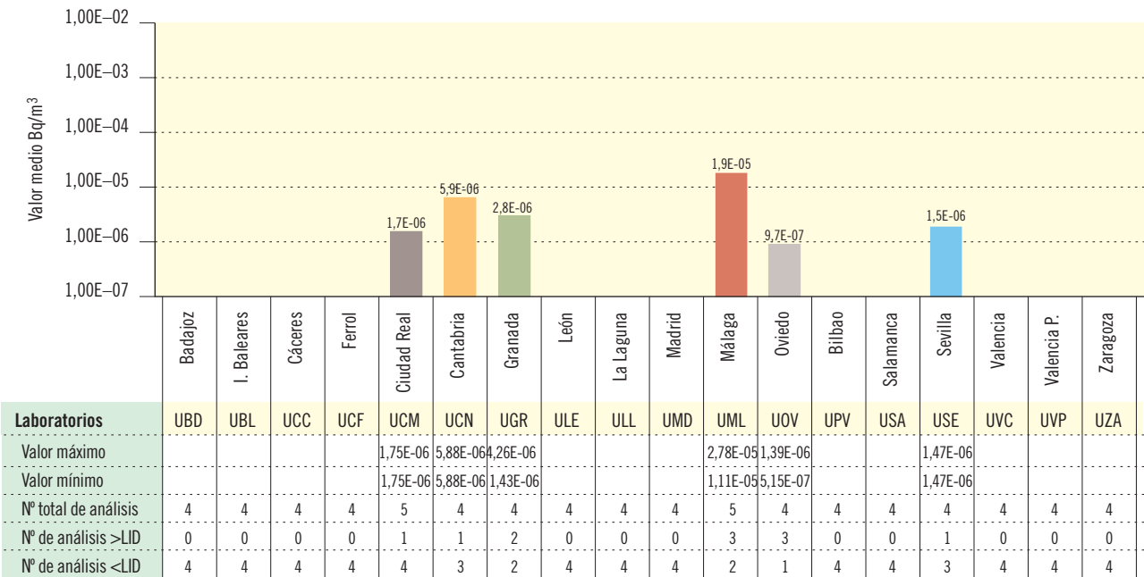
Figura 3.4b. Partículas de polvo en aire. Concentración de actividad de Sr-90 (Bq/m³)
