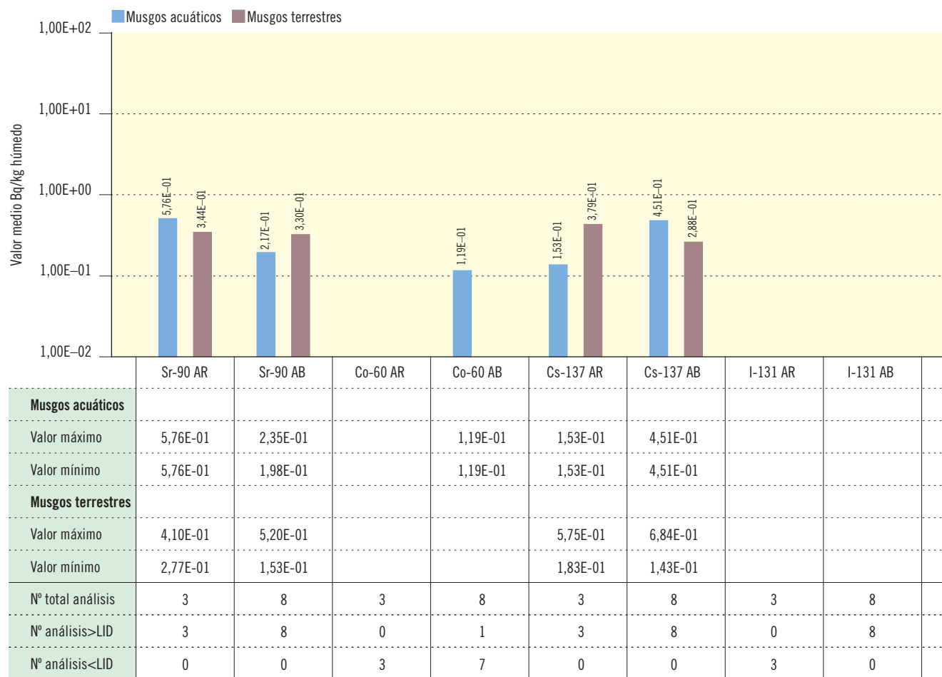
Figura 2.26b. Musgos. Central nuclear Santa María de Garoña. Concentración de actividad (Bq/kg húmedo)
