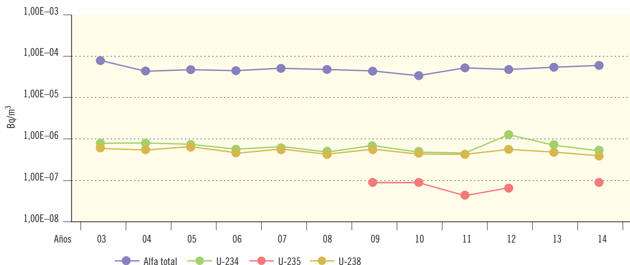
Figura 2.35. Juzbado. Partículas de polvo en aire. Valores de concentración de actividad (Bq/m 3 )
