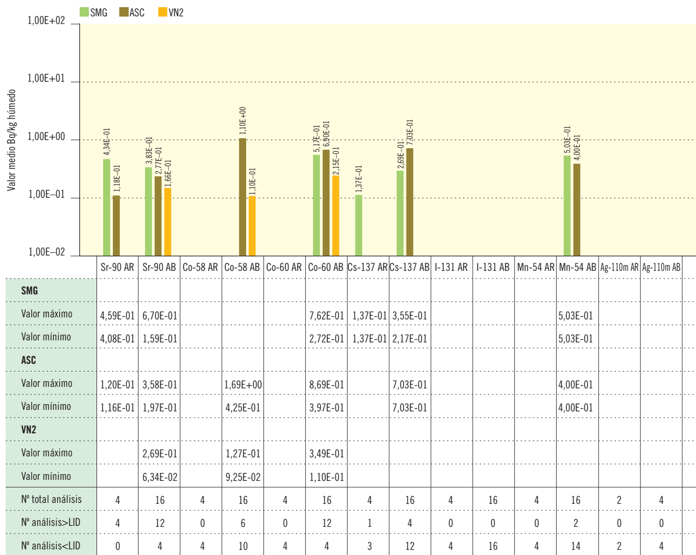
Figura 2.23b. Plantas acuáticas. Concentración de actividad (Bq/kg húmedo)
