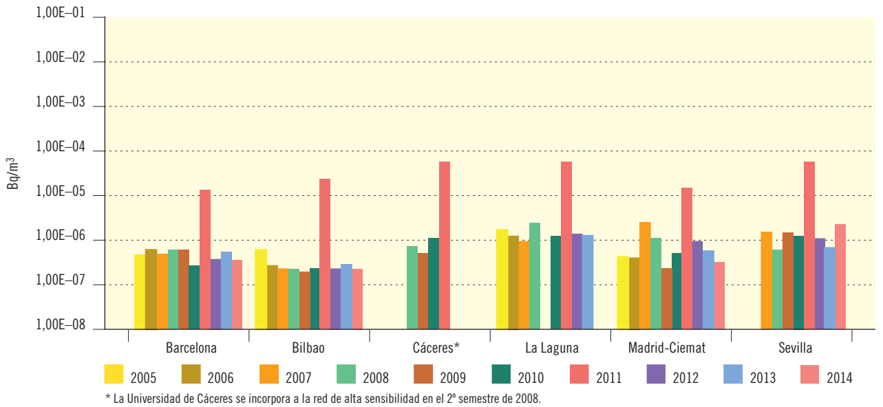
Figura 3.5b. Red de alta sensibilidad. Partículas de polvo en aire. Muestreador de alto flujo
