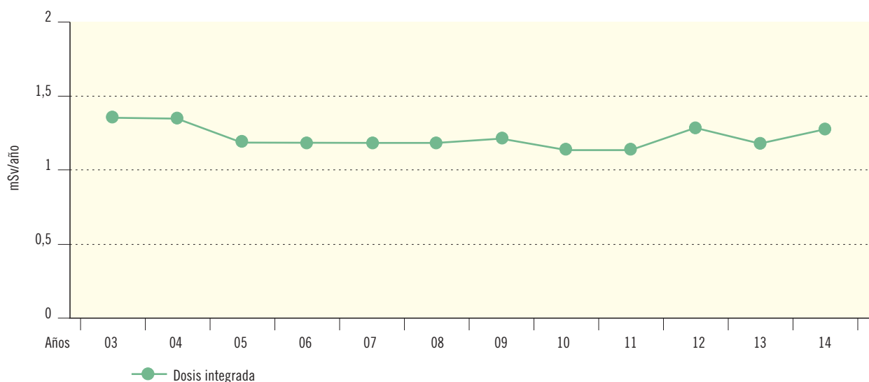
Figura 2.37. Juzbado. Radiación directa. Dosis integrada (DTL) (mSv/año)
