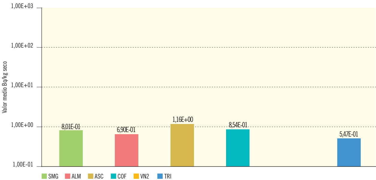
Figura 2.19b. Sedimentos de fondo. Concentración de actividad de Sr-90 (Bq/kg seco)
