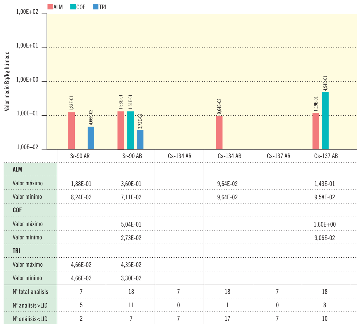
Figura 2.24b. Plantas de orilla. Concentración de actividad (Bq/kg húmedo)
