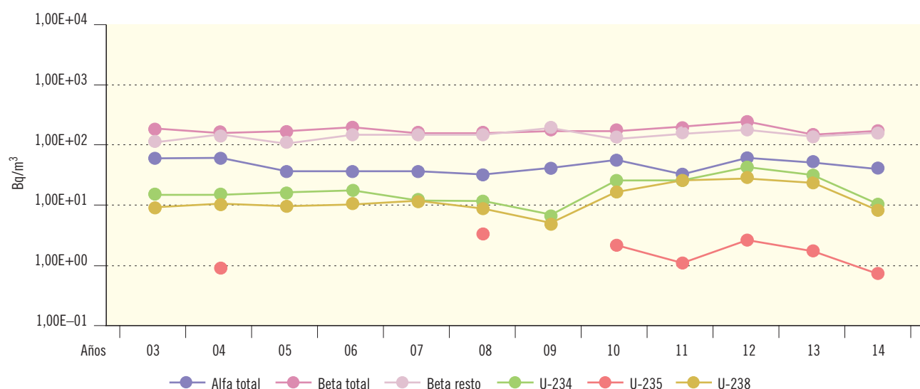
Figura 2.41. Juzbado. Agua superficial. Valores de concentración de actividad (Bq/m 3 )
