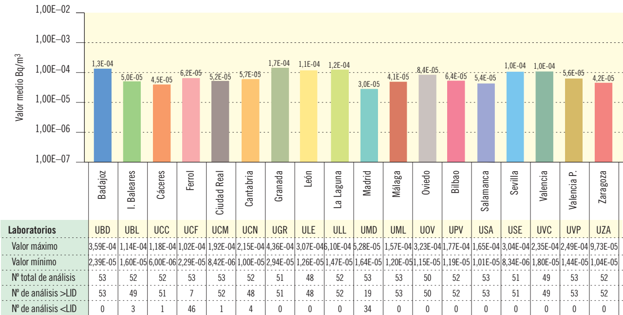
Figura 3.2b. Partículas de polvo en aire. Concentración del índice de actividad alfa total (Bq/m³)
