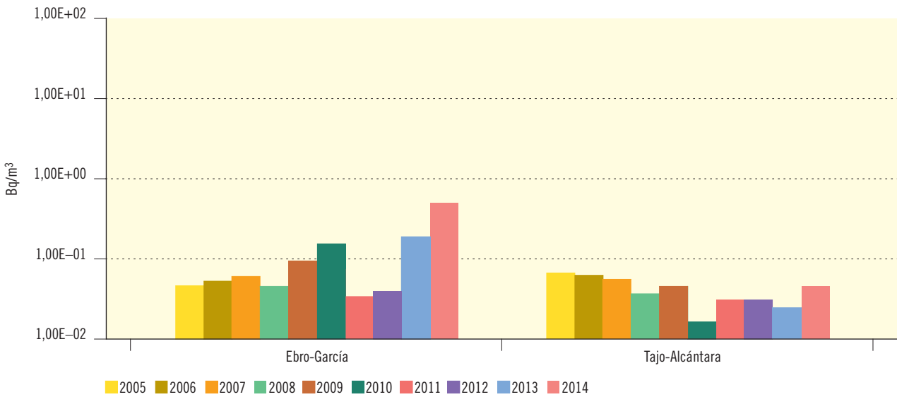
Figura 3.62b. Red de alta sensibilidad. Agua superficial. Concentración de actividad Cs-137 (Bq/m³)
