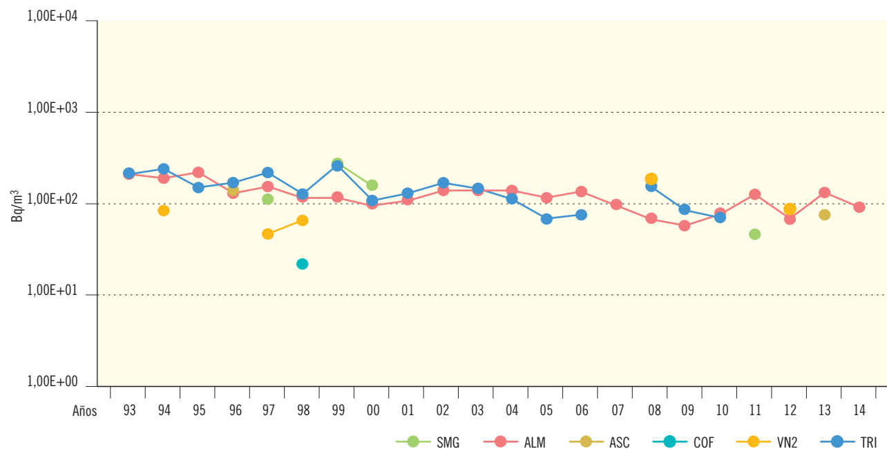
Figura 2.29b. Leche. Concentración de actividad de Cs-137 (Bq/m³)
