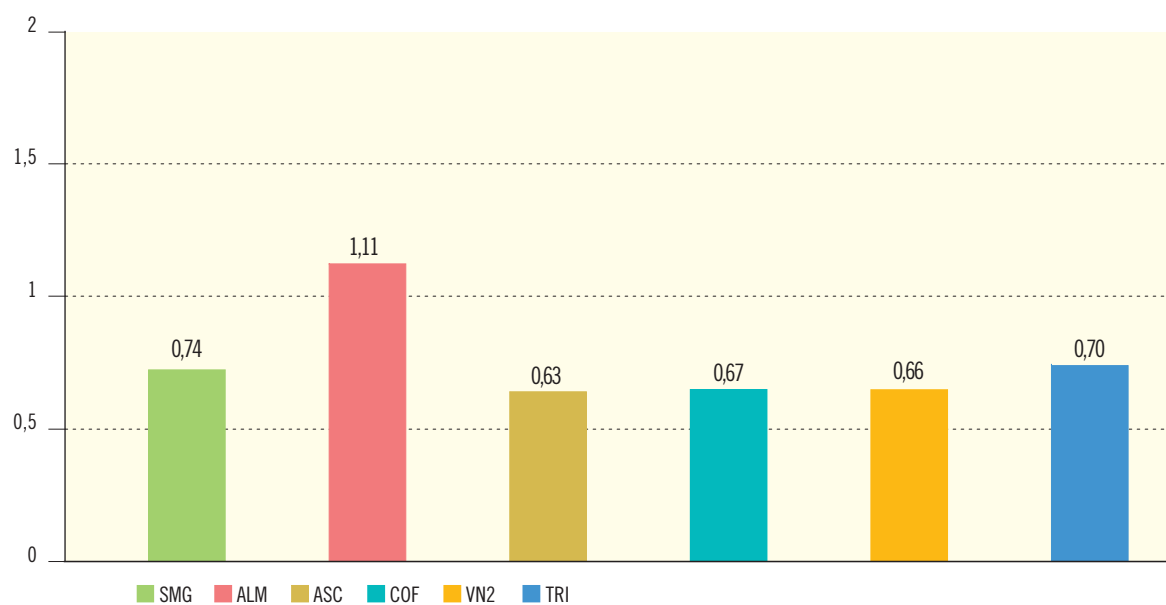
Figura 2.9b. Radiación directa. Dosis integrada (DTL) (mSv/año)
