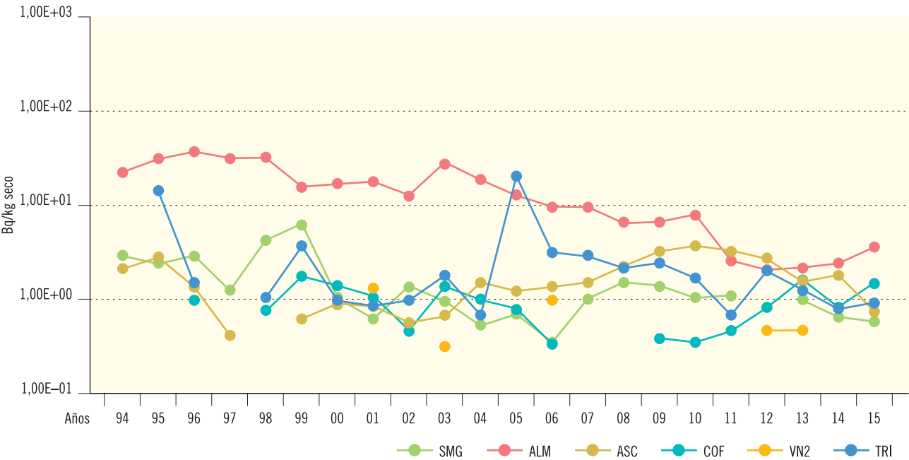
Figura 2.20b. Sedimentos de fondo. Concentración de actividad de Co-60 (Bq/kg seco) Valores de la campaña de 2015
