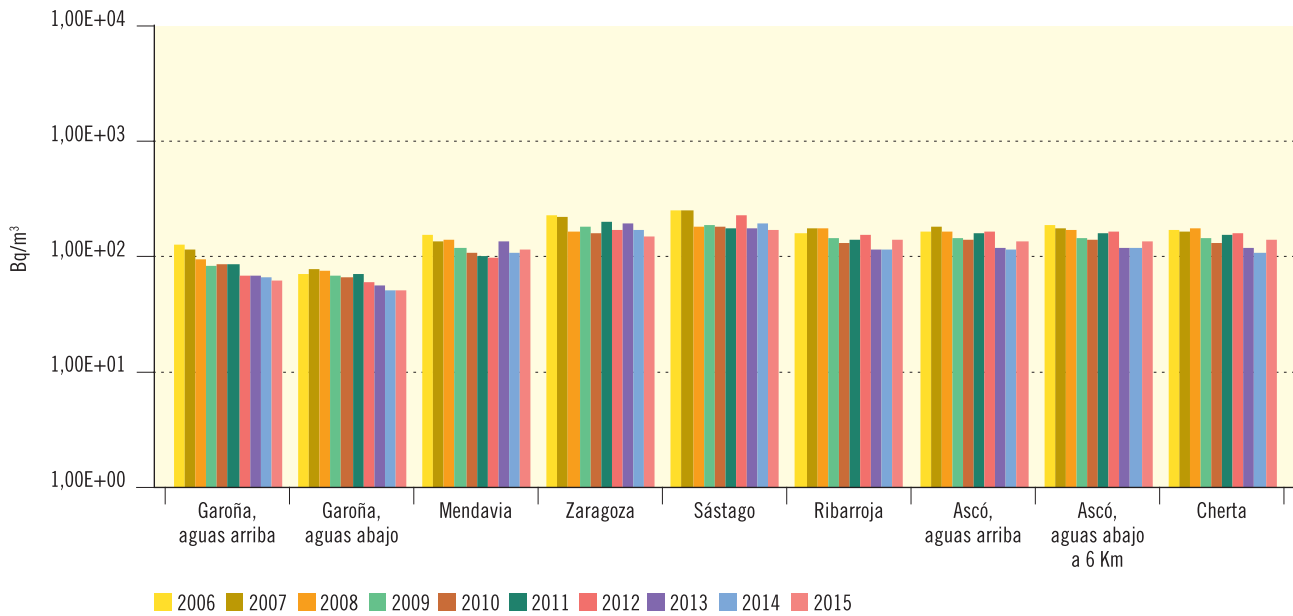
Figura 3.55. Río Ebro
