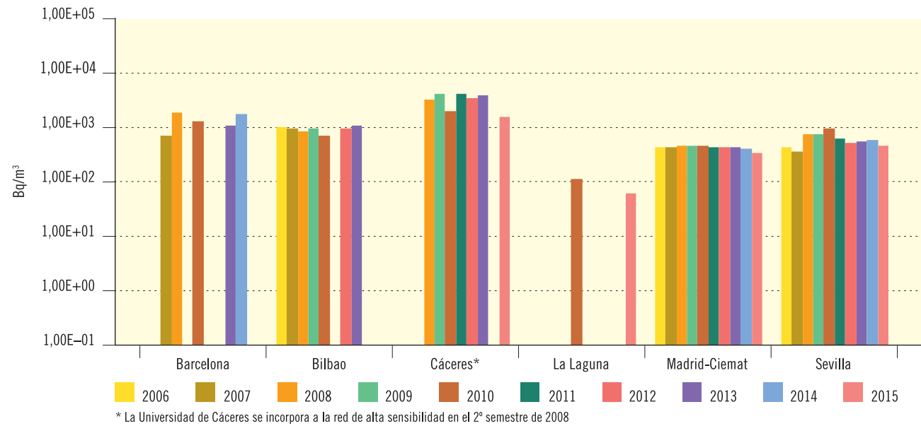
Figura 3.14b. Red de alta sensibilidad. Agua potable. Concentración de actividad de H-3 (Bq/m³)
