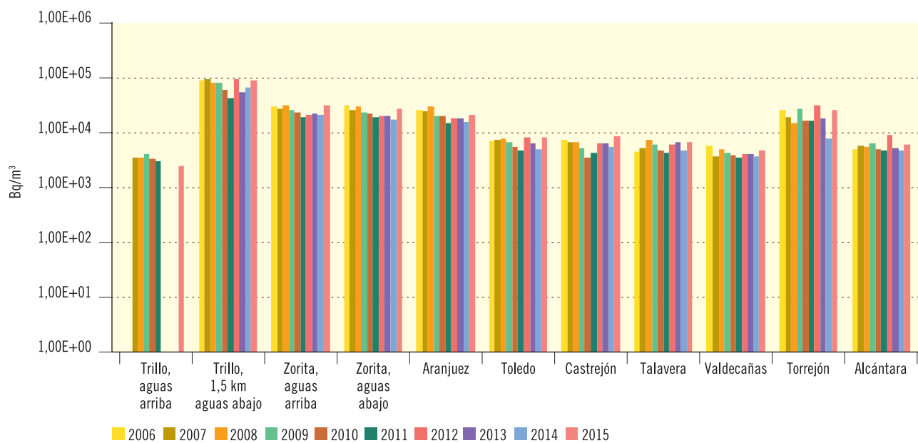
Figura 3.37. Río Tajo
