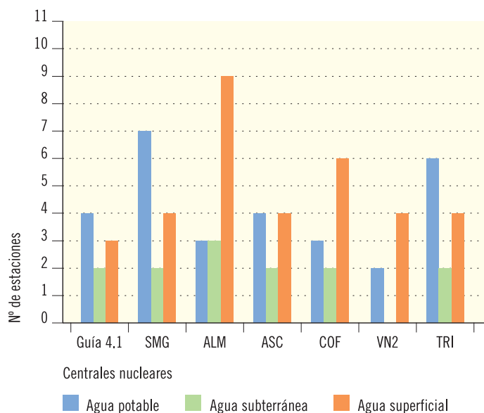
Figura 2.5. Número de estaciones de muestreo en los PVRA de las centrales nucleares. Año 2015
