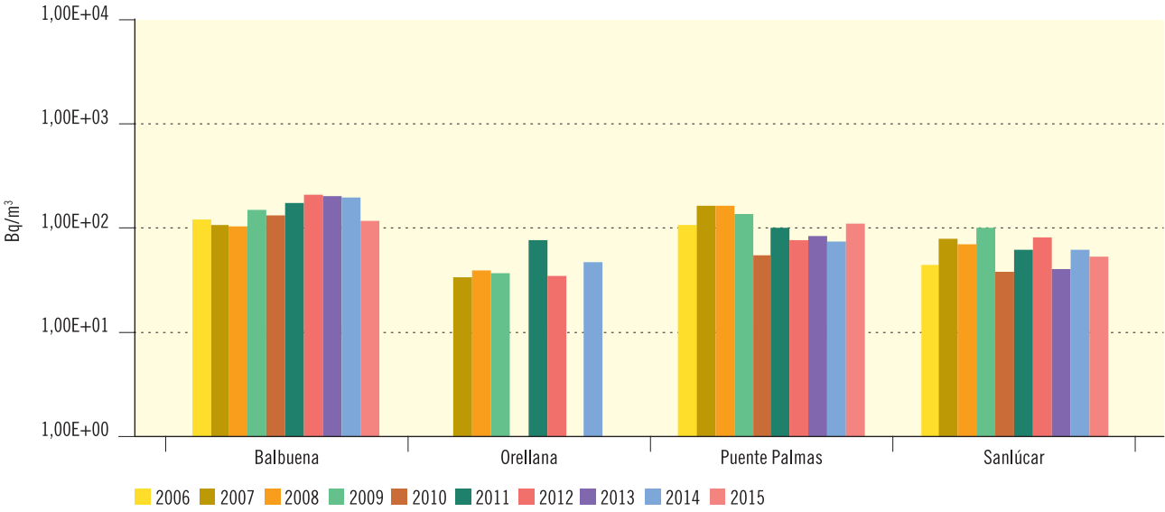
Figura 3.38. Río Guadiana
