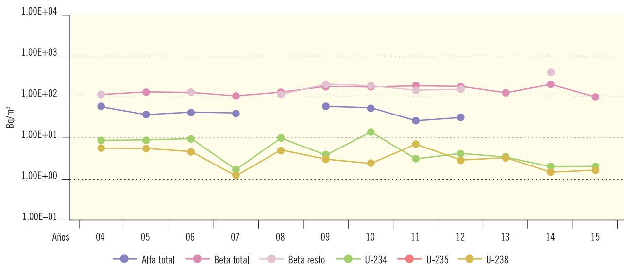
Figura 2.42. Juzbado. Agua potable. Valores de concentración de actividad (Bq/m 3 )
