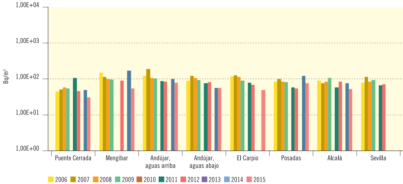
Figura 3.42. Río Guadalquivir
