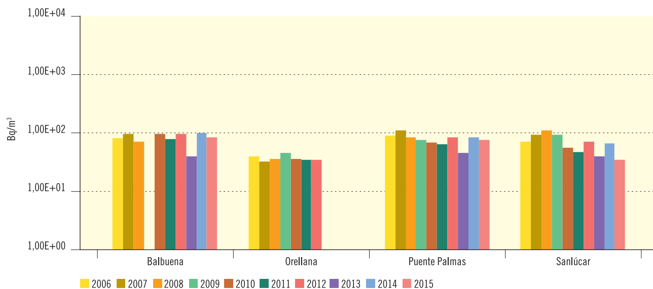
Figura 3.40. Río Guadiana
