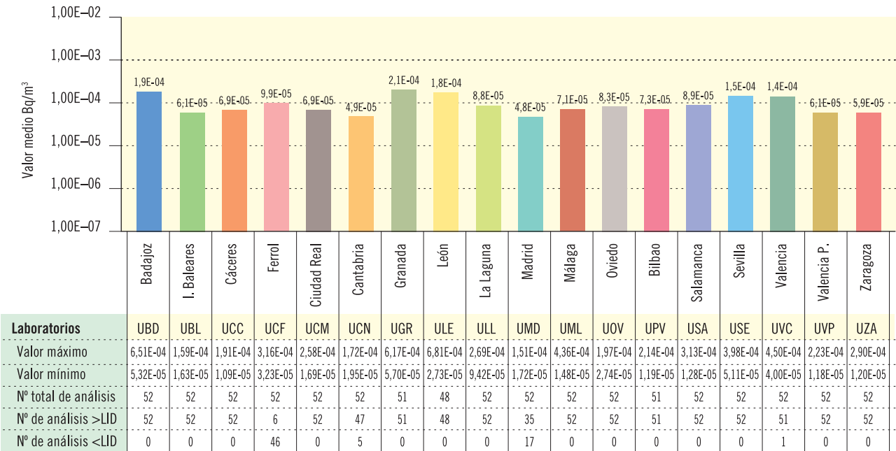
Figura 3.2b. Partículas de polvo en aire. Concentración del índice de actividad alfa total (Bq/m³) Valores de la campaña de 2015
