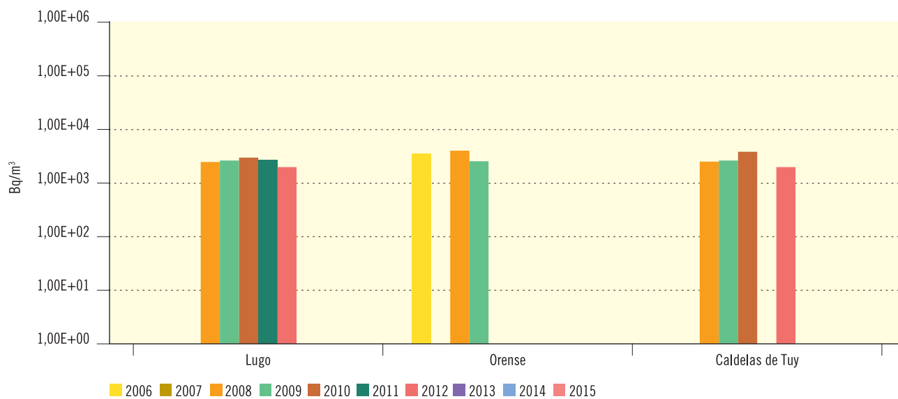
Figura 3.29. Río Miño
