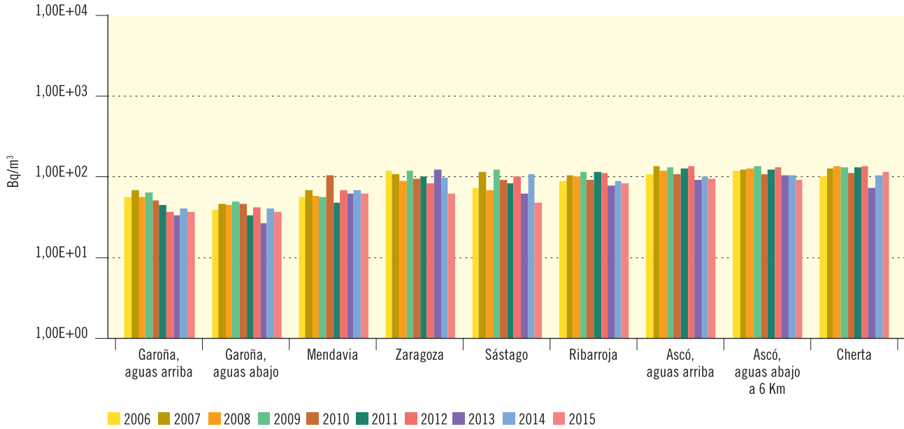
Figura 3.54. Río Ebro
