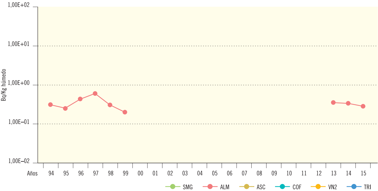
Figura 2.32b. Peces y mariscos. Concentración de actividad de Cs-134 (Bq/kg húmedo)
