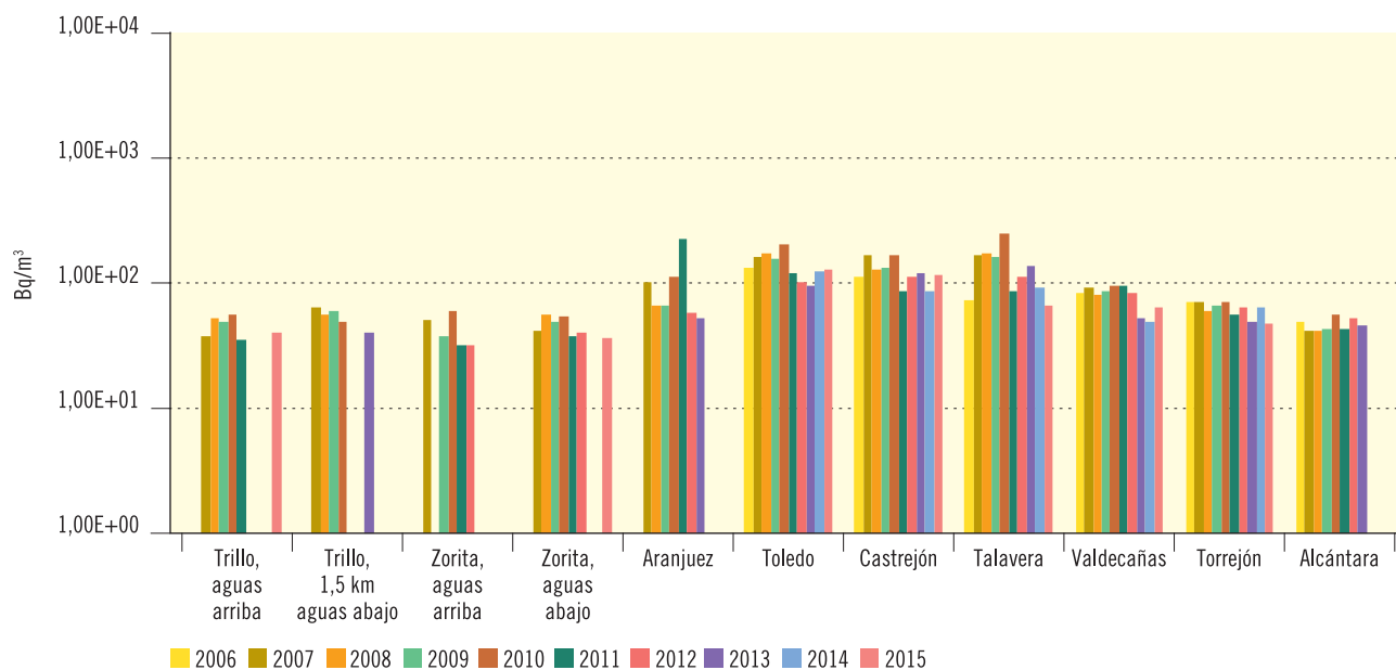
Figura 3.36. Río Tajo
