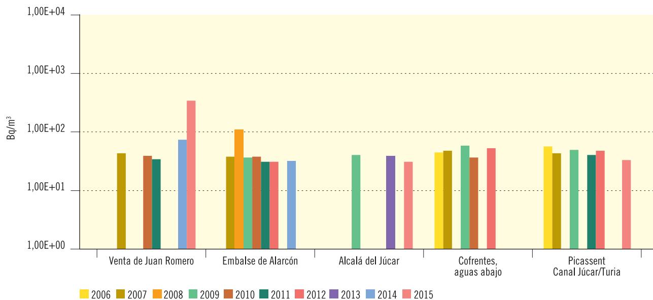
Figura 3.52. Río Júcar
