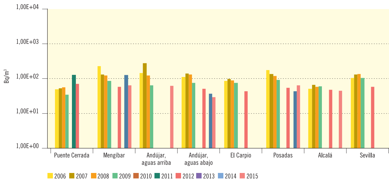
Figura 3.44. Río Guadalquivir
