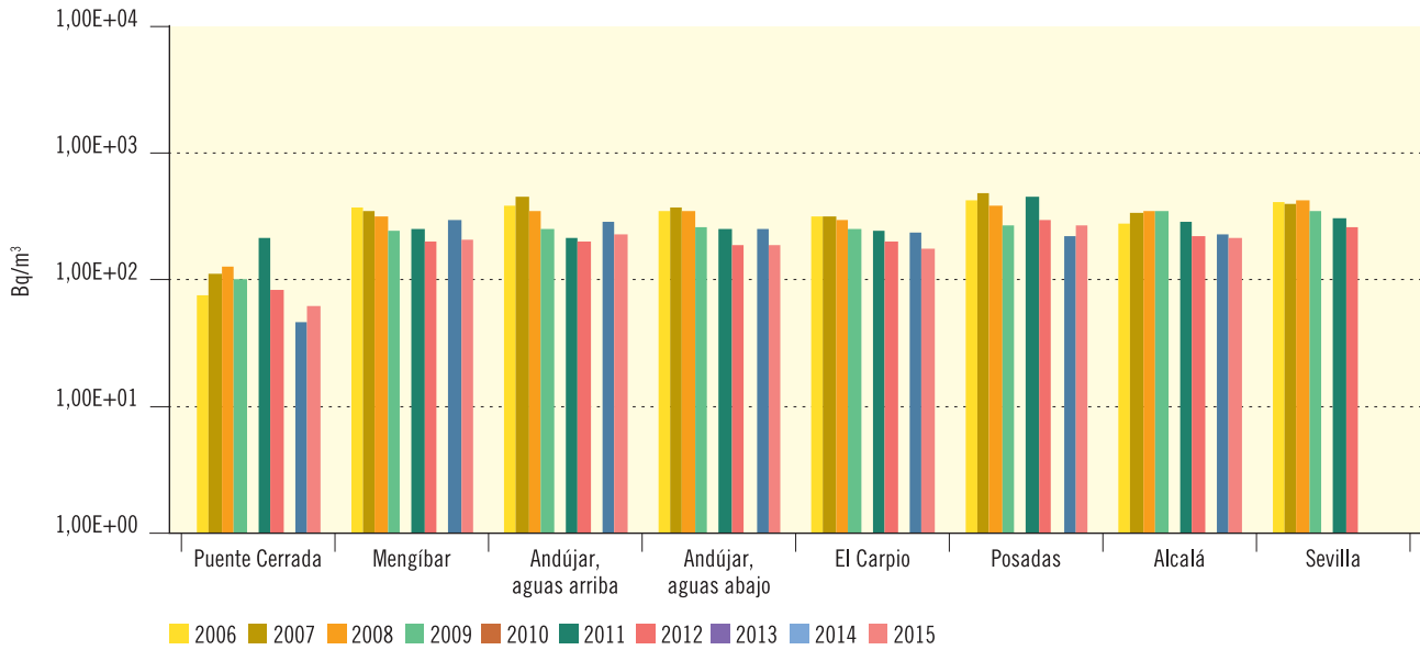
Figura 3.43. Río Guadalquivir
