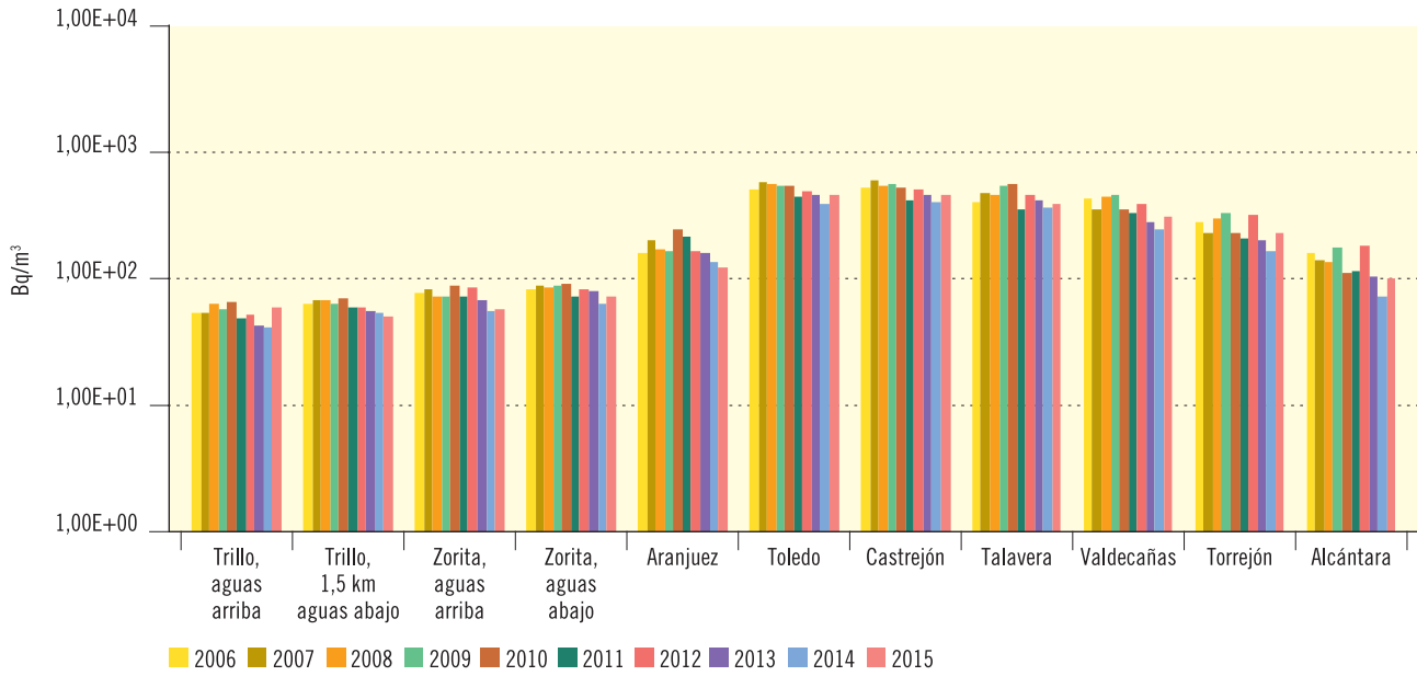
Figura 3.35. Río Tajo
