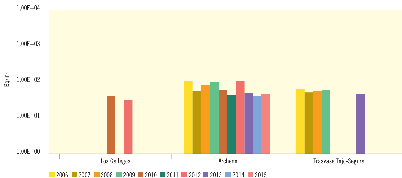
Figura 3.49. Río Segura
