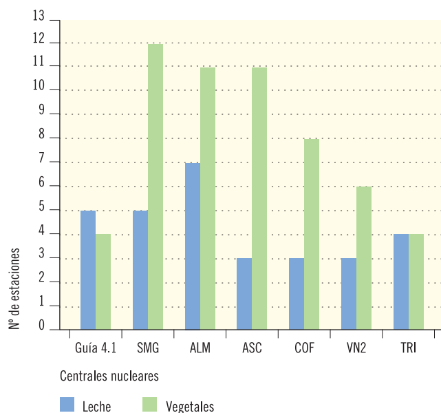
Figura 2.7. Número de estaciones de muestreo en los PVRA de las centrales nucleares. Año 2015
