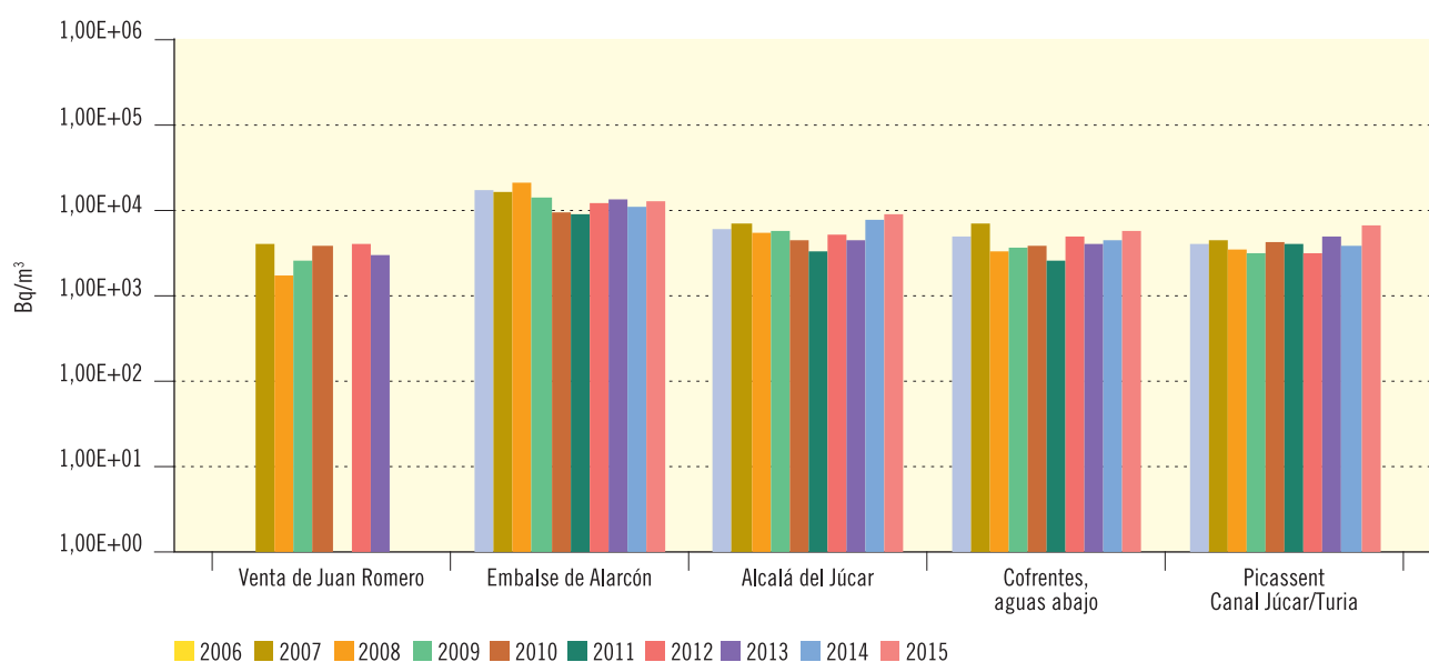
Figura 3.53. Río Júcar
