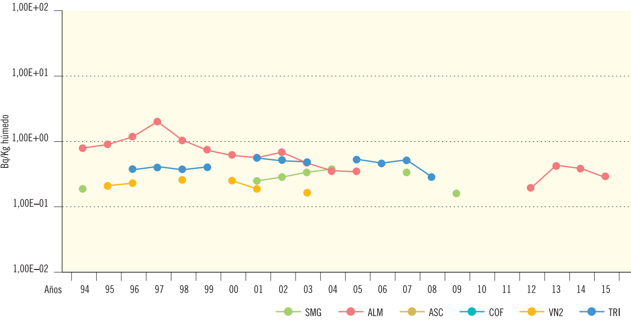
Figura 2.31b. Peces y mariscos. Concentración de actividad de Cs-137 (Bq/kg húmedo)
