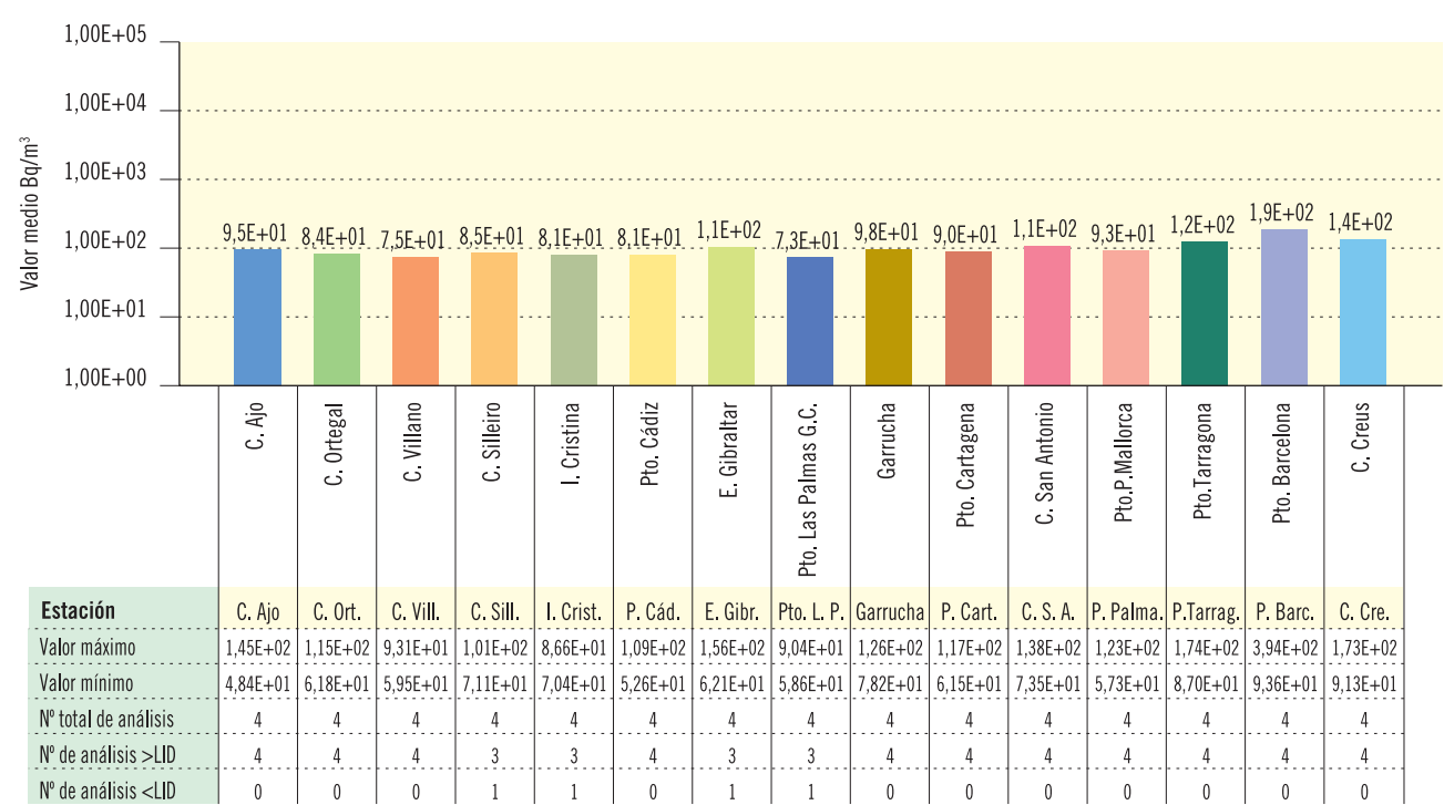
Figura 3.66b. Agua de mar. Concentración de actividad de H-3 (Bq/m³)
