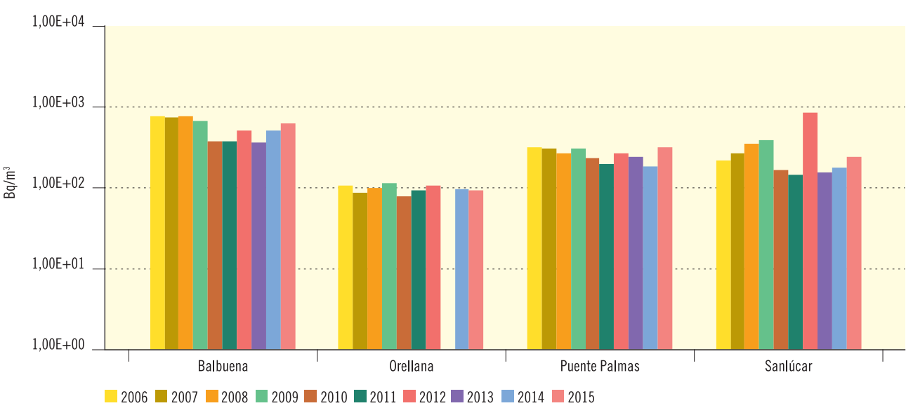
Figura 3.39. Río Guadiana
