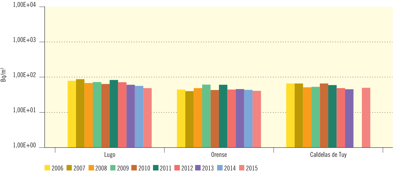
Figura 3.27. Río Miño Evolución temporal del índice de actividad beta total
