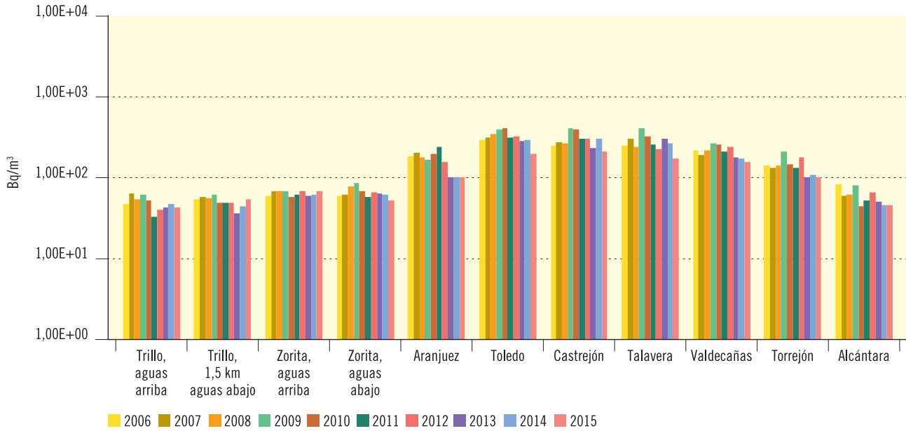
Figura 3.34. Río Tajo
