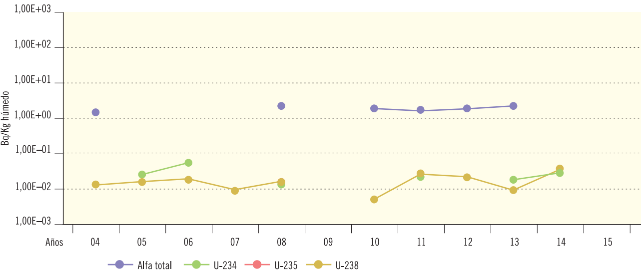
Figura 2.45. Juzbado. Carne y aves. Valores de concentración de actividad (Bq/kg húmedo) Evolución temporal valores medios
