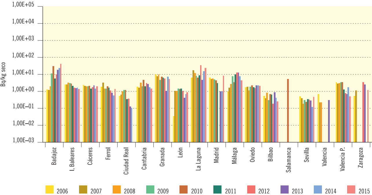
Figura 3.8a. Suelo
