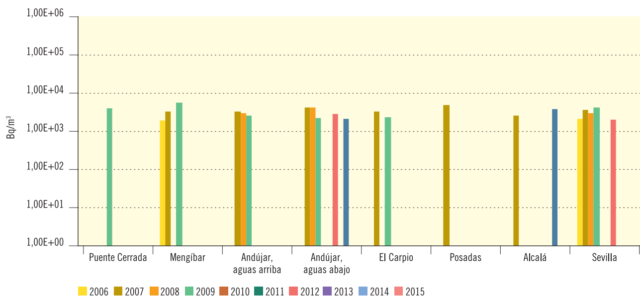
Figura 3.45. Río Guadalquivir
