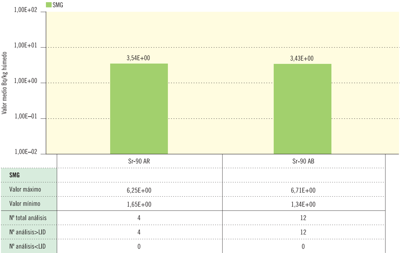
Figura 2.26b. Fauna terrestre. Concentración de actividad (Bq/kg húmedo)
