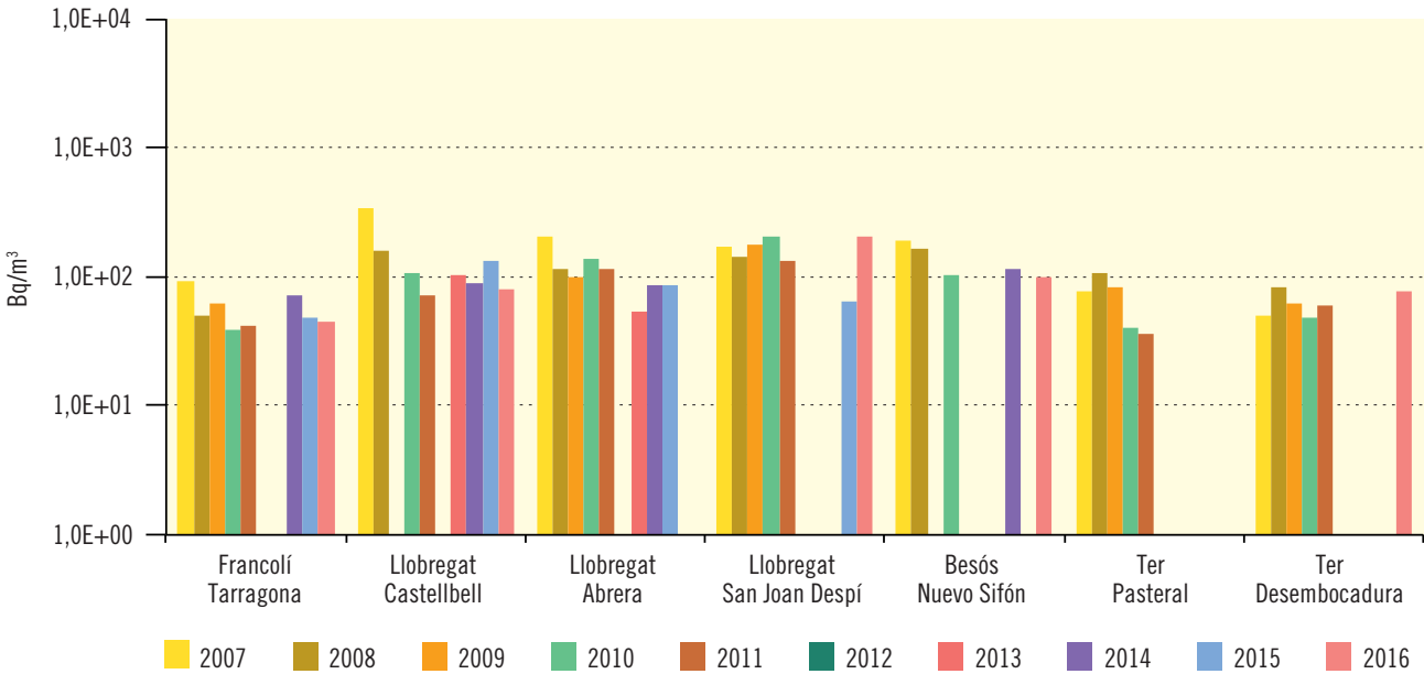
Figura 3.59. Cuencas catalanas Evolución temporal del índice de actividad beta resto
