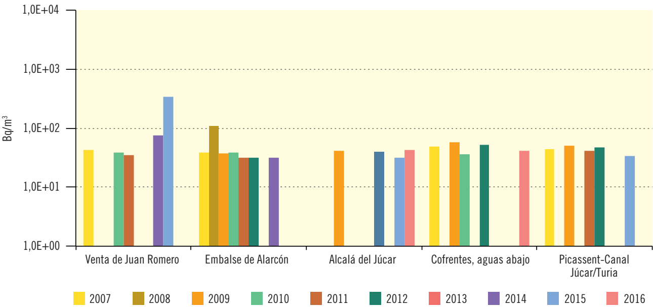
Figura 3.51. Río Júcar Evolución temporal del índice de actividad beta resto
