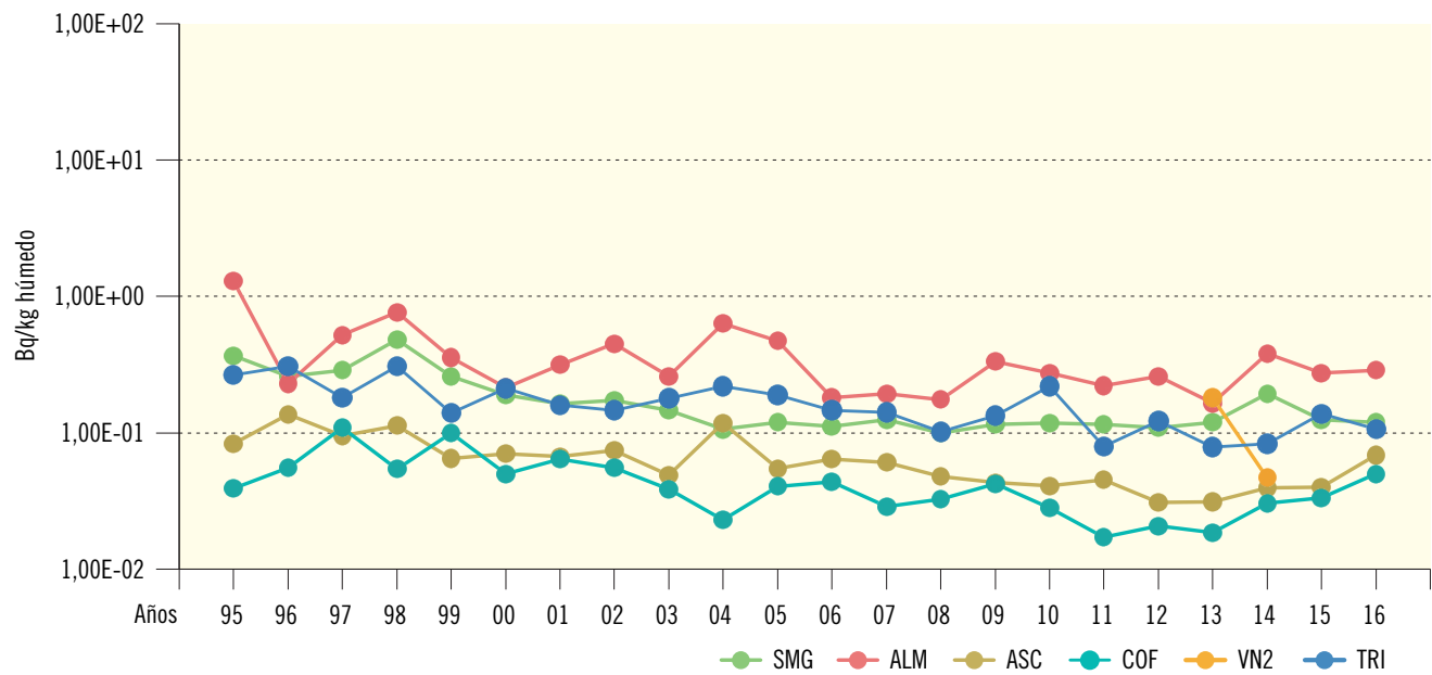
Figura 2.30a. Vegetales de hoja ancha. Evolución temporal de la concentración de actividad de Sr-90 Valores medios en la zona vigilada
