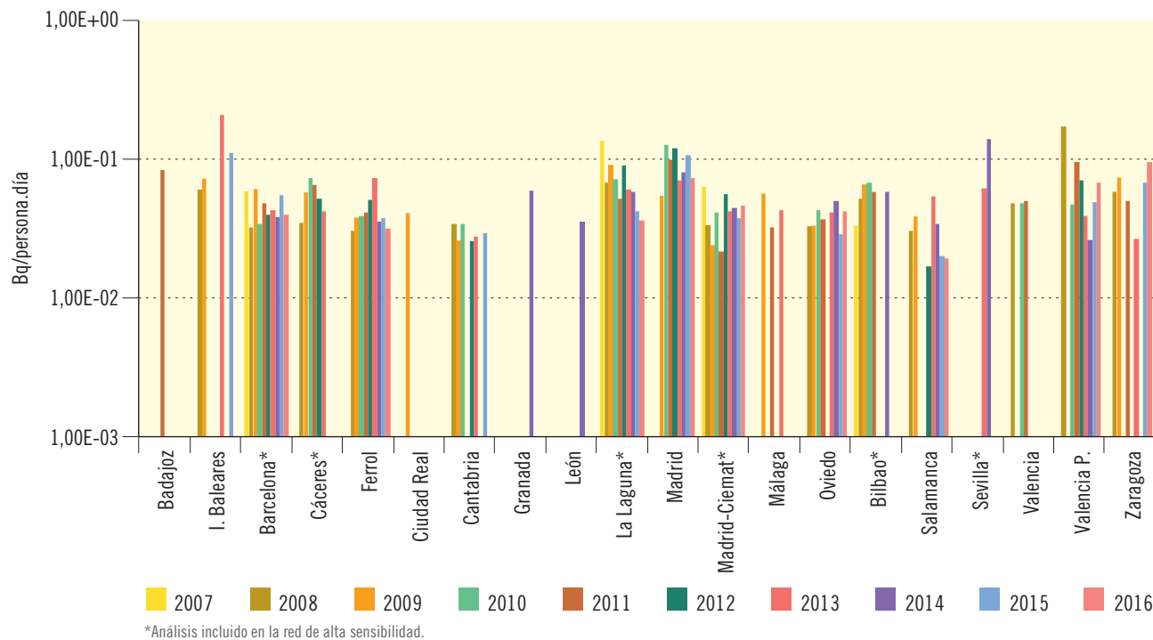
Figura 3.18b. Dieta tipo. Concentración de actividad de Cs-137 (Bq/persona.día) Valores de la campaña 2016
