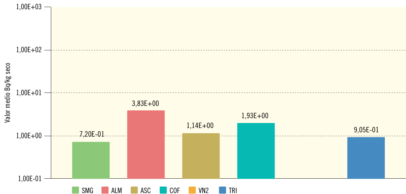
Figura 2.21b. Sedimentos de fondo. Concentración de actividad de Co-60 (Bq/kg seco) Valores de la campaña de 2016
