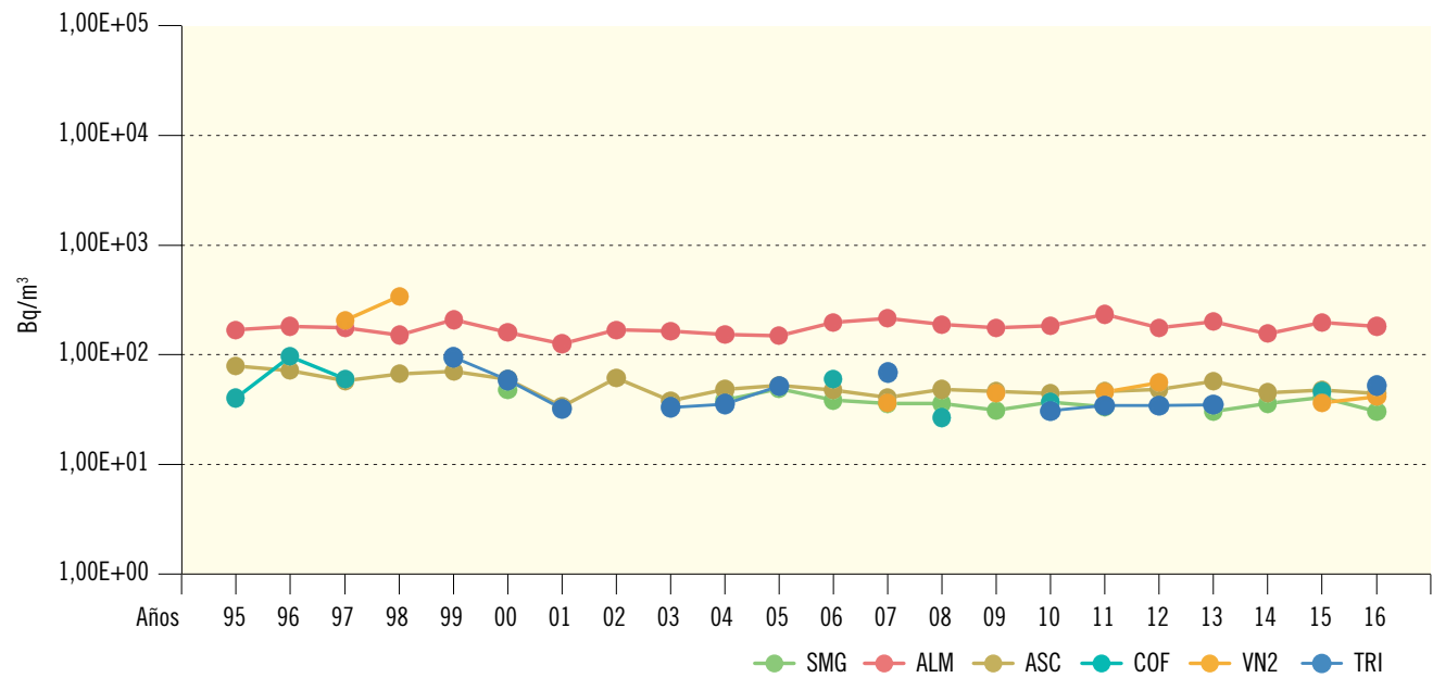
Figura 2.17a. Agua potable. Evolución temporal del índice de actividad beta resto Valores medios en la zona vigilada
