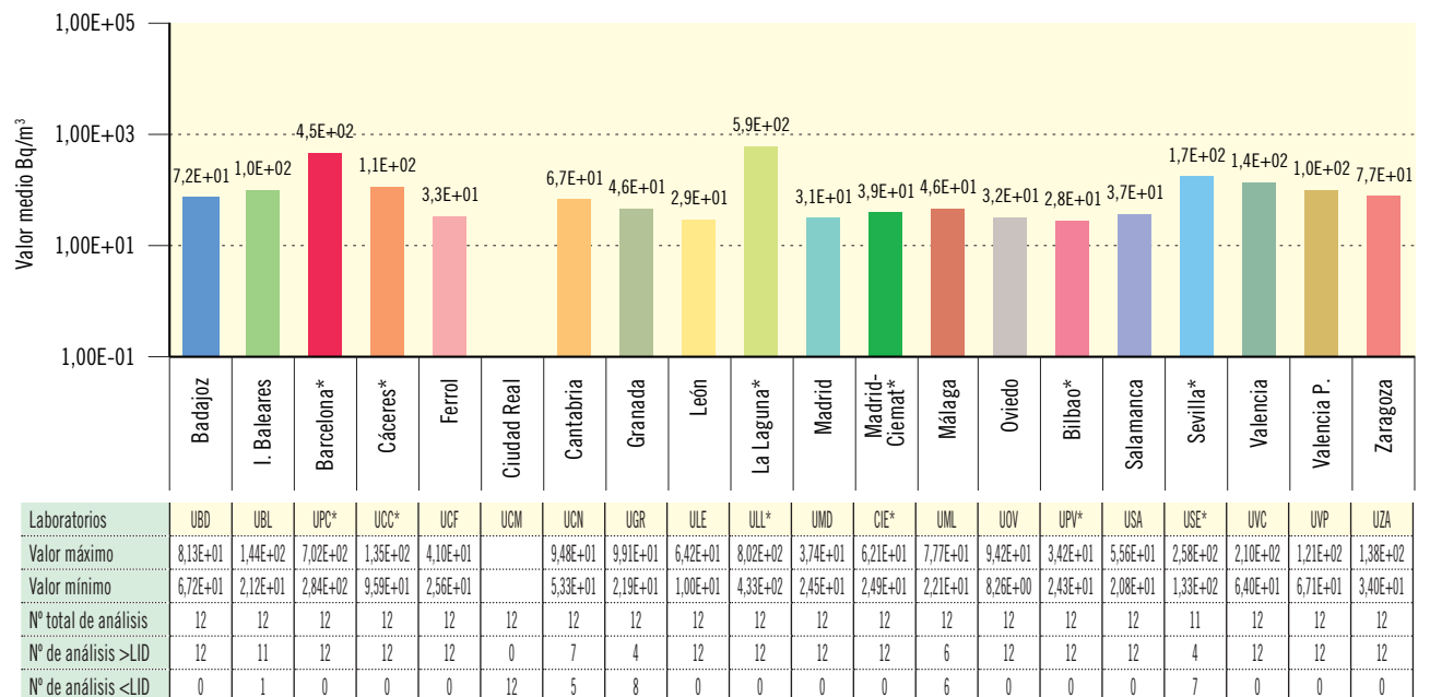
Figura 3.11b. Agua potable. Concentración del índice de actividad de beta total (Bq/m³)
