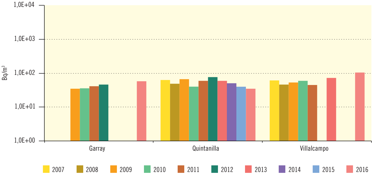
Figura 3.31. Río Duero Evolución temporal del índice de actividad beta resto
