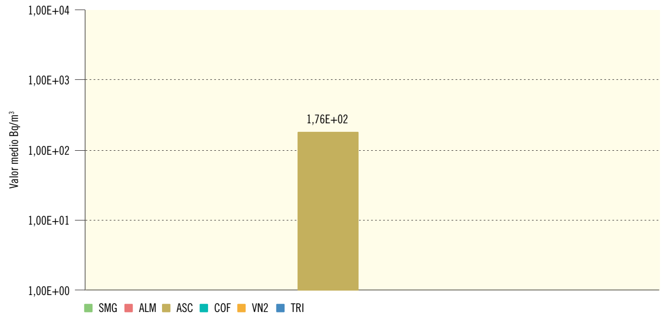
Figura 2.29b. Leche. Concentración de actividad de Cs-137 (Bq/m³) Valores de la campaña de 2016
