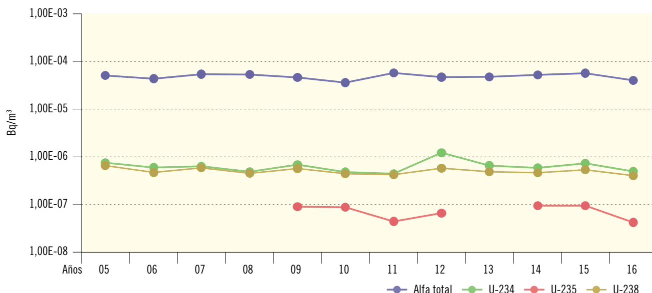
Figura 2.37. Juzbado. Partículas de polvo en aire. Valores de concentración de actividad (Bq/m 3 ) Evolución temporal valores medios
