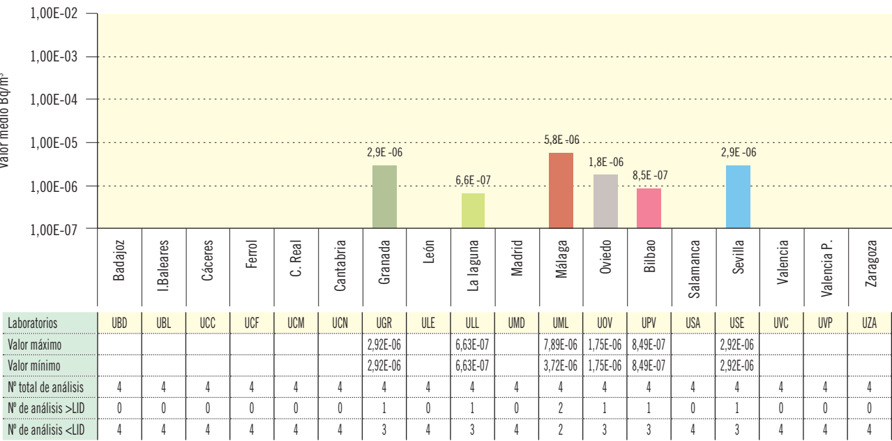
Figura 3.4b. Partículas de polvo en aire. Concentración de actividad de Sr-90 (Bq/m³) Valores de la campaña de 2016
