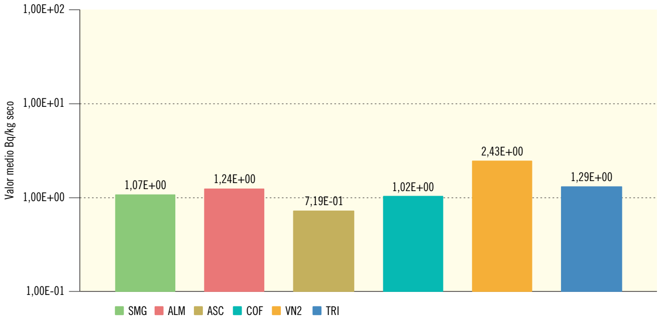
Figura 2.10b. Suelo. Concentración de actividad de Sr-90 (Bq/kg seco) Valores de la campaña de 2016
