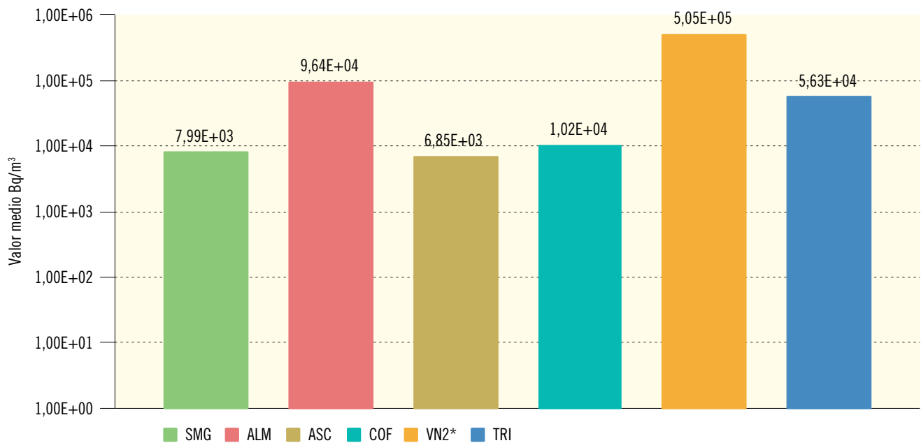
Figura 2.14b. Agua superficial. Concentración de actividad de H-3 (Bq/m³) Valores de la campaña de 2016
