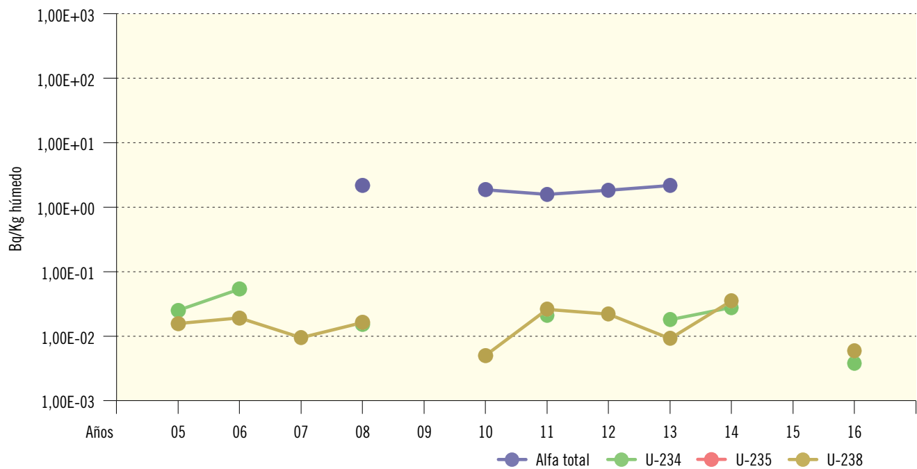
Figura 2.48. Juzbado. Carne y Aves. Valores de concentración de actividad (Bq/Kg húmedo) Evolución temporal valores medios
