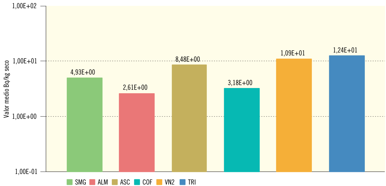
Figura 2.11b. Suelo. Concentración de actividad de Cs-137 Valores de la campaña de 2016
