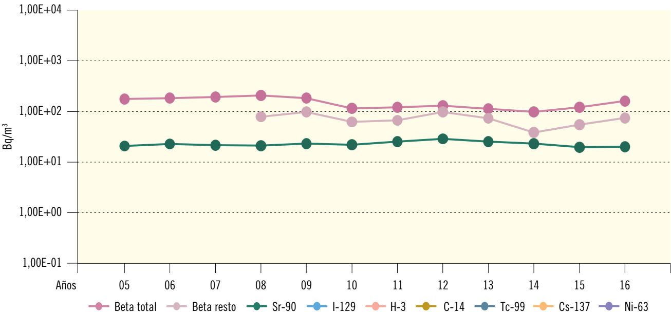
Figura 2.44. El Cabril. Agua superficial. Valores de concentración de actividad (Bq/m³) Evolución temporal valores medios
