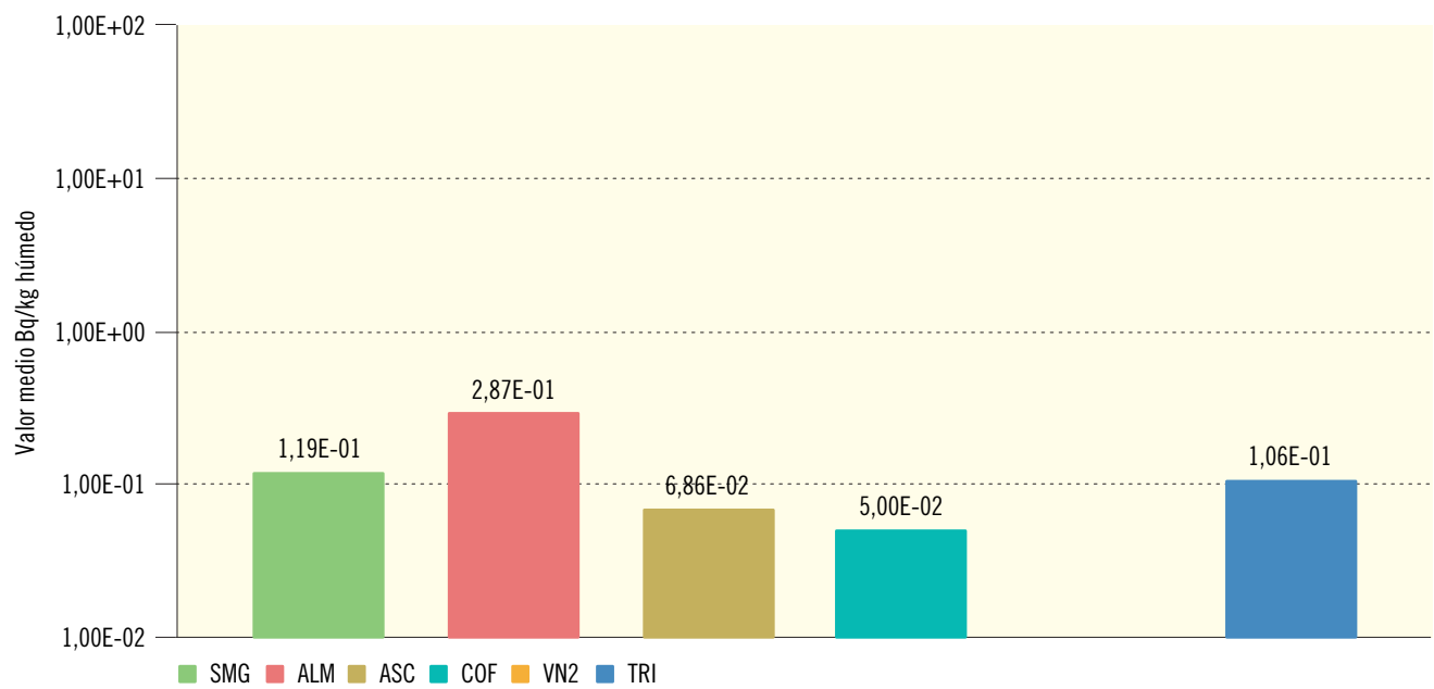
Figura 2.30b. Vegetales de hoja ancha. Concentración de actividad de Sr-90 (Bq/kg húmedo) Valores de la campaña de 2016
