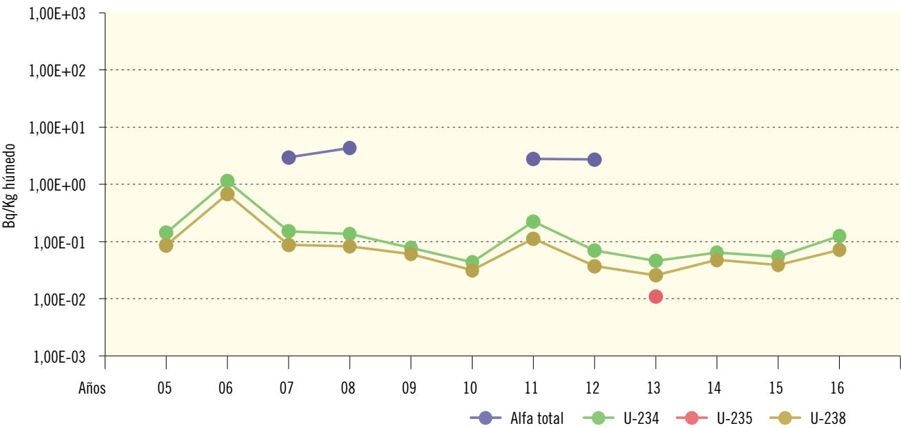
Figura 2.52. Juzbado. Peces. Valores de concentración de actividad (Bq/Kg húmedo) Evolución temporal valores medios
