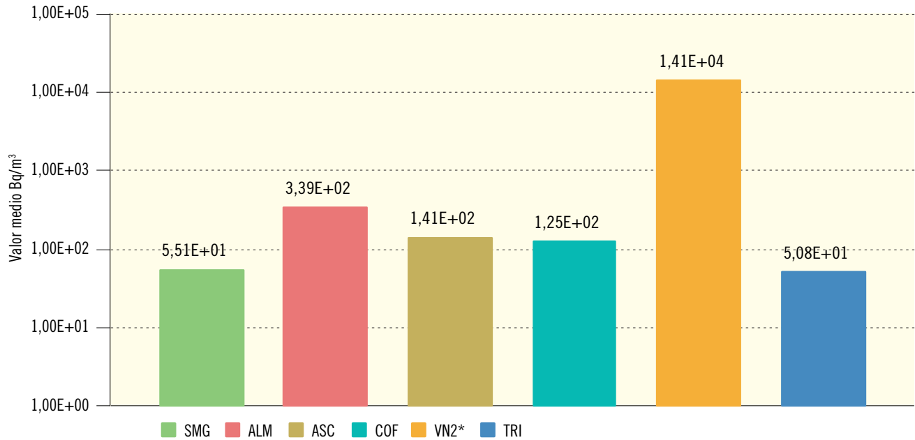
Figura 2.12b. Agua superficial. Concentración del índice de actividad beta total (Bq/m³) Valores de la campaña de 2016
