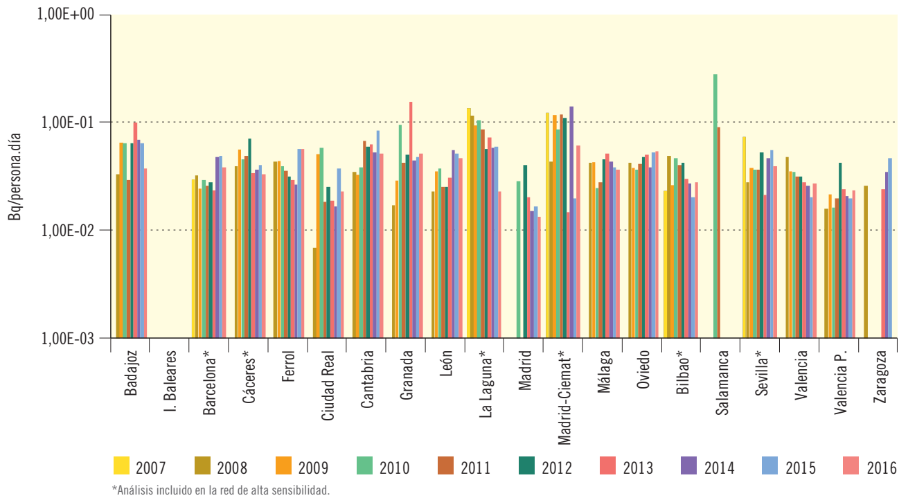
Figura 3.17b. Dieta tipo. Concentración de actividad de Sr-90 (Bq/persona.día)
