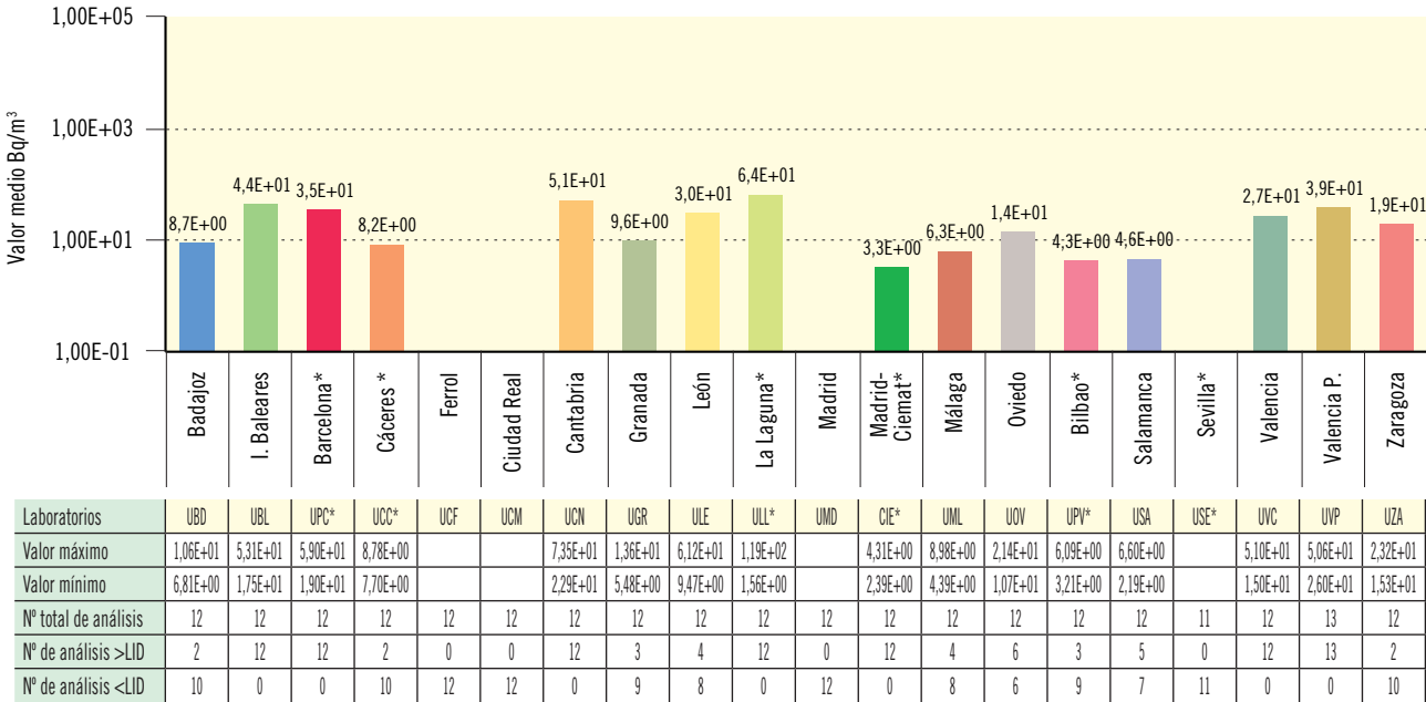
Figura 3.10b. Agua potable. Concentración del índice de actividad de alfa total (Bq/m³) Valores de la campaña de 2016
