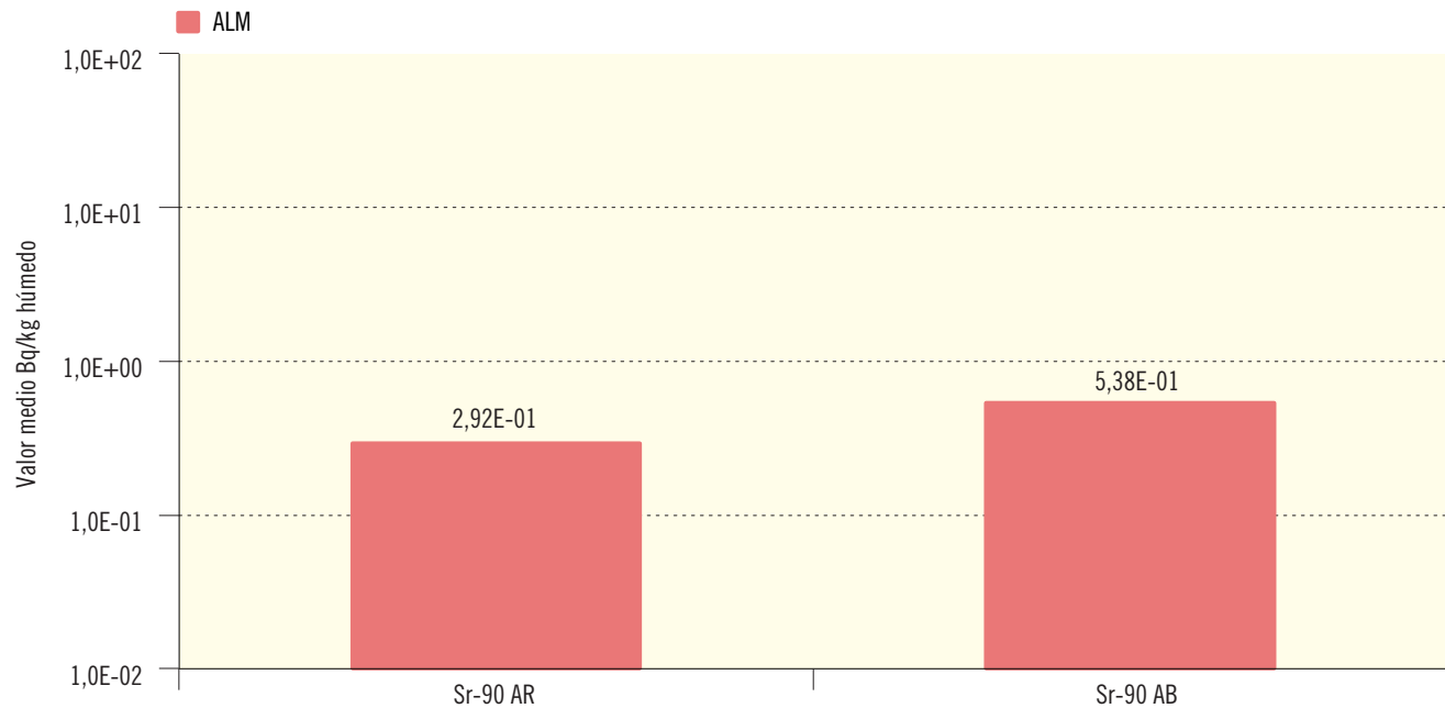
Figura 2.25b. Plantas terrestres. Concentración de actividad (Bq/kg húmedo) Valores de la campaña de 2016
