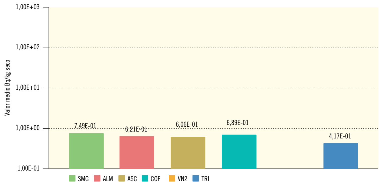
Figura 2.19b. Sedimentos de fondo. Concentración de actividad de Sr-90 (Bq/kg seco) Valores de la campaña de 2016
