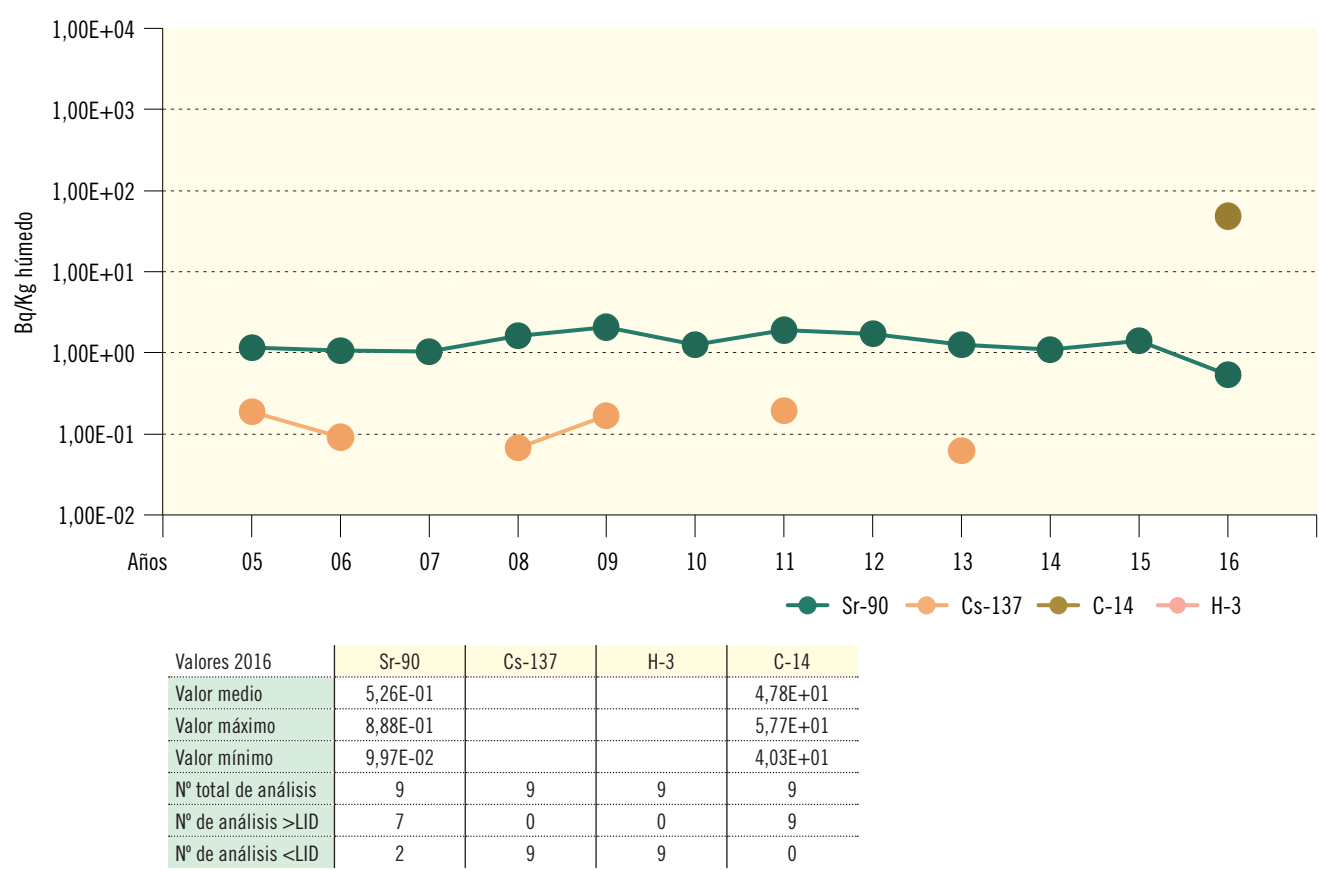
Figura 2.54. El Cabril. Plantas Terrestres. Valores de concentración de actividad (Bq/Kg húmedo) Evolución temporal valores medios
