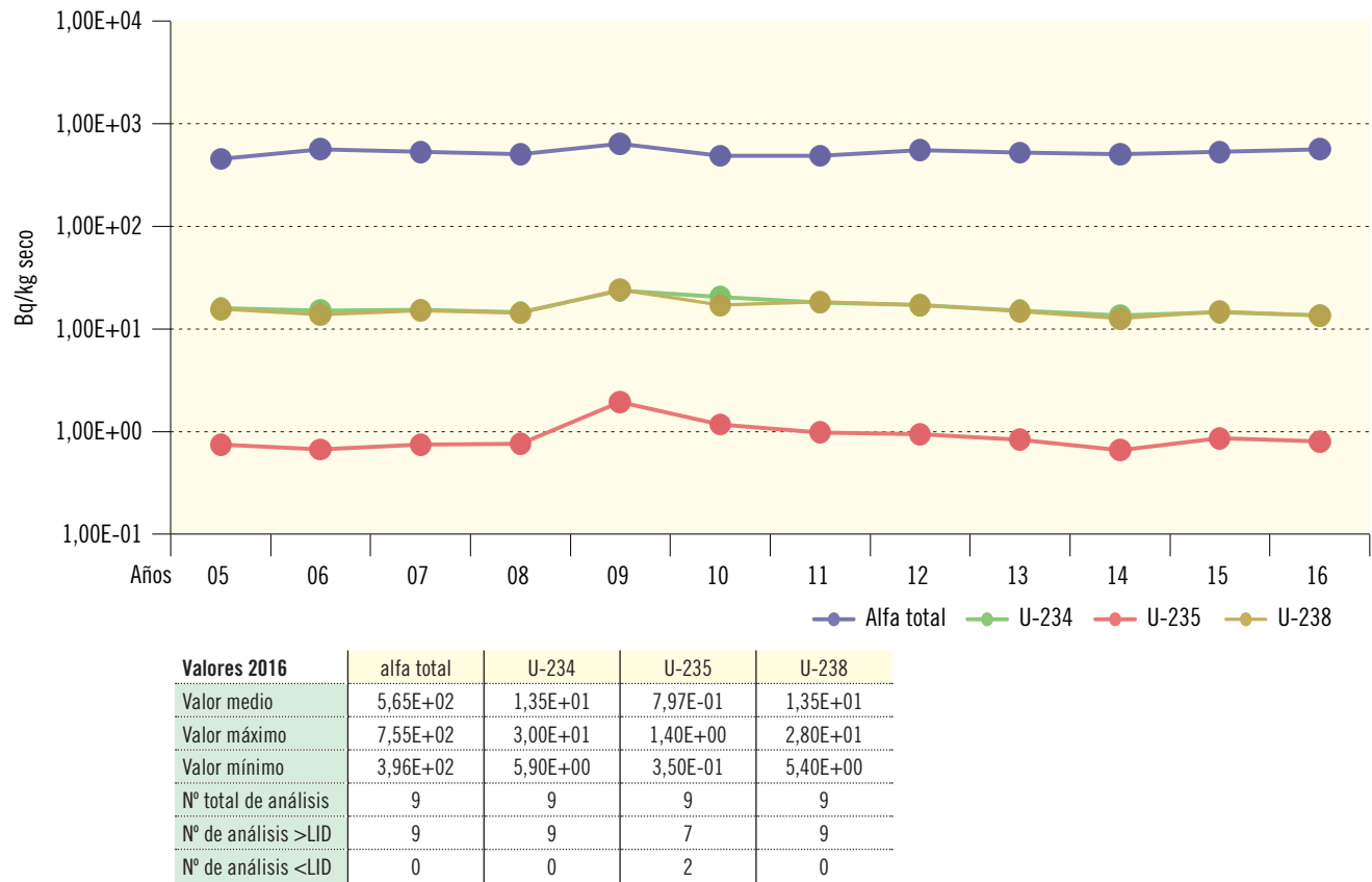
Figura 2.41. Juzbado. Suelo. Valores de concentración de actividad (Bq/kg seco) Evolución temporal valores medios
