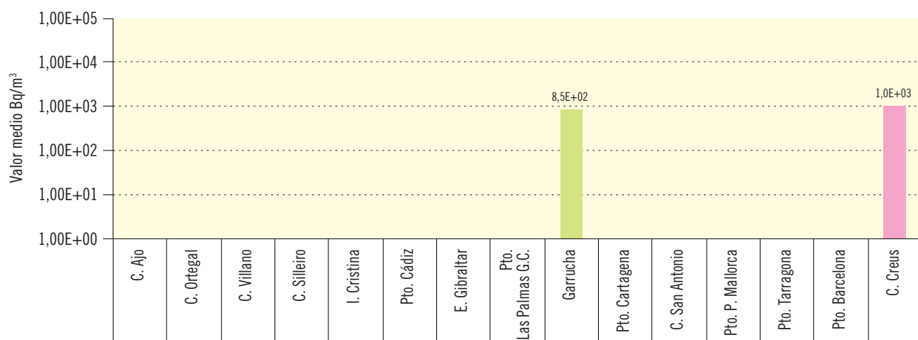
Figura 3.65b. Agua de mar. Concentración del índice de actividad beta resto (Bq/m³)
