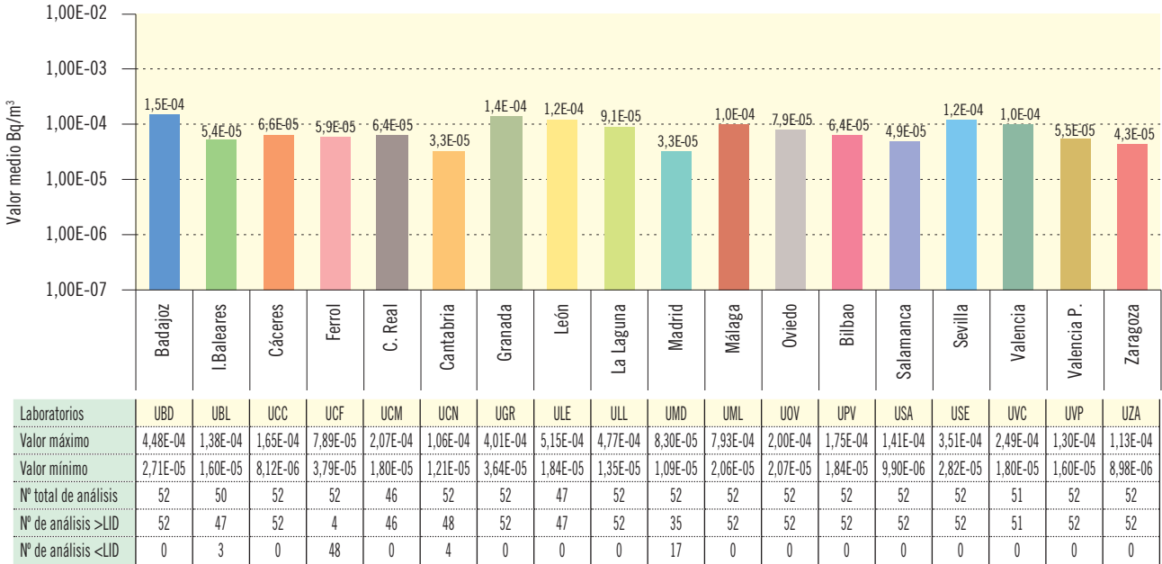
Figura 3.2b. Partículas de polvo en aire. Concentración del índice de actividad alfa total (Bq/m³) Valores de la campaña de 2016
