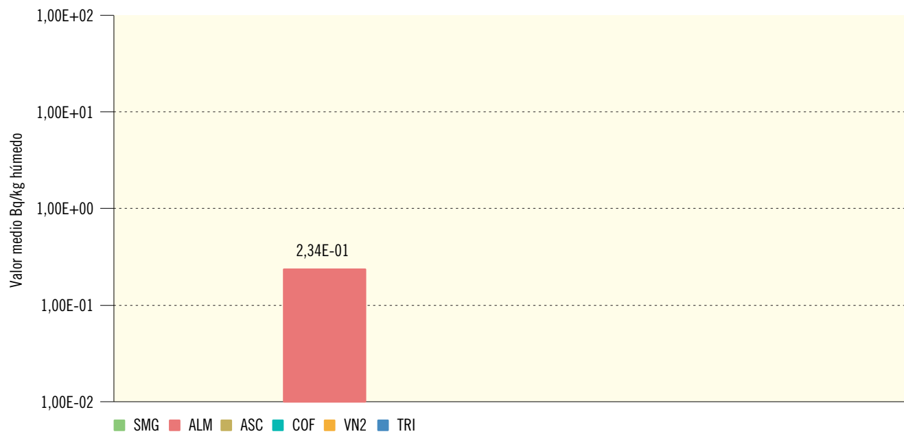
Figura 2.34b. Carne y aves. Concentración de actividad de Cs-137 (Bq/kg húmedo) Valores de la campaña de 2016
