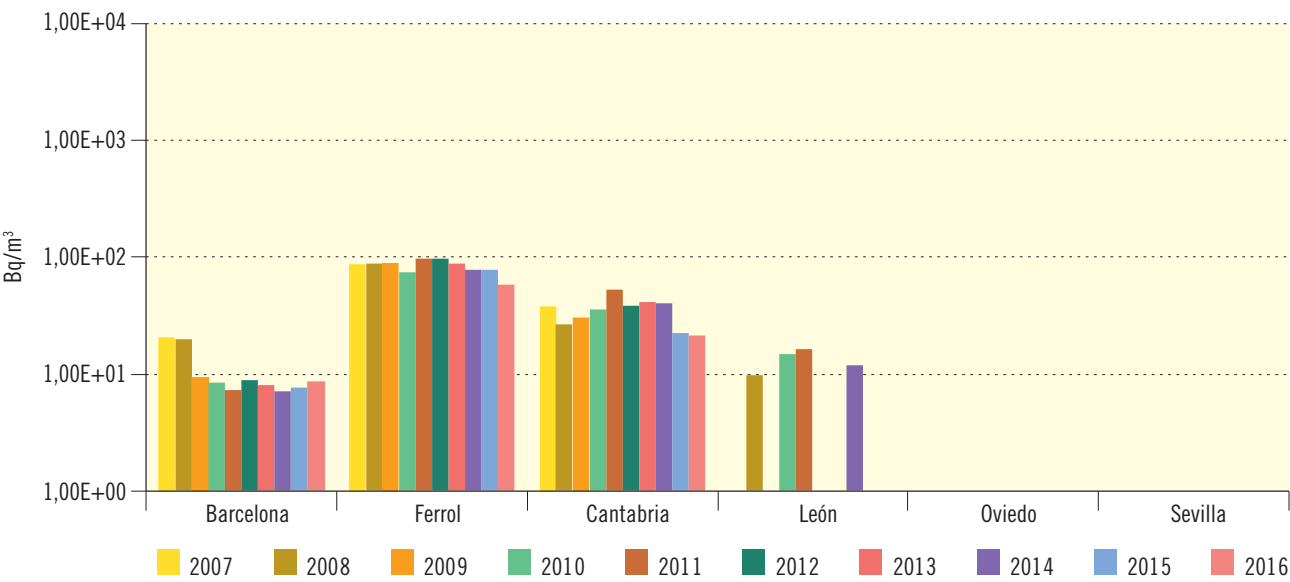
Figura 3.16a. Leche Evolución temporal de la concentración de actividad de Cs-137
