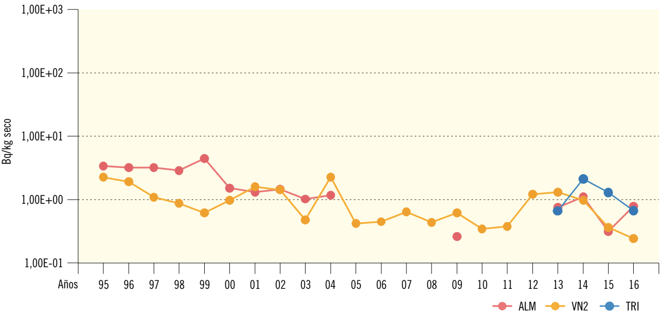
Figura 2.22a. Sedimentos de orilla. Evolución temporal de la concentración de actividad de Cs-137 Valores medios en la zona vigilada
