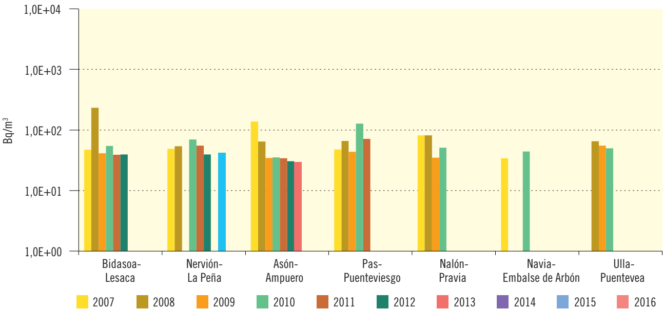
Figura 3.23. Cuencas del norte de España Evolución temporal del índice de actividad beta resto
