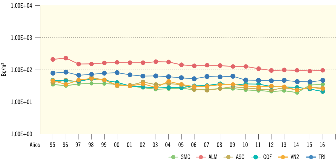
Figura 2.28a. Leche. Evolución temporal de la concentración de actividad de Sr-90 Valores medios en la zona vigilada
