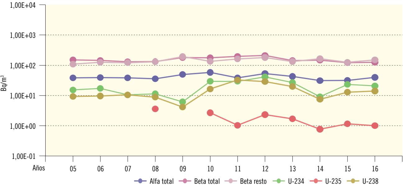
Figura 2.43. Juzbado. Agua superficial. Valores de concentración de actividad (Bq/m³) Evolución temporal valores medios
