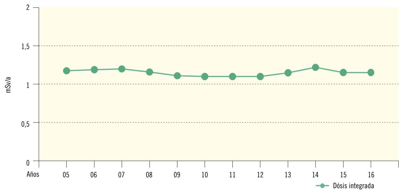
Figura 2.40. El Cabil. Radiación directa. Dosis integrada (DTL, mSv/año) Evolución temporal valores medios
