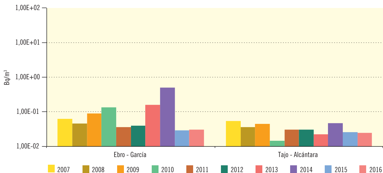
Figura 3.61a. Red de alta sensibilidad. Agua superficial Evolución temporal de la actividad de Cs-137
