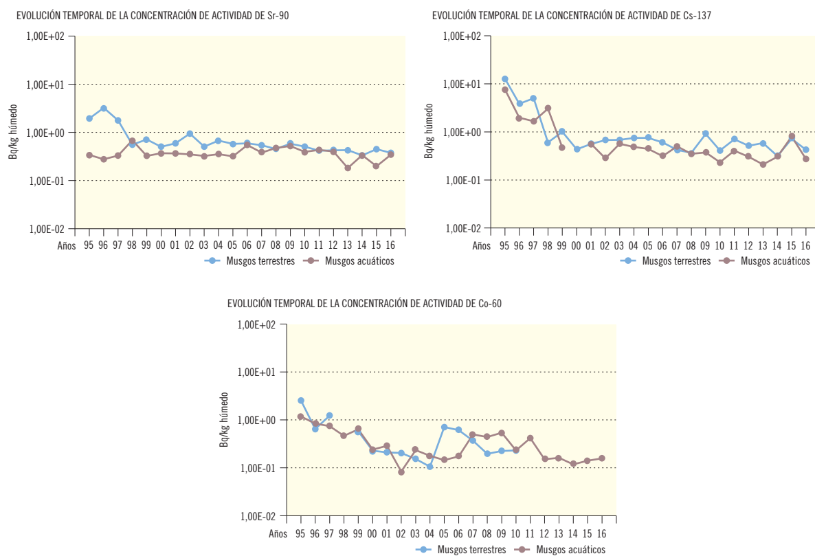
Figura 2.26b. Musgos. CN. STª María de Garoña. Concentración de actividad (Bq/kg húmedo)
