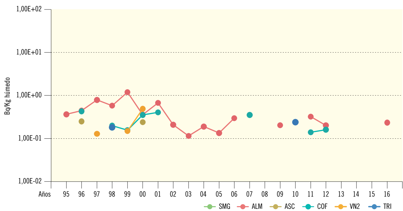
Figura 2.34b. Carne y aves. Concentración de actividad de Cs-137 (Bq/kg húmedo) Valores de la campaña de 2016
