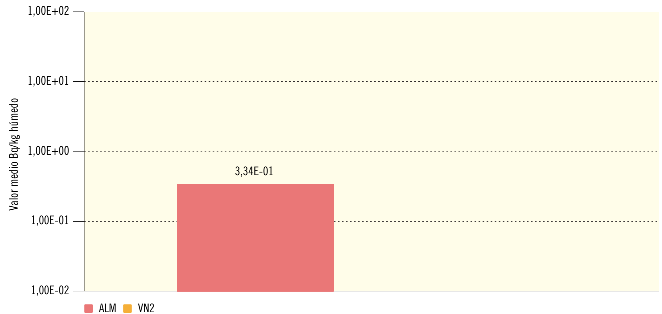
Figura 2.33b. Consumo animal. Concentración de actividad de Cs-137 (Bq/kg húmedo) Valores de la campaña de 2016
