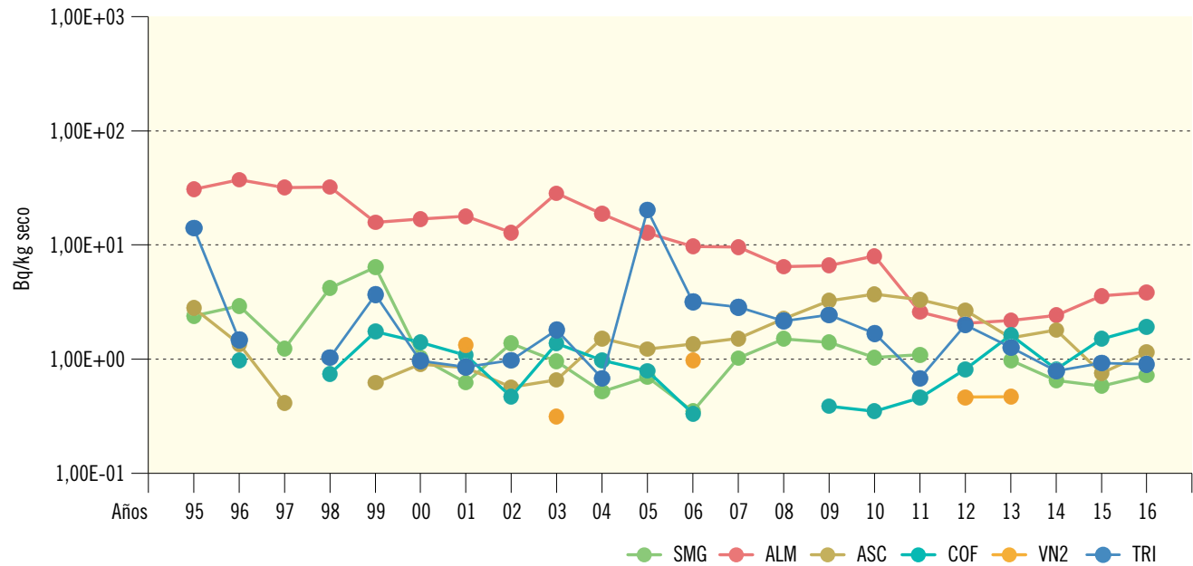
Figura 2.21a. Sedimentos de fondo. Evolucion temporal de la concentración de actividad de Co-60 Valores medios en la zona vigilada
