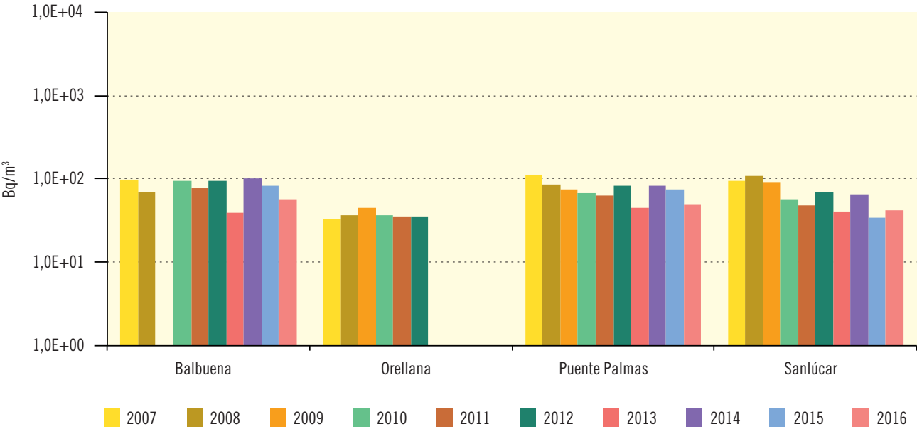
Figura 3.39. Río Guadiana Evolución temporal del índice de actividad beta resto
