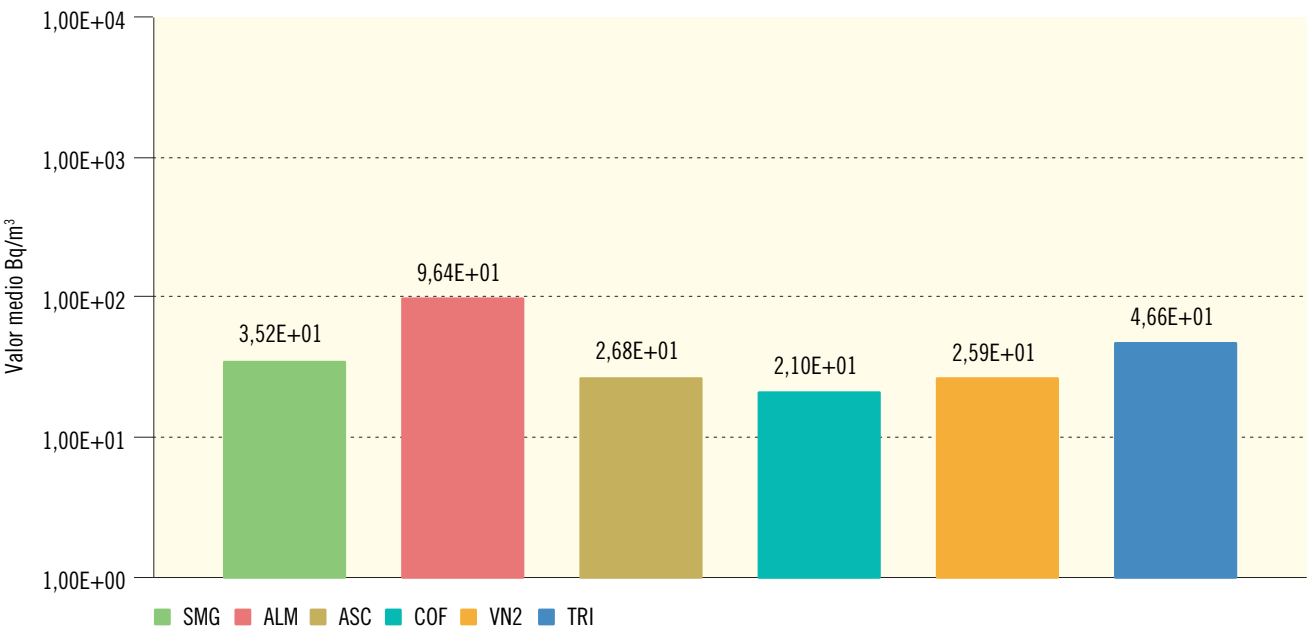
Figura 2.28b. Leche. Concentración de actividad de Sr-90 (Bq/m³) Valores de la campaña de 2016
