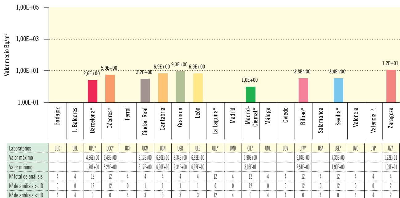
Figura 3.13b. Agua potable. Concentración de actividad de Sr-90 (Bq/m³)
