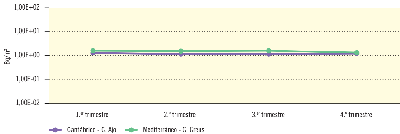
Figura 3.67b. Red de alta sensibilidad. Agua de mar. Concentración de actividad de Cs-137 (Bq/m³) Valores de la campaña de 2016
