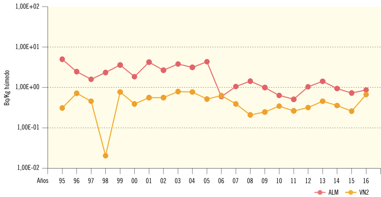
Figura 2.32b. Consumo animal. Concentración de actividad de Sr-90 (Bq/kg húmedo) Valores de la campaña de 2016
