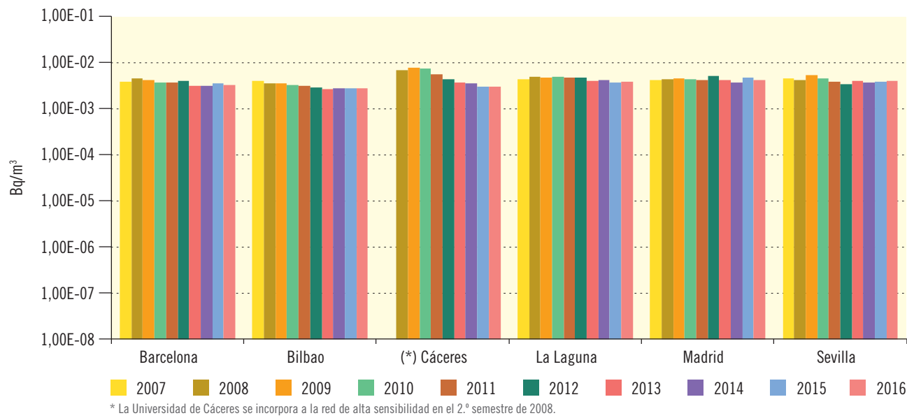
Figura 3.6b. Red de alta sensibilidad. Partículas de Polvo en aire. Muestreador alto flujo Concentración de actividad de Be-7 (Bq/m³). Valores de la campaña de 2016
