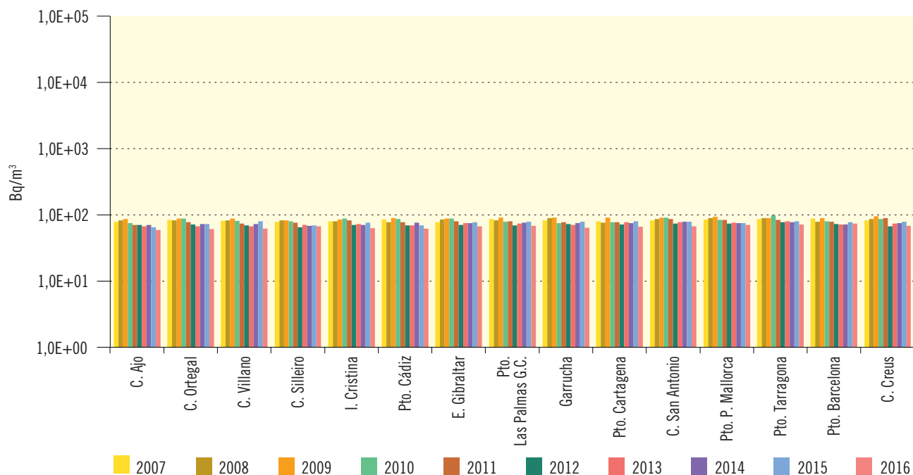
Figura 3.63a. Agua de mar
