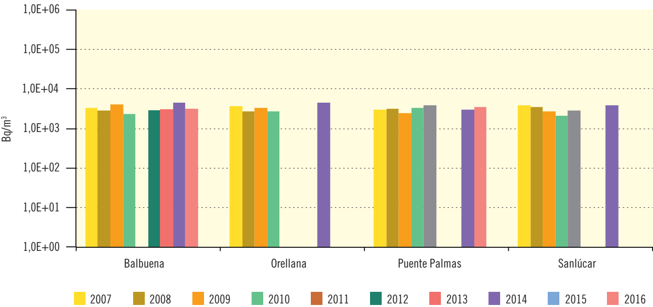
Figura 3.40. Río Guadiana Evolución temporal de concentración de actividad de H-3
