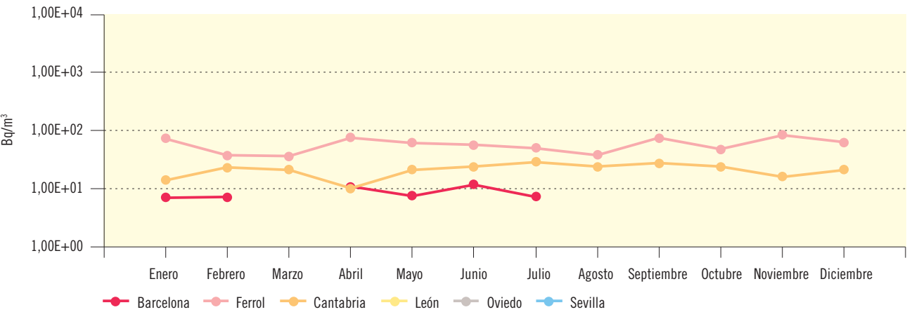
Figura 3.16b. Leche. Concentración de actividad de Cs-137 (Bq/m³) Valores de la campaña de 2016
