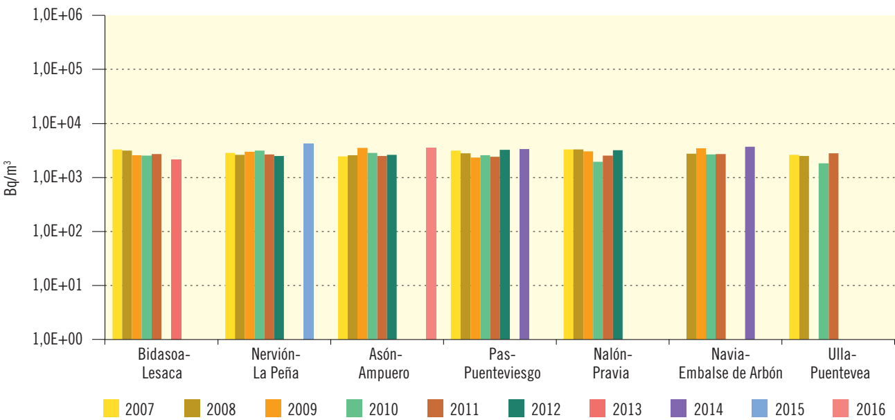
Figura 3.24. Cuencas del norte de España Evolución temporal de la concentración de actividad de H-3
