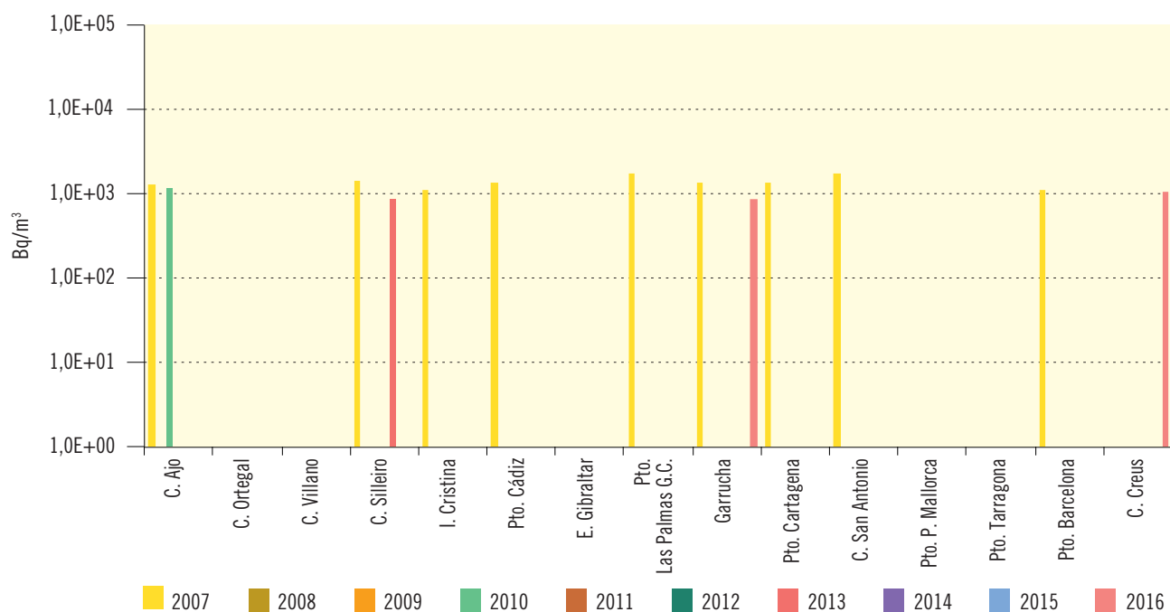
Figura 3.65a. Agua de mar
