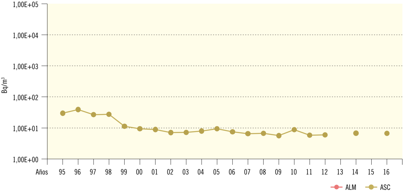
Figura 2.15a. Agua superficial. Evolucion temporal de la concentración de actividad de Sr-90 Valores medios en la zona vigilada
