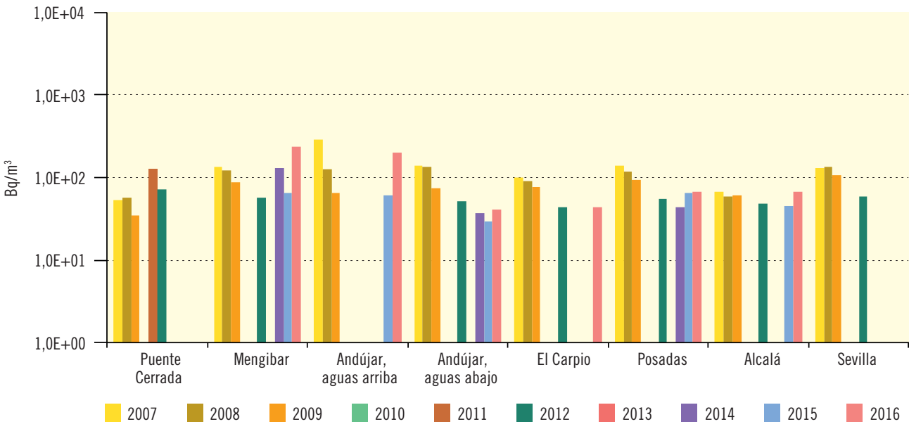
Figura 3.43. Río Guadalquivir Evolución temporal del índice de actividad beta resto
