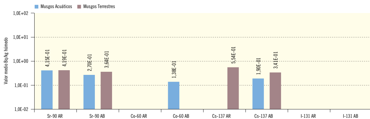
Figura 2.26b. Musgos. CN. STª María de Garoña. Concentración de actividad (Bq/kg húmedo)
