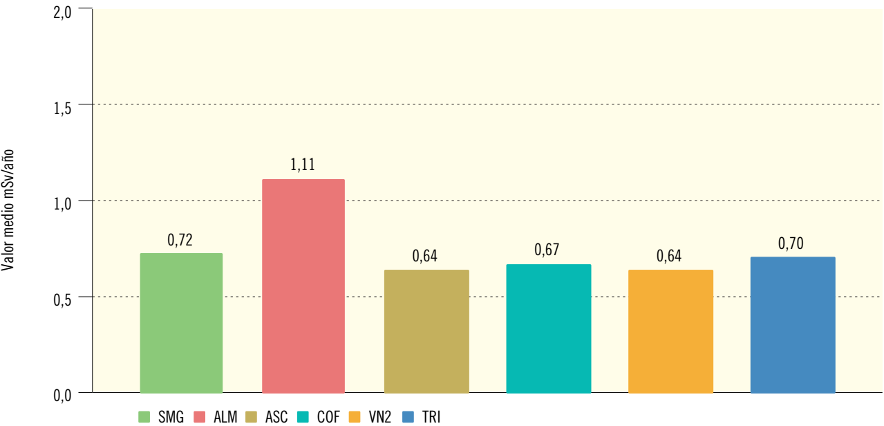
Figura 2.9b. Radiación directa. Dosis integrada (DTL). (mSv/año) Valores de la campaña de 2016
