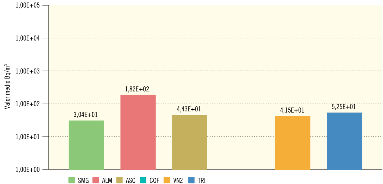
Figura 2.17b. Agua potable. Concentración del índice de actividad beta resto (Bq/m³) Valores de la campaña de 2016
