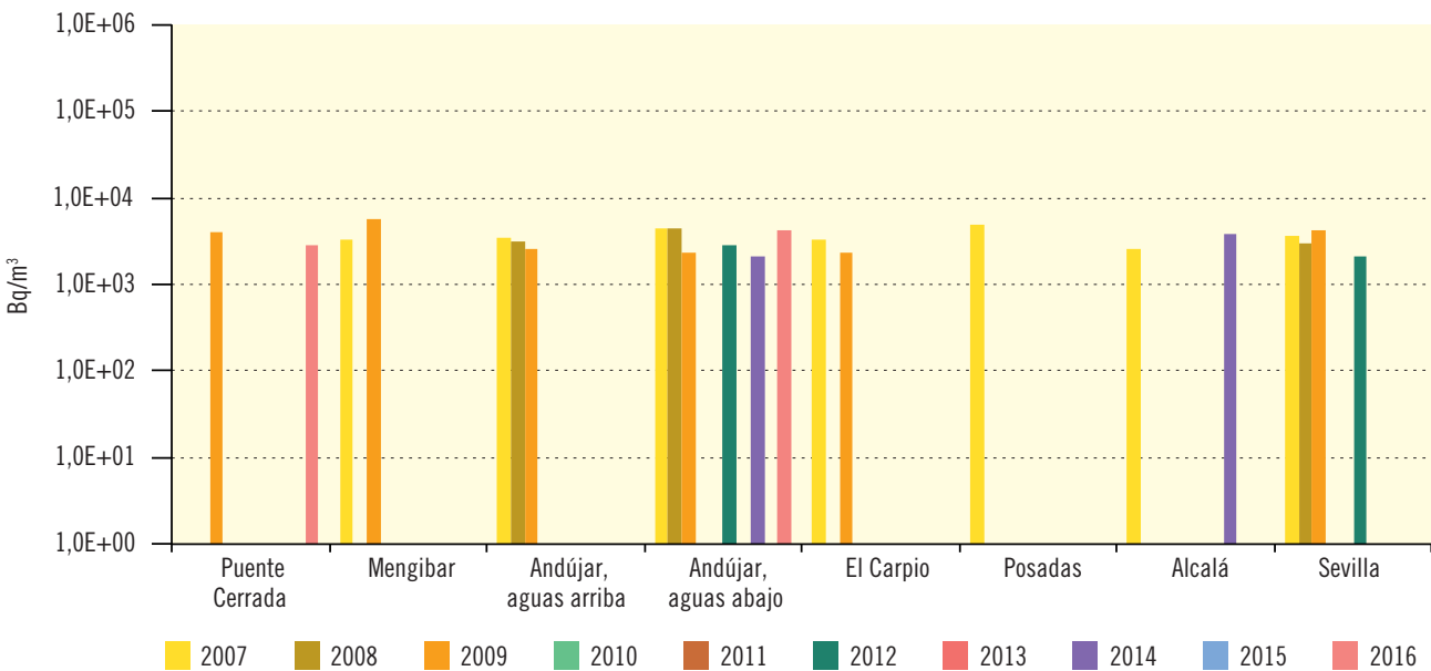
Figura 3.44. Río Guadalquivir Evolución temporal de concentración de actividad de H-3
