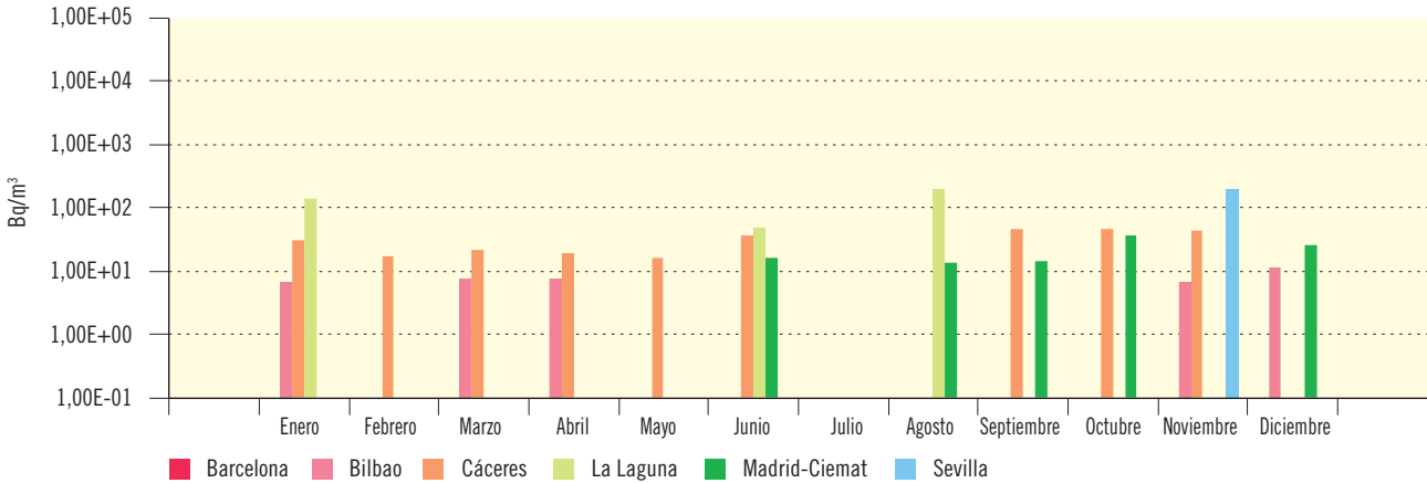
Figura 3.12b. Red de alta sensibilidad. Agua Potable. Concentración de actividad de beta resto (Bq/m³) Valores de la campaña de 2016
