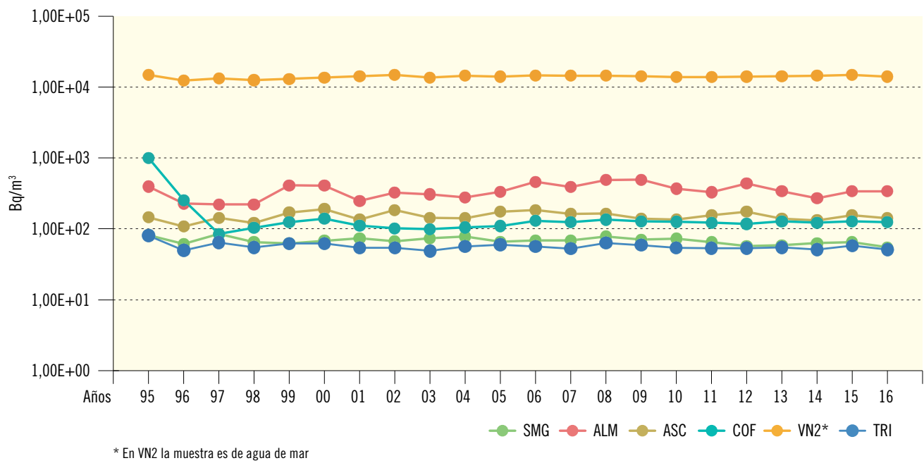
Figura 2.12b. Agua superficial. Concentración del índice de actividad beta total (Bq/m³) Valores de la campaña de 2016
