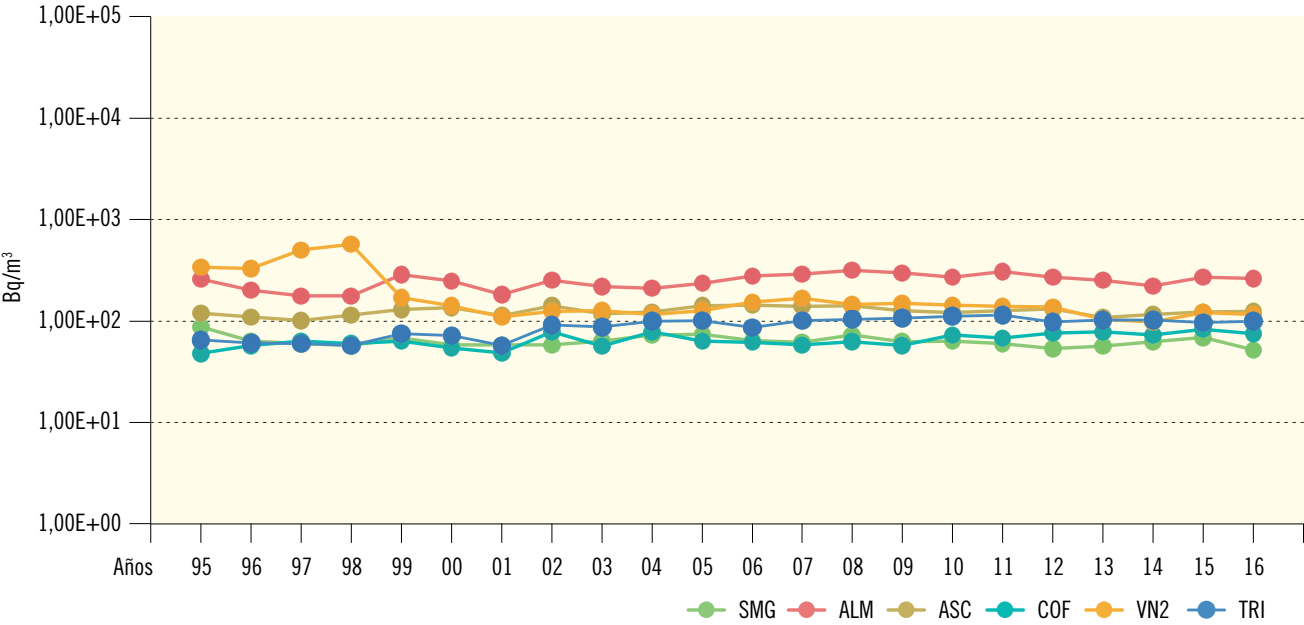
Figura 2.16a. Agua potable. Evolución temporal del índice de actividad beta total Valores medios en la zona vigilada
