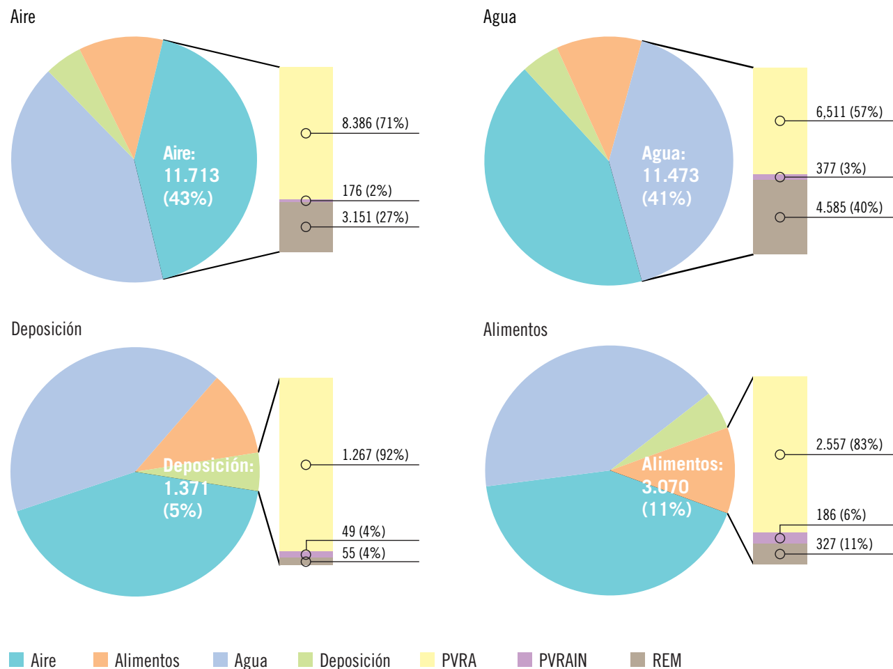
Figura 1.2. Programas de vigilancia radiológica ambiental. Campaña de 2016
