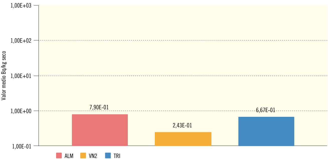
Figura 2.22b. Sedimentos de orilla. Concentración de actividad de Cs-137 (Bq/kg seco) Valores de la campaña de 2016
