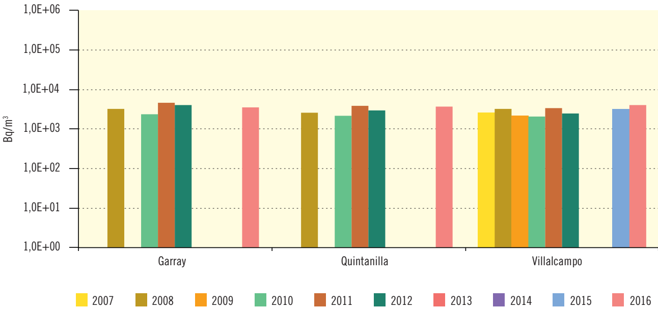
Figura 3.32. Río Duero Evolución temporal de concentración de actividad de H-3
