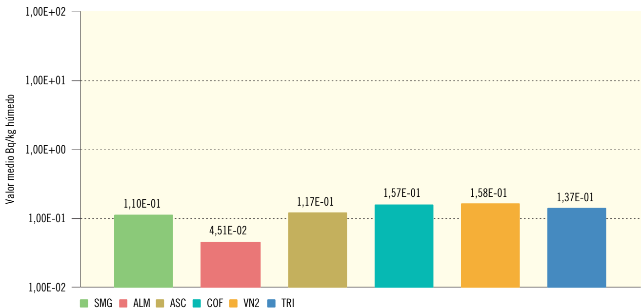
Figura 2.31b. Vegetales de hoja no ancha. Concentración de actividad de Sr-90 (Bq/kg húmedo) Valores de la campaña de 2016
