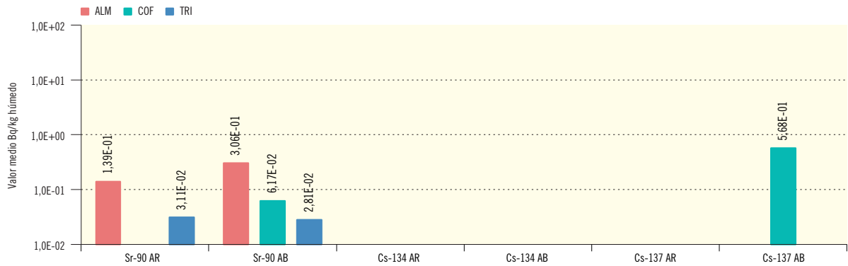
Figura 2.24b. Plantas de orilla. Concentración de actividad (Bq/kg húmedo) Valores de la campaña de 2016
