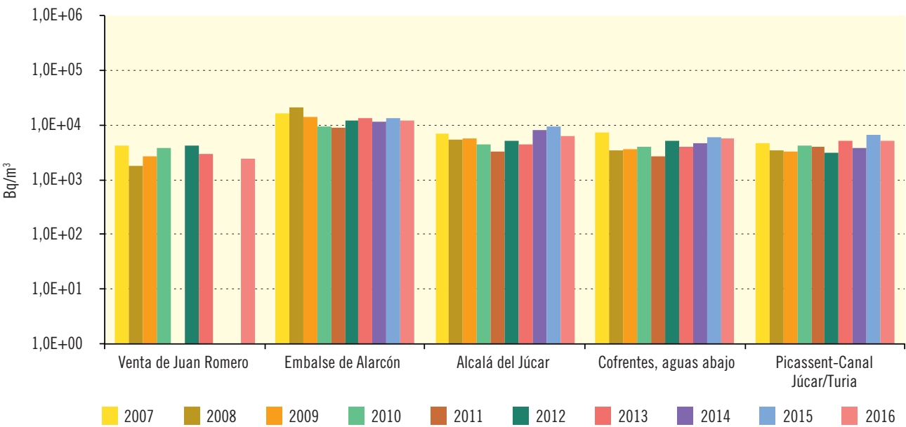
Figura 3.52. Río Júcar Evolución temporal de concentración de actividad de H-3
