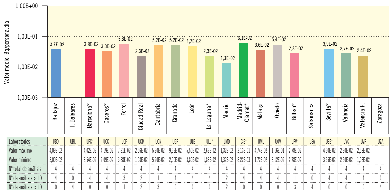
Figura 3.17b. Dieta tipo. Concentración de actividad de Sr-90 (Bq/persona.día)
