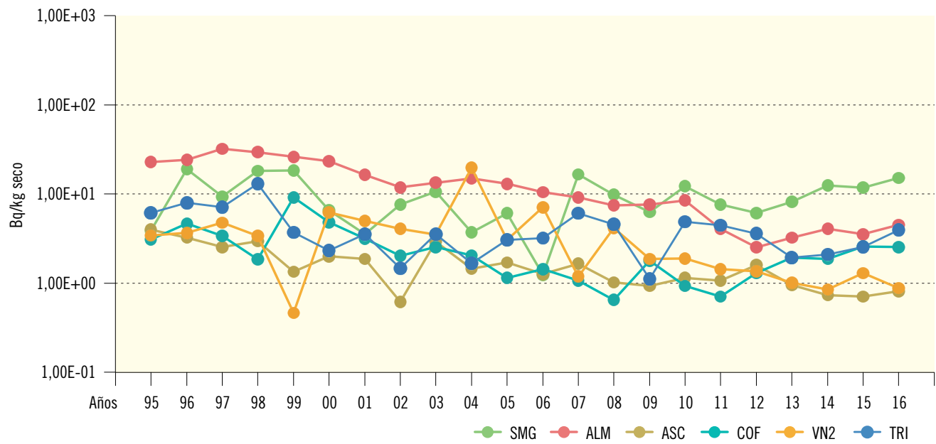
Figura 2.20a. Sedimentos de fondo. Evolución temporal de la concentración de actividad de Cs-137 Valores medios en la zona vigilada
