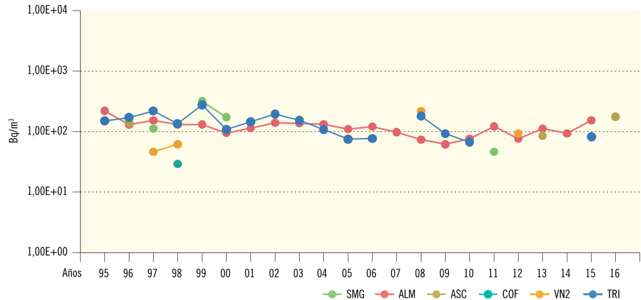
Figura 2.29a. Leche. Evolución temporal de la concentración de actividad de Cs-137 Valores medios en la zona vigilada
