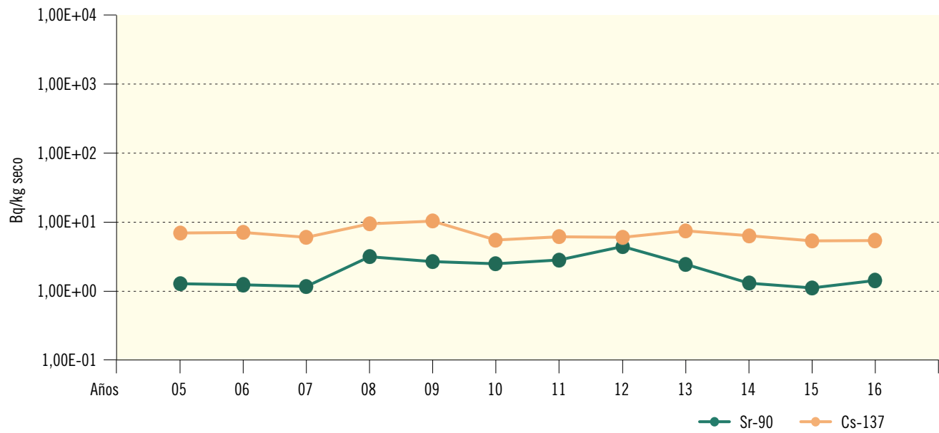
Figura 2.42. El Cabril. Suelo. Valores de concentración de actividad (Bq/kg seco) Evolución temporal valores medios
