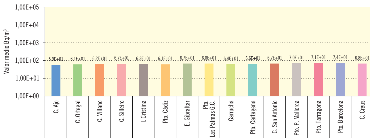
Figura 3.63b. Agua de mar. Concentración del índice de actividad alfa total (Bq/m³)
