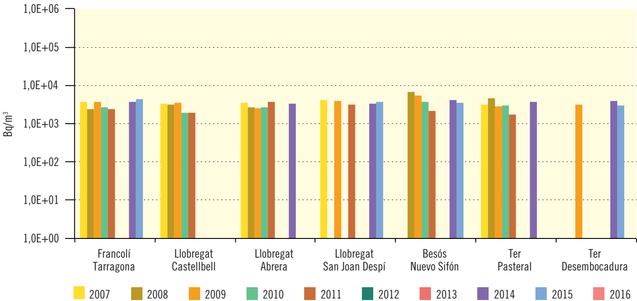
Figura 3.60. Cuencas catalanas Evolución temporal de la concentración de actividad de H-3
