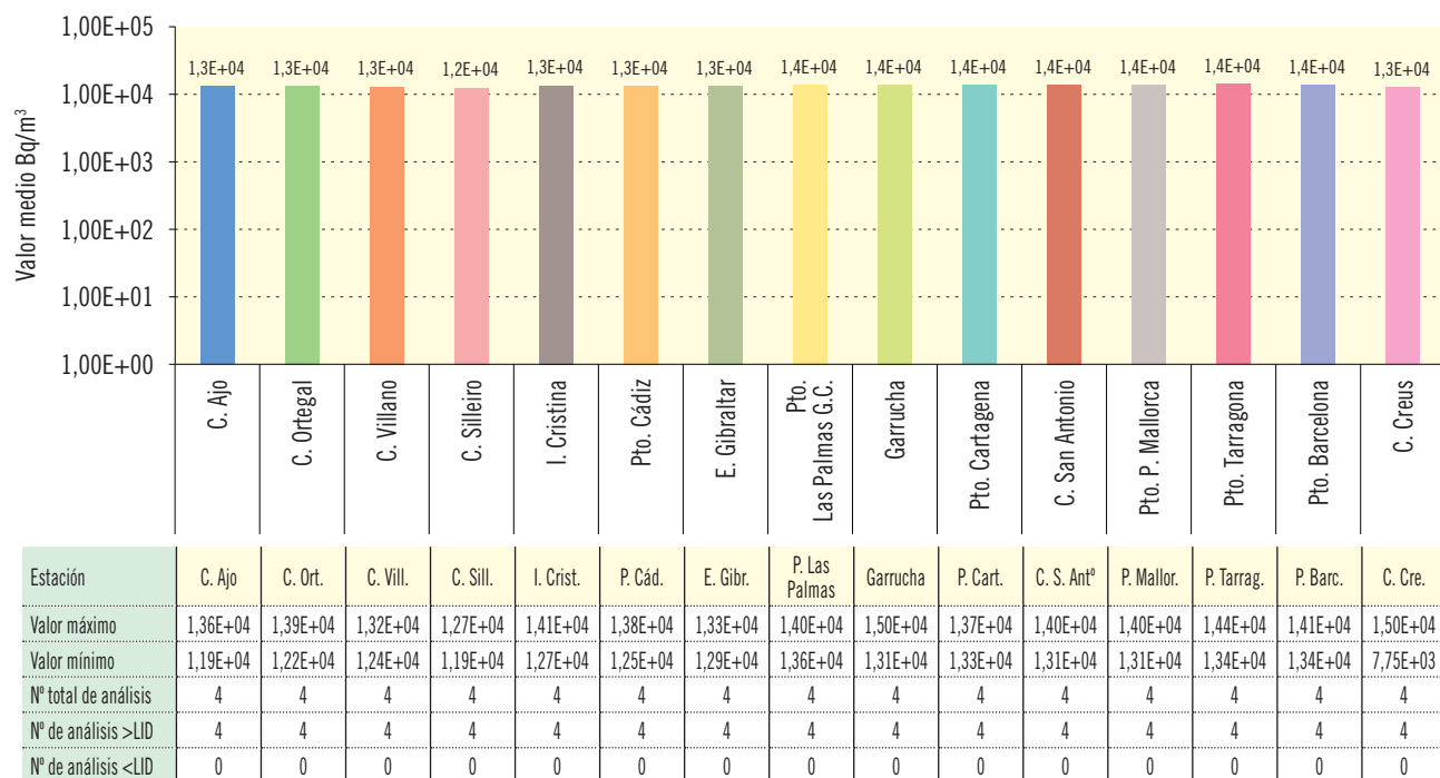
Figura 3.64b. Agua de mar. Concentración del índice de actividad beta total (Bq/m³)
