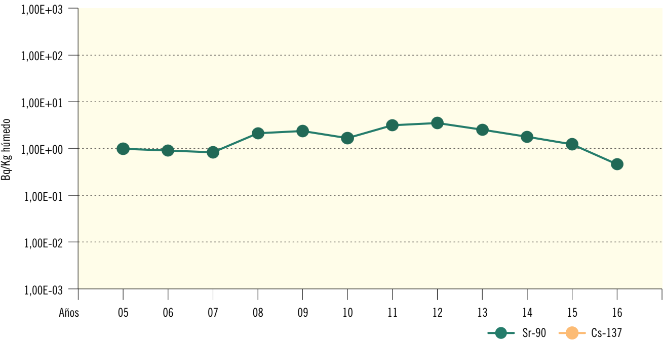
Figura 2.49. El Cabril. Carne y Aves. Valores de concentración de actividad (Bq/Kg húmedo) Evolución temporal valores medios
