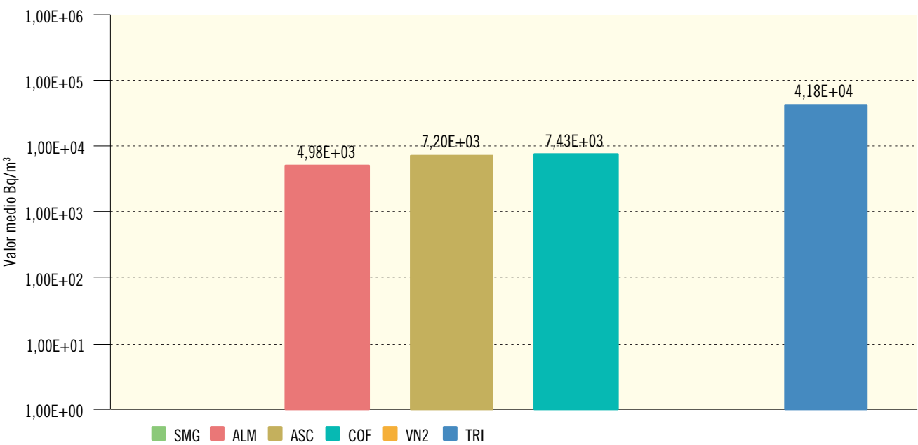
Figura 2.18b. Agua potable. Concentración de actividad de H-3 (Bq/m³) Valores de la campaña de 2016
