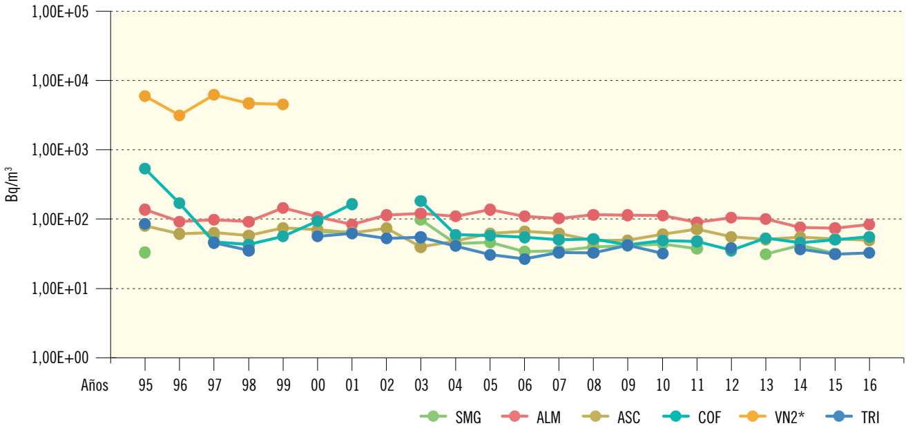
Figura 2.13b. Agua superficial. Concentración del índice de actividad beta resto (Bq/m³) Valores de la campaña de 2016
