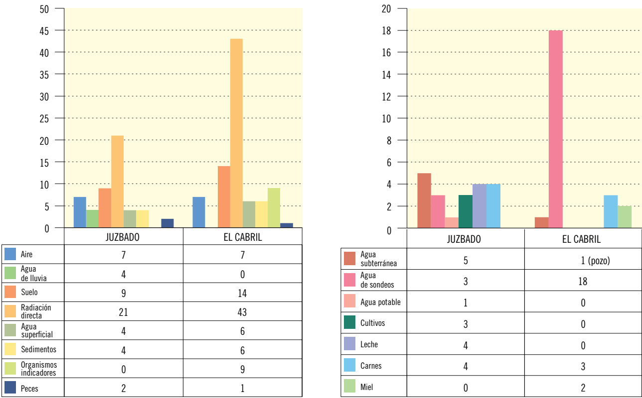
Figura 2.36. Número de estaciones de muestreo en los PVRA de las instalaciones del ciclo de combustible
