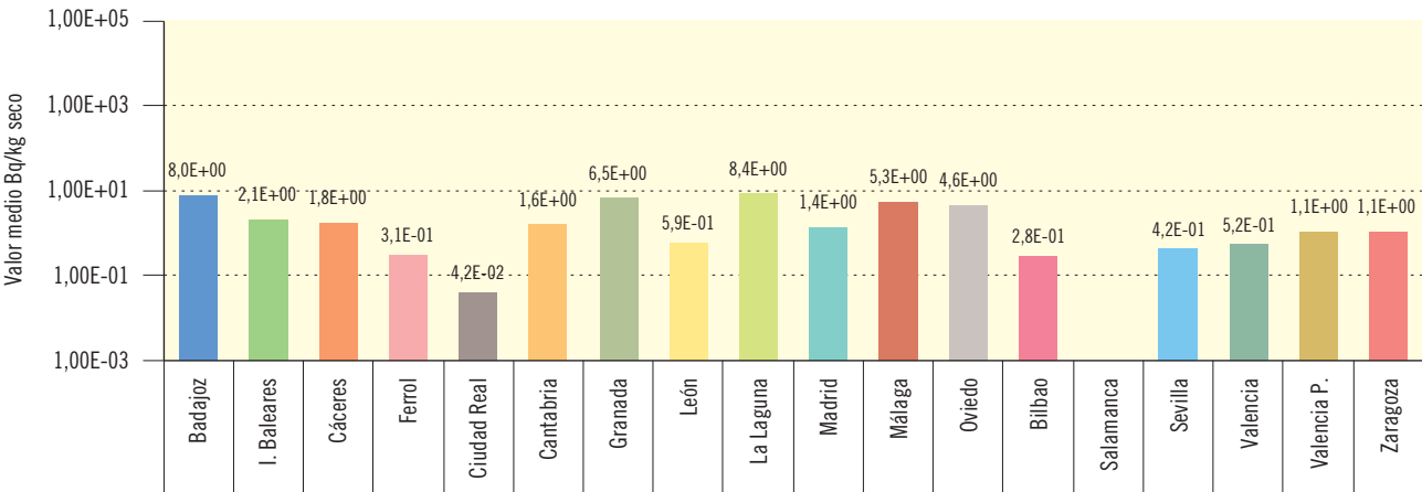
Figura 3.8b. Suelo. Concentración de actividad de Sr-90 (Bq/kg seco) Valores de la campaña de 2016
