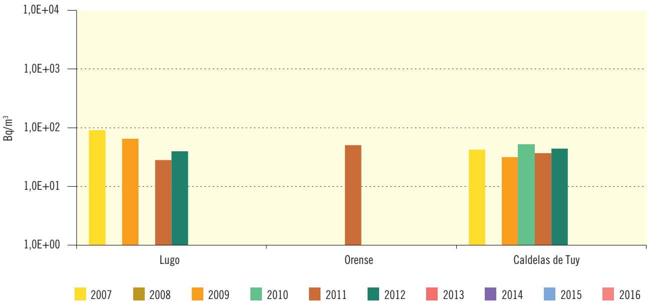
Figura 3.27. Río Miño Evolución temporal del índice de actividad beta resto
