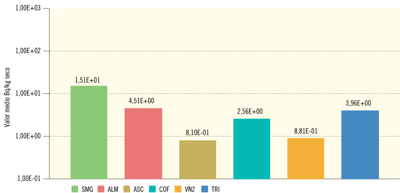
Figura 2.20b. Sedimentos de fondo. Concentración de actividad de Cs-137 (Bq/kg seco) Valores de la campaña de 2016
