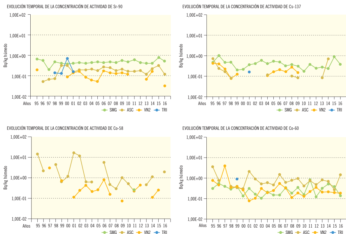
Figura 2.23b. Plantas acuáticas. Concentración de actividad (Bq/kg húmedo)
