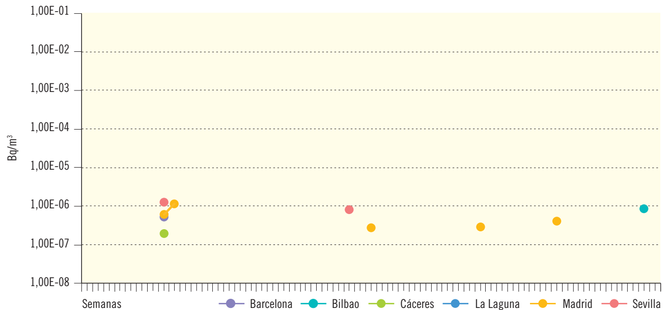
Figura 3.5b. Red de alta sensibilidad. Partículas de Polvo en aire. Muestreador alto flujo Concentración de actividad de Cs-137 (Bq/m³). Valores de la campaña de 2016
