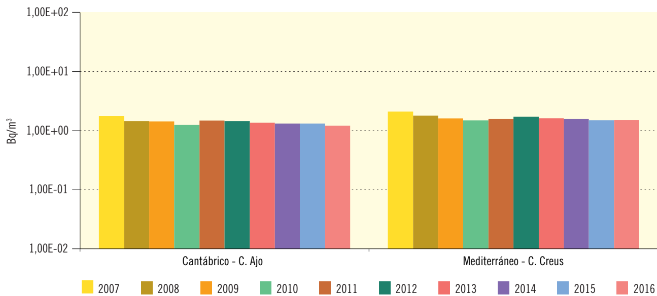
Figura 3.67a. Red de alta sensibilidad. Agua de mar Evolución temporal de la actividad de Cs-137
