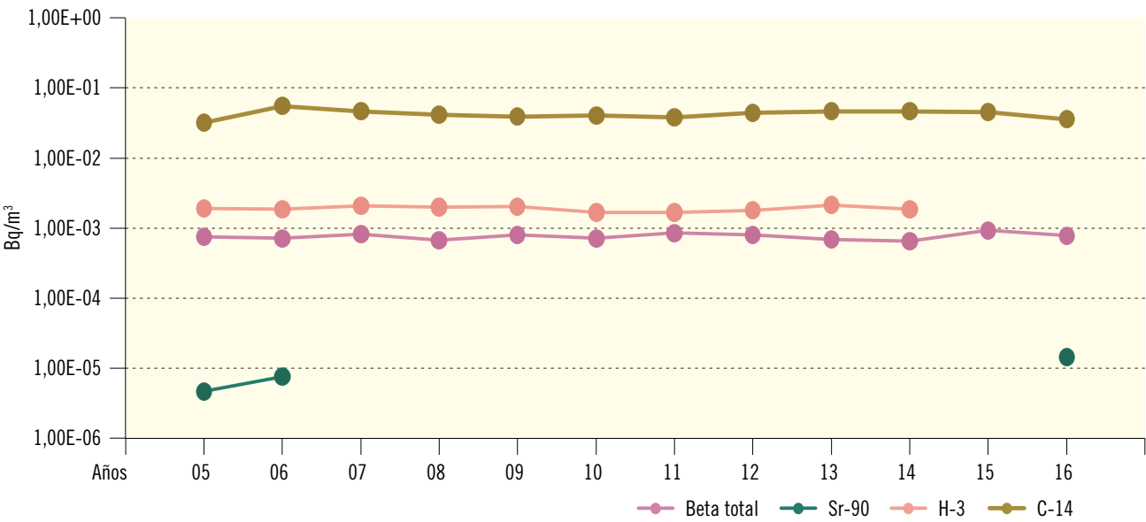
Figura 2.38. El Cabril. Aire. Valores de concentración de actividad (Bq/m³) Evolución temporal valores medios
