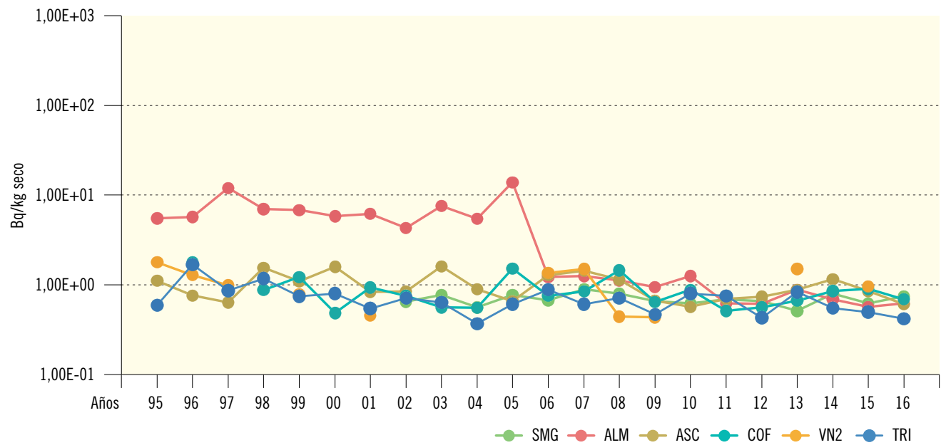
Figura 2.19a. Sedimentos de fondo. Evolución temporal de la concentración de actividad de Sr-90 Valores medios en la zona vigilada
