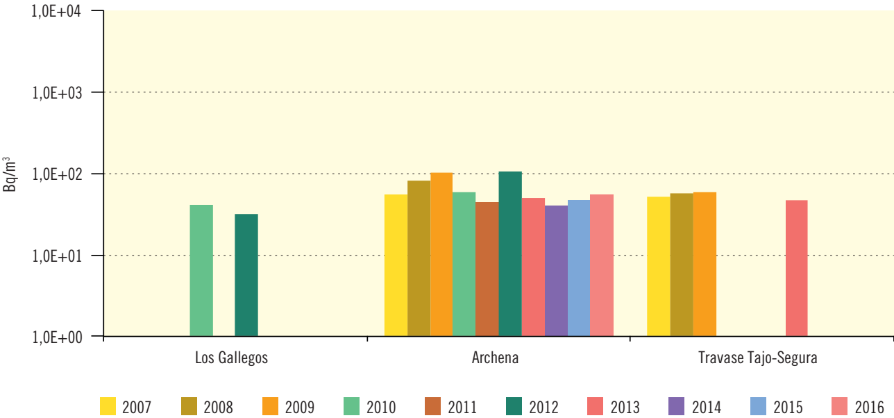
Figura 3.47. Río Segura Evolución temporal del índice de actividad beta resto
