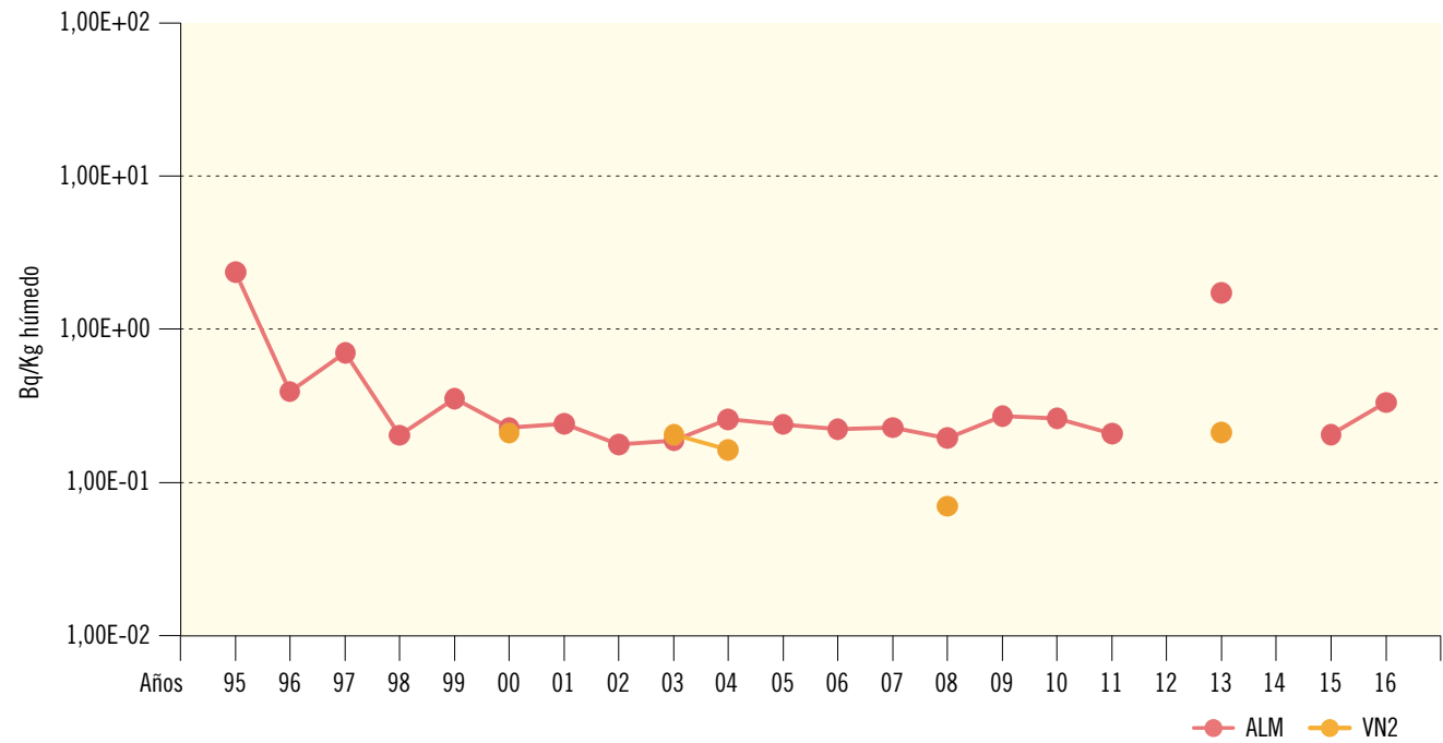
Figura 2.33b. Consumo animal. Concentración de actividad de Cs-137 (Bq/kg húmedo) Valores de la campaña de 2016
