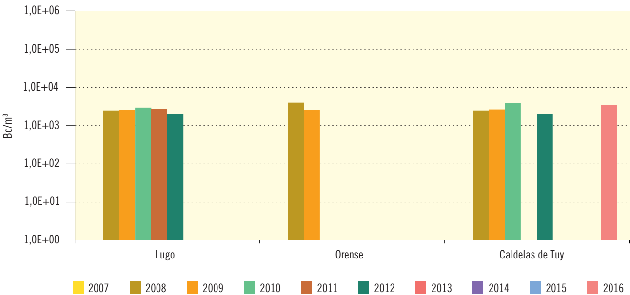
Figura 3.28. Río Miño Evolución temporal de la concentración de actividad de H-3
