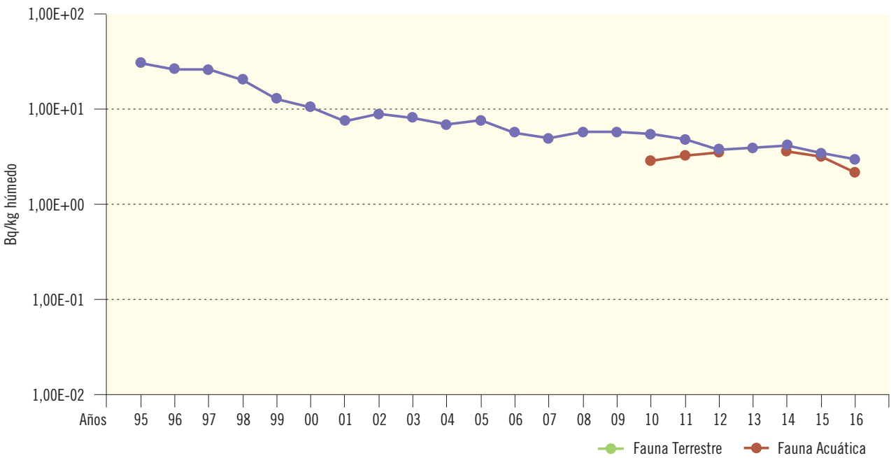
Figura 2.27b. Fauna terrestre y acuática. CN. STª María de Garoña. Concentración de actividad (Bq/kg húmedo) Valores de la campaña de 2016
