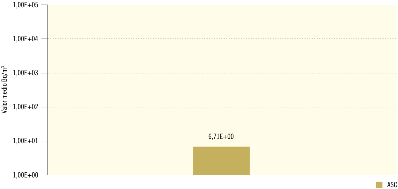
Figura 2.15b. Agua superficial. Concentración de actividad de Sr-90 (Bq/m³) Valores de la campaña de 2016
