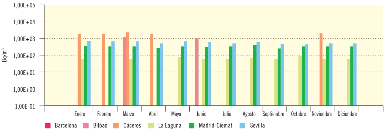
Figura 3.14b. Red de alta sensibilidad. Agua Potable. Concentración de actividad de H-3 (Bq/m³) Valores de la campaña de 2016
