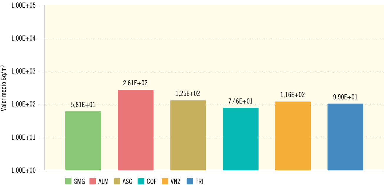
Figura 2.16b. Agua potable. Concentración del índice de actividad beta total (Bq/m³) Valores de la campaña de 2016
