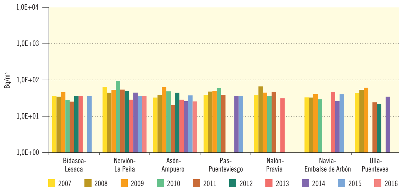
Figura 3.21. Cuencas del norte de España Evolución temporal del índice de actividad alfa total
