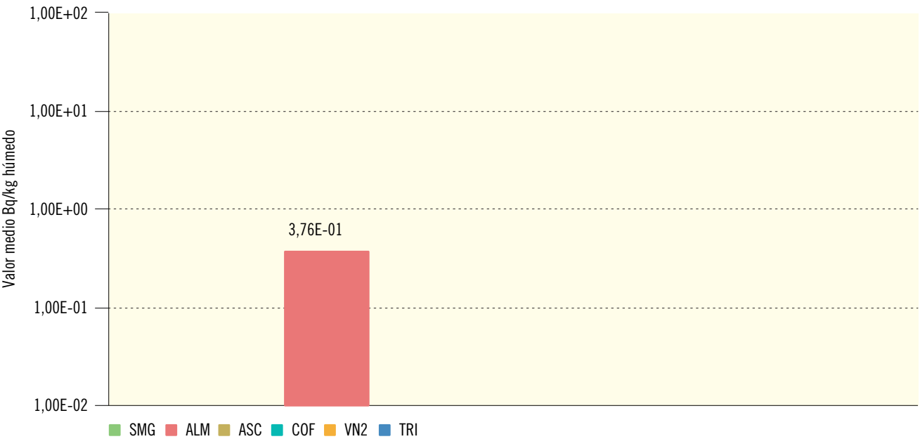
Figura 2.35b. Peces y mariscos. Concentración de actividad de Cs-137 (Bq/kg húmedo) Valores de la campaña de 2016
