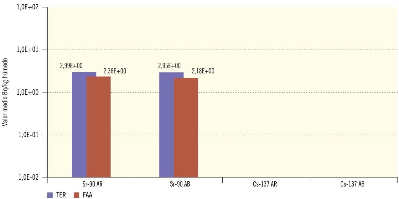
Figura 2.27b. Fauna terrestre y acuática. CN. STª María de Garoña. Concentración de actividad (Bq/kg húmedo) Valores de la campaña de 2016
