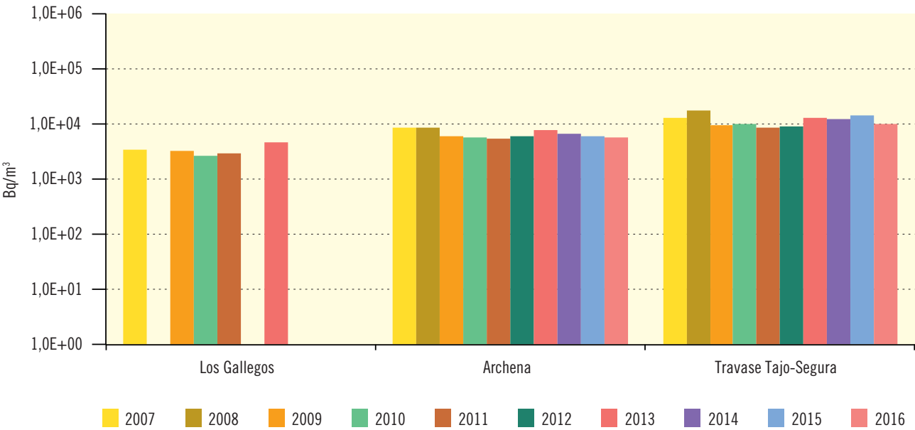
Figura 3.48. Río Segura Evolución temporal de concentración de actividad de H-3
