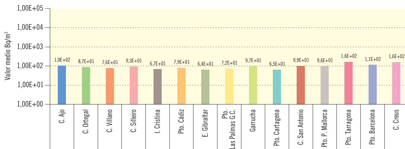
Figura 3.66b. Agua de mar. Concentración de actividad de H-3 (Bq/m³)
