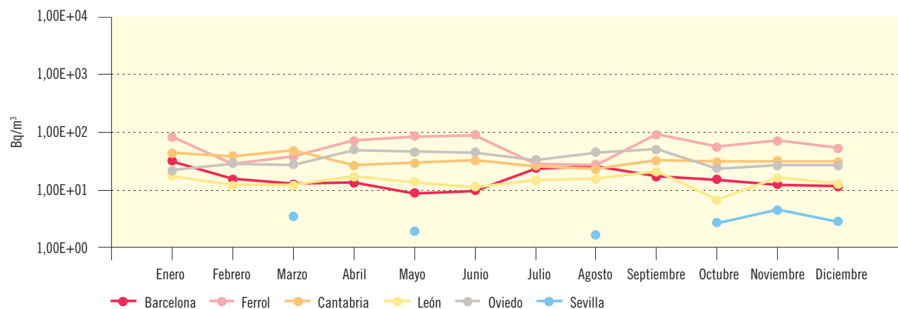
Figura 3.15b. Leche. Concentración de actividad de Sr-90 (Bq/m³)
