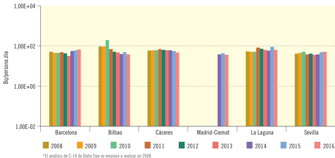
Figura 3.19a. Red de alta sensibilidad. DIETA TIPO
