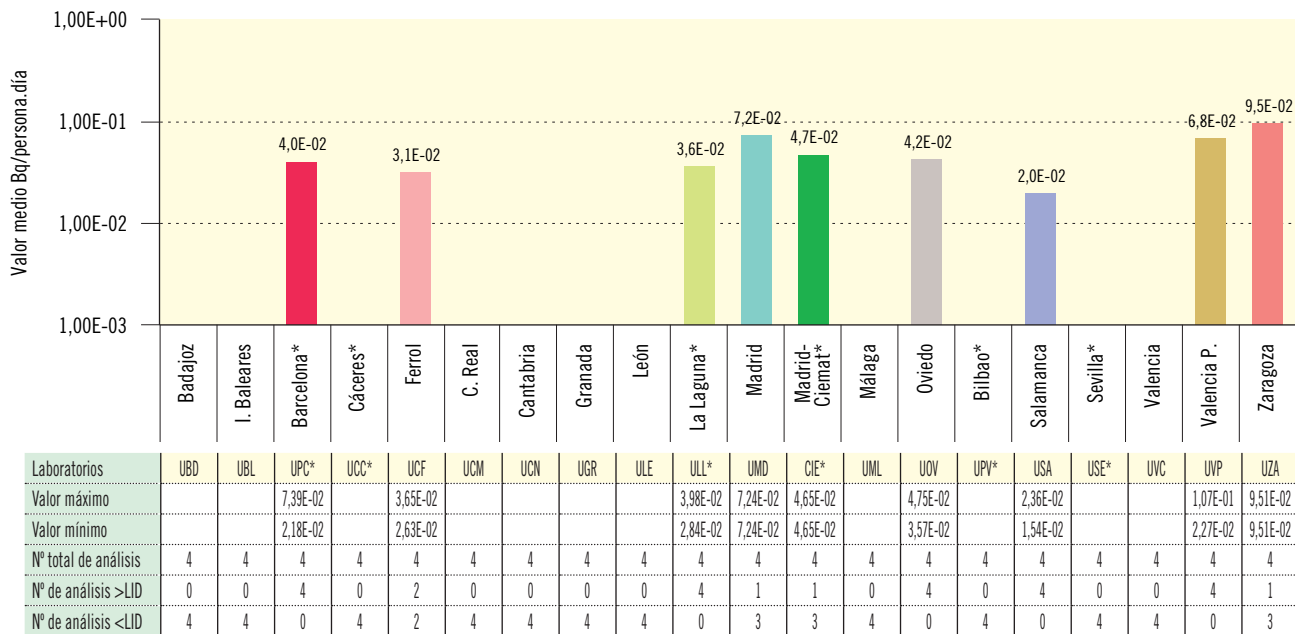
Figura 3.18b. Dieta tipo. Concentración de actividad de Cs-137 (Bq/persona.día) Valores de la campaña 2016
