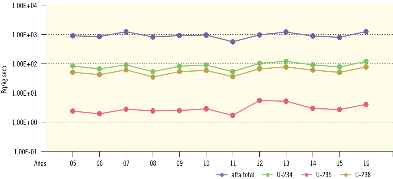
Figura 2.46. Juzbado. Sedimentos de fondo. Valores de concentración de actividad (Bq/kg seco) Evolución temporal valores medios
