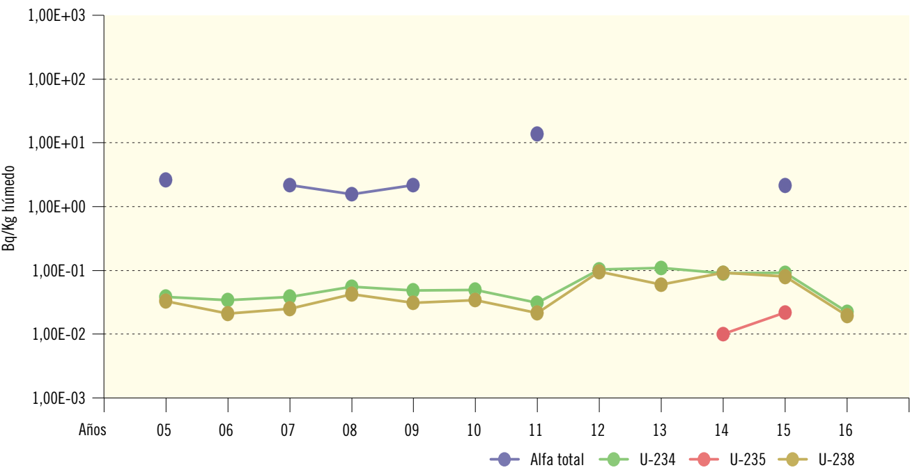
Figura 2.50. Juzbado. Vegetales de hoja no ancha. Valores de concentración de actividad (Bq/Kg húmedo) Evolución temporal valores medios
