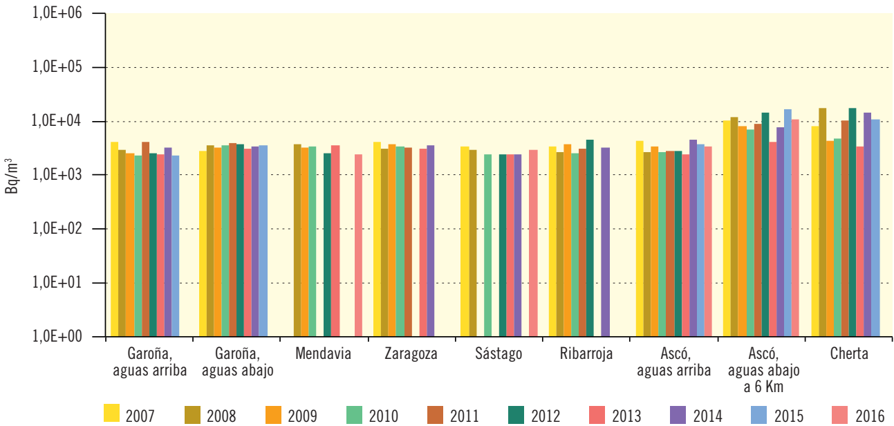
Figura 3.56. Río Ebro Evolución temporal de concentración de actividad de H-3
