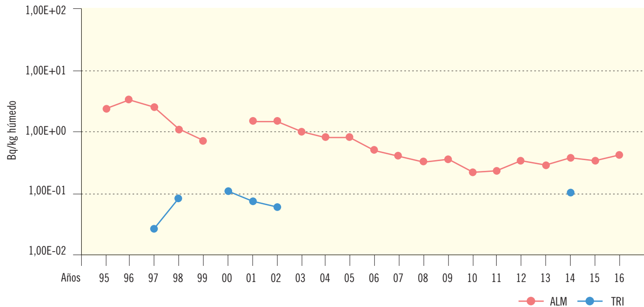
Figura 2.25b. Plantas terrestres. Concentración de actividad (Bq/kg húmedo) Valores de la campaña de 2016
