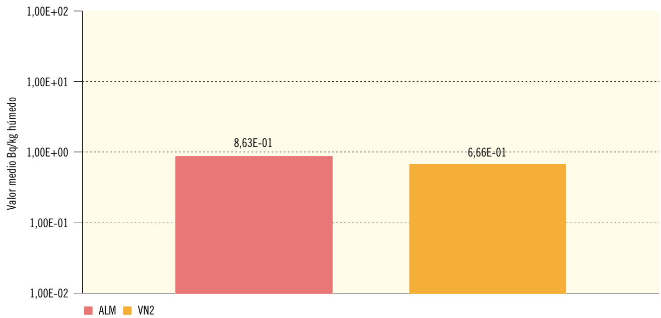
Figura 2.32b. Consumo animal. Concentración de actividad de Sr-90 (Bq/kg húmedo) Valores de la campaña de 2016
