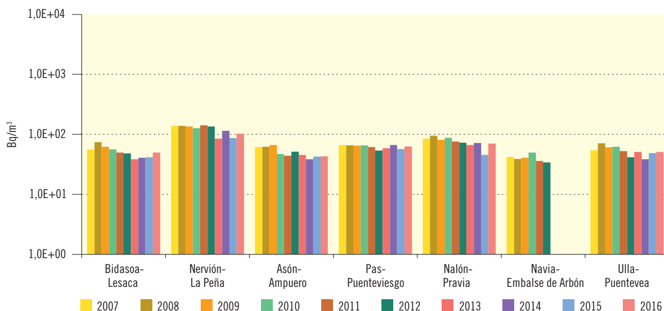
Figura 3.22. Cuencas del norte de España Evolución temporal del índice de actividad beta total
