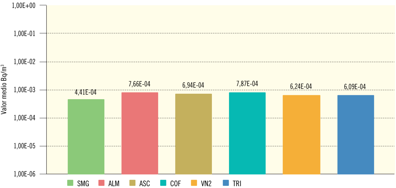
Figura 2.8b. Partículas de polvo en aire. Concentración del índice de actividad beta total (Bq/m³) Valores de la campaña de 2016
