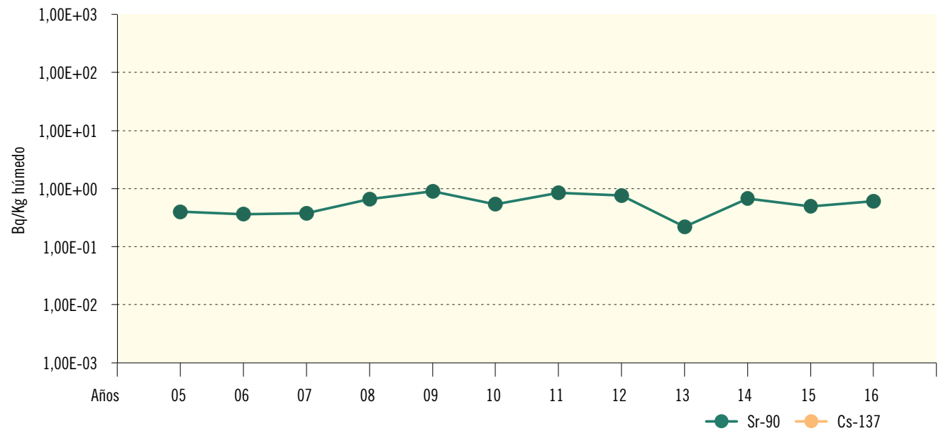
Figura 2.53. El Cabril. Peces. Valores de concentración de actividad (Bq/Kg húmedo) Evolución temporal valores medios
