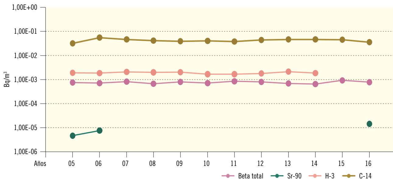
Figura 2.38. El Cabril. Aire. Valores de concentración de actividad (Bq/m 3 )
