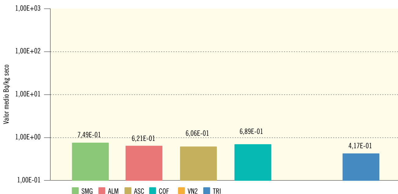
Figura 2.19b. Sedimentos de fondo. Concentración de actividad de Sr-90 (Bq/kg seco) Valores de la campaña de 2016
