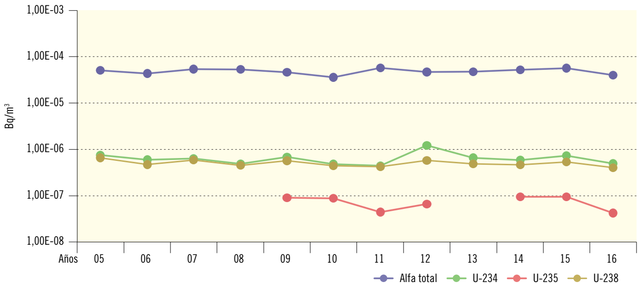
Figura 2.37. Juzbado. Partículas de polvo en aire. Valores de concentración de actividad (Bq/m³) Evolución temporal valores medios
