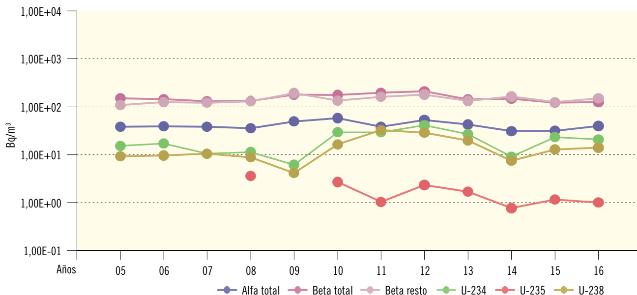
Figura 2.43. Juzbado. Agua superficial. Valores de concentración de actividad (Bq/m 3 ) Evolución temporal valores medios
