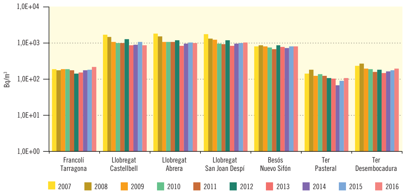
Figura 3.58. Cuencas catalanas Evolución temporal del índice de actividad beta total
