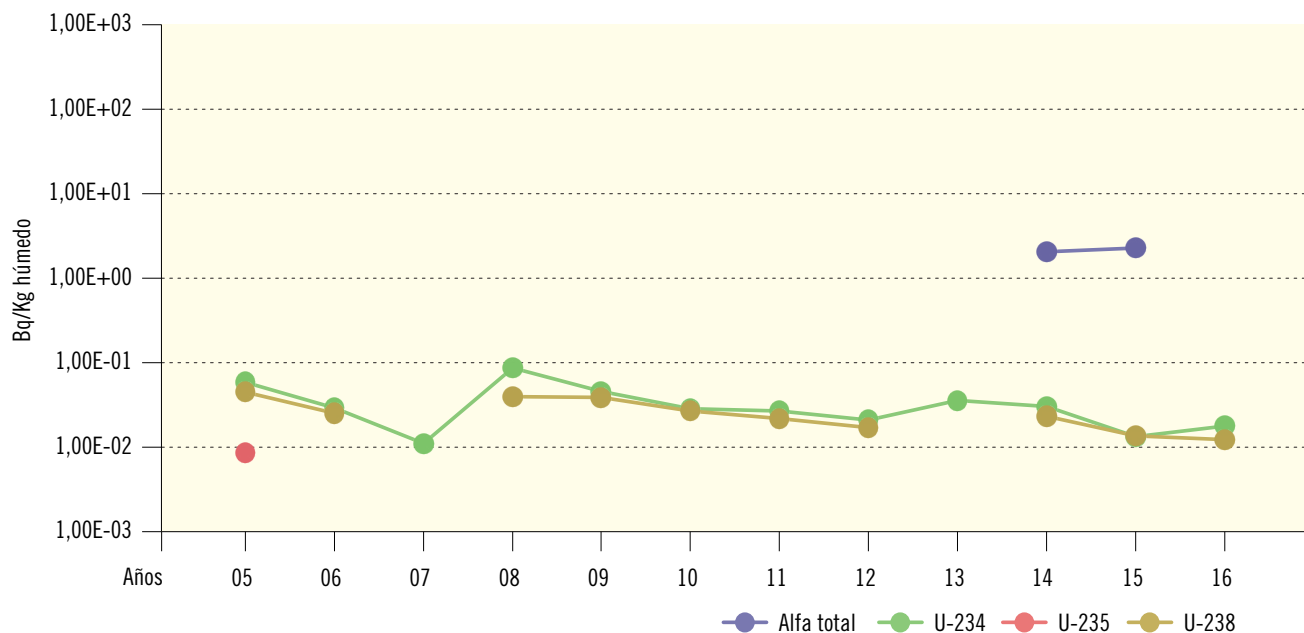
Figura 2.51. Juzbado. Vegetales de hoja ancha. Valores de concentración de actividad (Bq/Kg húmedo) Evolución temporal valores medios
