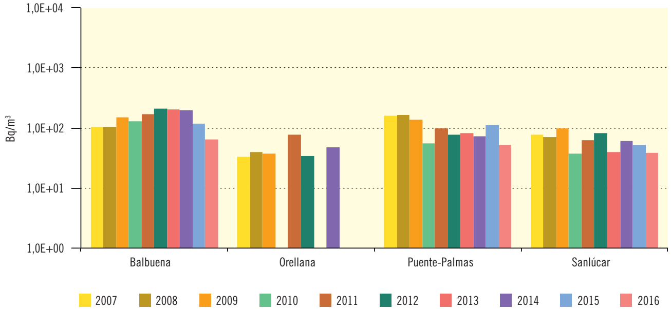
Figura 3.37. Río Guadiana Evolución temporal del índice de actividad alfa total
