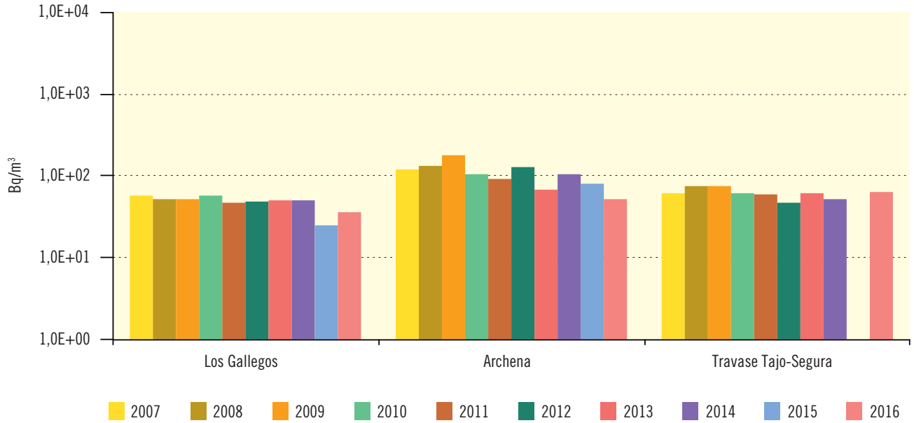
Figura 3.45. Río Segura Evolución temporal del índice de actividad alfa total
