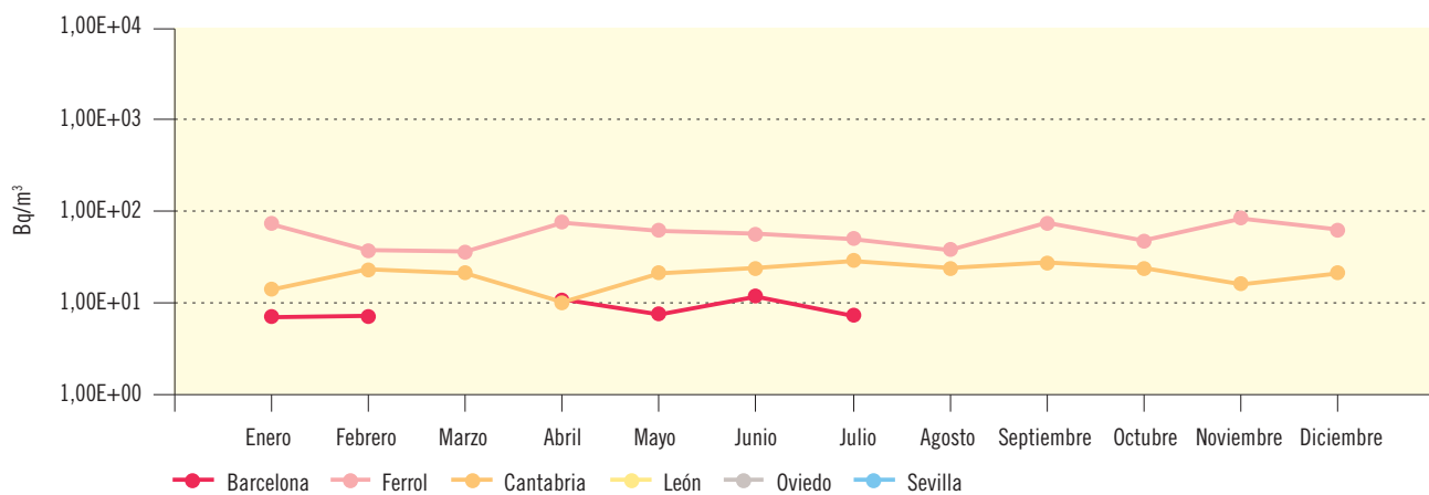
Figura 3.16b. Leche. Concentración de actividad de Cs-137 (Bq/m³)
