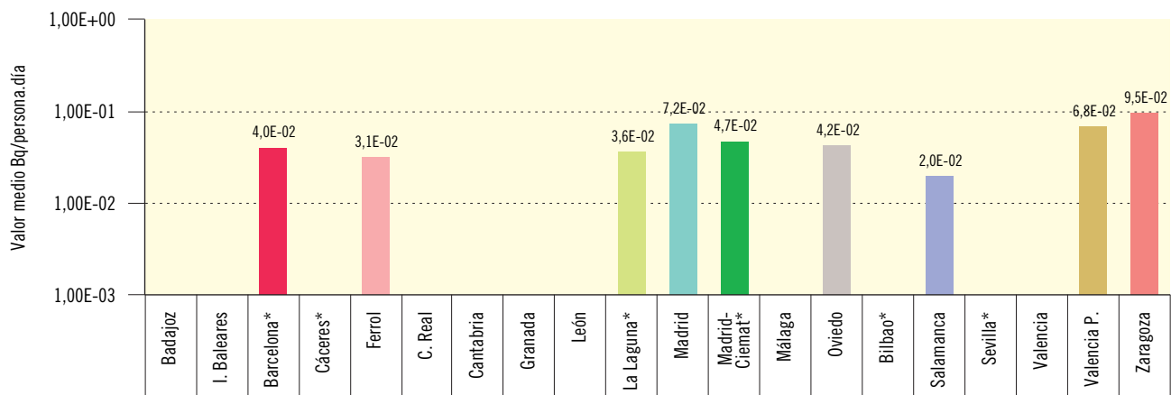
Figura 3.18b. Dieta tipo. Concentración de actividad de Cs-137 (Bq/persona.día)
