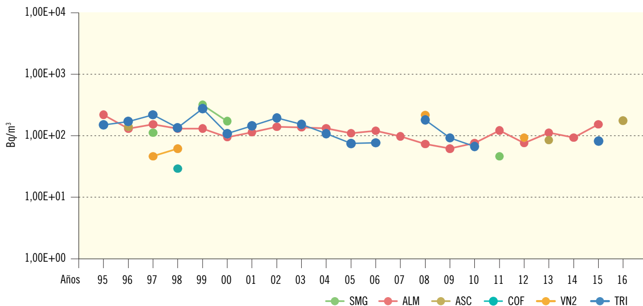
Figura 2.29b. Leche. Concentración de actividad de Cs-137 (Bq/m³)
