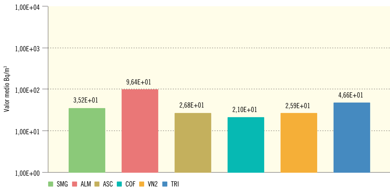
Figura 2.28b. Leche. Concentración de actividad de Sr-90 (Bq/m³)
