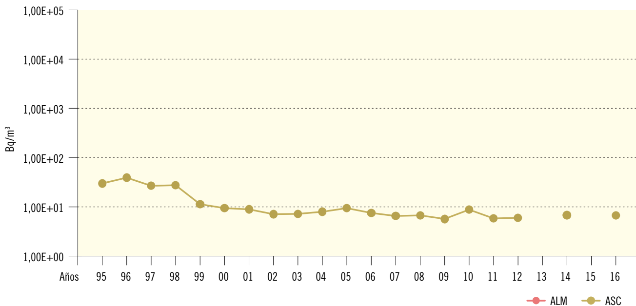
Figura 2.15a. Agua superficial. Evolucion temporal de la concentración de actividad de Sr-90
