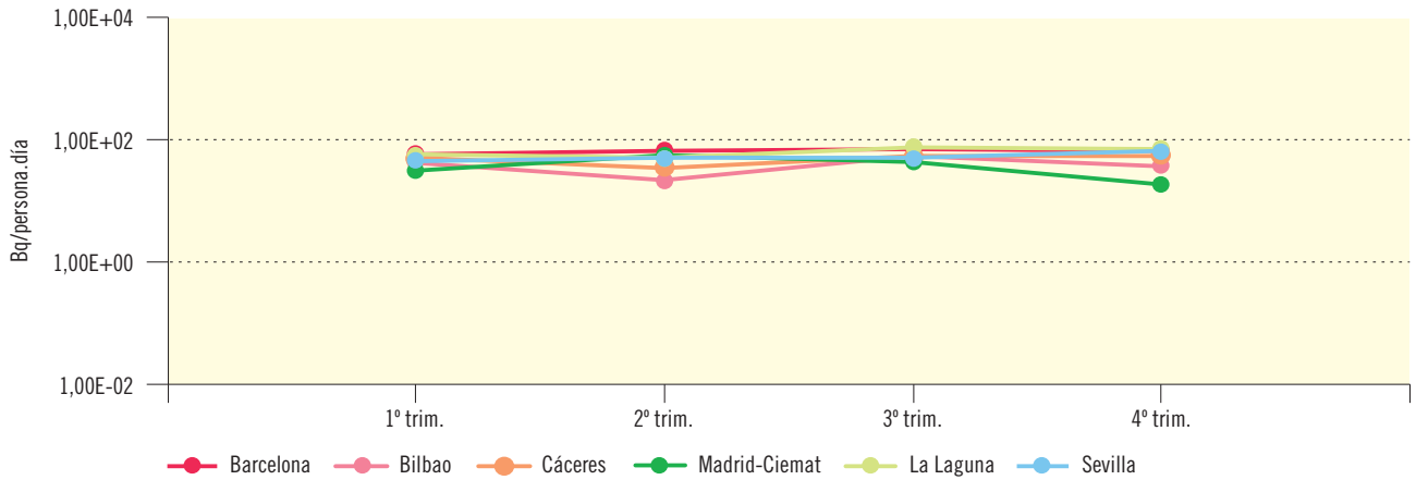
Figura 3.19b. Red de alta sensibilidad. Dieta tipo. Concentración de actividad de C-14 (Bq/persona.día) Valores trimestrales de la campaña de 2016
