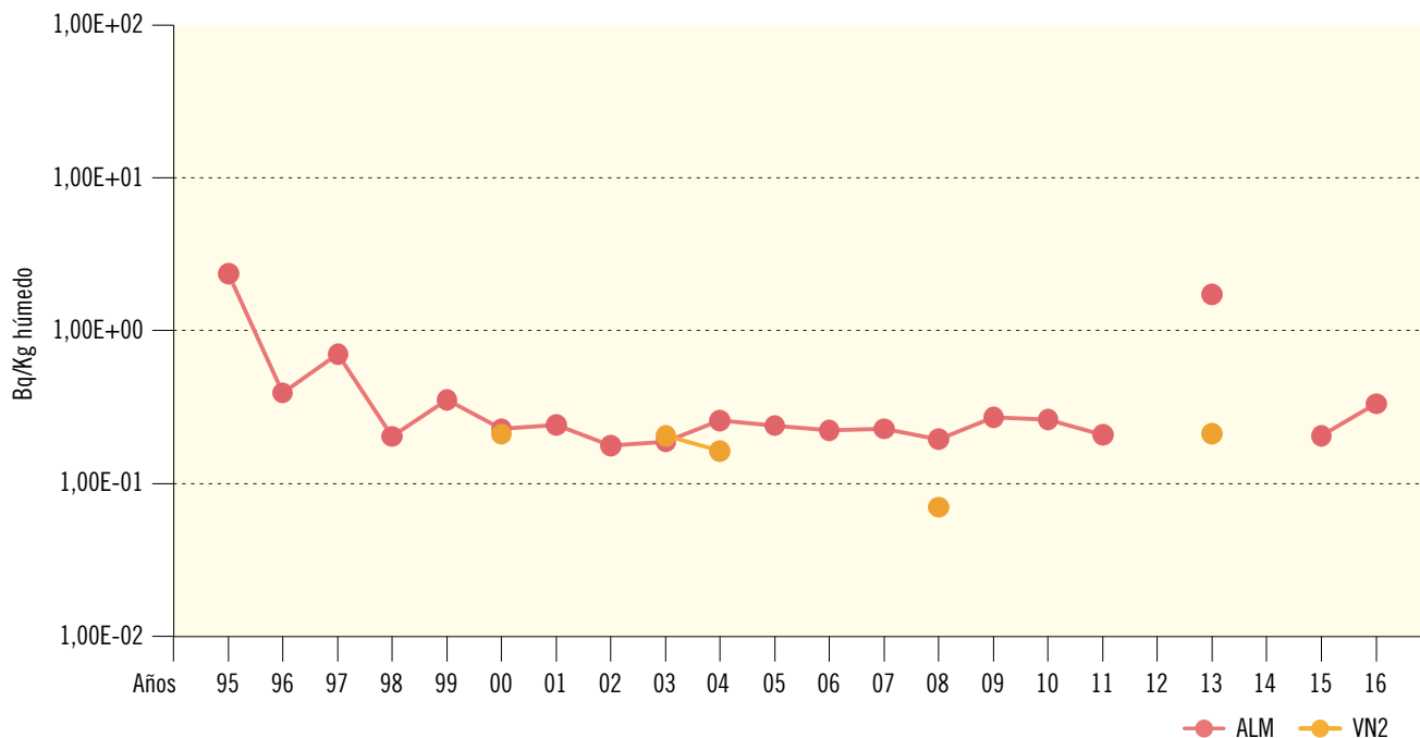
Figura 2.33b. Consumo animal. Concentración de actividad de Cs-137 (Bq/kg húmedo)
