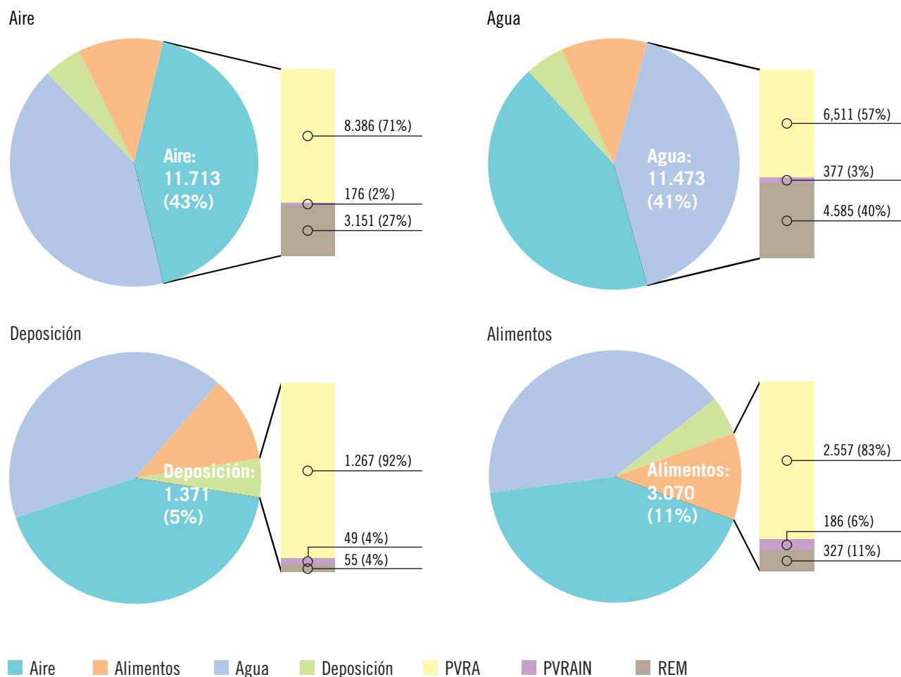
Figura 1.2. Programas de vigilancia radiologica ambiental. Campaña de 2016 Número de análisis realizados en cada vía
