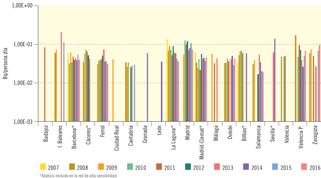
Figura 3.18b. Dieta tipo. Concentración de actividad de Cs-137 (Bq/persona.día)
