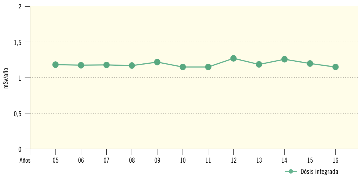
Figura 2.39. Juzbado. Radiación directa. Dosis integrada (DTL, mSv/año) Evolución temporal valores medios
