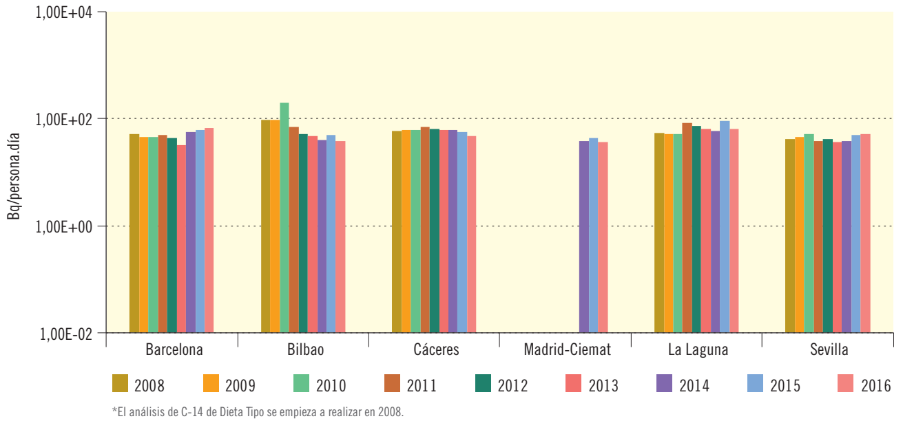
Figura 3.19a. Red de alta sensibilidad. DIETA TIPO Evolución temporal de concentración de actividad de C-14*
