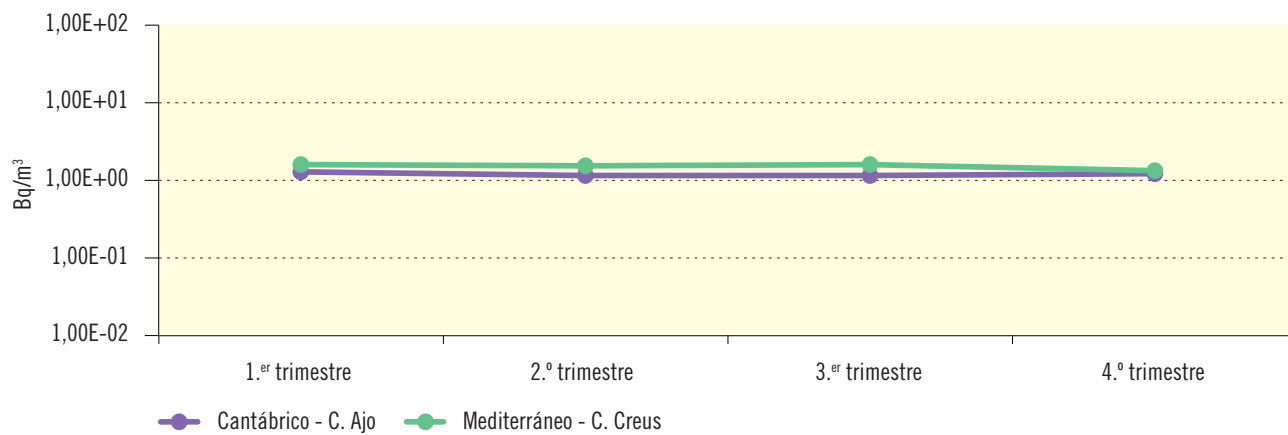
Figura 3.67b. Red de alta sensibilidad. Agua de mar. Concentración de actividad de Cs-137 (Bq/m³)
