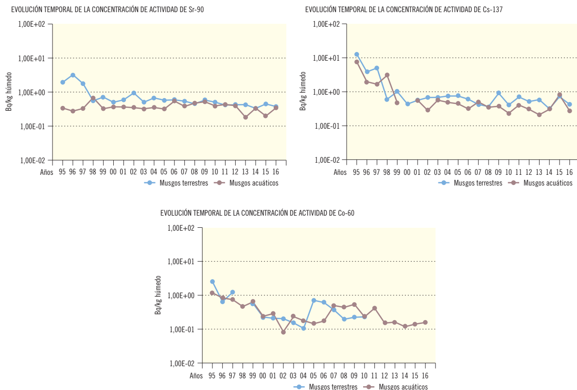
Figura 2.26b. Musgos. CN. STª María de Garoña. Concentración de actividad (Bq/kg húmedo) Valores de la campaña de 2016
