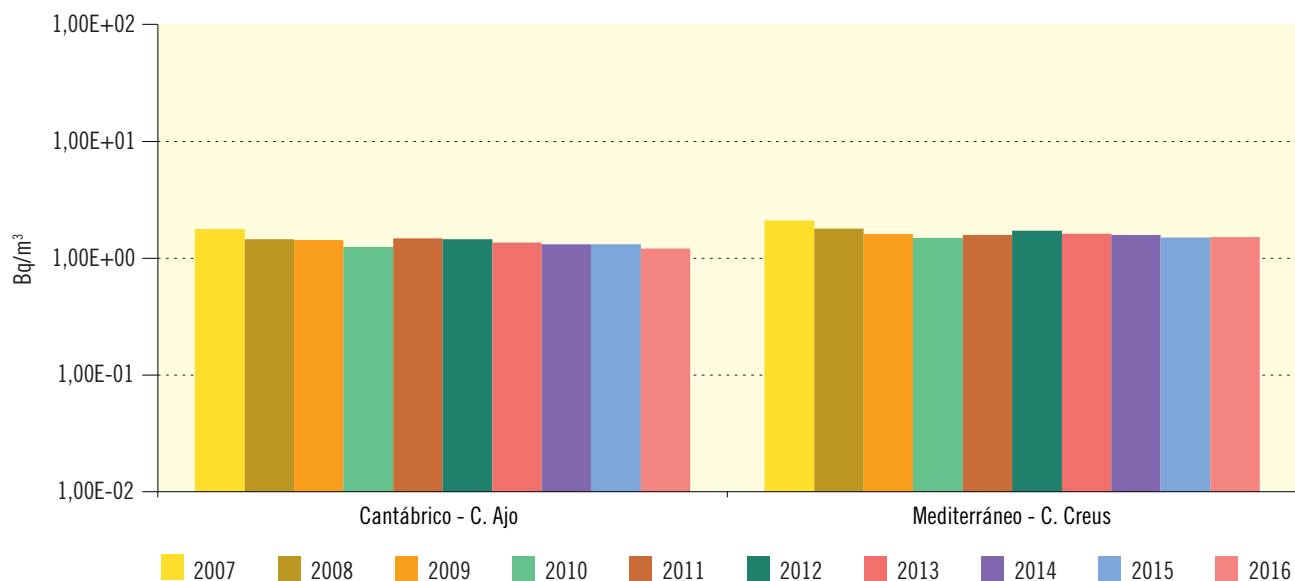
Figura 3.67a. Red de alta sensibilidad. Agua de mar
