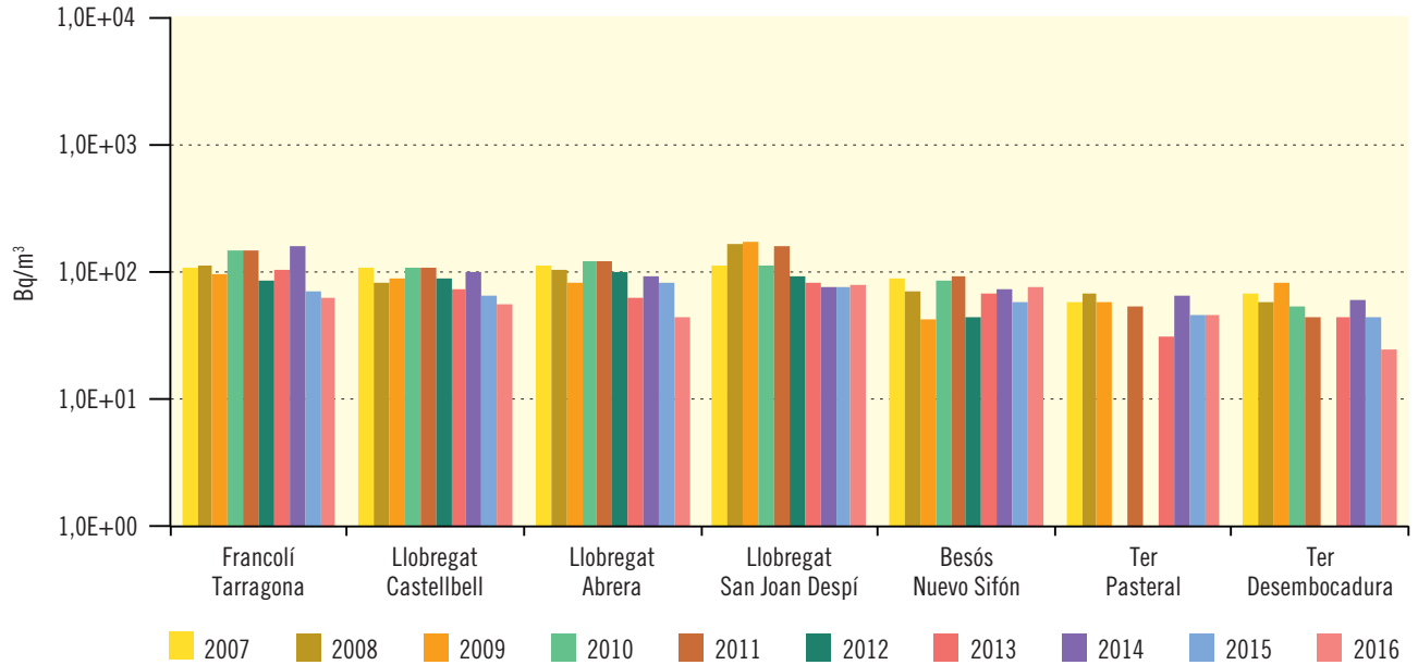
Figura 3.57. Cuencas catalanas Evolución temporal del índice de actividad alfa total
