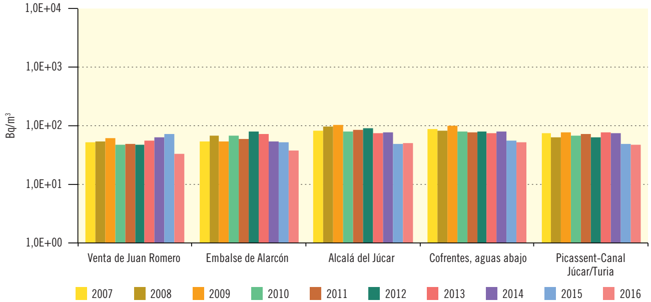
Figura 3.49. Río Júcar Evolución temporal del índice de actividad alfa total
