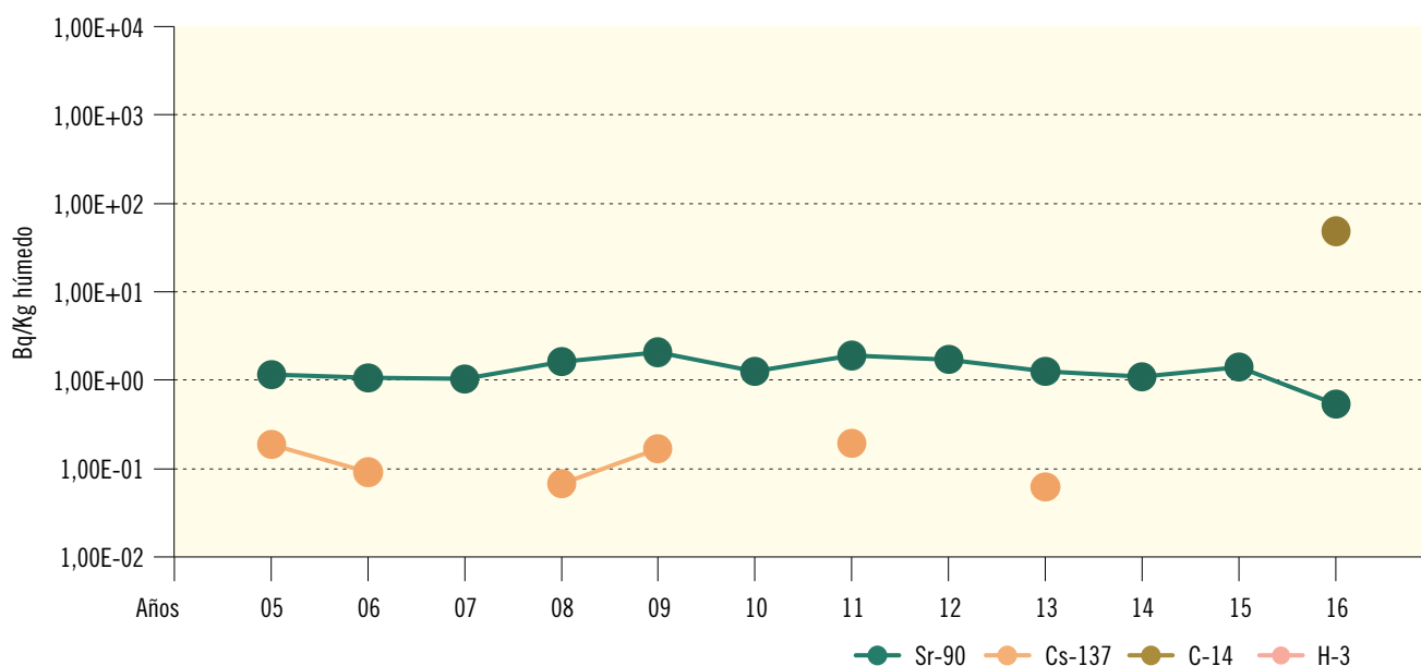
Figura 2.54. El Cabril. Plantas Terrestres. Valores de concentración de actividad (Bq/Kg húmedo) Evolución temporal valores medios
