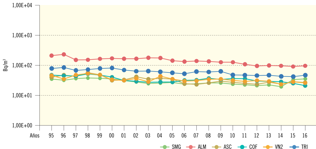
Figura 2.28b. Leche. Concentración de actividad de Sr-90 (Bq/m³)
