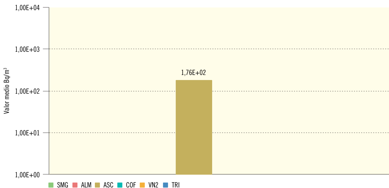
Figura 2.29b. Leche. Concentración de actividad de Cs-137 (Bq/m³)
