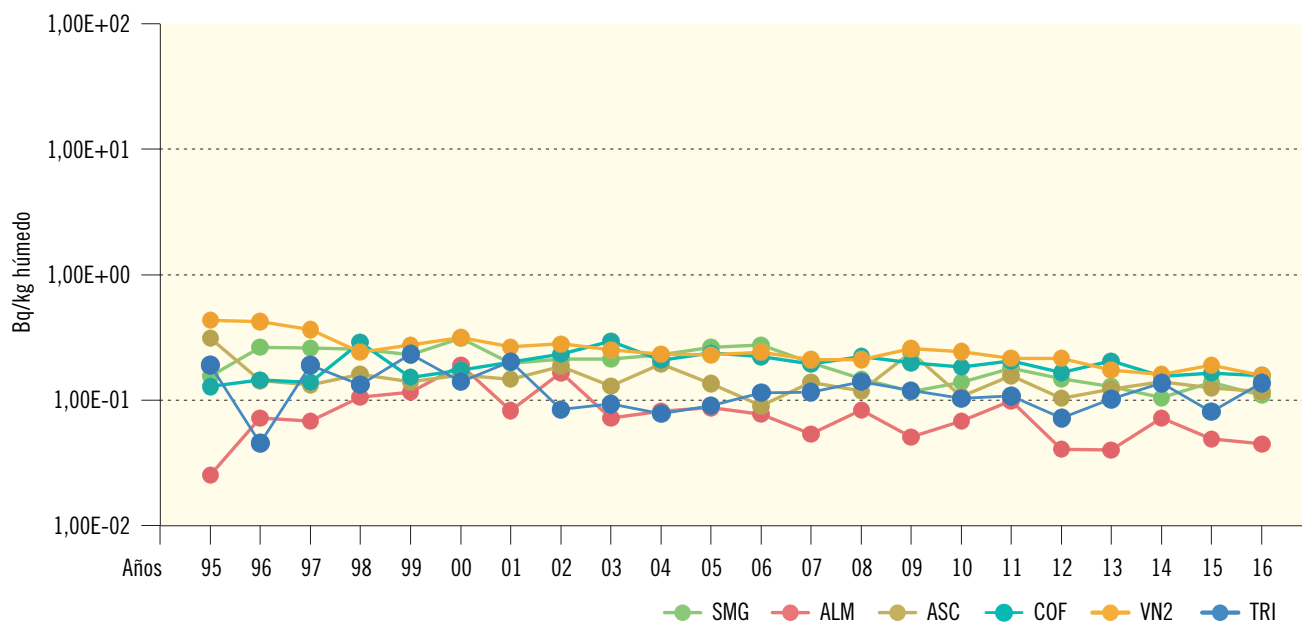
Figura 2.31b. Vegetales de hoja no ancha. Concentración de actividad de Sr-90 (Bq/kg húmedo)
