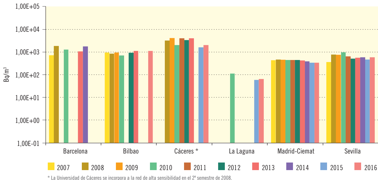
Figura 3.14a. Red de alta sensibilidad. Agua potable.
