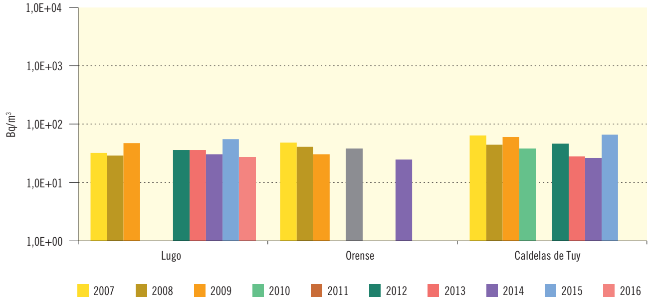
Figura 3.25. Río Miño Evolución temporal del índice de actividad alfa total
