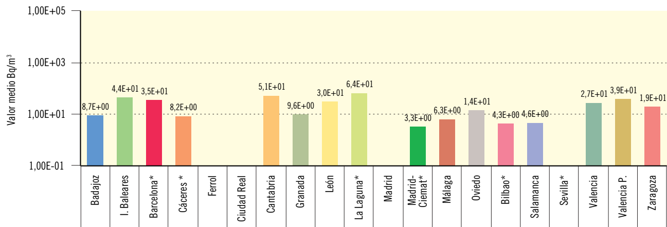
Figura 3.10b. Agua potable. Concentración del índice de actividad de alfa total (Bq/m³)
