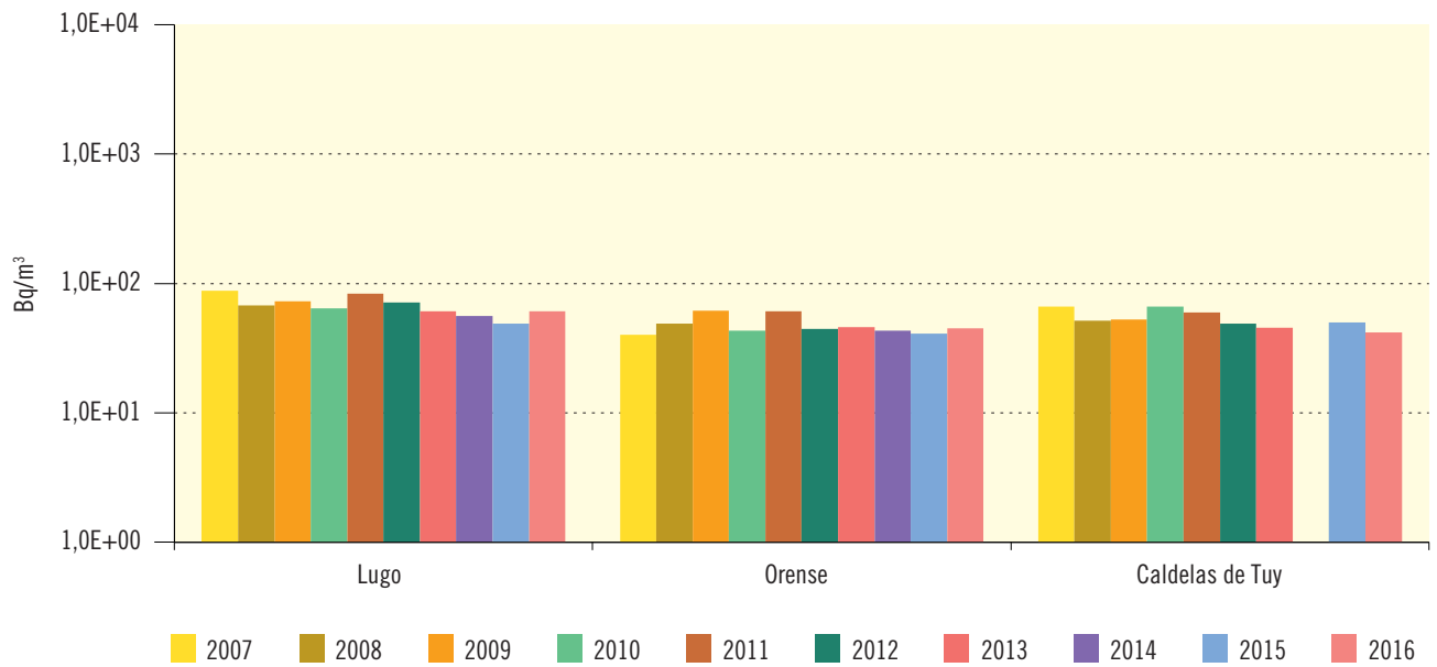
Figura 3.26. Río Miño Evolución temporal del índice de actividad beta total
