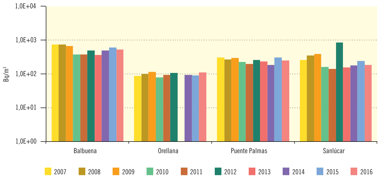
Figura 3.38. Río Guadiana Evolución temporal del índice de actividad beta total
