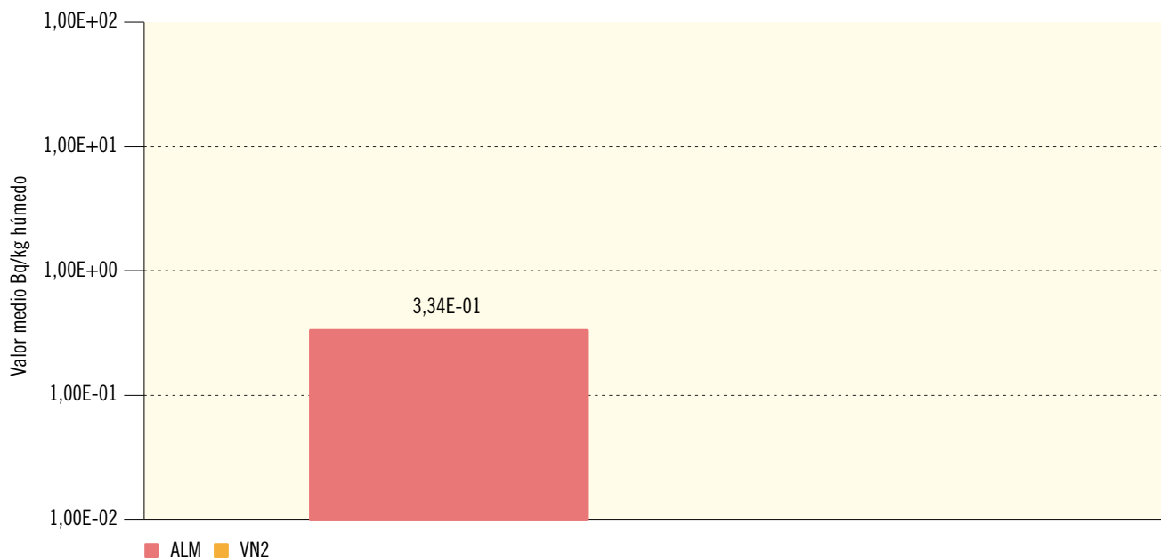
Figura 2.33b. Consumo animal. Concentración de actividad de Cs-137 (Bq/kg húmedo)
