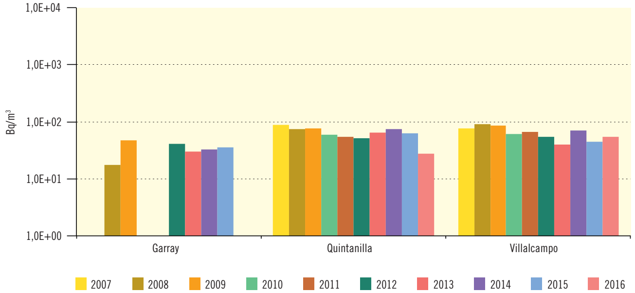
Figura 3.29. Río Duero Evolución temporal del índice de actividad alfa total
