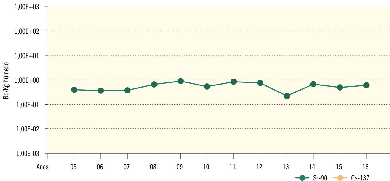
Figura 2.53. El Cabril. Peces. Valores de concentración de actividad (Bq/Kg húmedo) Evolución temporal valores medios
