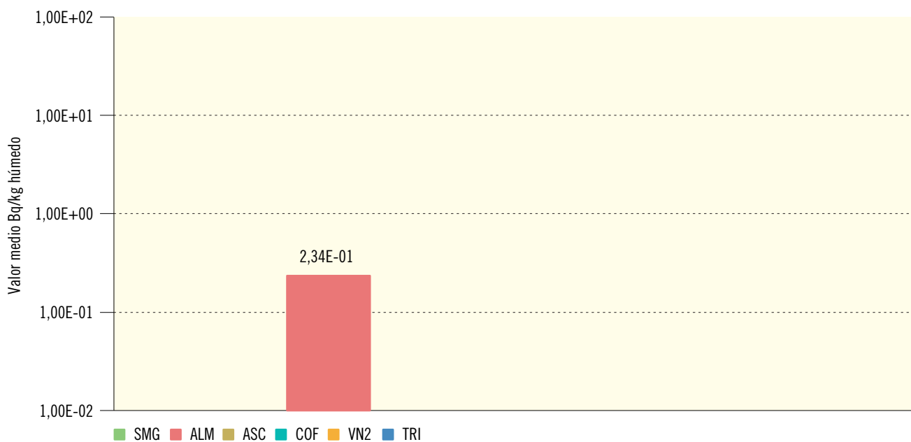
Figura 2.34b. Carne y aves. Concentración de actividad de Cs-137 (Bq/kg húmedo) Valores de la campaña de 2016
