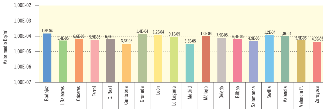
Figura 3.2b. Partículas de polvo en aire. Concentración del índice de actividad alfa total (Bq/m³) Valores de la campaña de 2016
