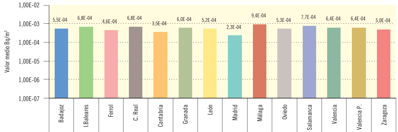
Figura 3.3b. Partículas de polvo en aire. Concentración del índice de actividad beta total (Bq/m³) Valores de la campaña de 2016
