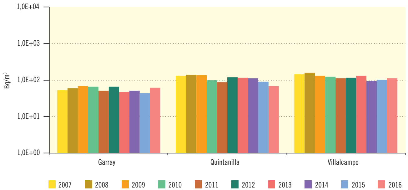
Figura 3.30. Río Duero Evolución temporal del índice de actividad beta total
