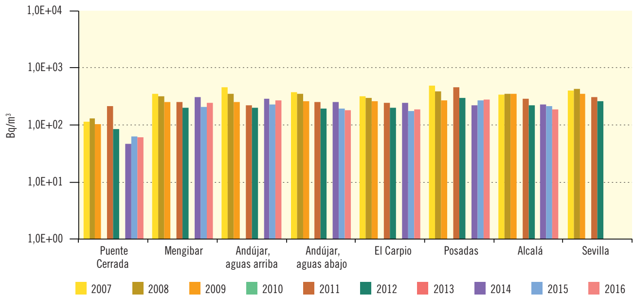
Figura 3.42. Río Guadalquivir Evolución temporal del índice de actividad beta total
