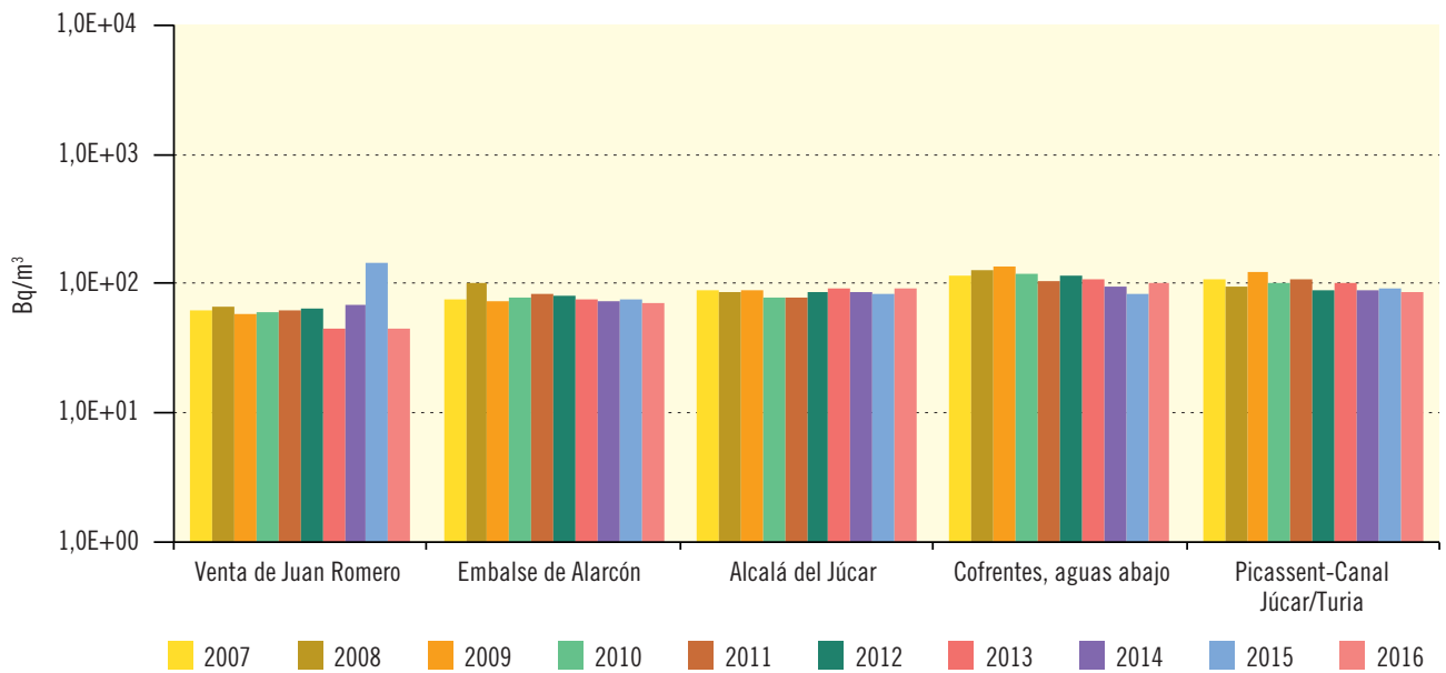
Figura 3.50. Río Júcar Evolución temporal del índice de actividad beta total
