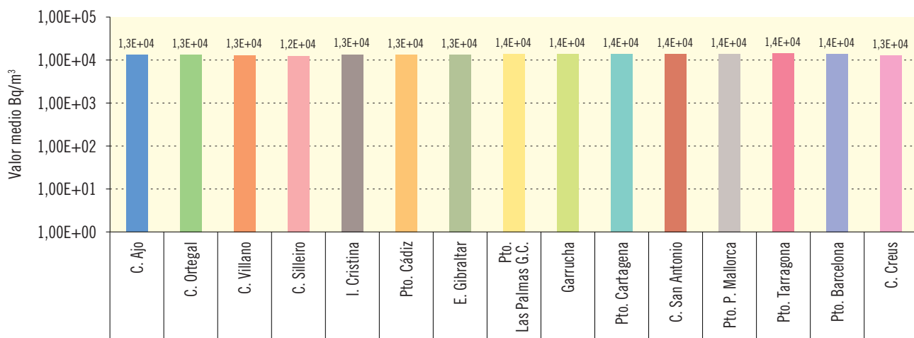
Figura 3.64b. Agua de mar. Concentración del índice de actividad beta total (Bq/m³)
