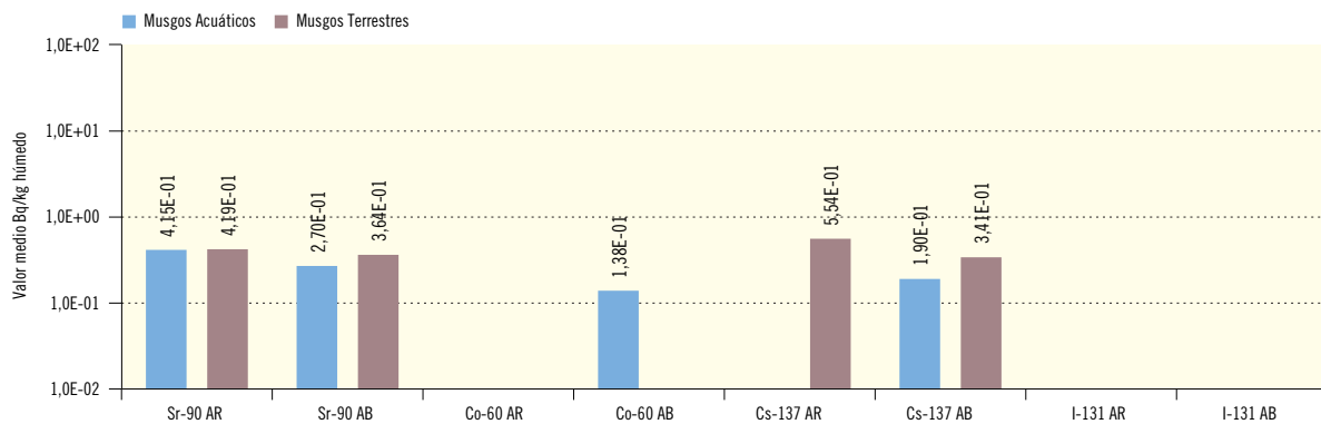
Figura 2.26b. Musgos. CN. STª María de Garoña. Concentración de actividad (Bq/kg húmedo) Valores de la campaña de 2016
