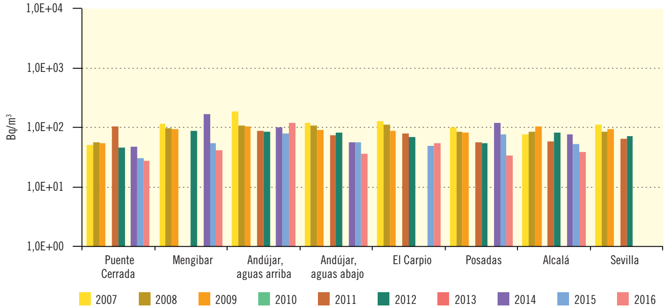
Figura 3.41. Río Guadalquivir Evolución temporal del índice de actividad alfa total
