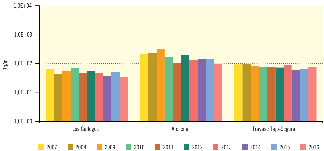
Figura 3.46. Río Segura Evolución temporal del índice de actividad beta total
