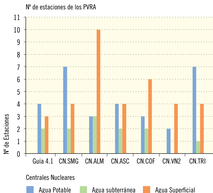
Figura 2.5. Número de estaciones de muestreo en los PVRA de las centrales nucleares. Año 2016
