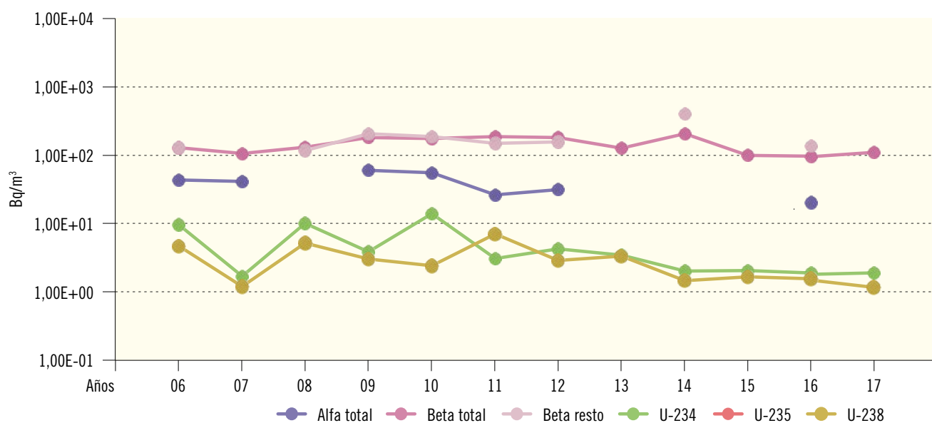
Figura 2.45. Juzbado. Agua potable. Valores de concentración de actividad (Bq/m 3 ) Evolución temporal valores medios
