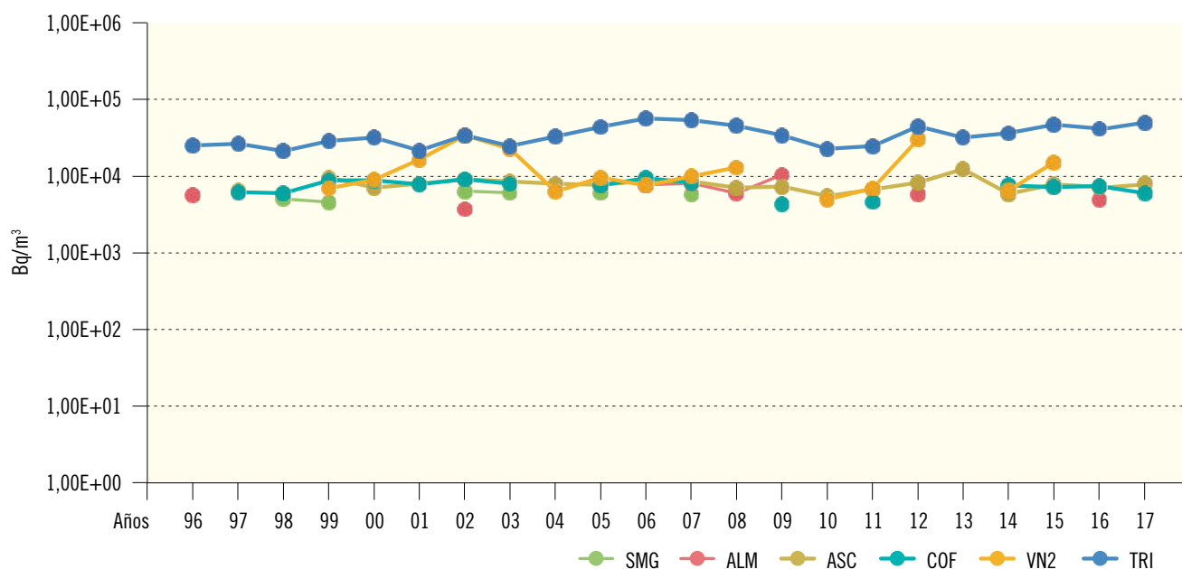
Figura 2.18b. Agua potable. Concentración de actividad de H-3 (Bq/m³)
