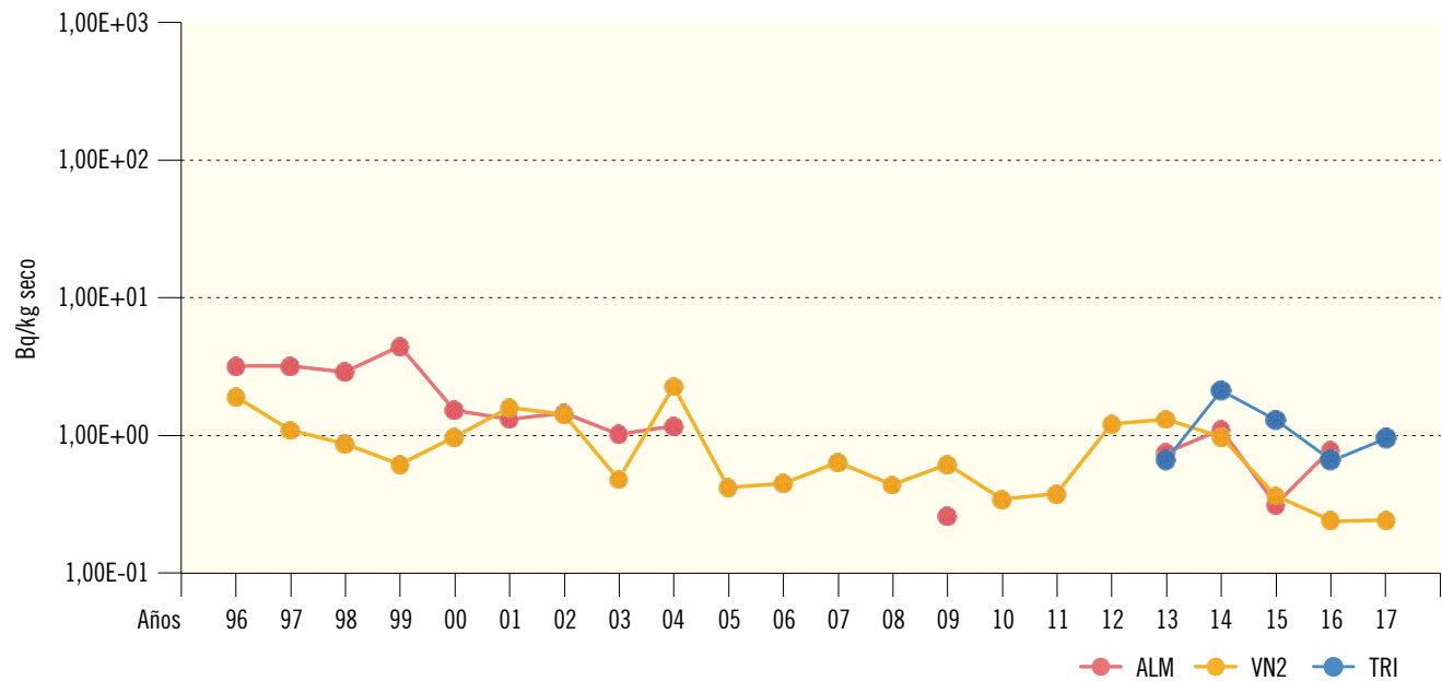
Figura 2.23a. Sedimentos de orilla. Evolución temporal de la concentración de actividad de Cs-137 Valores medios en la zona vigilada
