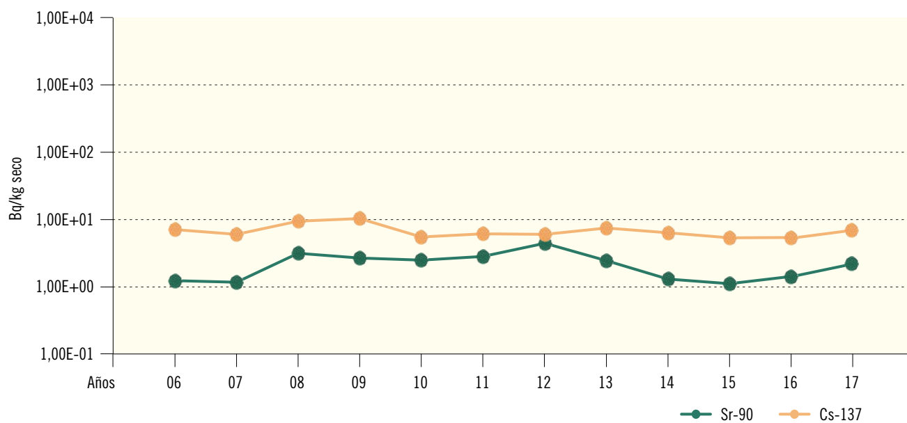
Figura 2.42. El Cabril. Suelo. Valores de concentración de actividad (Bq/kg seco)
