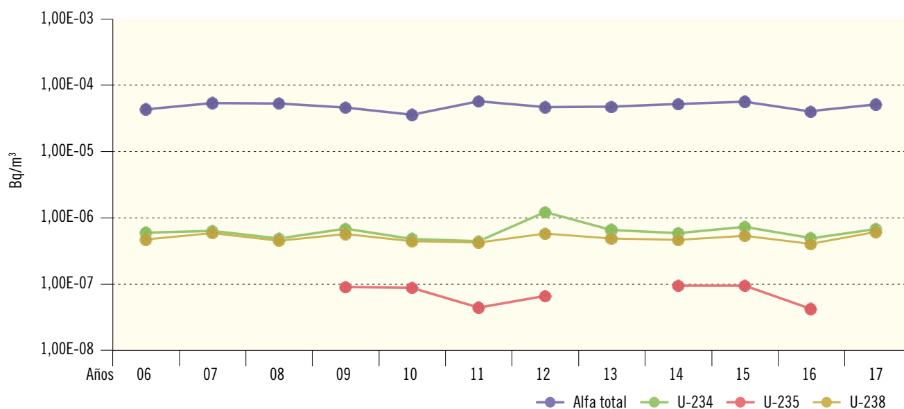
Figura 2.37. Juzbado. Partículas de polvo en aire. Valores de concentración de actividad (Bq/m³)
