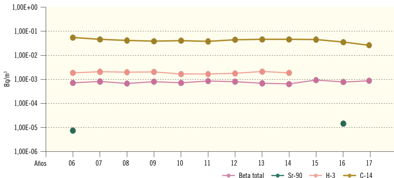
Figura 2.38. El Cabril. Aire. Valores de concentración de actividad (Bq/m³)
