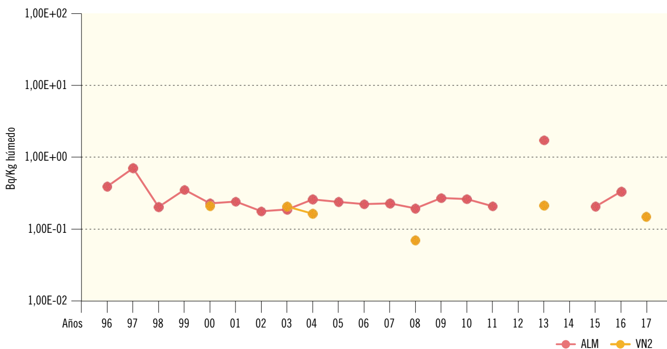
Figura 2.34b. Consumo animal. Concentración de actividad de Cs-137 (Bq/kg húmedo)
