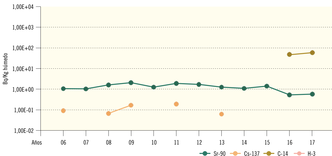
Figura 2.54. El Cabril. Plantas Terrestres. Valores de concentración de actividad (Bq/Kg húmedo)
