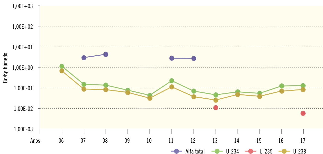
Figura 2.52. Juzbado. Peces. Valores de concentración de actividad (Bq/Kg húmedo)
