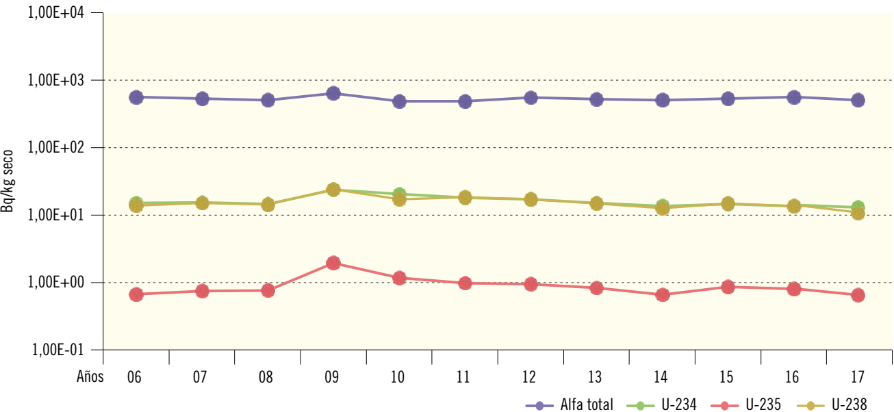
Figura 2.41. Juzbado. Suelo. Valores de concentración de actividad (Bq/kg seco) Evolución temporal valores medios
