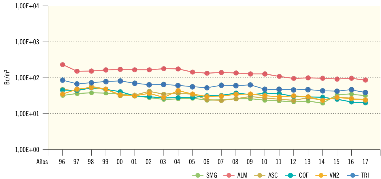
Figura 2.29a. Leche. Evolución temporal de la concentración de actividad de Sr-90 Valores medios en la zona vigilada
