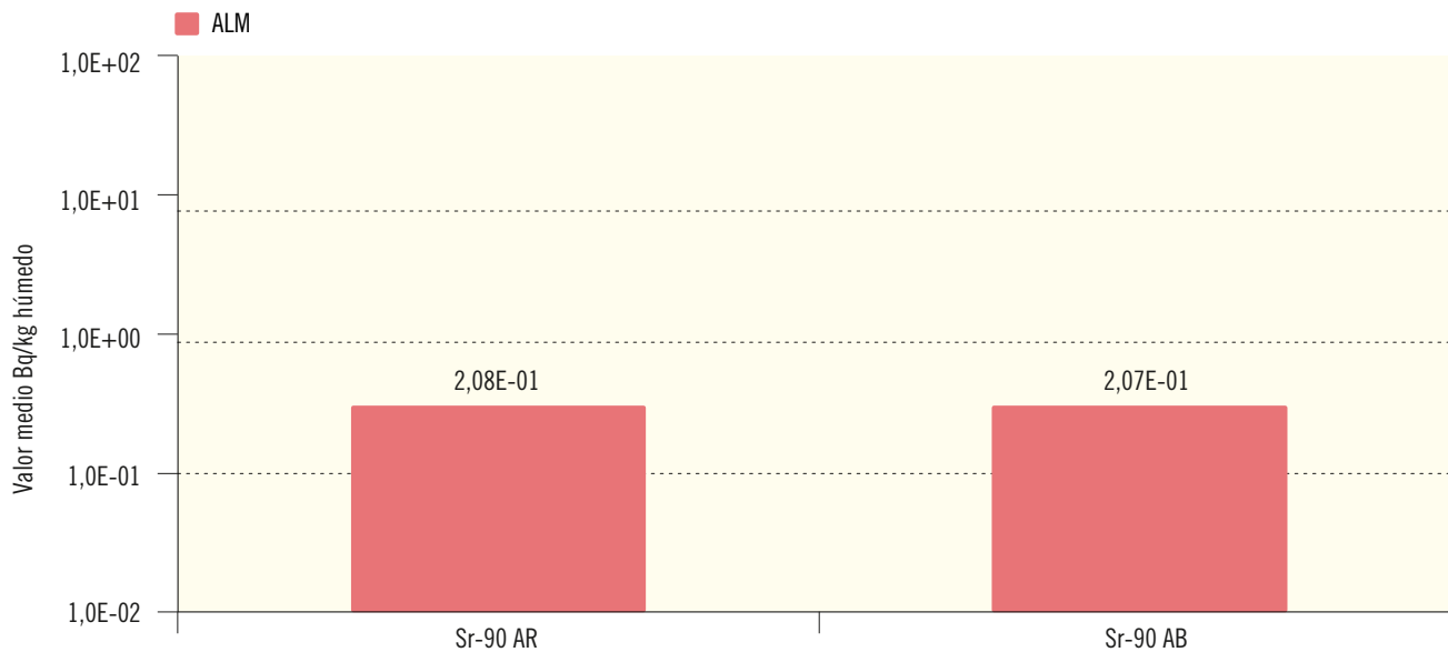
Figura 2.26b. Plantas terrestres. Concentración de actividad (Bq/kg húmedo)
