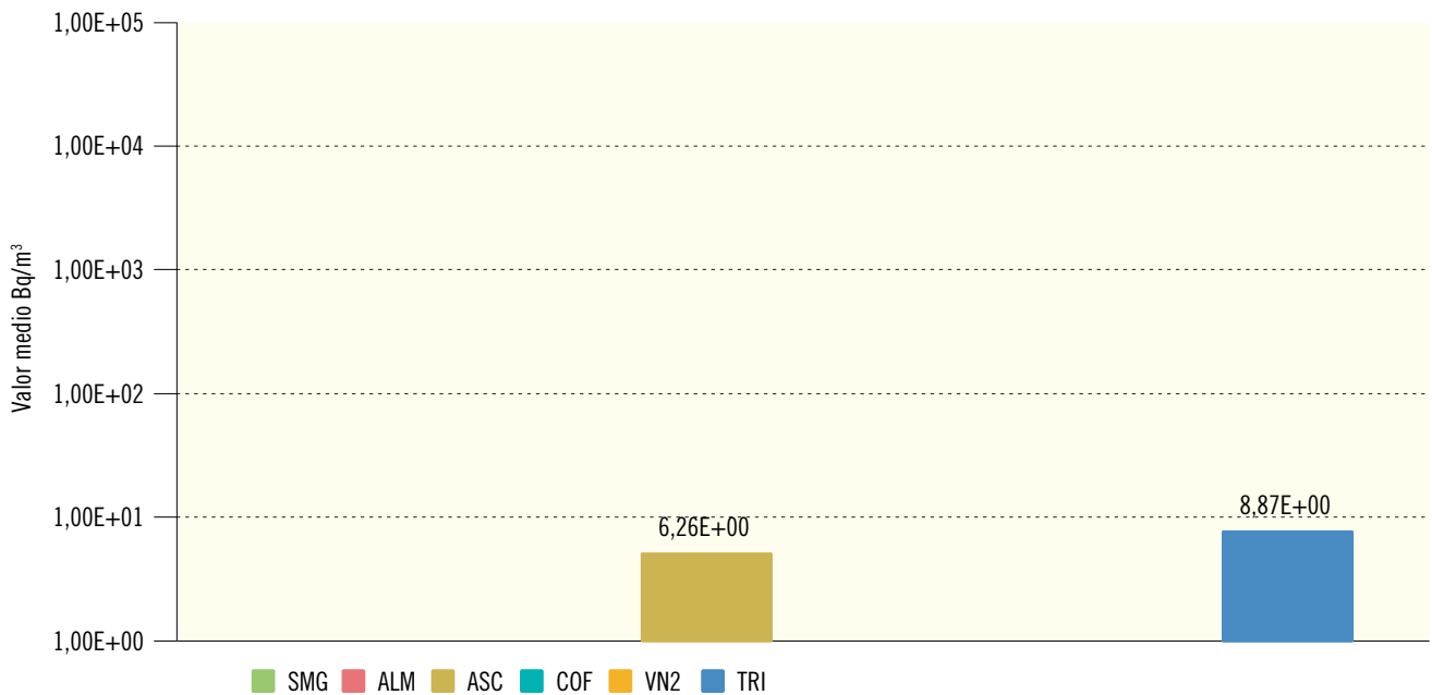
Figura 2.19b. Agua potable. Concentración de actividad de Sr-90 (Bq/m³) Valores de la campaña de 2017
