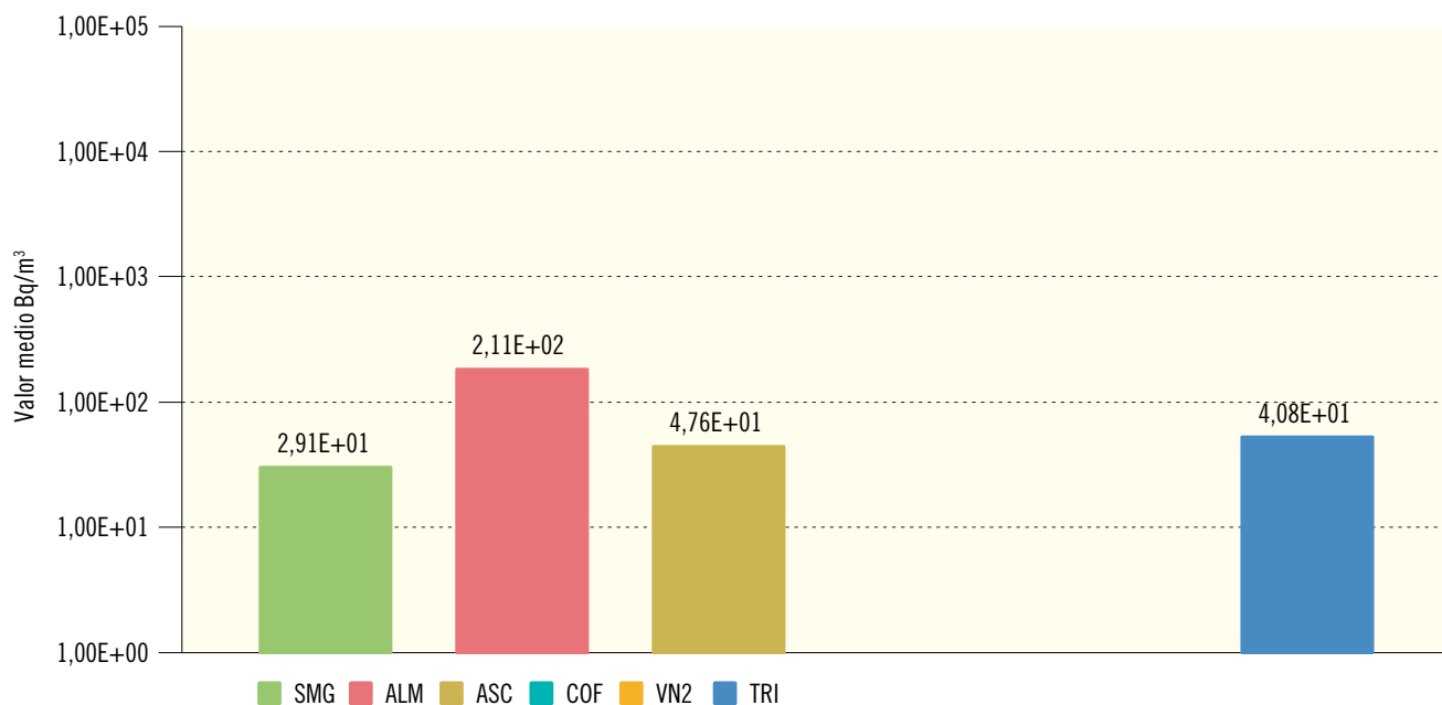
Figura 2.17b. Agua potable. Concentración del índice de actividad beta resto (Bq/m³)
