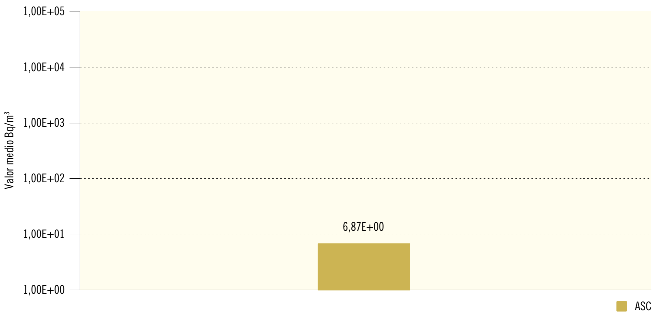
Figura 2.15b. Agua superficial. Concentración de actividad de Sr-90 (Bq/m³) Valores de la campaña de 2017
