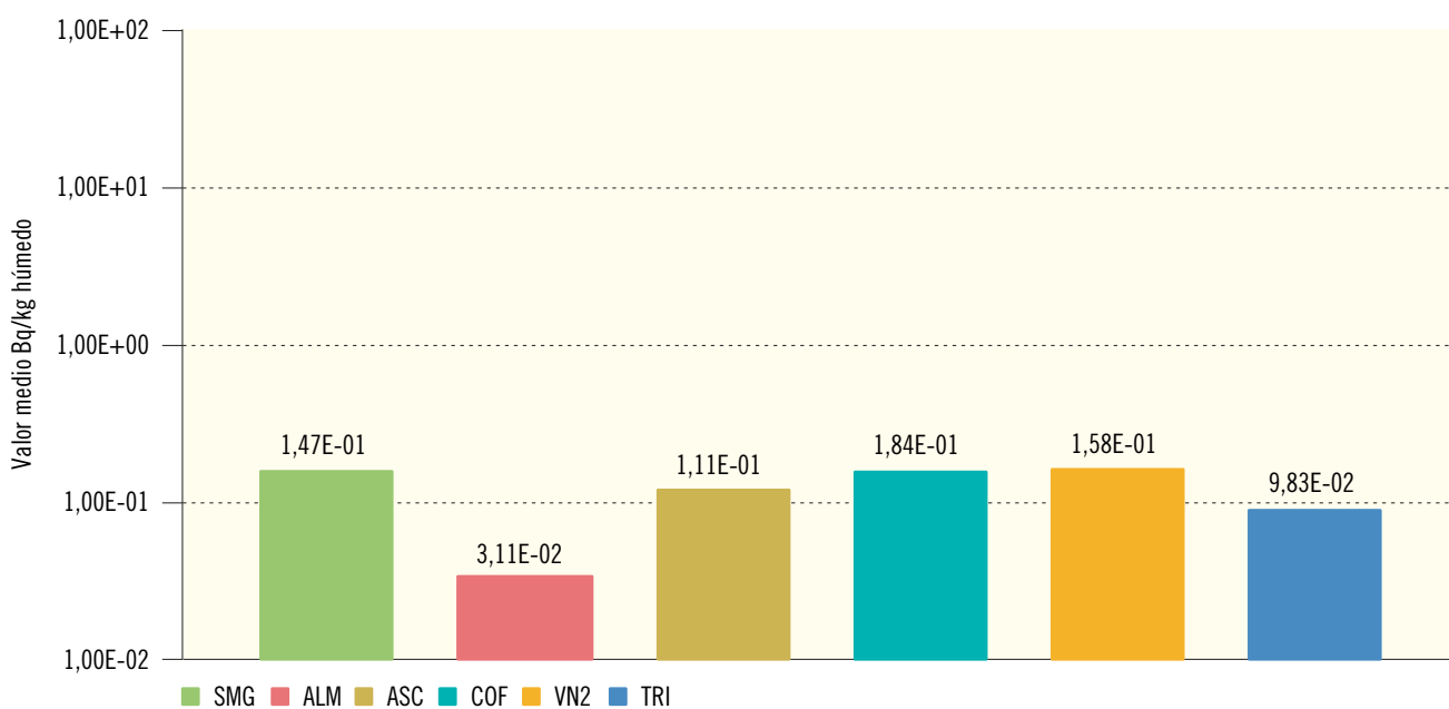
Figura 2.32b. Vegetales de hoja no ancha. Concentración de actividad de Sr-90 (Bq/kg húmedo)
