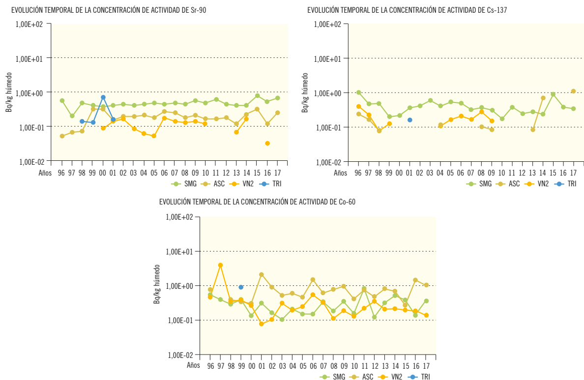
Figura 2.24b. Plantas acuáticas. Concentración de actividad (Bq/kg húmedo)
