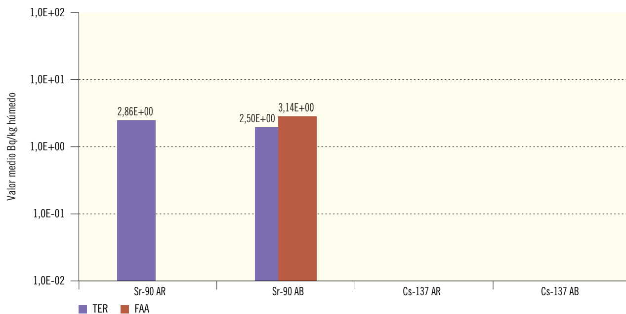
Figura 2.28b. Fauna terrestre y acuática. CN. STª María de Garoña. Concentración de actividad (Bq/kg húmedo)
