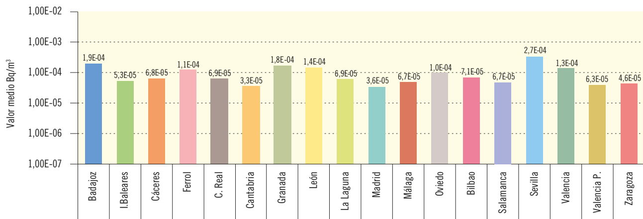
Figura 3.2b. Partículas de polvo en aire. Concentración del índice de actividad alfa total (Bq/m³)
