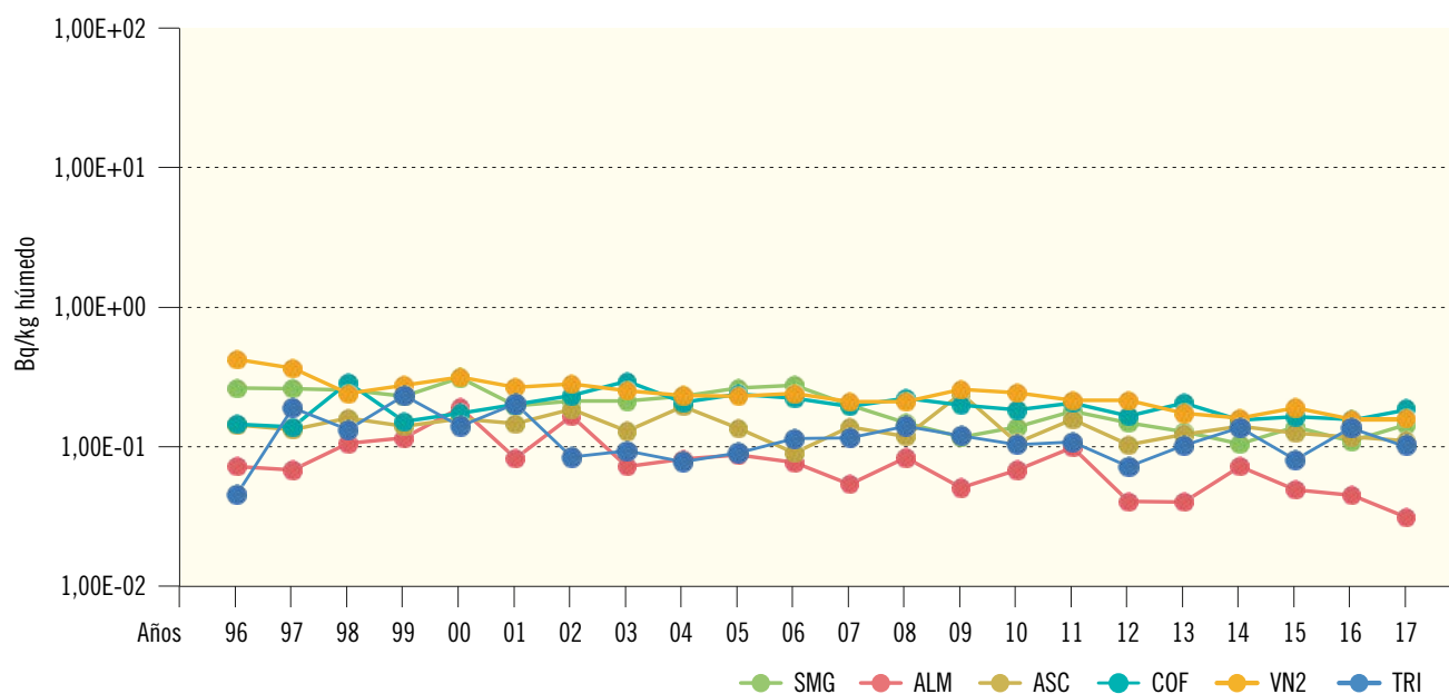
Figura 2.32b. Vegetales de hoja no ancha. Concentración de actividad de Sr-90 (Bq/kg húmedo)
