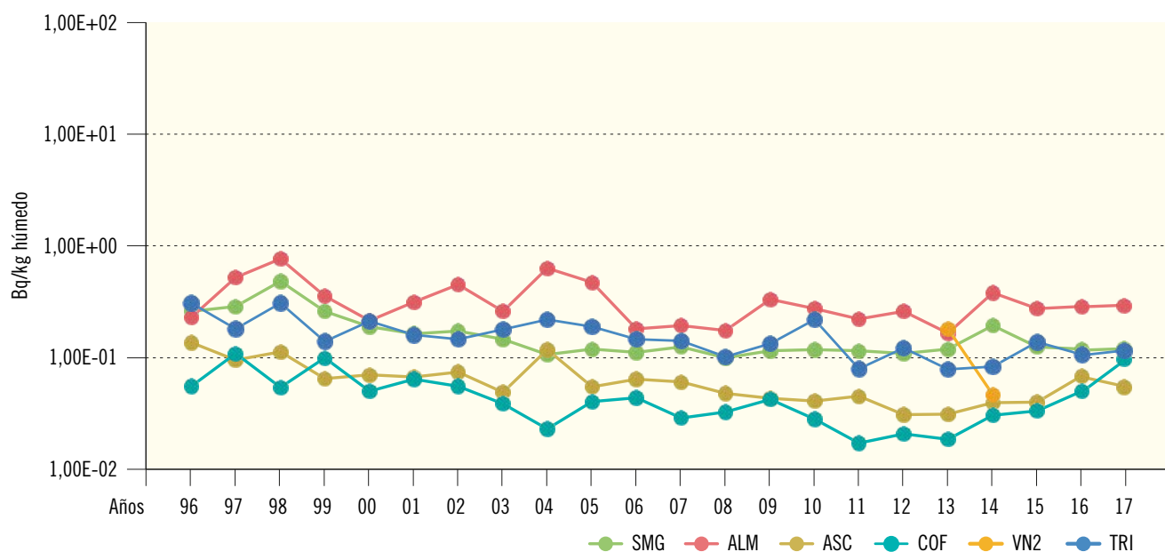
Figura 2.31b. Vegetales de hoja ancha. Concentración de actividad de Sr-90 (Bq/kg húmedo)
