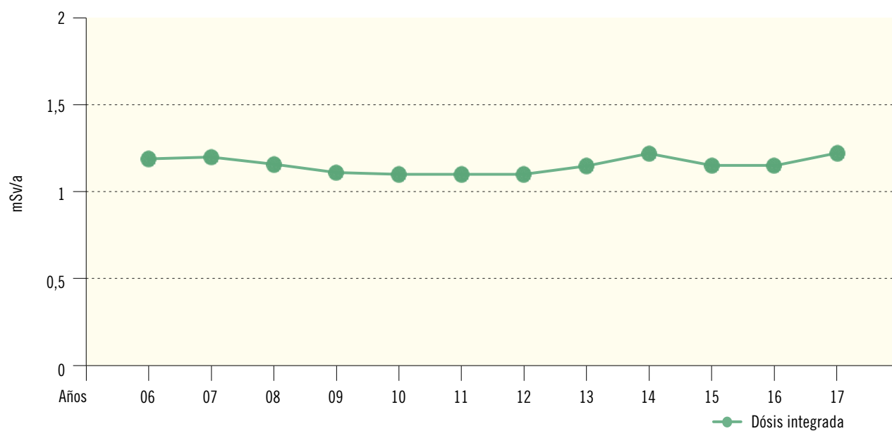
Figura 2.40. El Cabril. Radiación directa. Dosis integrada (DTL, mSv/año)
